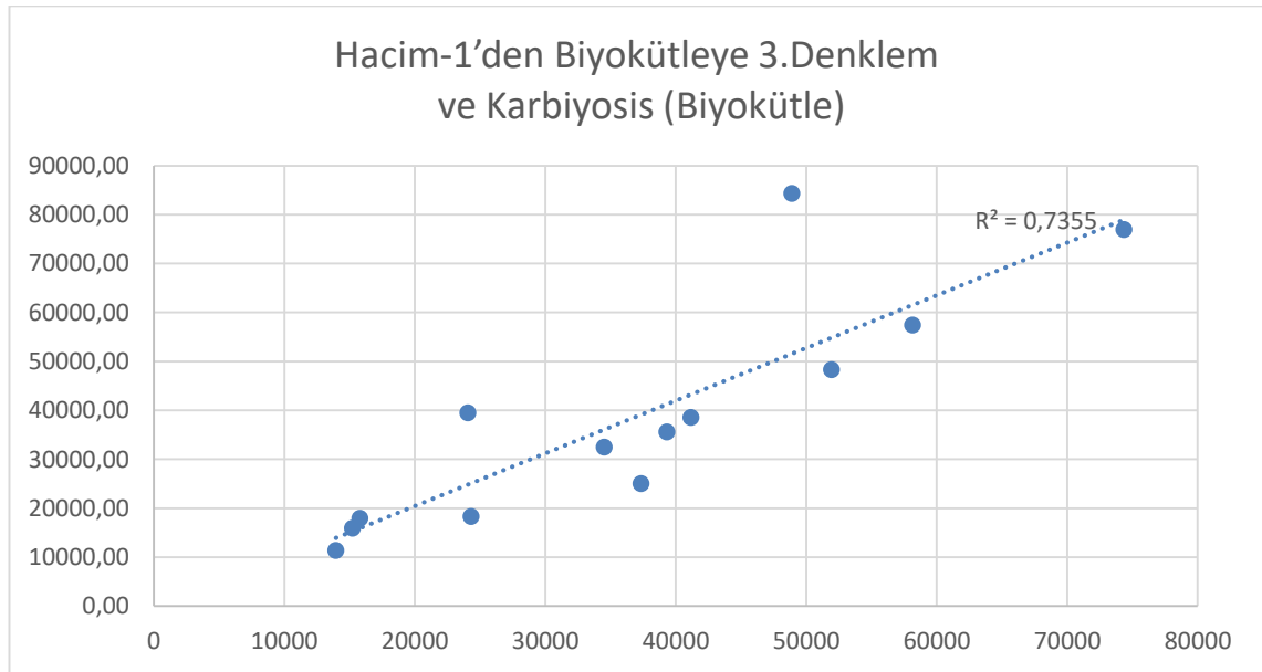
Şekil 4.19. Hacim-1'den biyokütleye üretilen 3. denklemden elde edilen biyokütle ile Karbiyosis'den elde edilen biyokütle değerlerinin karşılaştırılması
