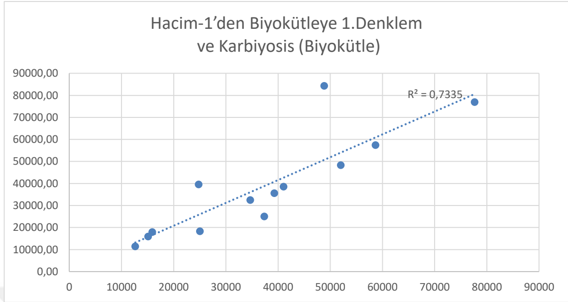
Şekil 4.18. Hacim-1'den biyokütleye üretilen 1. denklemden elde edilen biyokütle ile Karbiyosis'den elde edilen biyokütle değerlerinin karşılaştırılması
