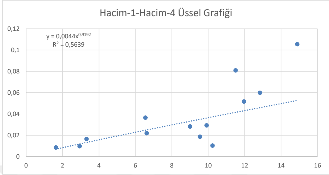
Şekil 4.6. Hacim-1’den Hacim-4’e üretilen üssel denklem, R 2 değeri ve grafiği
