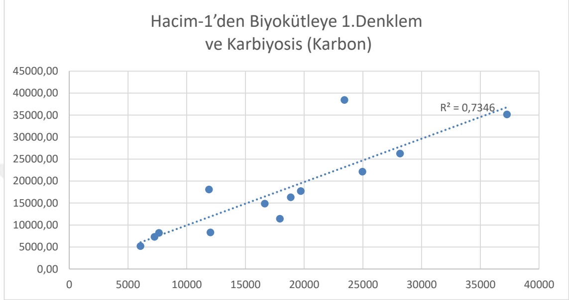
Şekil 4.20. Hacim-1'den biyokütleye üretilen 1. denklemden elde edilen karbon ile Karbiyosis'den elde edilen karbon değerlerinin karşılaştırılması
