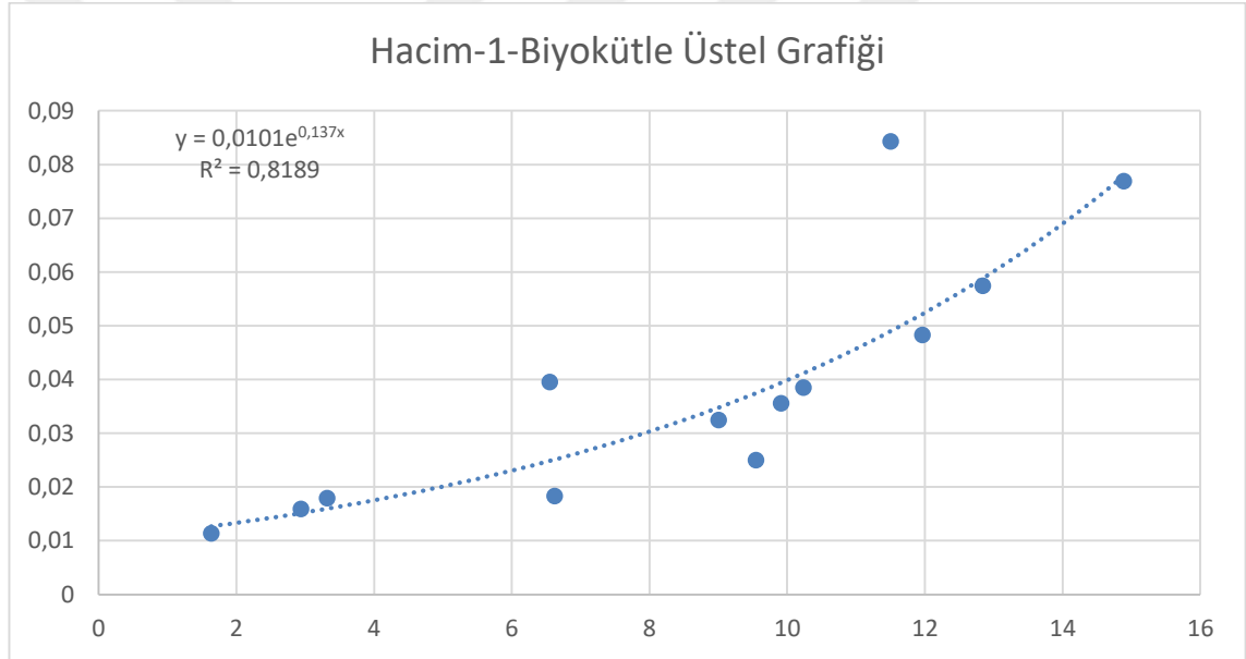
Şekil 4.7. Hacim-1'den biyokütleye üretilen üstel denklem, R^2 değeri ve grafiği
