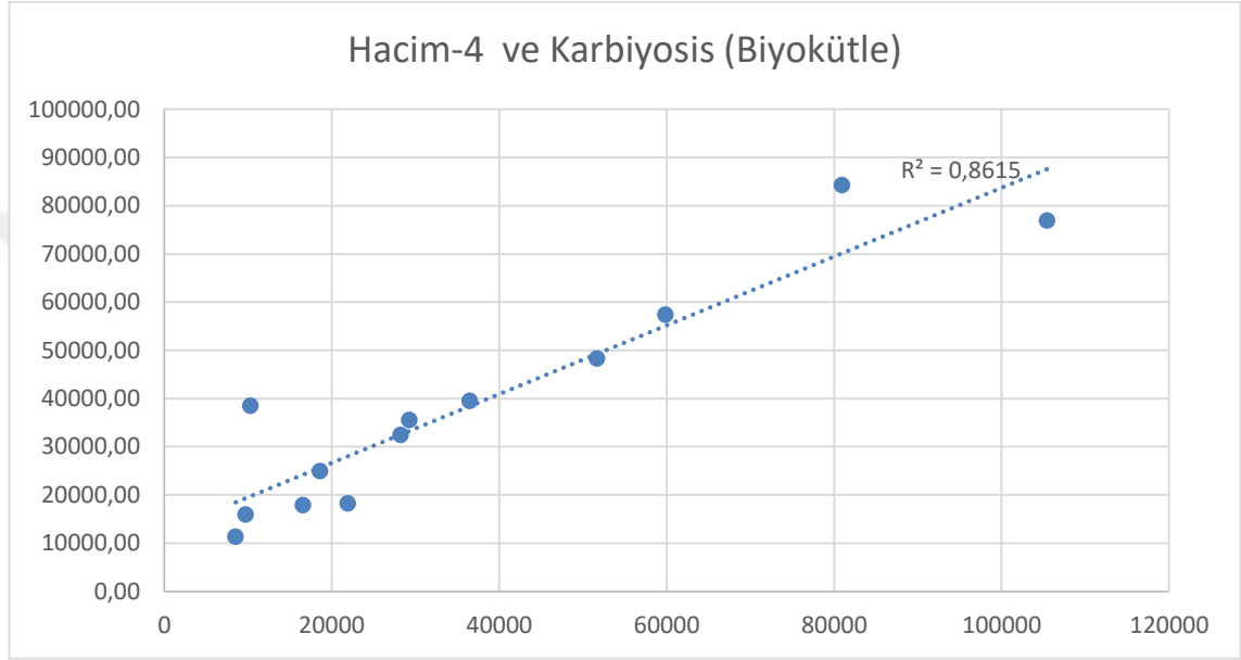
Şekil 4.12. Hacim-4'ten üretilen biyoküteller ile Karbiyosis'den elde edilen biyokütle değerlerinin karşılaştırılması
