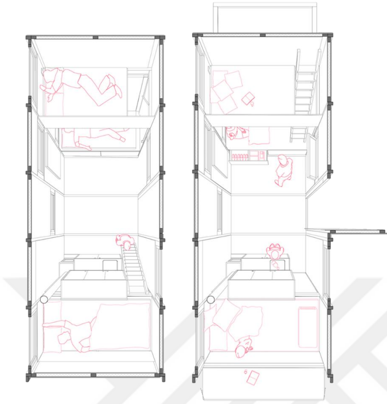
Şekil 2.25. Sınırdaki Barınak üst kat plan kullanım diyagramları (Anonim, 2020a).
