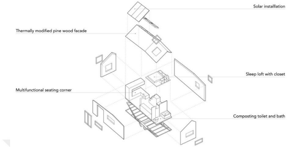
Şekil 2.9. Çağdaş Tiny House izometrik görüntüsü (Anonim, 2016).
