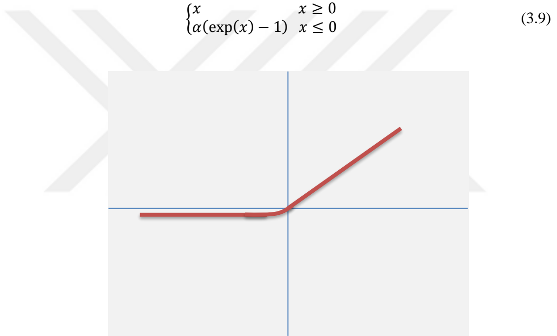
Şekil 3.8. ELU fonksiyonu.
