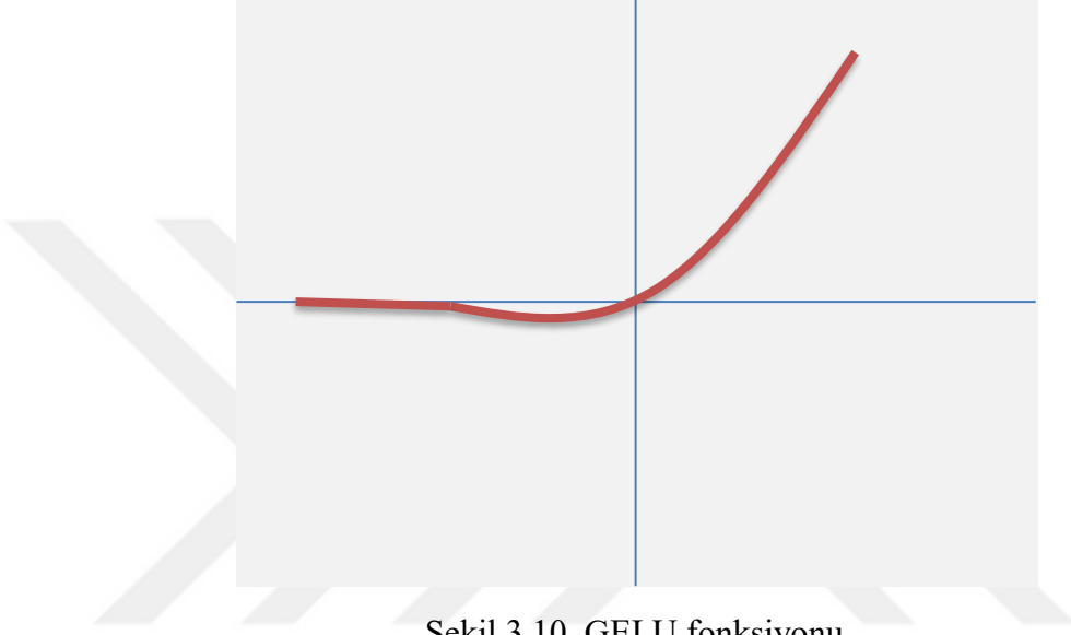
Şekil 3.10. GELU fonksiyonu.
