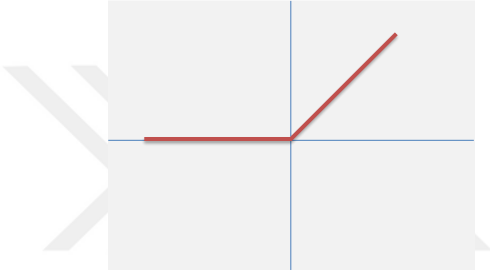
Şekil 3.5. ReLU fonksiyonu.
