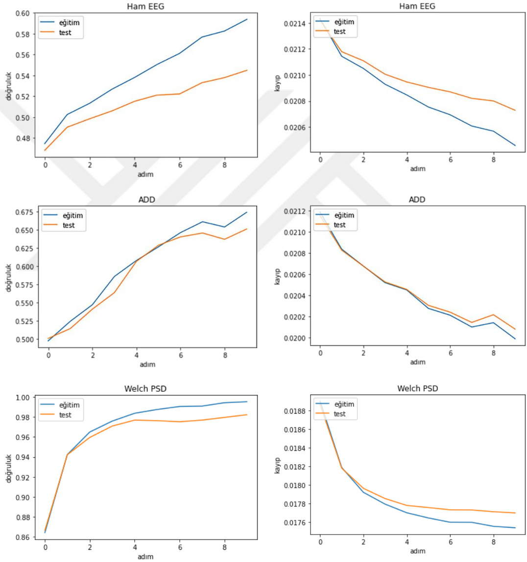
Şekil 4.7. Modelin doğruluk ve kayıp grafikleri.
