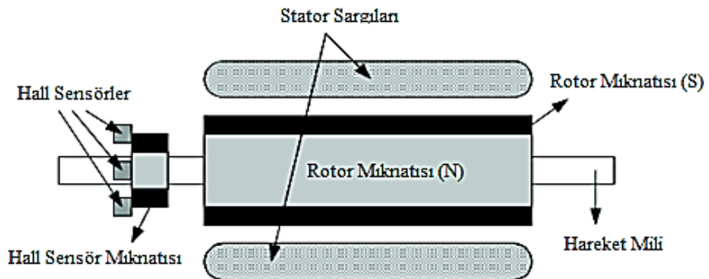
Şekil 3.7. BLDC motor üzerindeki Hall etkili sensörlerin yerleşimi (Yedamale, 2003)
