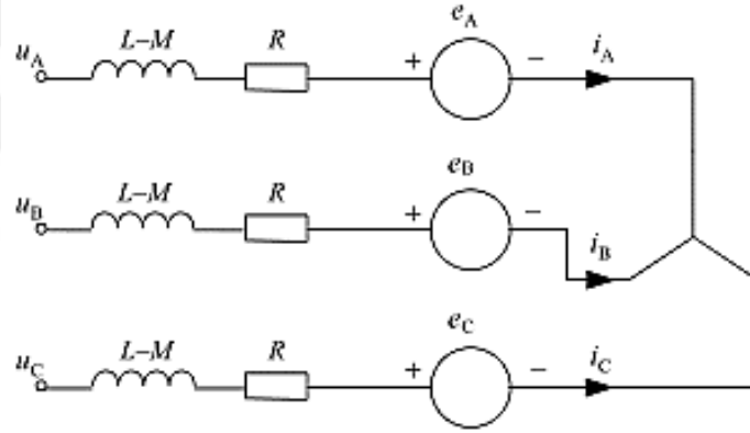
Şekil 3.2. Yıldız bağlı üç fazlı BLDC motorun devre şeması (Xia, 2012).
