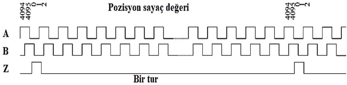
Şekil 3.8. Dörtlü darbe enkoderi çıkış sinyalleri (Semiconductor, 2013)
