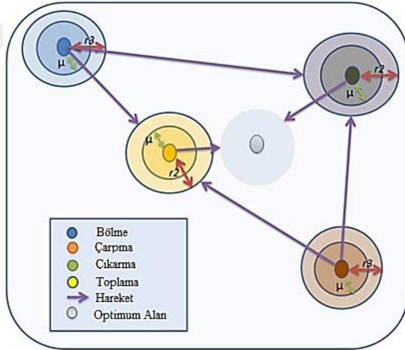
Şekil 3.27. Aritmetik optimizasyon algoritması güncelleme modeli
