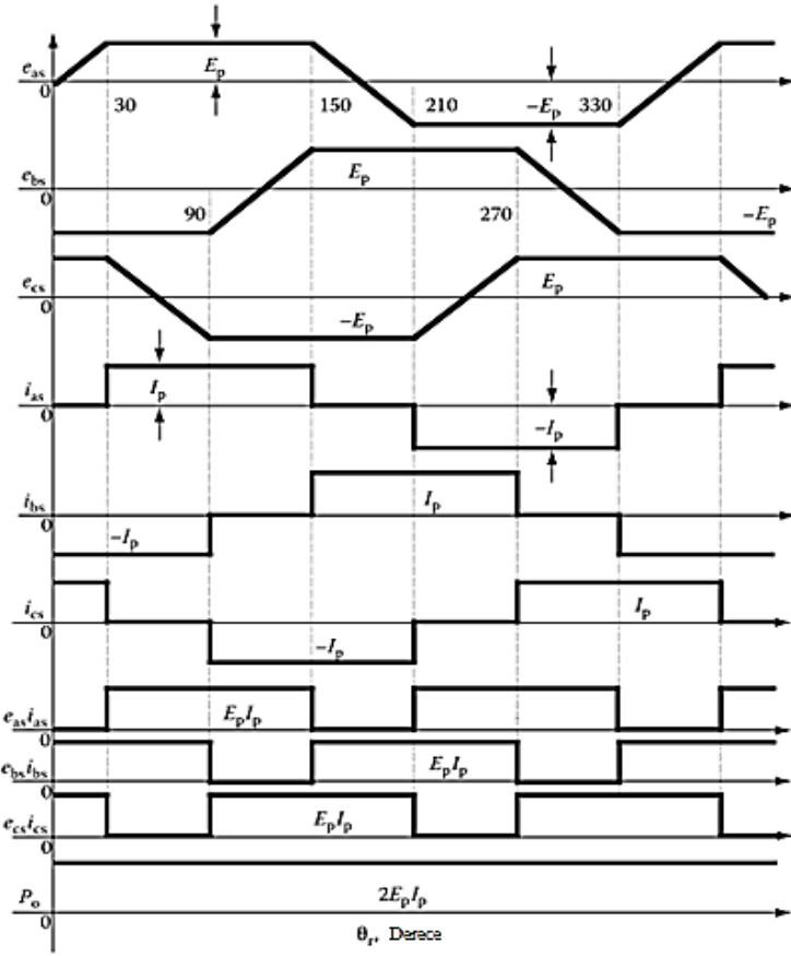
Şekil 3.3. BLDC motorun üç faza ait zıt EMK ve faz akım dalga formu (Krishnan, 2017)
