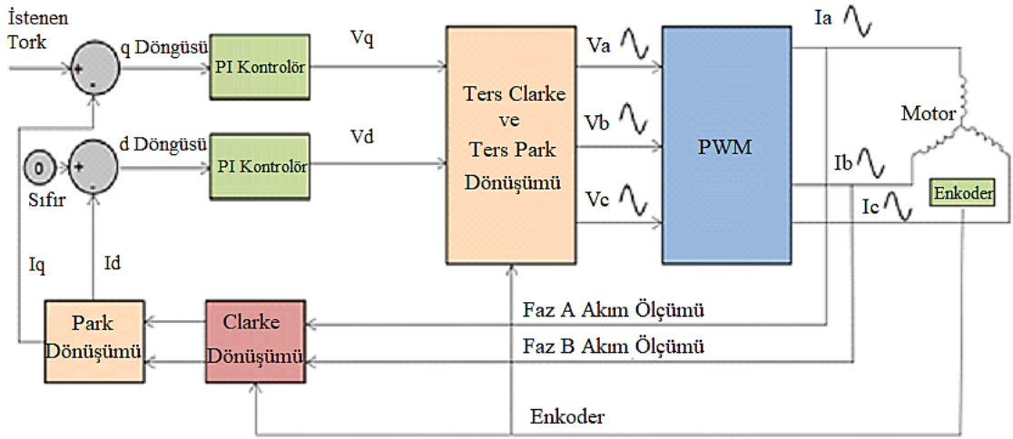
Şekil 3.15. Alan yönelimli kontrol sürücüsünün blok şeması (Kiran ve Puttaswamy, 2014)
