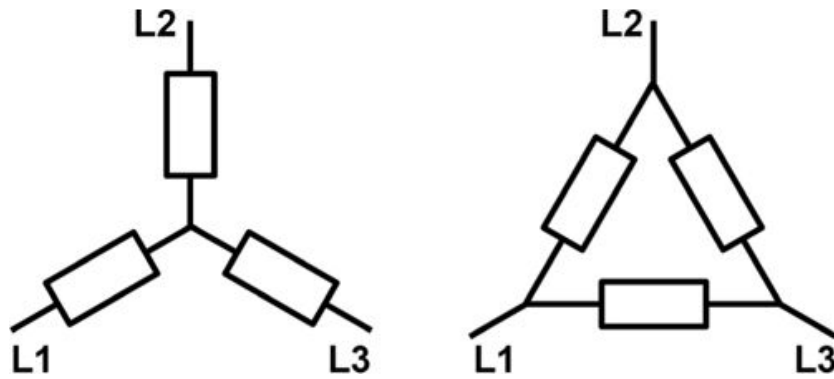
Şekil 3.4. Yıldız (solda) ve üçgen (sağda) bağlantı şekilleri (Buchi, 2012)
