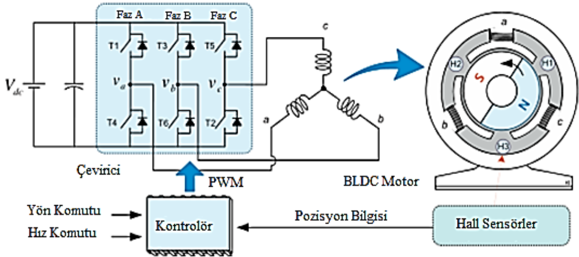
Şekil 3.6. BLDC motora bağlı dönüştürücü devresi (Kim, 2017)
