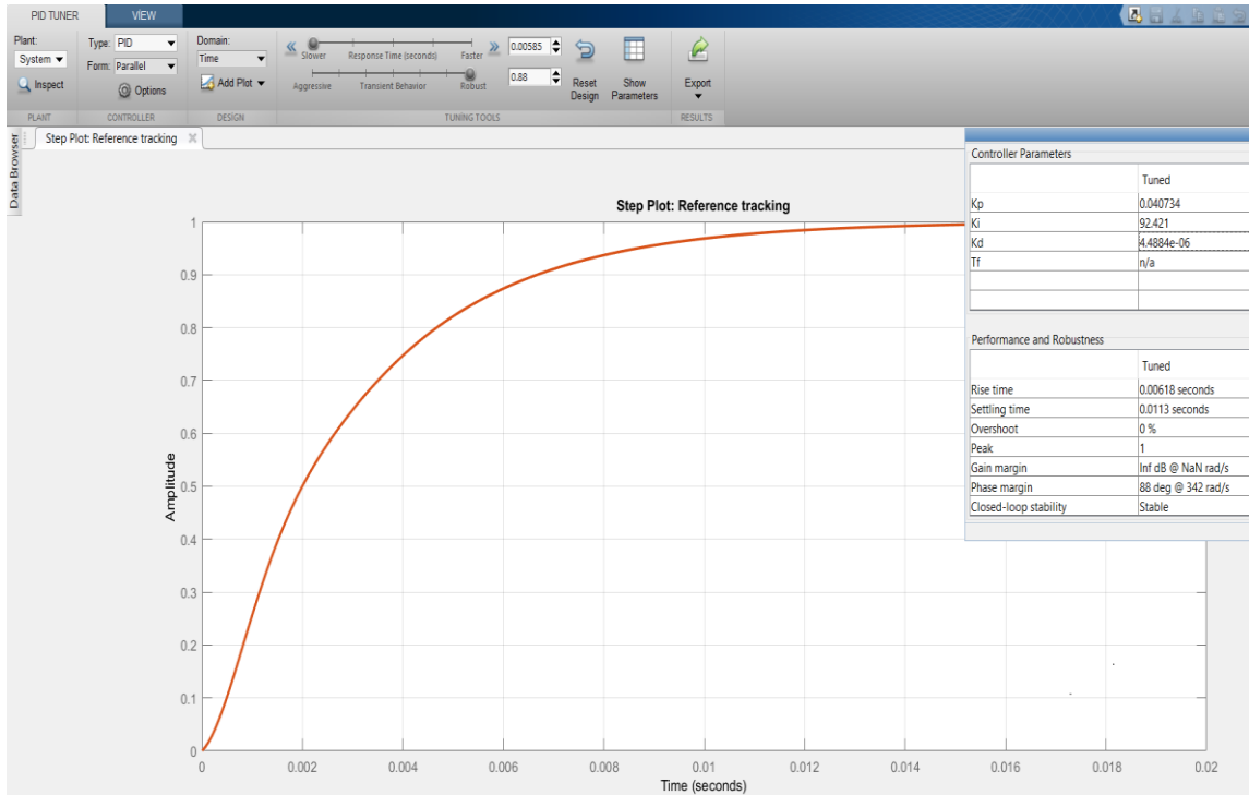
Şekil 3.25 BLDC motorun MATLAB PID Tuner basamak cevabı
