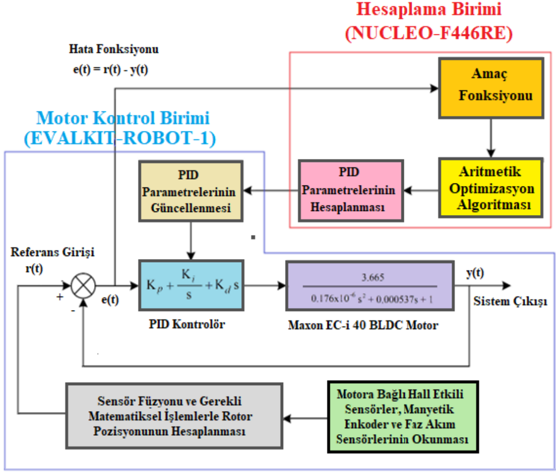
Şekil 3.36. Önerilen yöntemin motor pozisyon kontrol blok diyagramı
