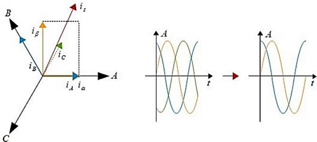
Şekil 3.13. Clarke Dönüşümü
