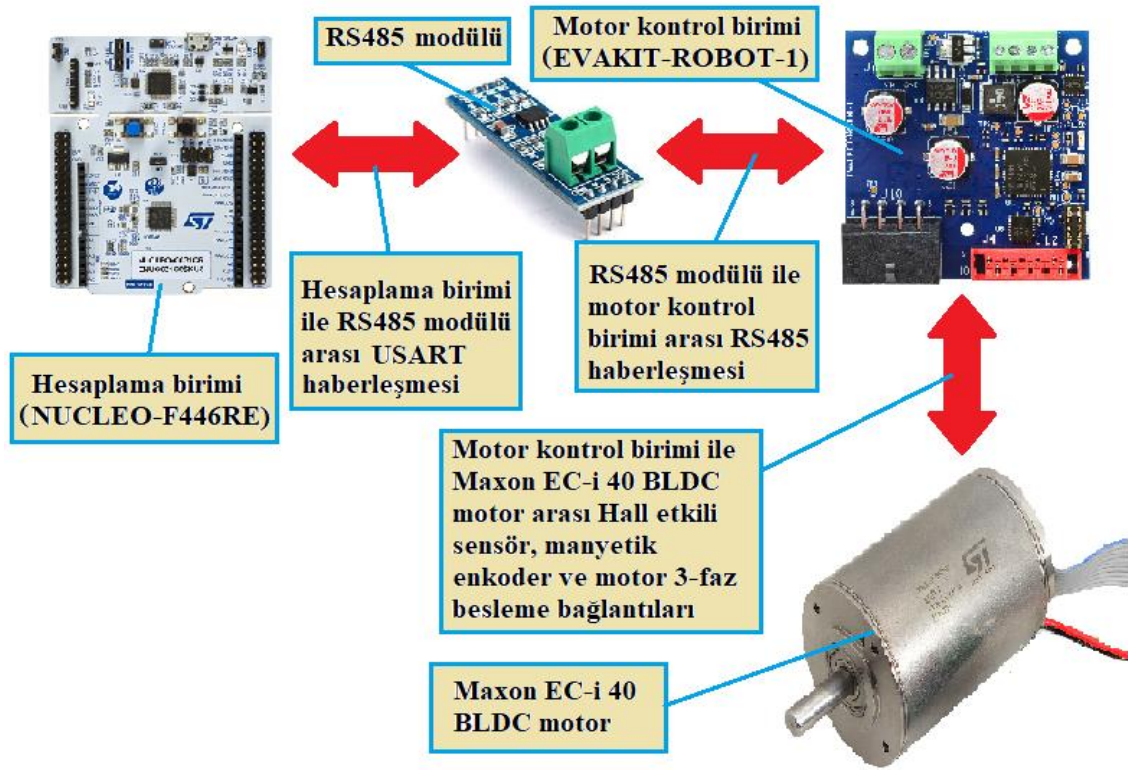
Şekil 3.34. Önerilen yöntem için kurulan sistemin bağlantı blok diyagramı
