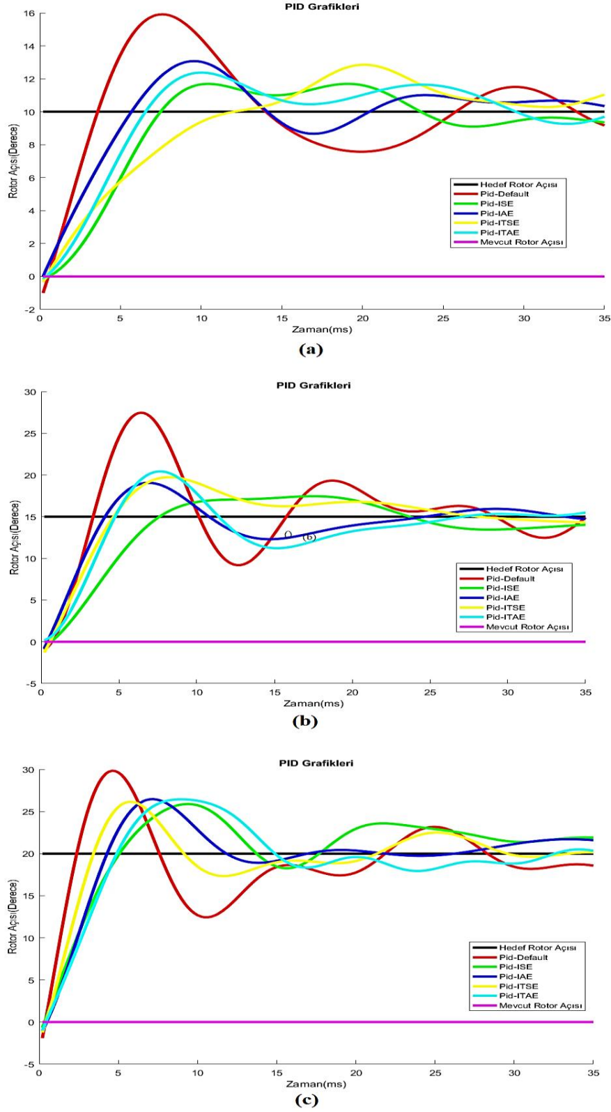
Şekil 4.4. (a) Rotor pozisyonu 0^\circ 'de iken rotor pozisyonuna eklenen -10^\circ gürültüye göre PID kontrolörün tepkisi, (b) Rotor pozisyonu 0^\circ 'de iken rotor pozisyonuna eklenen -15^\circ gürültüye göre PID kontrolörün tepkisi ve (c) Rotor pozisyonu 0^\circ 'de iken rotor pozisyonuna eklenen -20^\circ gürültüye göre PID kontrolörün tepkisi
