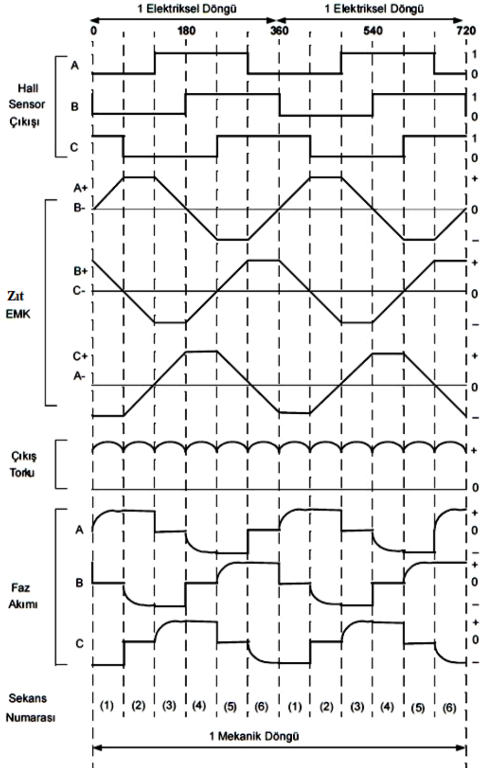
Şekil 3.10. Hall etkili sensör, Zıt EMK, tork ve faz akım değerleri (Yedamale, 2003)
