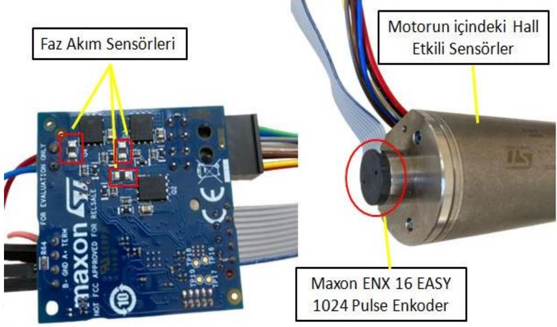
Şekil 3.37. Rotor pozisyon kontrolünde kullanılan sensörlerin yerleşimi
