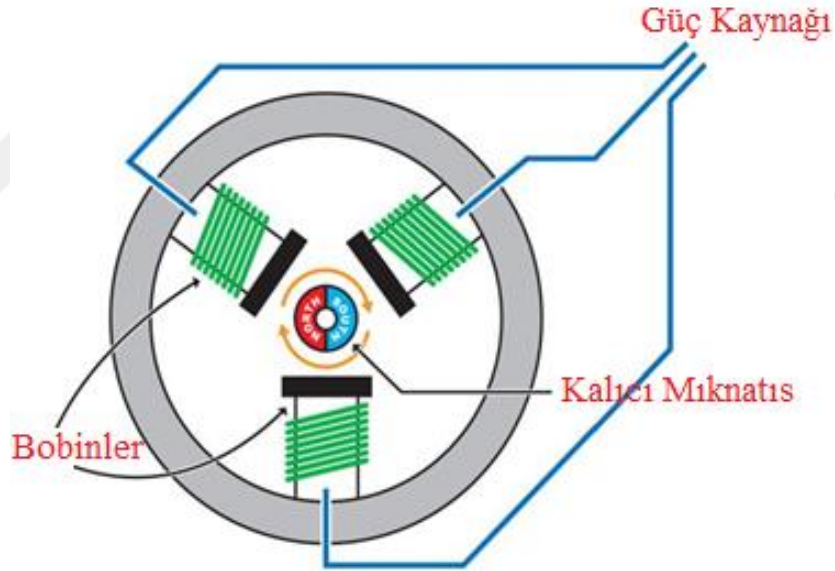
Şekil 3.1. BLDC motorun temel yapısı (Kiran ve Puttaswamy, 2014)
