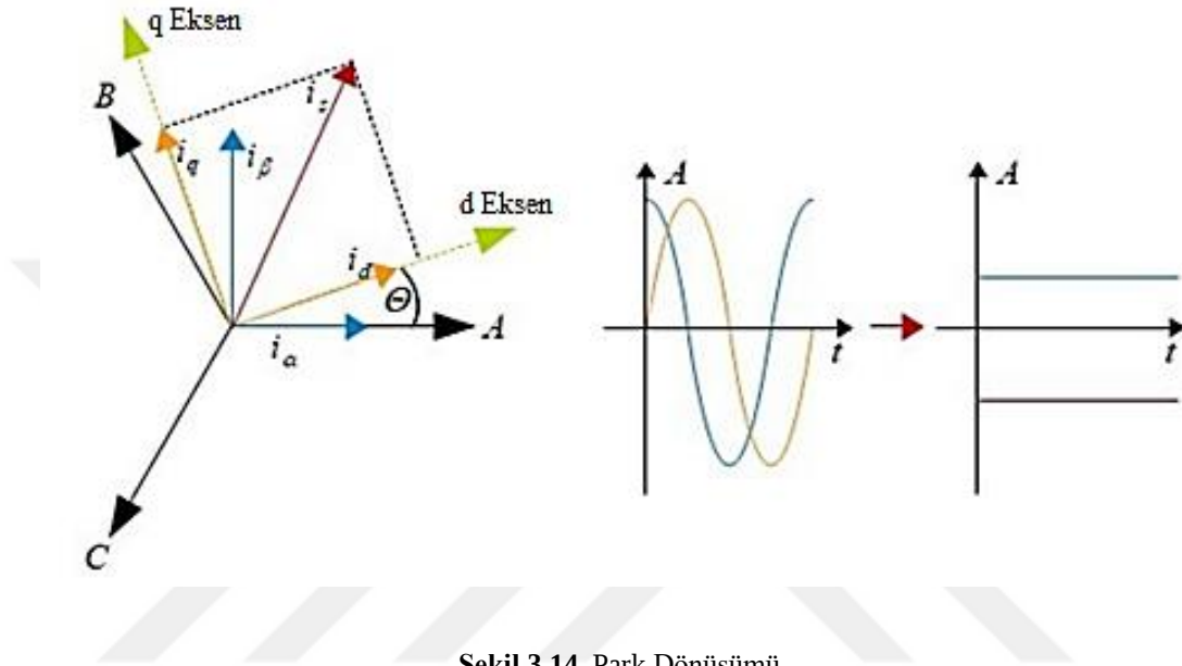
Şekil 3.14. Park Dönüşümü
