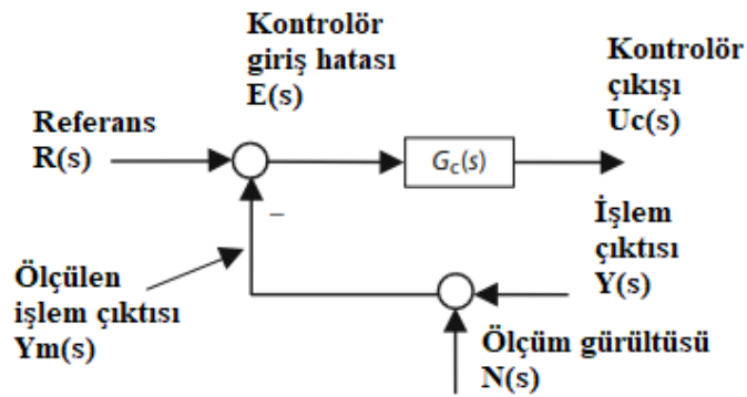
Şekil 3.19 PID kontrolör için giriş ve çıkış sinyalleri
