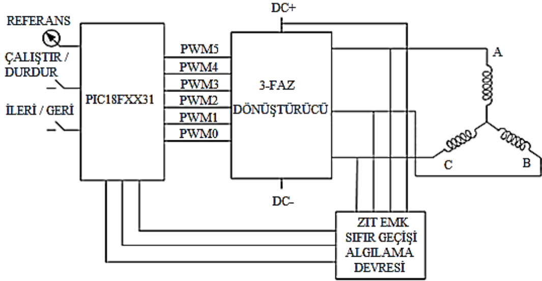
Şekil 3.16. Zıt EMK kontrol yöntemi ile BLDC motor kontrol blok diyagramı (Yedamale, 2003)
