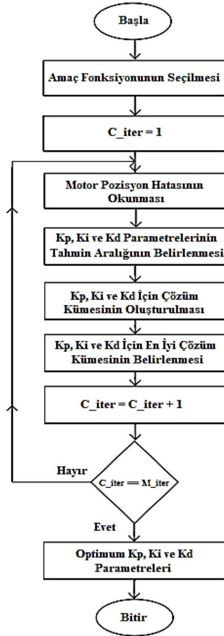
Şekil 3.42. BLDC motor pozisyon kontrolünde PID kontrolör parametrelerini optimize eden AOA'nın akış diyagramı
