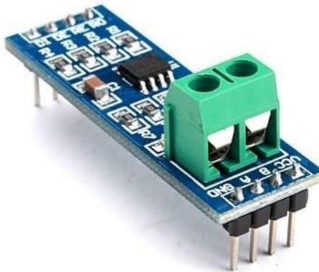
Şekil 3.33. RS485-TTL seri dönüştürücü kartının görüntüsü
