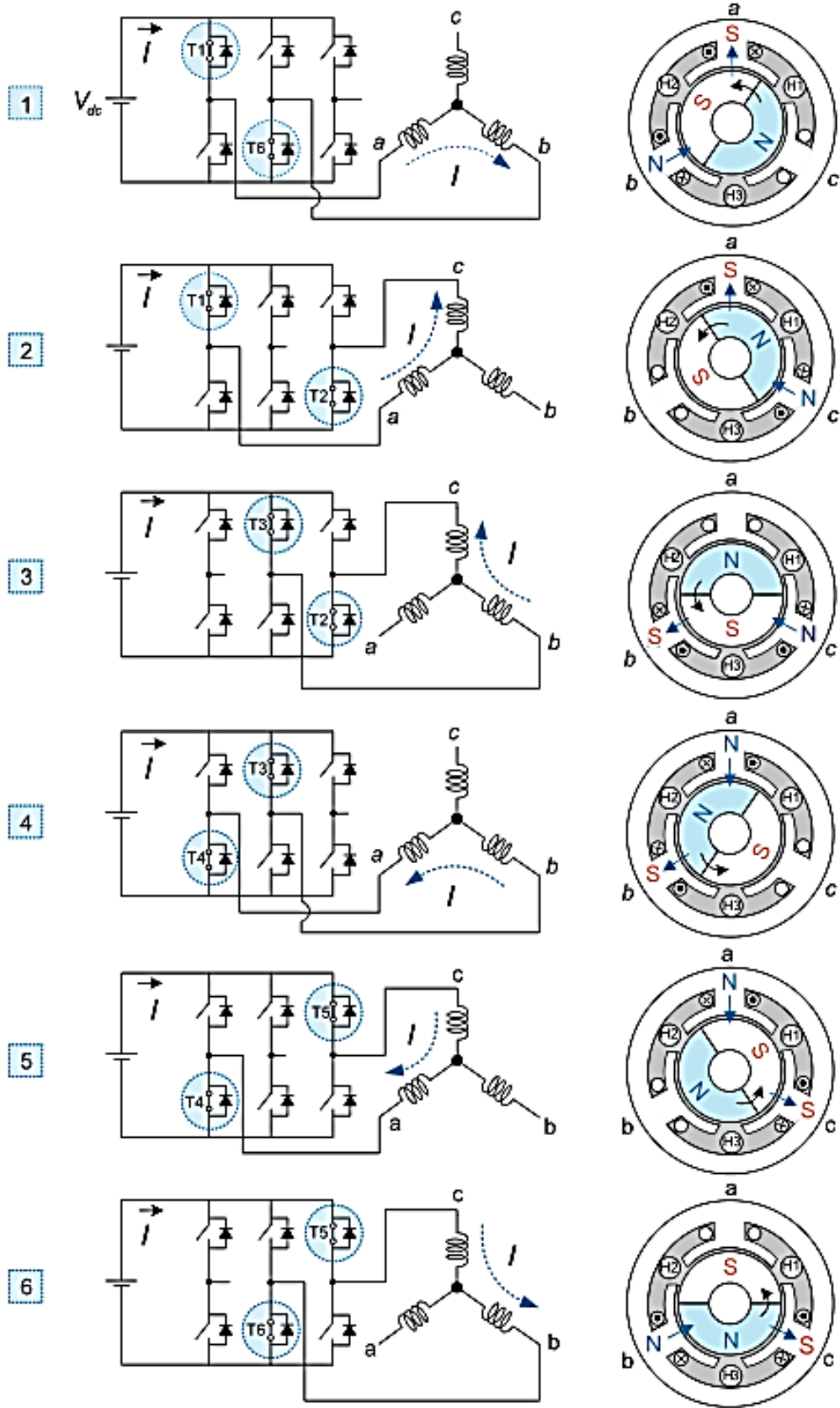
Şekil 3.11. Hall etkili sensörlere göre izlenmesi gereken ikili anahtarlama sırası (Kim, 2017)
