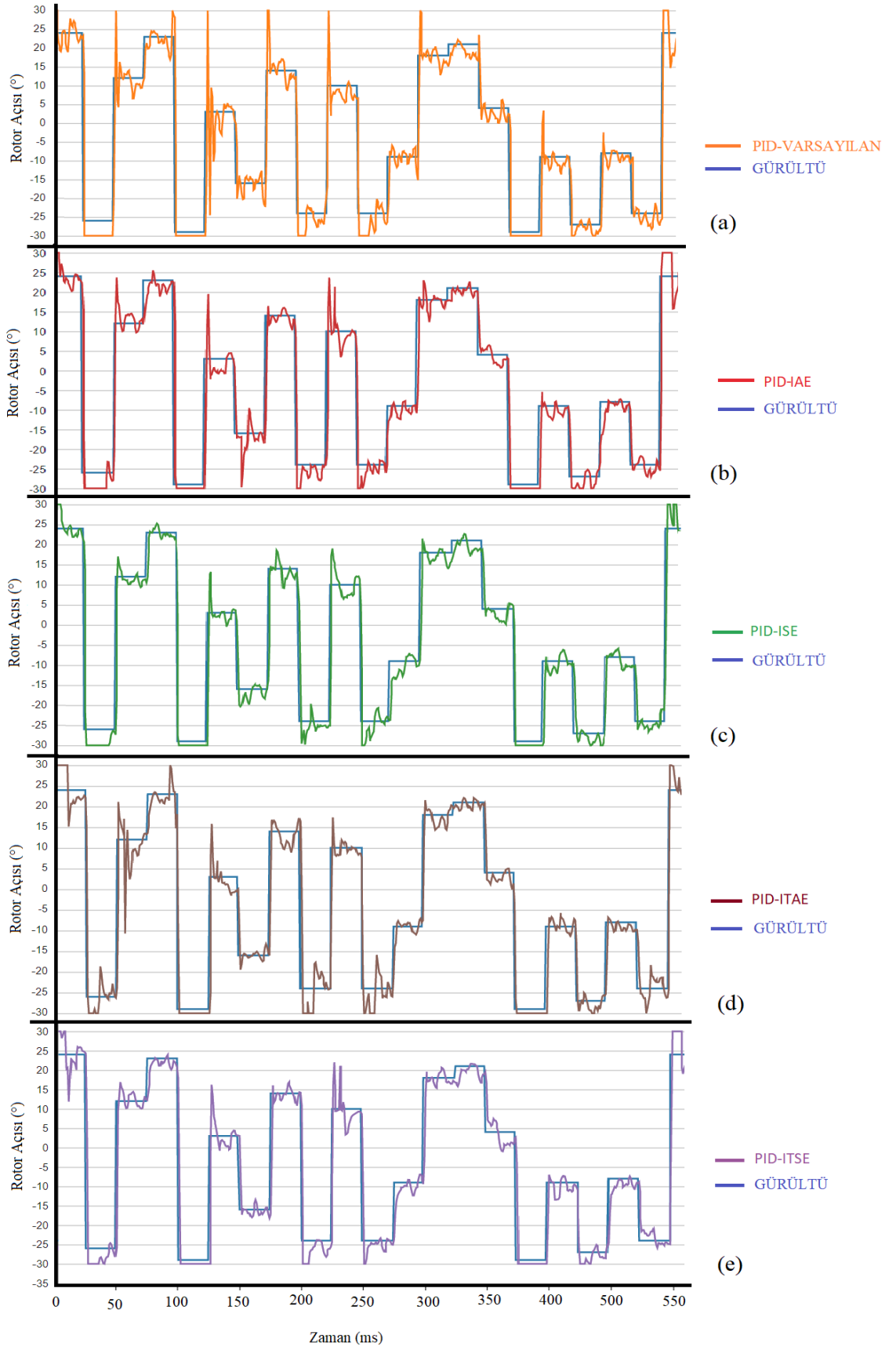
Şekil 4.1. Rotor pozisyon hatasına göre PID kontrolörün tepkisi
