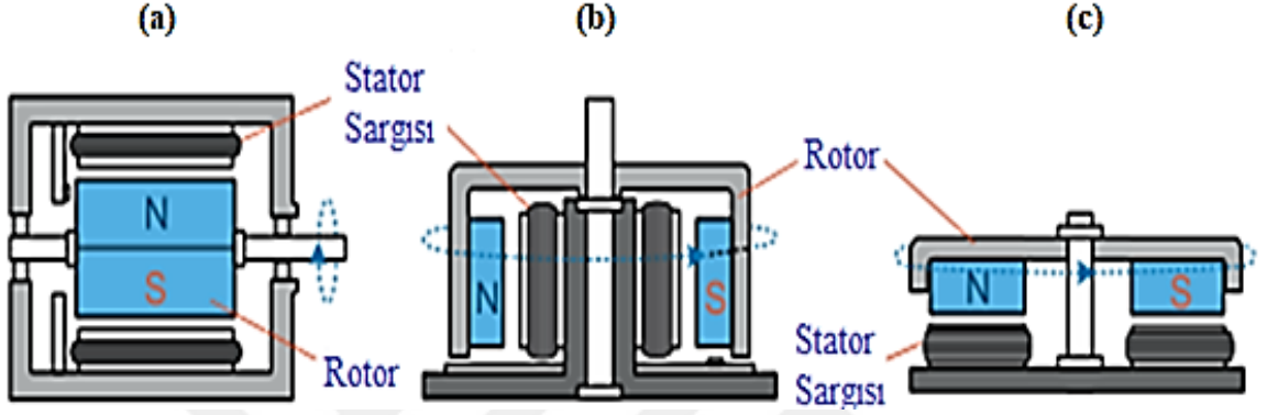
Şekil 3.5. BLDC motorun tasarım tipleri, (a) Radyal akı (iç rotor), (a) Radyal akı (dış rotor) ve (c) Eksenel akı (Kim, 2017)
