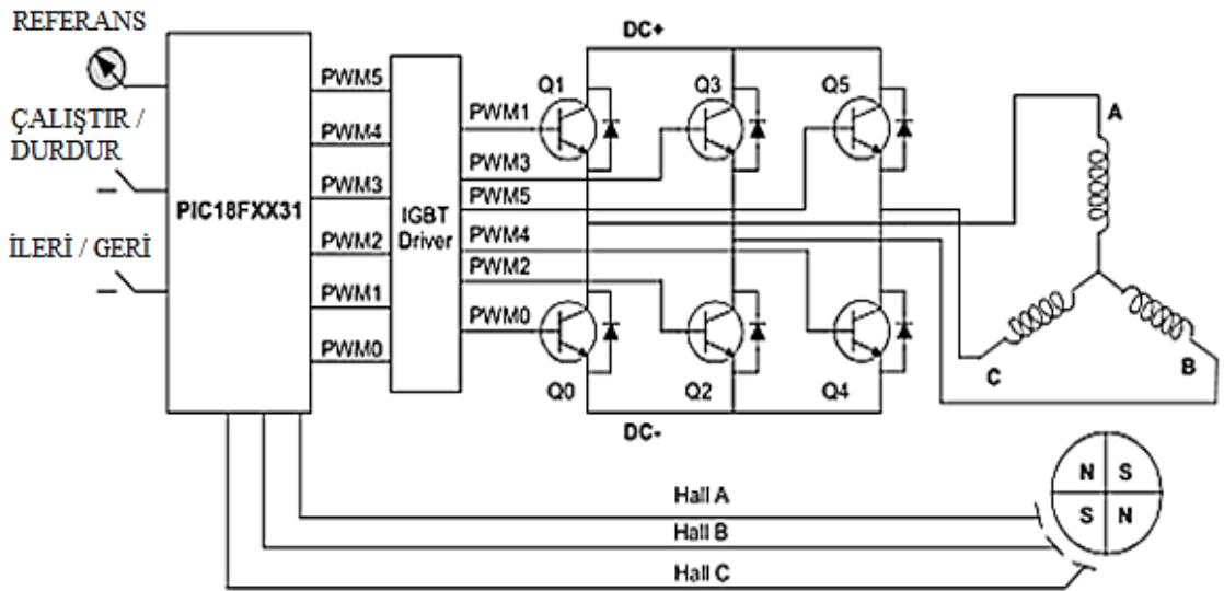
Şekil 3.9. Altı adımlı kontrol yöntemi blok diyagramı (Yedamale, 2003)
