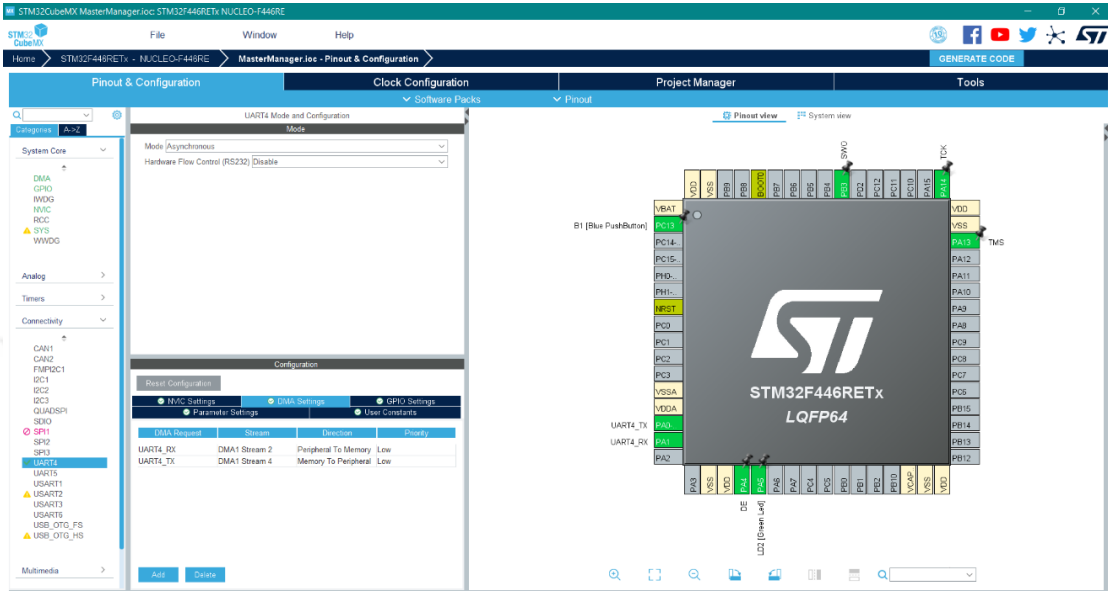
Şekil 3.40. STM32F446RET6 mikrokontrolörün STM32CubeMX konfigürasyonu
