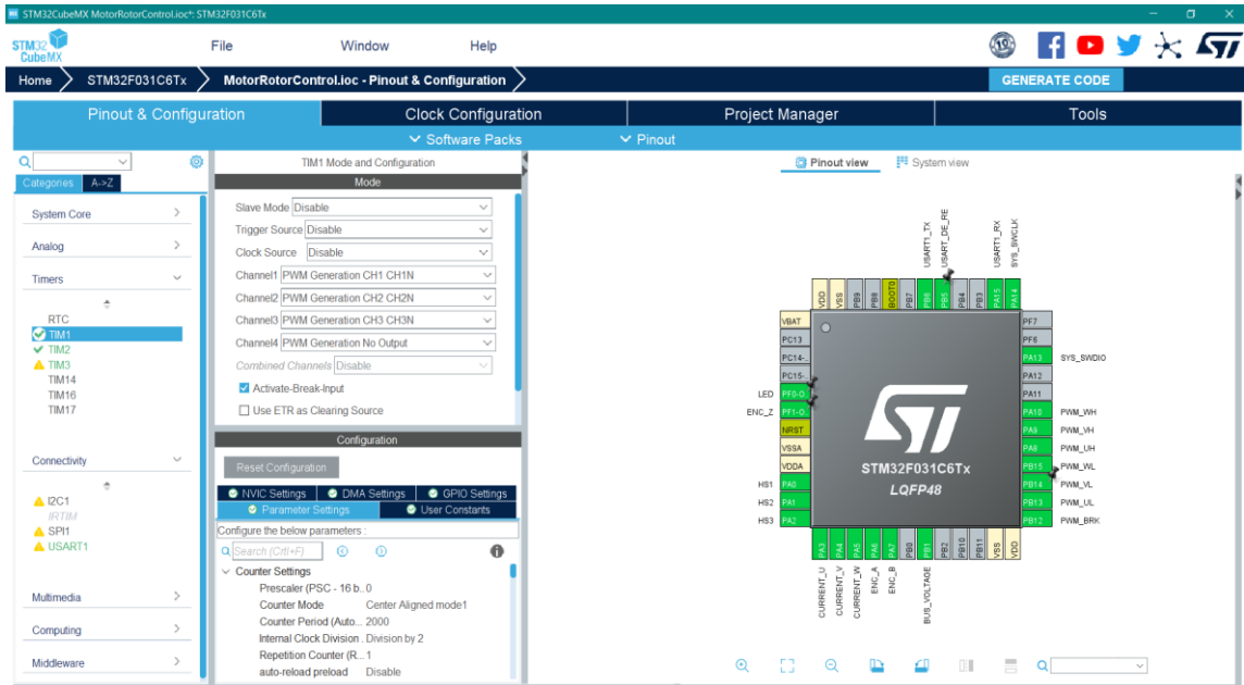
Şekil 3.38. STM32F031C6T6 mikrokontrolörün STM32CubeMX konfigürasyonu
