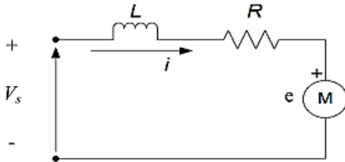
Şekil 3.17. BLDC motorun tek faz eşdeğer devresi (Kiruthika ve ark., 2013)
