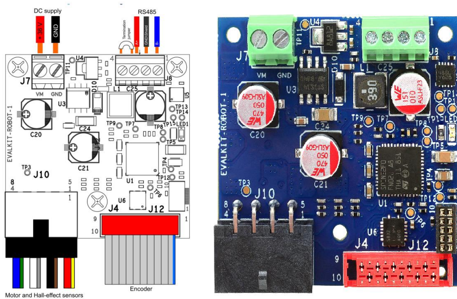
Şekil 3.31. EVALKIT-ROBOT-1 kartının görüntüsü
