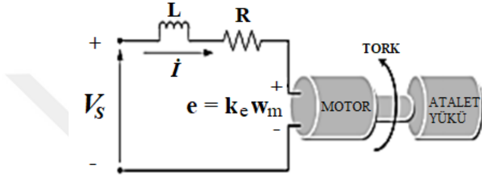
Şekil 3.18. BLDC motorun eşdeğer elektromekanik sistemi
