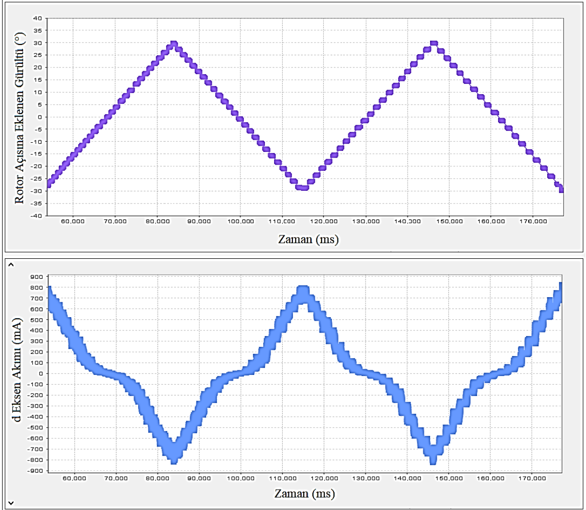
Şekil 4.2. Rotor pozisyon hatasına göre d eksen akımının değişimi
