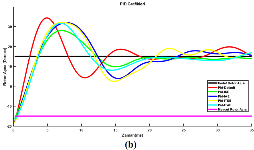
Şekil 4.3. (a) Rotor pozisyonu -5^\circ 'de iken rotor pozisyonuna eklenen -10^\circ gürültüye göre PID kontrolörün tepkisi ve (b) Rotor pozisyonu -15^\circ 'de iken rotor pozisyonuna eklenen -30^\circ gürültüye göre PID kontrolörün tepkisi
