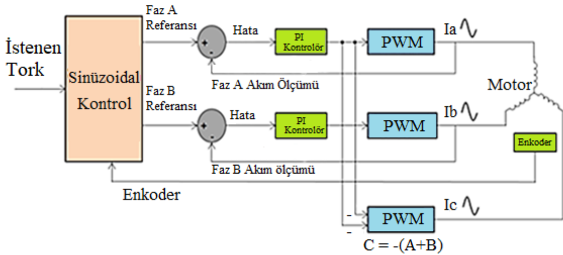
Şekil 3.12. Sinüzoidal kontrol blok diyagramı
