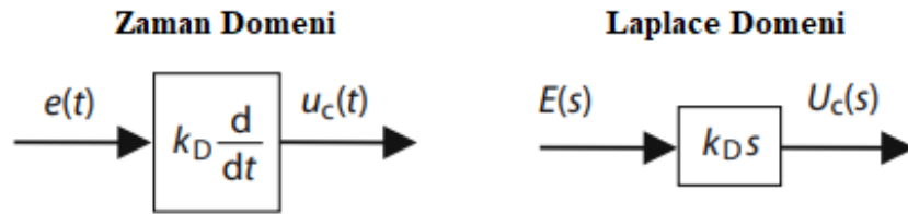
Şekil 3.22 Türevsel kontrol blok diyagramları
