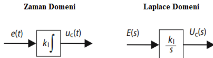
Şekil 3.21 İntegral kontrol blok diyagramları
