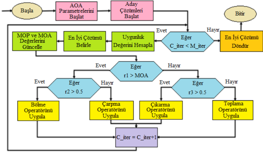
Şekil 3.28. Aritmetik optimizasyon algoritması akış diyagramı
