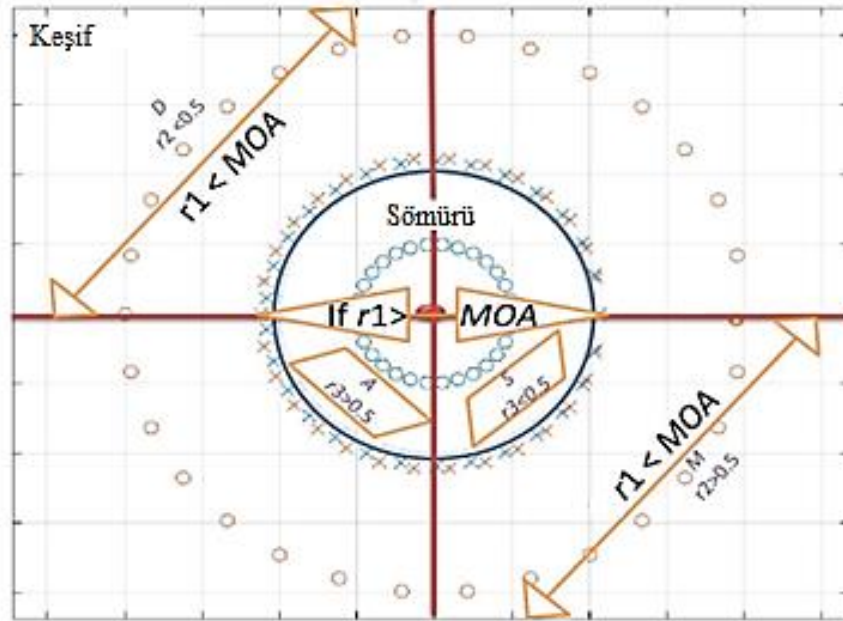
Şekil 3.26. Aritmetik optimizasyon algoritmasının arama aşamaları
