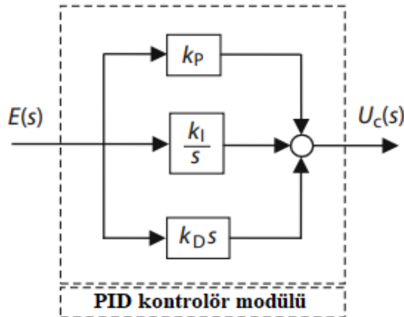
Şekil 3.23 Paralel PID kontrol blok diyagramı (Johnson ve Moradi, 2005)
