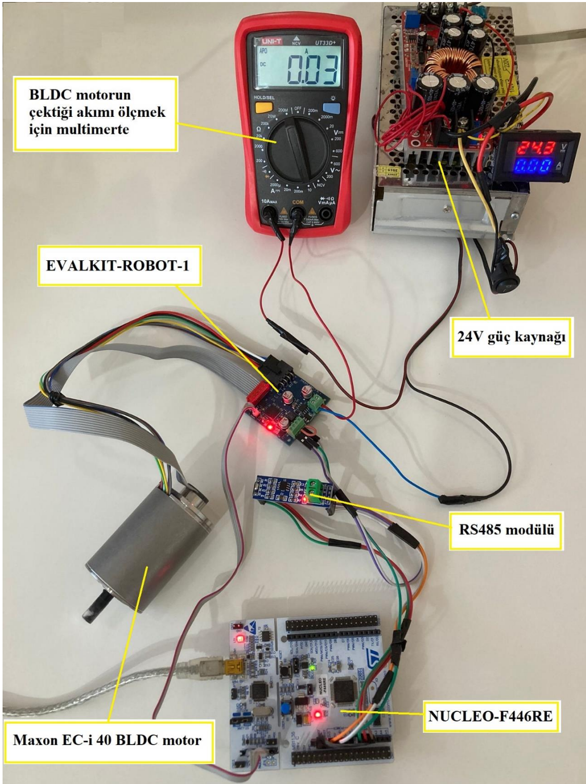
Şekil 3.35. Önerilen yöntem için kurulan deney düzeneği
