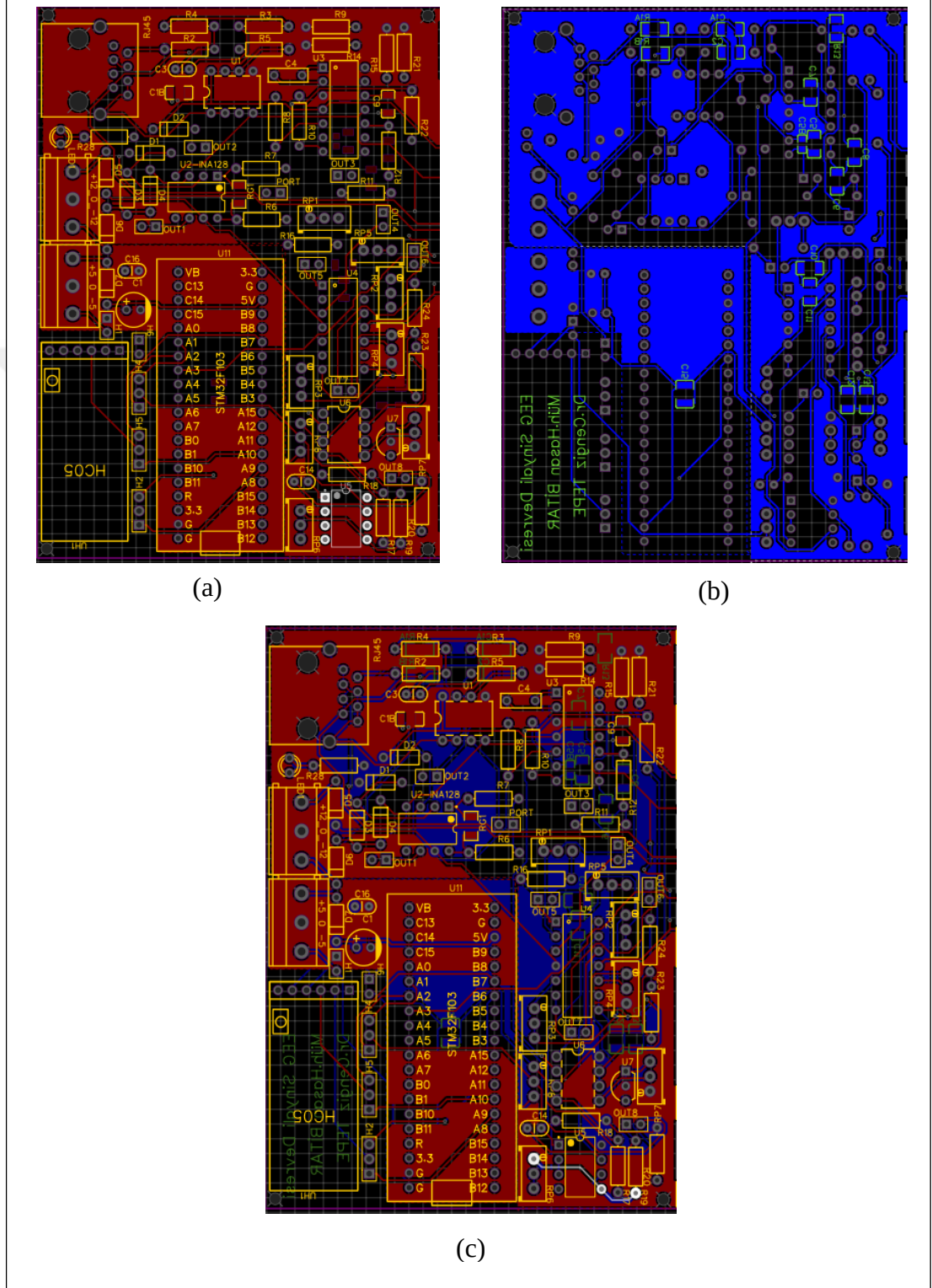
Şekil 5.30. EasyEDA yazılımında baskı devre çizimi (a) Ön katmanı (b) Arka katmanı (c) Tüm katmanları birlikte
