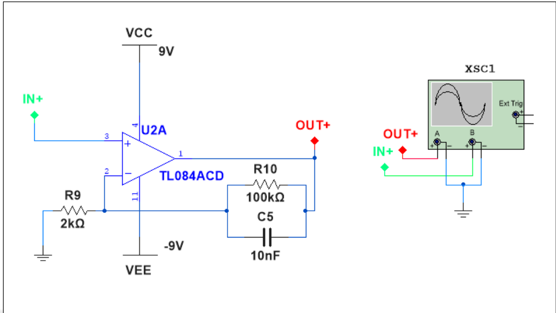
Şekil 5.12. Ana yükseltecinin devre şeması
