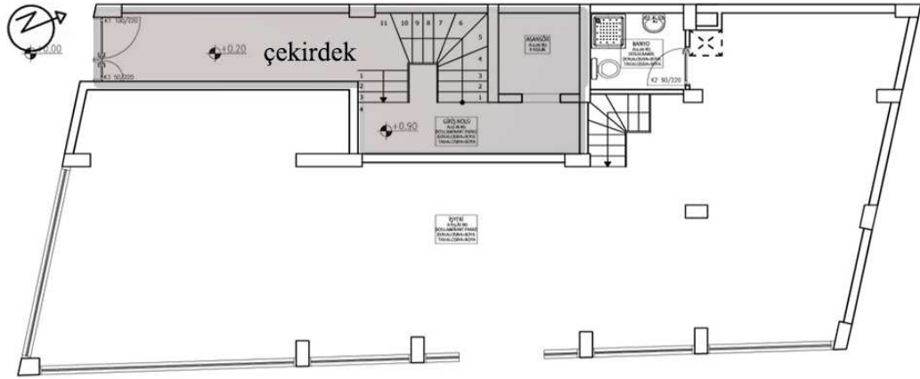
Şekil 5.61. Şenol Kankaya Apartmanı Giriş Kat Planı (Kocabaldır, 2016)
