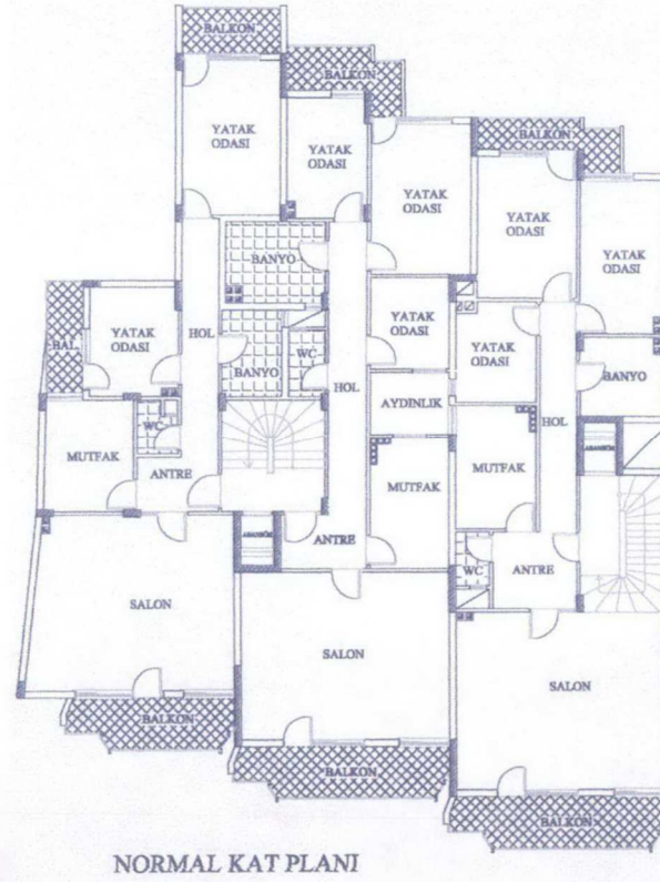
Şekil 5.10. Dura Apartmanı Normal Kat Planı (Ç.B. Arşivi)
