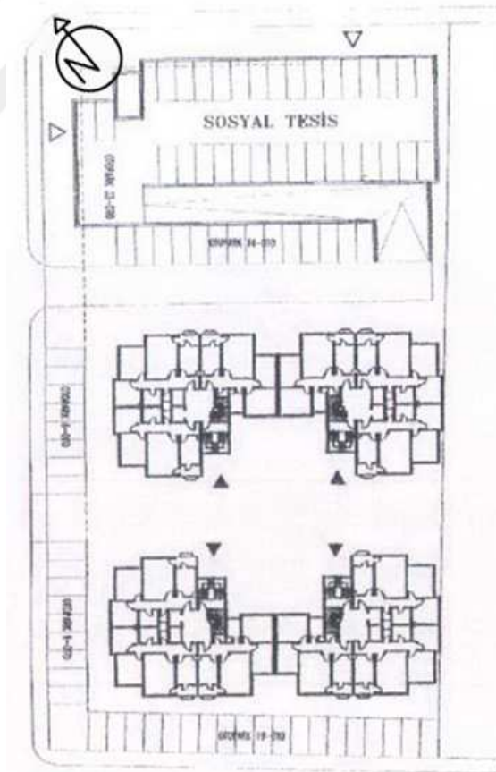
Şekil 5.43. Barışkent II Sitesi Vaziyet Planı (Ç.B. Arşivi)
