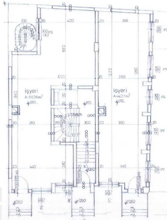
Şekil 5.12. Erdoğan Şair Apartmanı Giriş Kat Planı (Ç.B. Arşivi)
