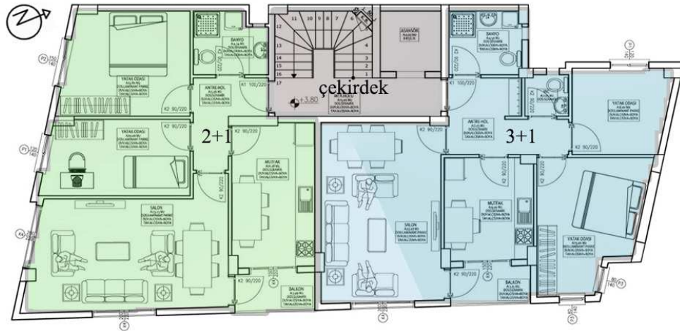
Şekil 5.62. Şenol Kankaya Apartmanı Normal Kat Planı (Kocabaldır, 2016)
