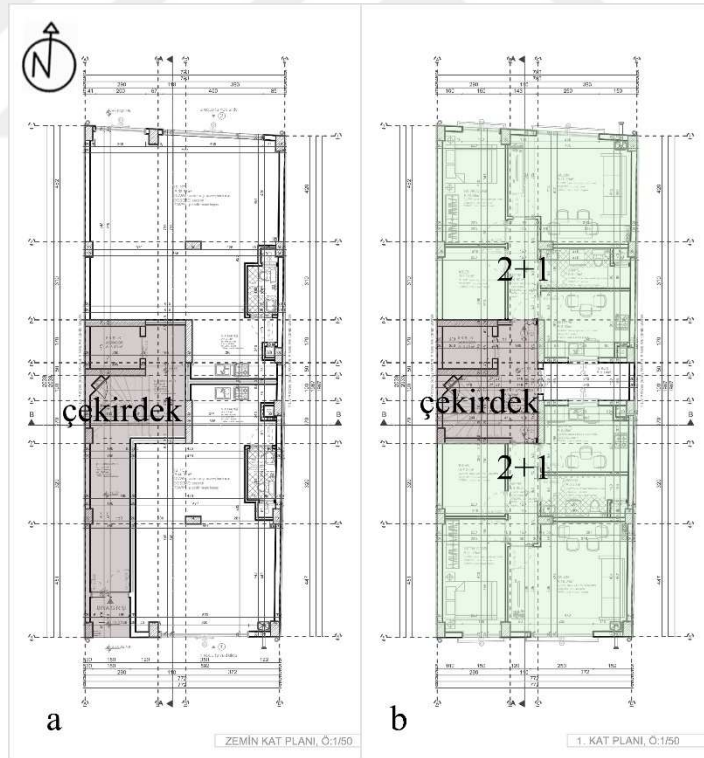
Şekil 5.75. Abdülbari Seçkin Apartmanı Zemin ve Normal Kat Planı a. Zemin Kat Planı (Girgin Albayrak, 2022) b. Normal Kat Planı (Girgin Albayrak, 2022)
