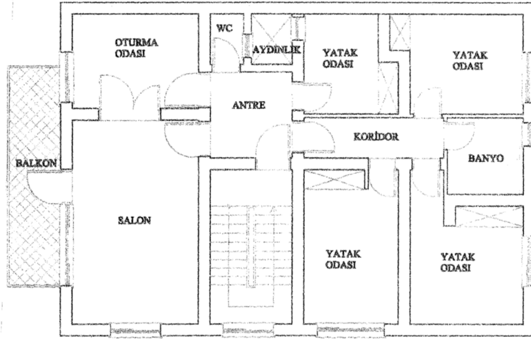
Şekil 5.4. Hüseyin Cevat Soral Evi Normal Kat Planı (Ç.B. Arşivi)
