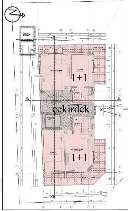
Şekil 5.67. İhlamur Apartmanı Giriş Kat Planı (Tekinalp, 2018)
