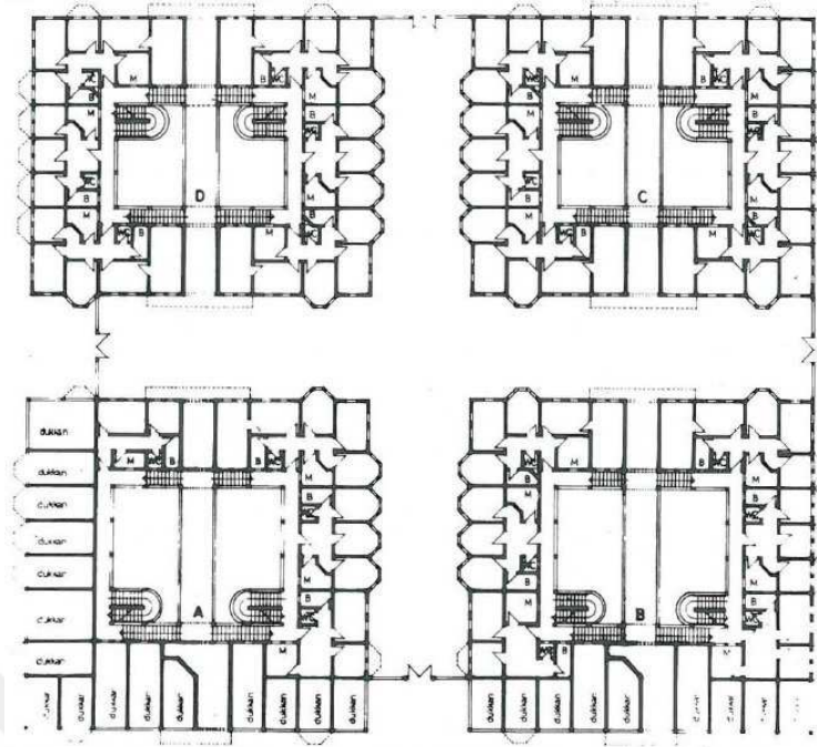
Şekil 2.22. Harikzedegan Apartmanı Planı (Yavuz Y. , 1993)
