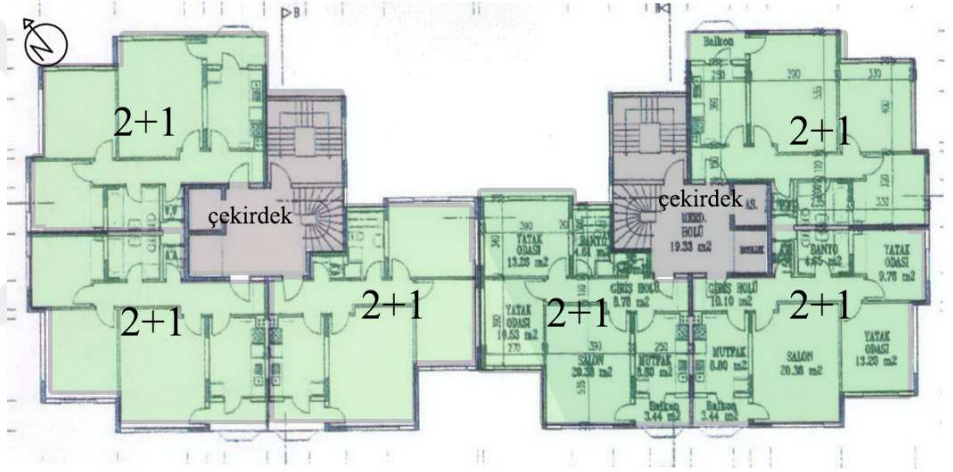
Şekil 5.45. Barışkent II Sitesi Normal Kat Planı (Ç.B. Arşivi)
