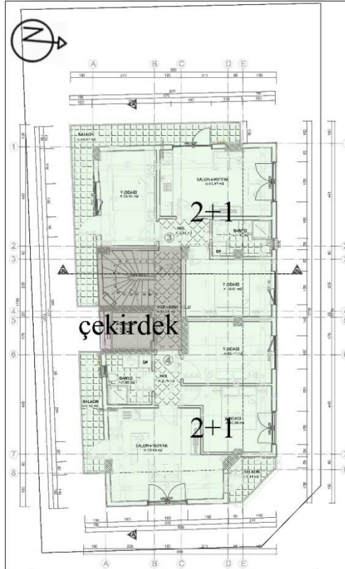
Şekil 5.68. İhlamur Apartmanı Normal Kat Planı (Tekinalp, 2018)
