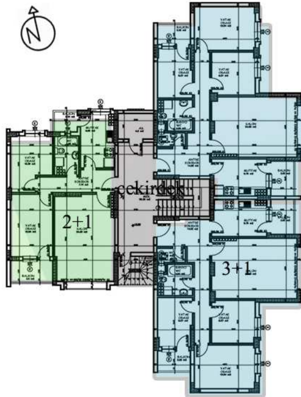
Şekil 5.57. Özgürkent Sitesi D1-D2 Tipi Giriş Kat Planı (Ç.B. Arşivi)
