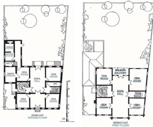
Şekil 4.1. Çanakkale Yalı Örneği Kat Planları (ÇEYAP, 2006)
