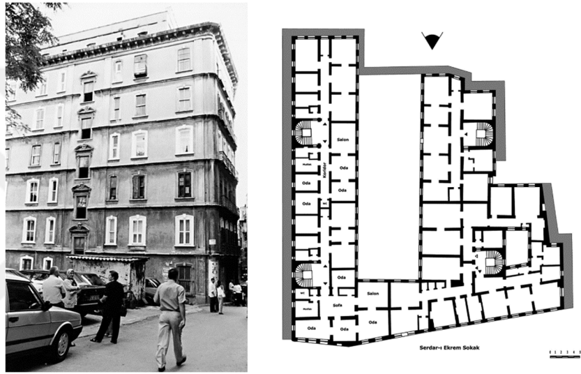
Şekil 2.21. Doğan Apartmanı Görsel ve Planı (Öncel, 2014)
