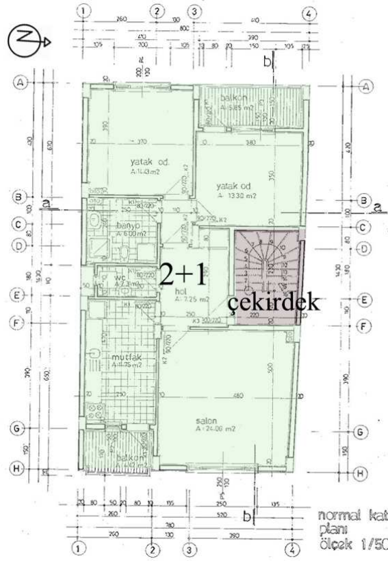
Şekil 5.31. Turhan Karakaya Apartmanı Normal Kat Planı (Ç.B. Arşivi)
