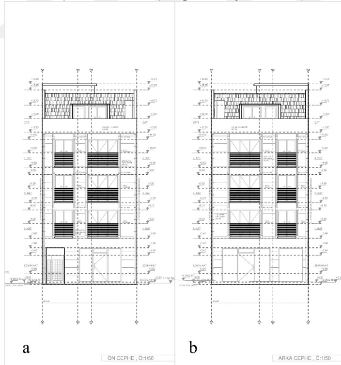
Şekil 5.77. Abdülbari Seçkin Apartmanı Görünüşler a.Kuzey Cephe (Girgin Albayrak, 2022) b. Güney Cephe (Girgin Albayrak, 2022)
