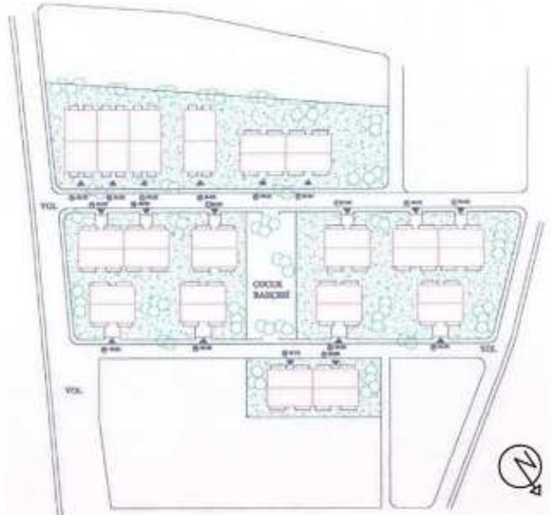
Şekil 5.33. Yeni Kordon Sitesi Vaziyet Planı (Ç.B. Arşivi)
