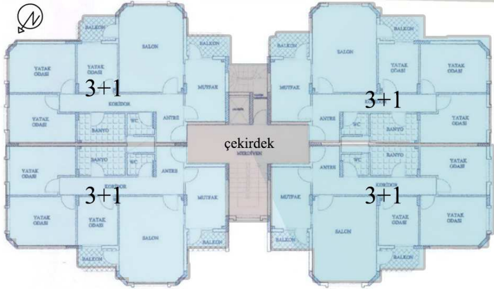
Şekil 5.26. Uğur 96 Koop. Normal Kat Planı (Ç.B. Arşivi)
