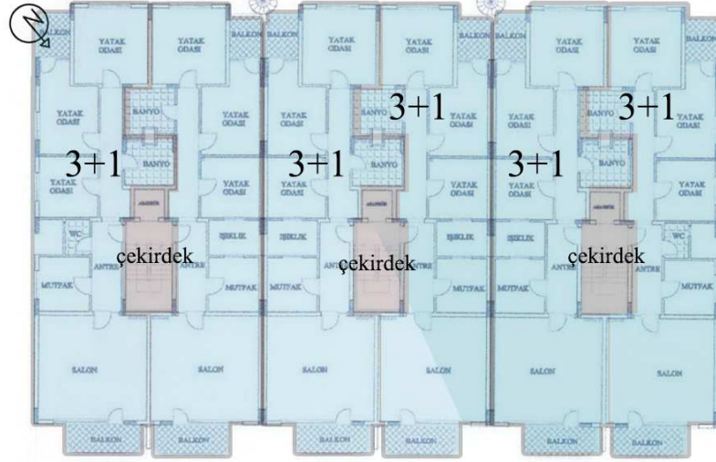
Şekil 5.34. Yeni Kordon Sitesi A-B-C Tipi Giriş Kat Planı (Ç.B. Arşivi)
