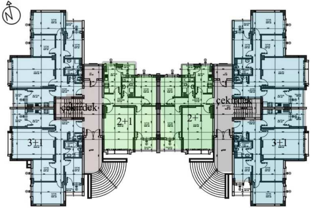
Şekil 5.55. Özgürkent Sitesi A1-A2 Tipi Giriş Kat Planı (Ç.B. Arşivi)
