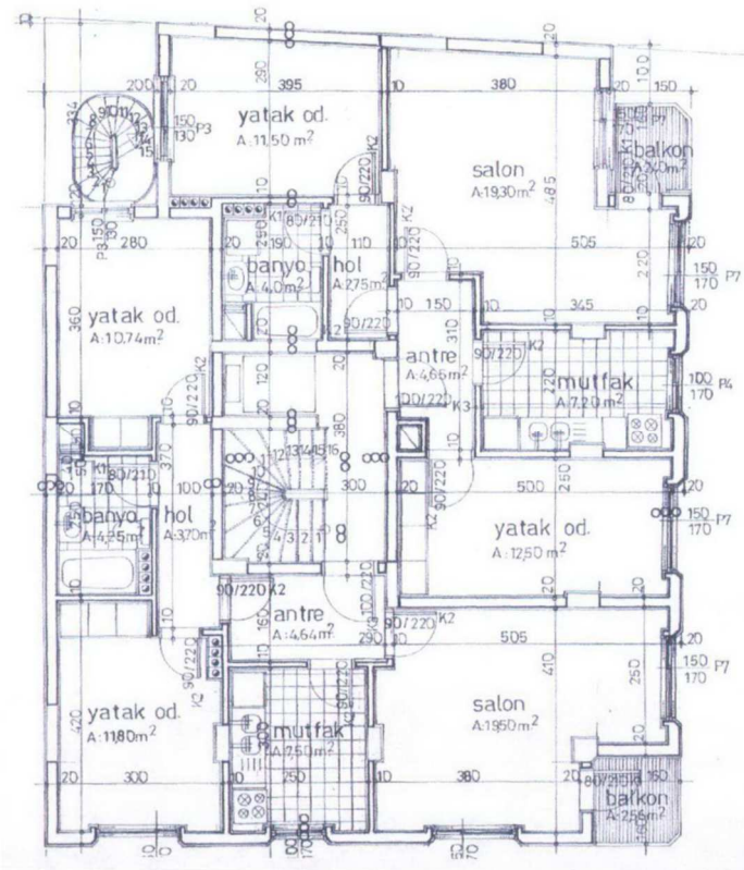
Şekil 5.13. Erdoğan Şair Apartmanı Normal Kat Planı (Ç.B. Arşivi)
