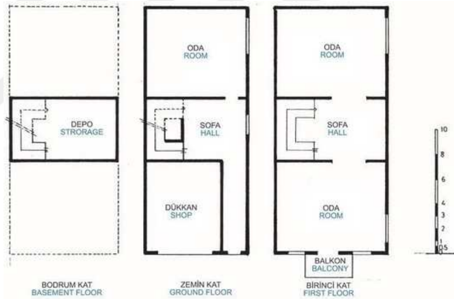
Şekil 4.2. Çanakkale Geleneksel Konutu Plan Örneği (ÇEYAP, 2006)
