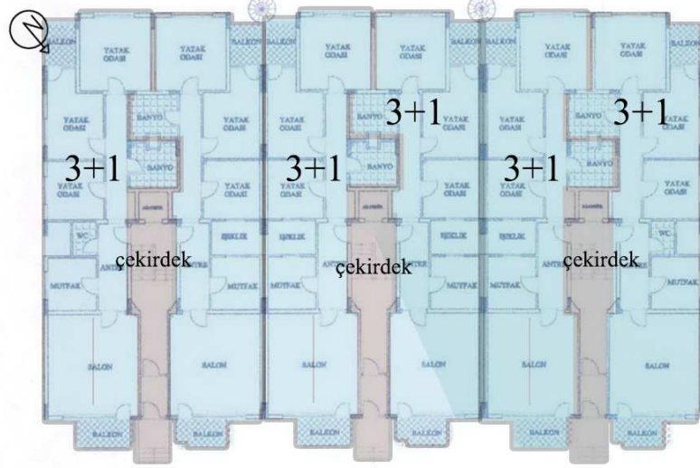
Şekil 5.34. Yeni Kordon Sitesi A-B-C Tipi Giriş Kat Planı (Ç.B. Arşivi)
