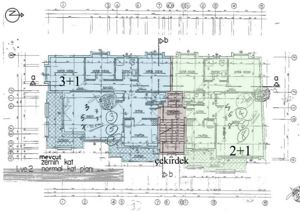
Şekil 5.49. Kent Apartmanı Normal Kat Planı (Ç.B. Arşivi)
