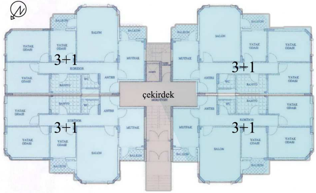
Şekil 5.25. Uğur 96 Koop. Giriş Kat Planı (Ç.B. Arşivi)
