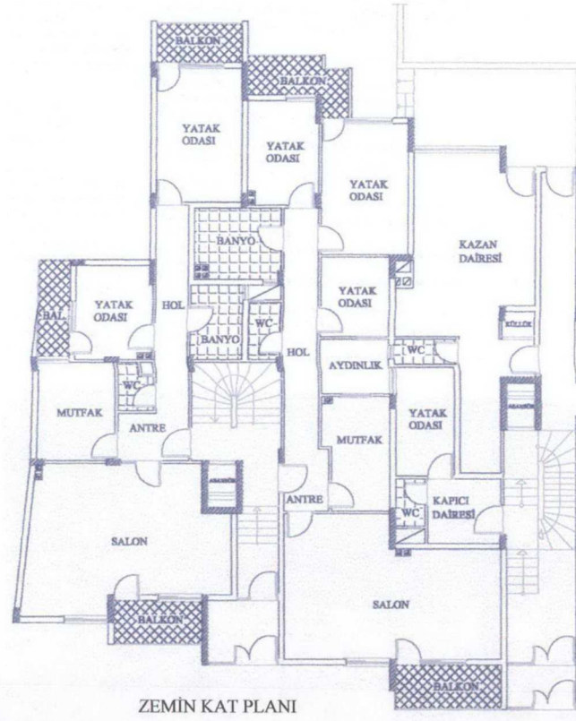
Şekil 5.9. Dura Apartmanı Giriş Kat Planı (Ç.B. Arşivi)
