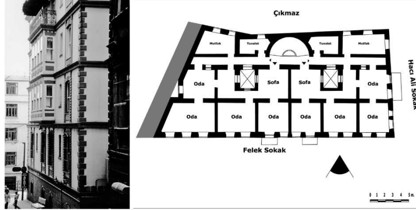
Şekil 2.19. Comando Apartmanı Görsel ve Planı (Öncel, 2014)
