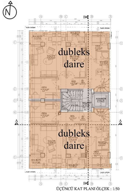
Şekil 5.72. Muğdat Keskin Apartmanı Üçüncü Kat Planı (Aytaç, 2021)
