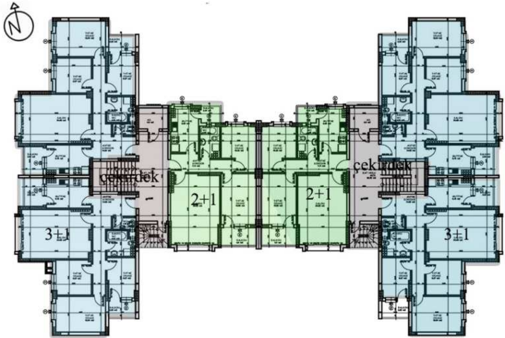
Şekil 5.56. Özgürkent Sitesi A1-A2 Tipi Normal Kat Planı (Ç.B. Arşivi)
