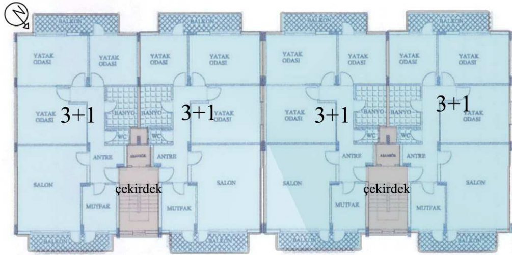
Şekil 5.38. Yeni Kordon Sitesi E-F Tipi Giriş Kat Planı (Ç.B. Arşivi)
