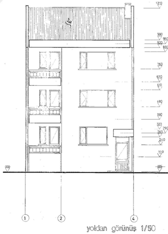
Şekil 5.32. Turhan Karakaya Apartmanı Bombacı Veli Sokaktan Görünüş (Ç.B. Arşivi)
