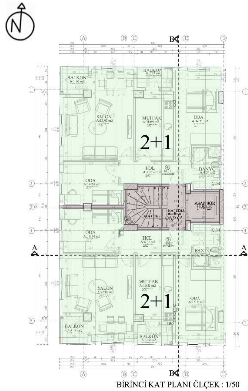
Şekil 5.71. Muğdat Keskin Apartmanı Normal Kat Planı (Aytaç, 2021)
