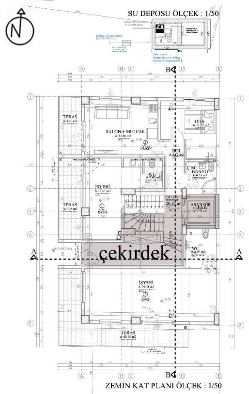
Şekil 5.70. Muğdat Keskin Apartmanı Giriş Kat Planı (Aytaç, 2021)
