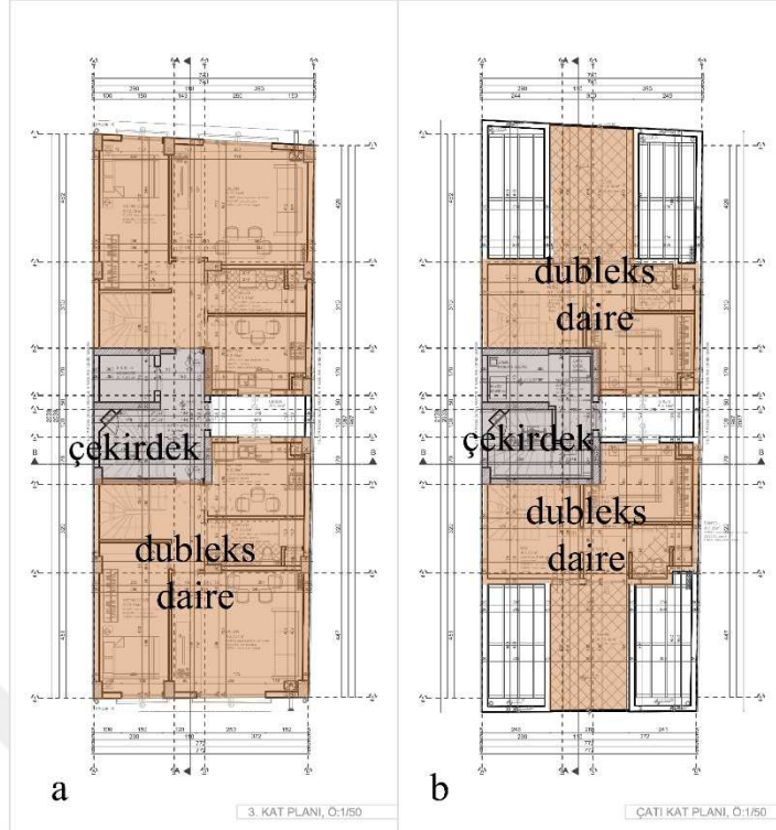
Şekil 5.76. Abdülbari Seçkin Apartmanı Üçüncü Kat ve Çatı Katı Planı a.Üçüncü Kat Planı (Girgin Albayrak, 2022) b. Çatı Katı Planı (Girgin Albayrak, 2022)
