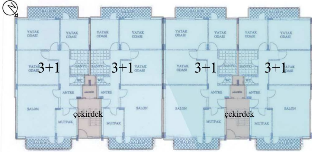
Şekil 5.37. Yeni Kordon Sitesi D Tipi Normal Kat Planı (Ç.B. Arşivi)
