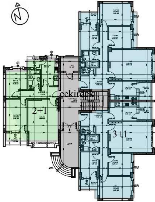
Şekil 5.57. Özgürkent Sitesi D1-D2 Tipi Giriş Kat Planı (Ç.B. Arşivi)
