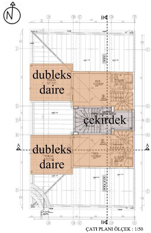
Şekil 5.73. Muğdat Keskin Apartmanı Çatı Katı Planı (Aytaç, 2021)
