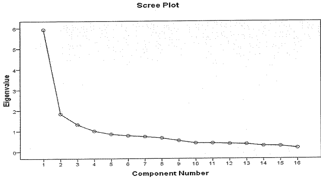
Şekil 6.1. Tüketicilerin gıda satın alma ölçeği faktör çizgi grafiği
