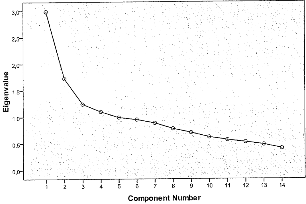
Şekil 6.2. Tüketicilerin gıda tüketim davranışları ölçeği faktör çizgi grafiği
