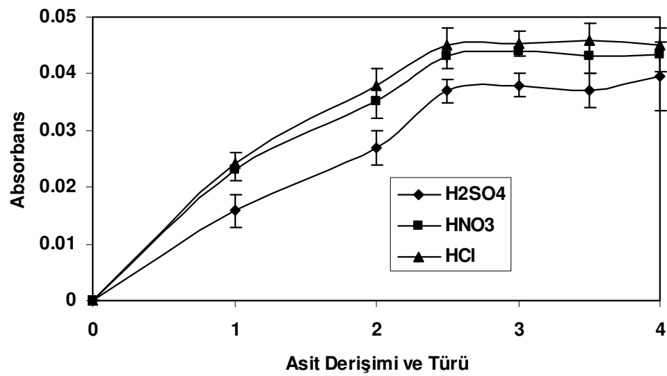
Şekil 3.31. Au(III) iyonlarının geri kazanılmasında elüent türü ve derişiminin etkisi.
