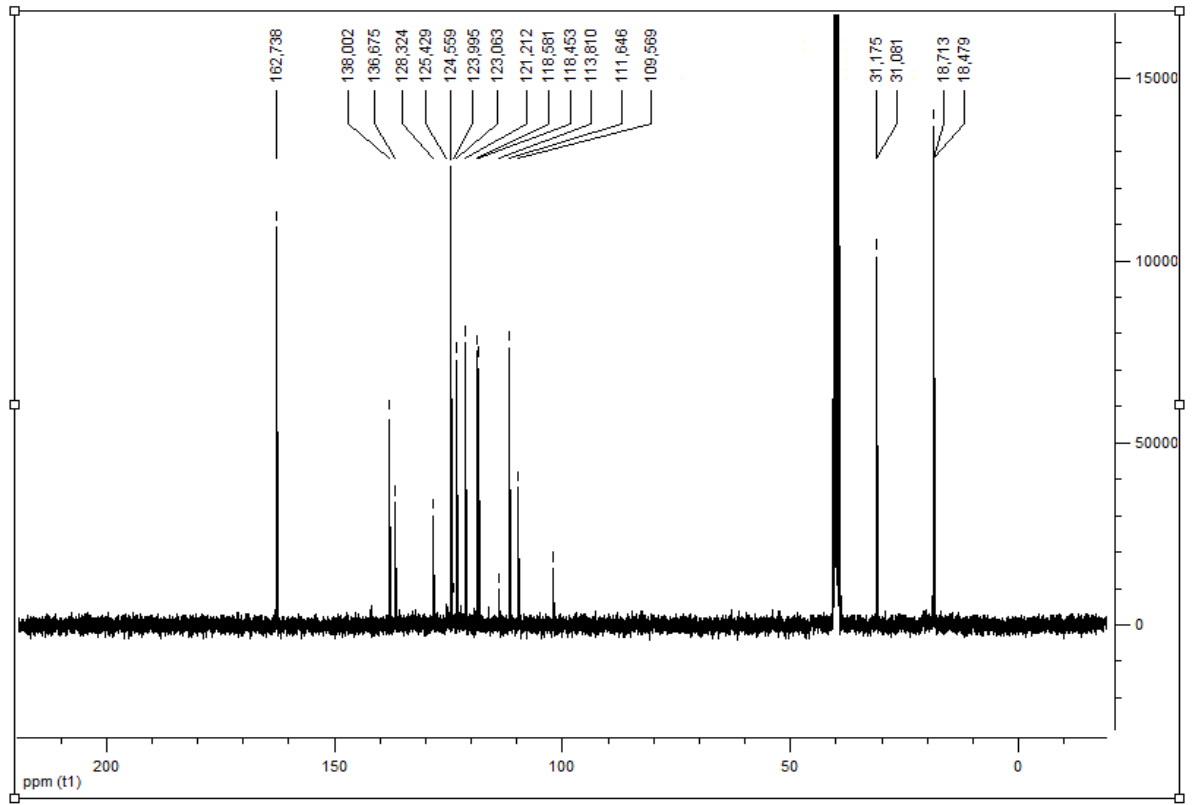
Şekil 3.16. Monomer'in 13 C-NMR spektrumu.
