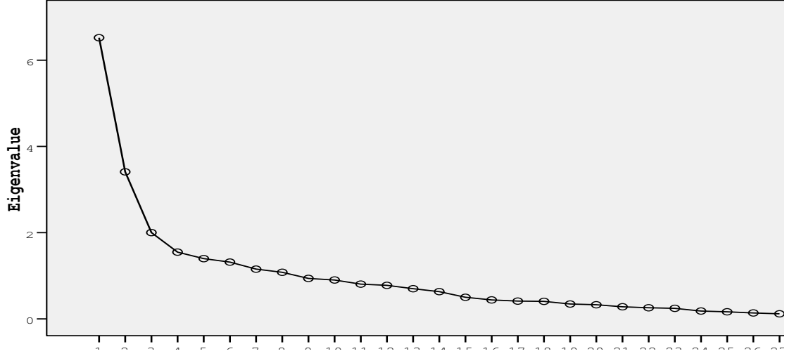
Şekil 9. Öz-değer Grafiği
