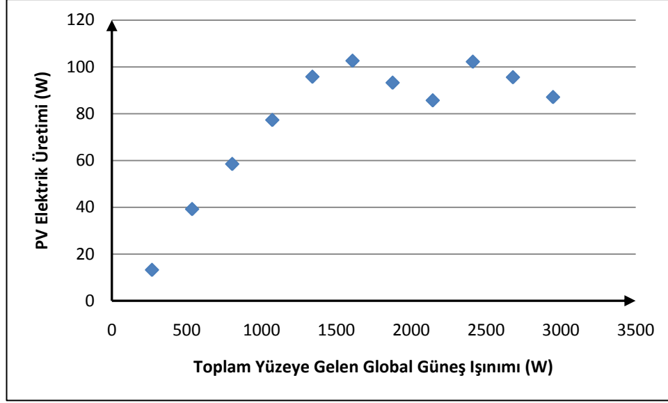
Şekil B.103 : Nisan '10 ayında ortalamadan 0.5 standart sapma düşük PV elektrik üretimi ve toplam yüzeye gelen global güneş ışınımı ilişkisi.
