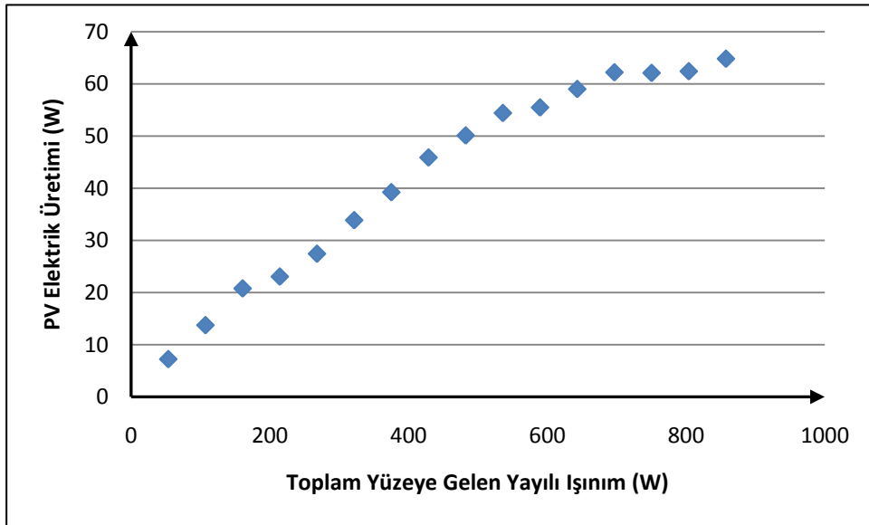
Şekil B.20 : Mart ayında ortalamadan 0.5 standart sapma düşük PV elektrik üretimi ve toplam yüzeye gelen yayılı ışınım ilişkisi.
