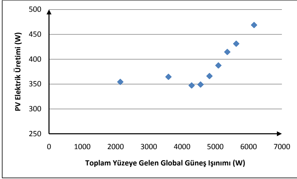
Şekil B.13 : Mart ayında ortalamadan 1.5 standart sapma büyük PV elektrik üretimi ve toplam yüzeye gelen global güneş ışıınımlı ilişkisi.
