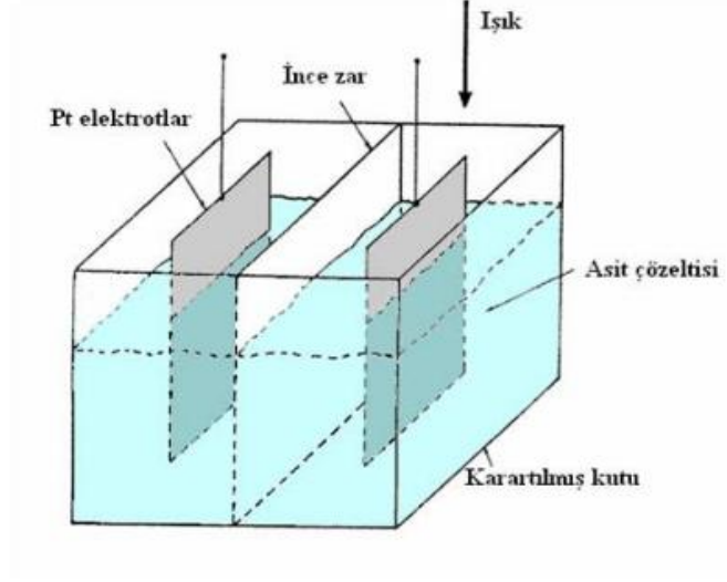
Şekil 2.1 : Becquerel'in fotovoltaik etkiyi gözlemlediği deney düzeneği (Gül, 2008).
