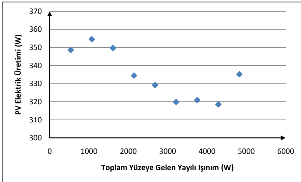
Şekil B.8 : Mart ayında ortalamadan 1 standart sapma büyük PV elektrik üretim değerleri ile toplam yüzeye gelen yayılı ışıınımlı ilişkisi.
