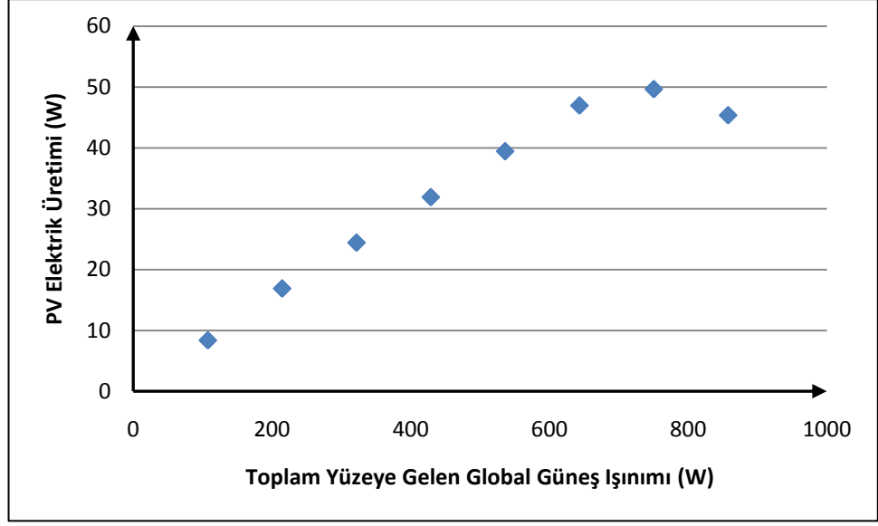
Şekil B.79 : Temmuz '09 ayında ortalamadan 0.5 standart sapma düşük PV elektrik üretimi ve toplam yüzeye gelen global güneş ışıınımlı ilişkisi.
