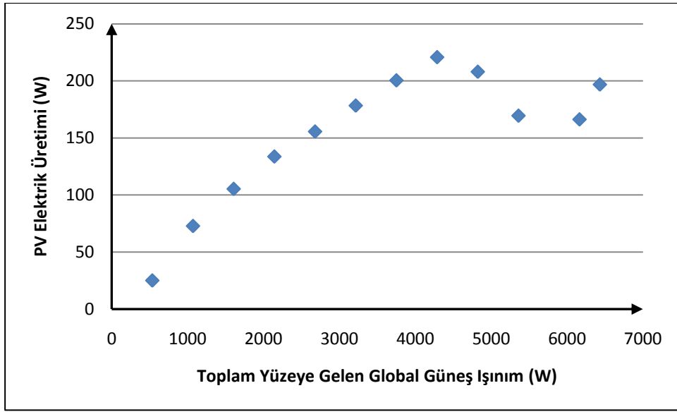
Şekil B.37 : Mayıs '09 ayında toplam yüzeye gelen yayılı ışınlm ve PV elektrik üretimi ilişkisi.
