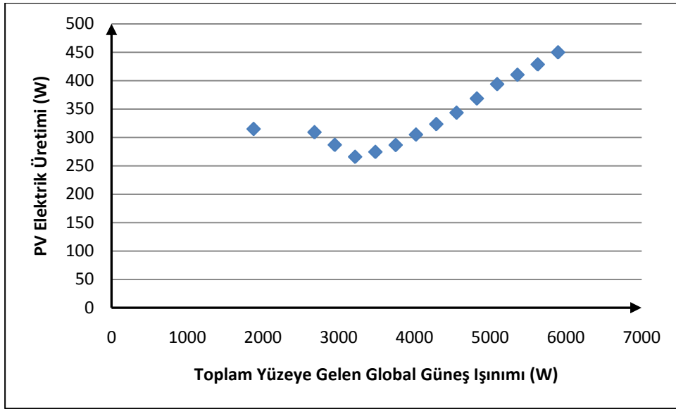
Şekil B.73 : Temmuz '09 ayında ortalamadan 1.5 standart sapma büyük PV elektrik üretimi ve toplam yüzeye gelen global güneş ışıınımlı ilişkisi.
