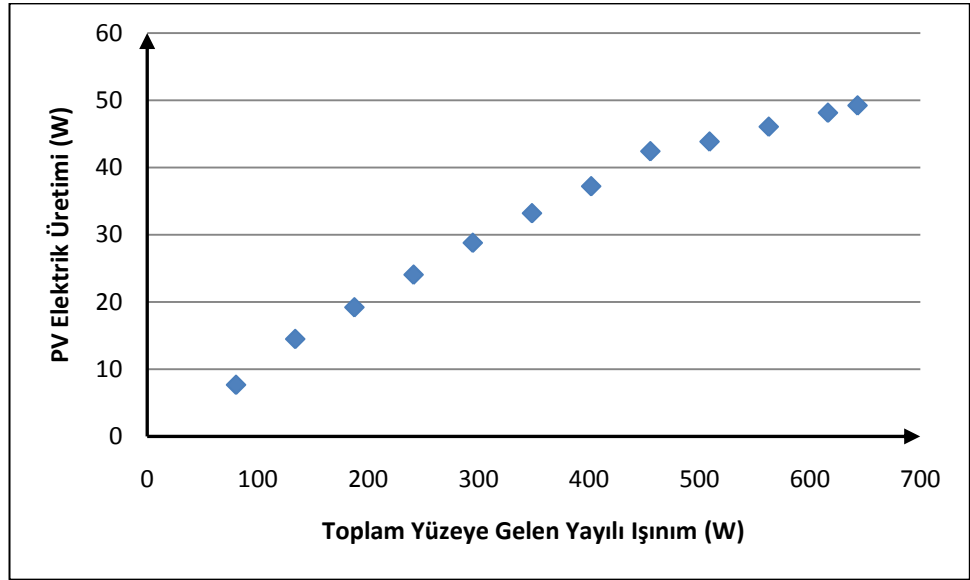
Şekil B.80 : Temmuz '09 ayında ortalamadan 0.5 standart sapma düşük PV elektrik üretimi ve toplam yüzeye gelen yayılı ışıınımlı ilişkisi.
