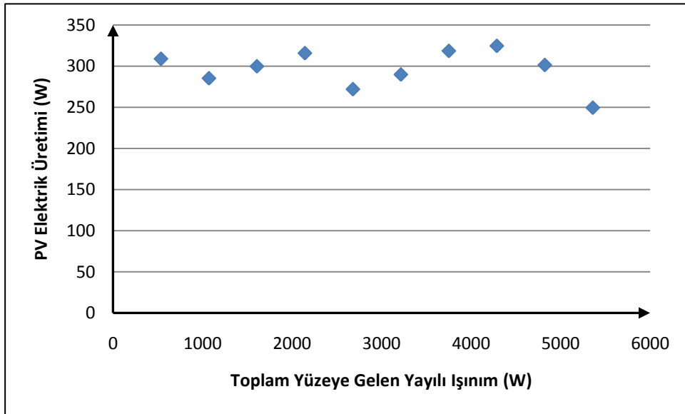
Şekil B.32 : Nisan '09 ayında ortalamadan 1 standart sapma büyük PV elektrik üretim değerleri ile toplam yüzeye gelen yayılı ışıınımlı ilişkisi.
