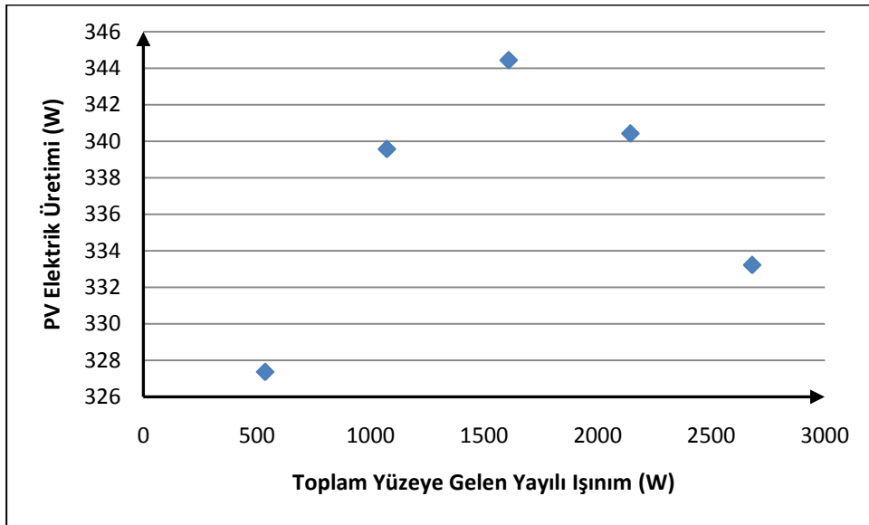
Şekil B.50 : Mayıs '09 ayında ortalamadan 1.5 standart sapma büyük PV elektrik üretimi ve toplam yüzeye gelen yayılı ışıınımlı ilişkisi.
