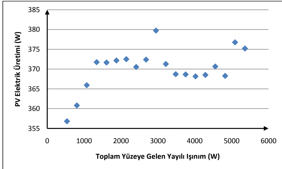
Şekil 4.22 : Ortalamadan 1.5 standart sapma yukarı ve gruplara ayrılmış PV elektrik üretimi ile toplam yüzeye gelen yayılı ışınım ilişkisi.
