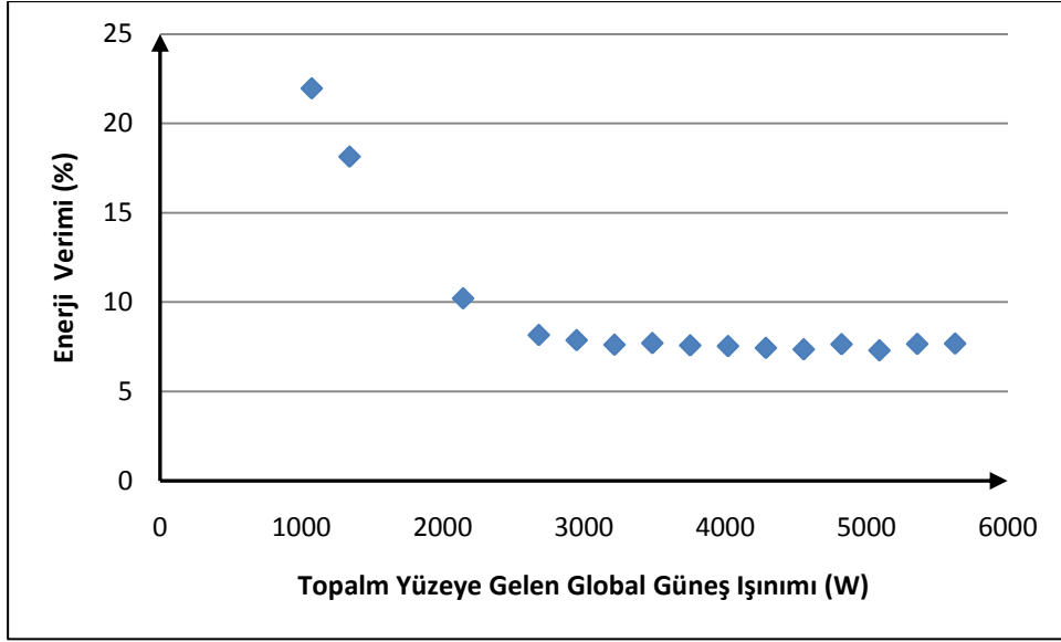
Şekil 4.79 : Şubat ayında ortalamadan 1 standart sapma yukarı PV elektrik üretimi ve toplam yüzeye gelen global güneş ışıınımlı ilişkisi.
