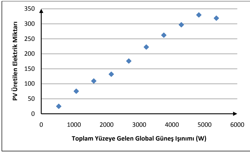
Şekil B.25 : Nisan '09 ayında toplam yüzeye gelen global güneş ışıını ve PV elektrik üretimi ilişkisi.
