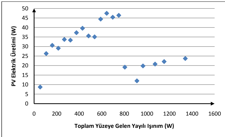
Şekil 4.28 : Ortalamadan 0.5 standart sapma küçük ve gruplara ayrılmış PV elektrik üretimi ile toplam yüzeye gelen yayılı ışıınım ilişkisi.
