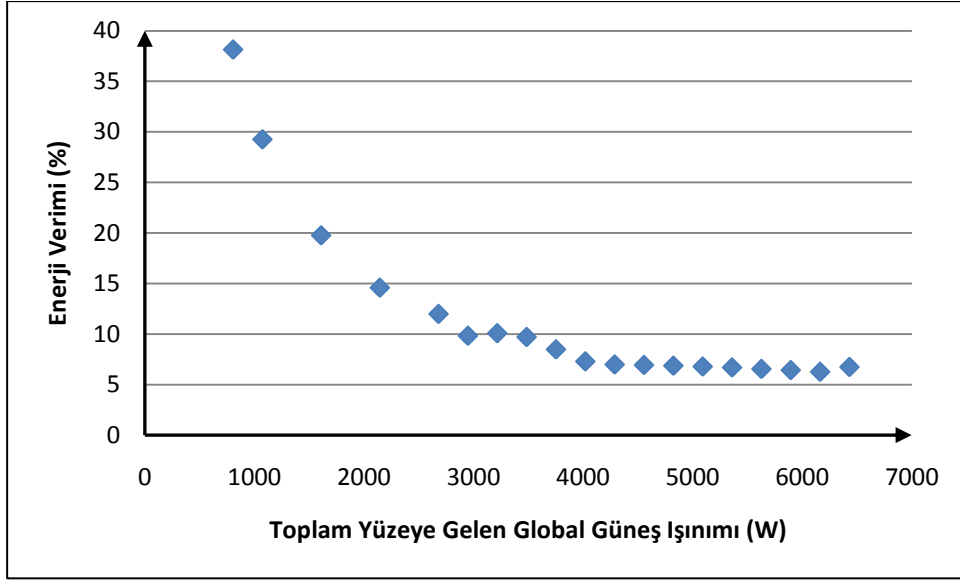
Şekil 4.42 : Ortalamadan 1 standart sapma büyük verilere karşılık gelen enerji verimliliği ve toplam yüzeye gelen global güneş ışıınımlı ilişkisi.
