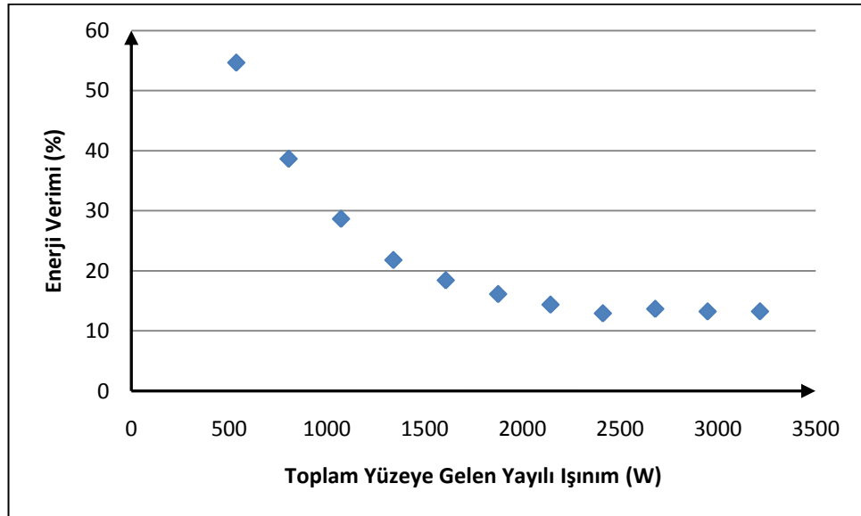
Şekil 4.82 : Şubat ayında ortalamadan 1.5 standart sapma yukarı PV enerji verimlilikleri ve toplam yüzeye gelen yayılı ışınım ilişkisi.
