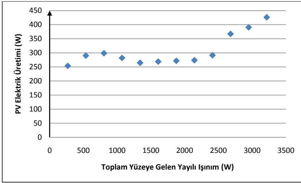
Şekil 4.58 : Şubat ayında ortalamadan 1 standart sapma büyük PV elektrik üretim değerleri ile toplam yüzeye gelen yayılı ışınım ilişkisi.
