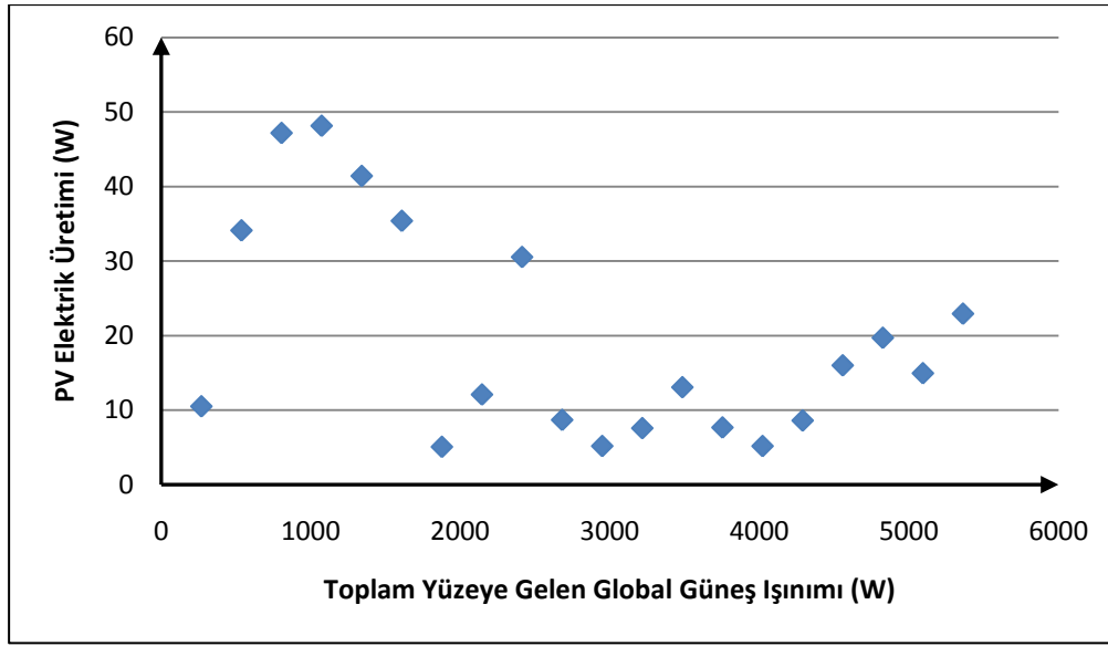
Şekil 4.27 : Ortalamadan 0.5 standart sapma küçük ve gruplara ayrılmış PV elektrik üretimi ile toplam yüzeye gelen global ışıınım ilişkisi.
