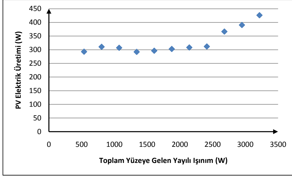
Şekil 4.64 : Şubat ayında ortalamadan 1.5 standart sapma büyük PV elektrik üretimi ve toplam yüzeye gelen yayıllı ışınımı ilişkisi.
