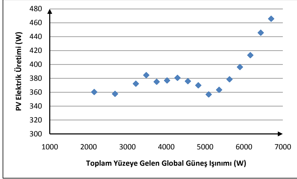
Şekil 4.21 : Ortalamadan 1.5 standart sapma yukarı ve gruplara ayrılmış PV elektrik üretimi ile toplam yüzeye gelen global ışınım ilişkisi.
