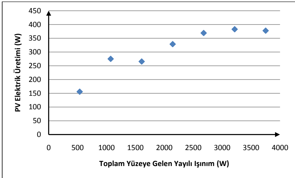
Şekil B.110 : Mayıs '10 ayında toplam yüzeye gelen yayılı ışıını ve PV elektrik üretimi ilişkisi.
