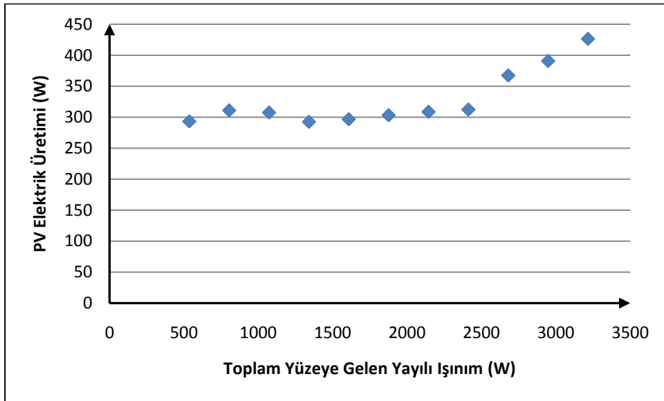
Şekil B.74 : Temmuz '09 ayında ortalamadan 1.5 standart sapma büyük PV elektrik üretimi ve toplam yüzeye gelen yayılı ışıınımlı ilişkisi.
