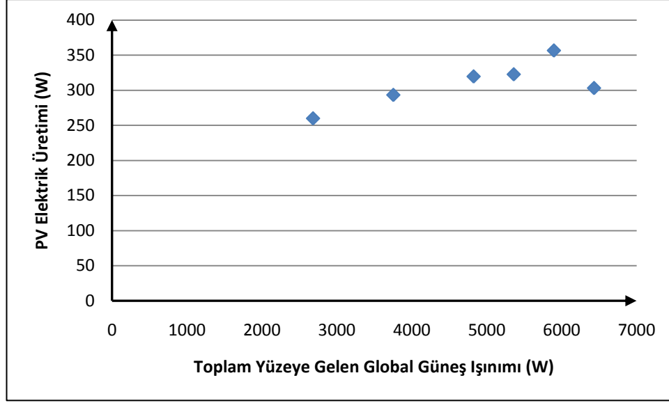
Şekil B.43 : Mayıs '09 ayında ortalamadan 1 standart sapma büyük PV elektrik üretim değerleri ile toplam yüzeye gelen global güneş ışıınımlı ilişkisi.
