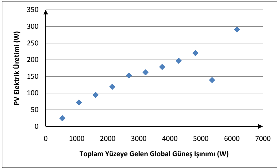
Şekil B.61 : Temmuz '09 ayında toplam yüzeye gelen global güneş ışıını ve PV elektrik üretimi ilişkisi.
