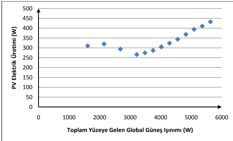
Şekil 4.63 : Şubat ayında ortalamadan 1.5 standart sapma büyük PV elektrik üretimi ve toplam yüzeye gelen global güneş ışıınımı ilişkisi.
