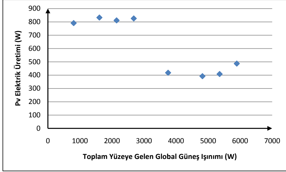
Şekil B.115 : Mayıs '10 ayında ortalamadan 1 standart sapma büyük PV elektrik üretim değerleri ile toplam yüzeye gelen global güneş ışıınımlı ilişkisi.
