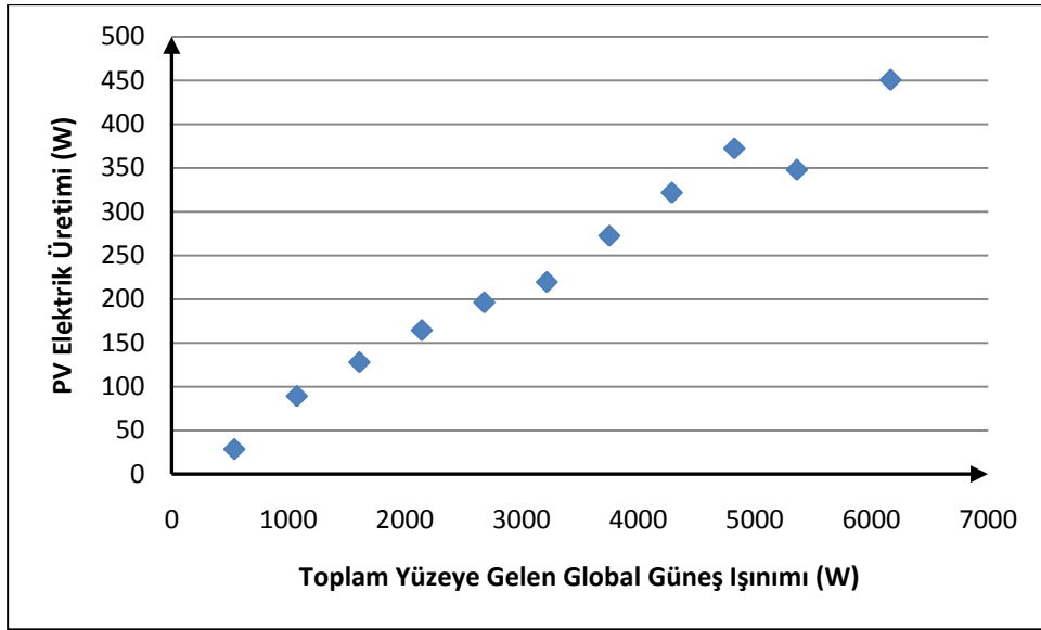
Şekil B.109 : Mayıs '10 ayında toplam yüzeye gelen global güneş ışıını ve PV elektrik üretimi ilişkisi.
