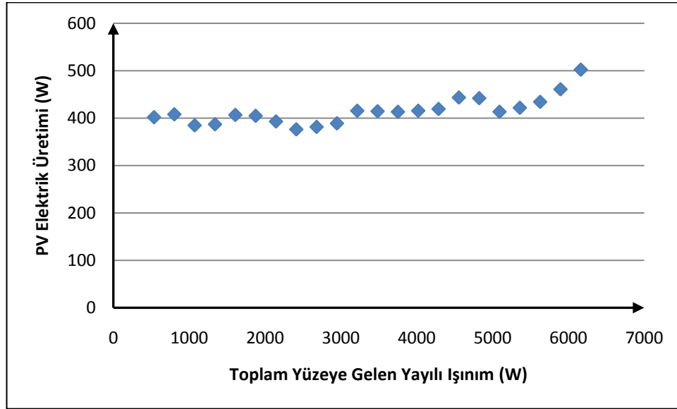
Şekil B.92 : Nisan '10 ayında ortalamadan 1 standart sapma büyük PV elektrik üretim değerleri ile toplam yüzeye gelen yayılı ışıınımlı ilişkisi.
