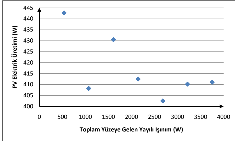
Şekil B.116 : Mayıs '10 ayında ortalamadan 1 standart sapma büyük PV elektrik üretim değerleri ile toplam yüzeye gelen yayılı ışıınımlı ilişkisi.
