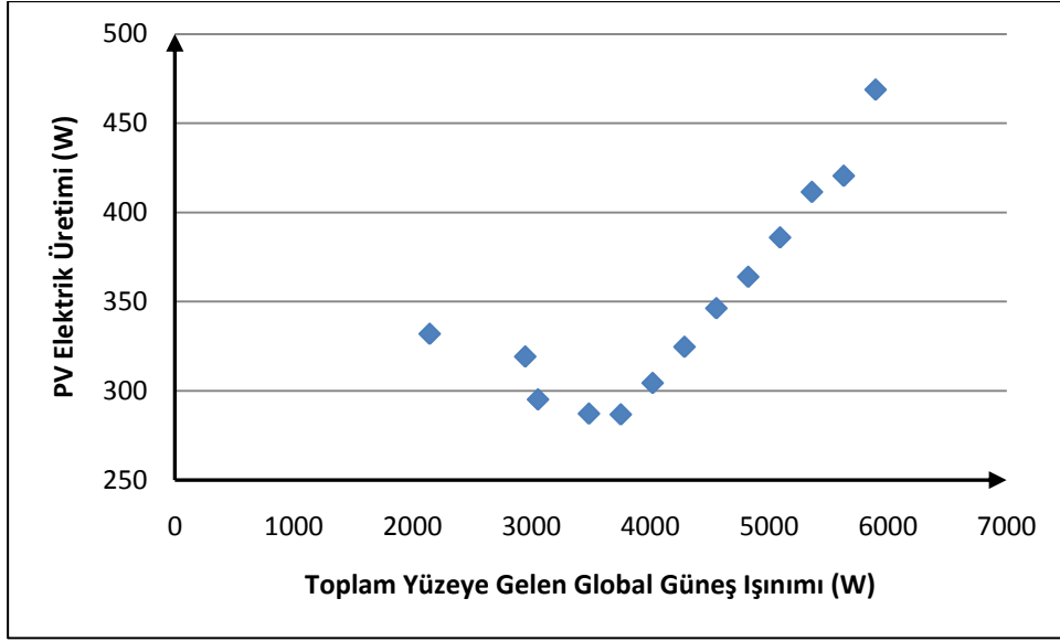
Şekil B.7 : Mart ayında ortalamadan 1 standart sapma büyük PV elektrik üretim değerleri ile toplam yüzeye gelen global güneş ışıınımlı ilişkisi.
