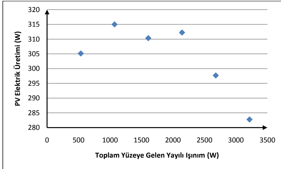
Şekil B.44 : Mayıs '09 ayında ortalamadan 1 standart sapma büyük PV elektrik üretim değerleri ile toplam yüzeye gelen yayıllı ışıınımlı ilişkisi.
