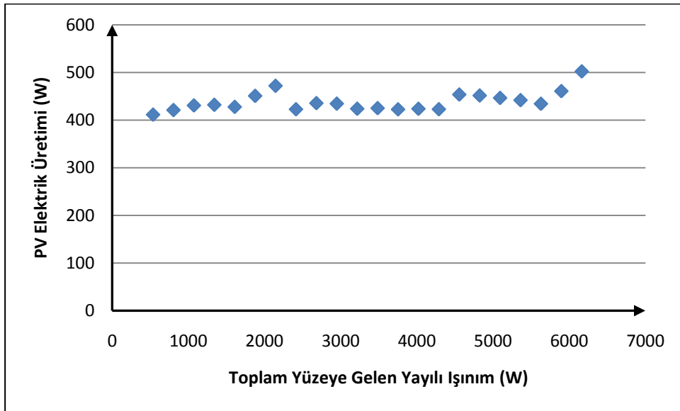
Şekil B.98 : Nisan '10 ayında ortalamadan 1.5 standart sapma büyük PV elektrik üretimi ve toplam yüzeye gelen yayılı ışıınımlı ilişkisi.
