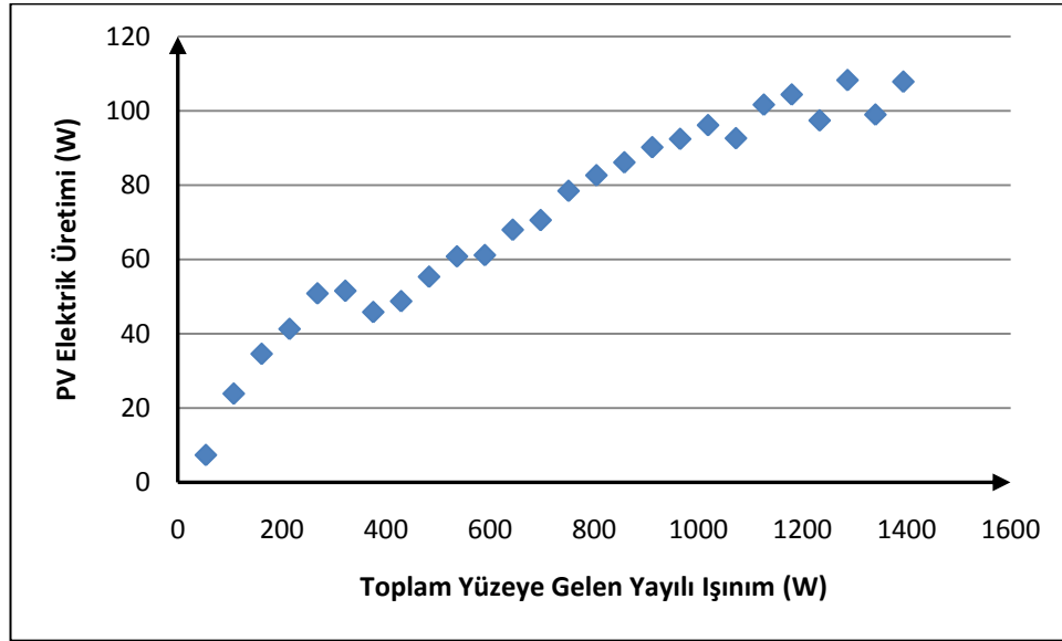
Şekil B.104 : Nisan '10 ayında ortalamadan 0.5 standart sapma düşük PV elektrik üretimi ve toplam yüzeye gelen yayılı ışınım ilişkisi.
