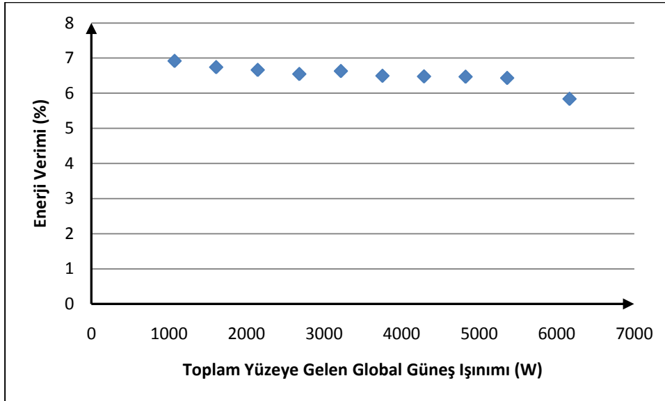
Şekil 4.40 : Toplam yüzeye gelen global güneş ışınlamı ve enerji verimliliği saçılma diyagramı.
