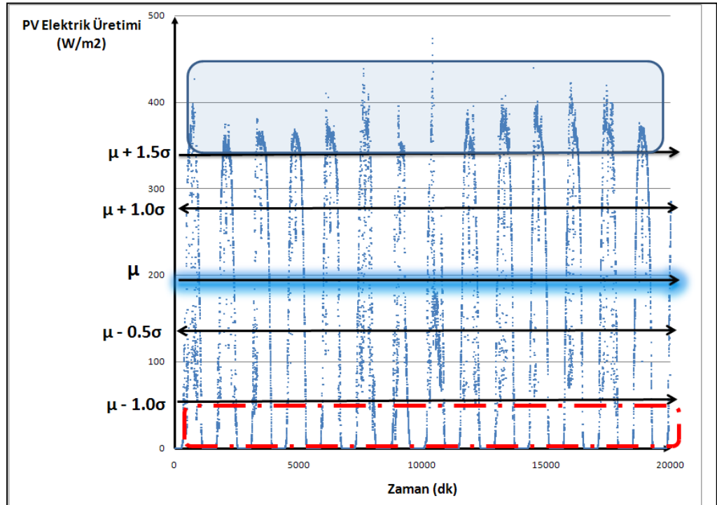
Şekil 4.1 : Ağustos ayı pv güç zaman serisi
