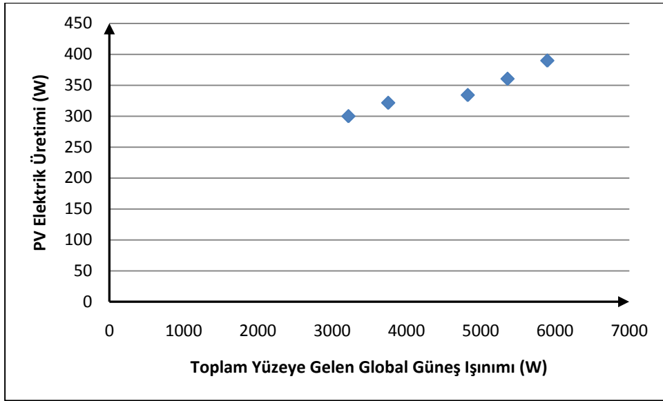
Şekil B.49 : Mayıs '09 ayında ortalamadan 1.5 standart sapma büyük PV elektrik üretimi ve toplam yüzeye gelen global güneş ışıınımlı ilişkisi.
