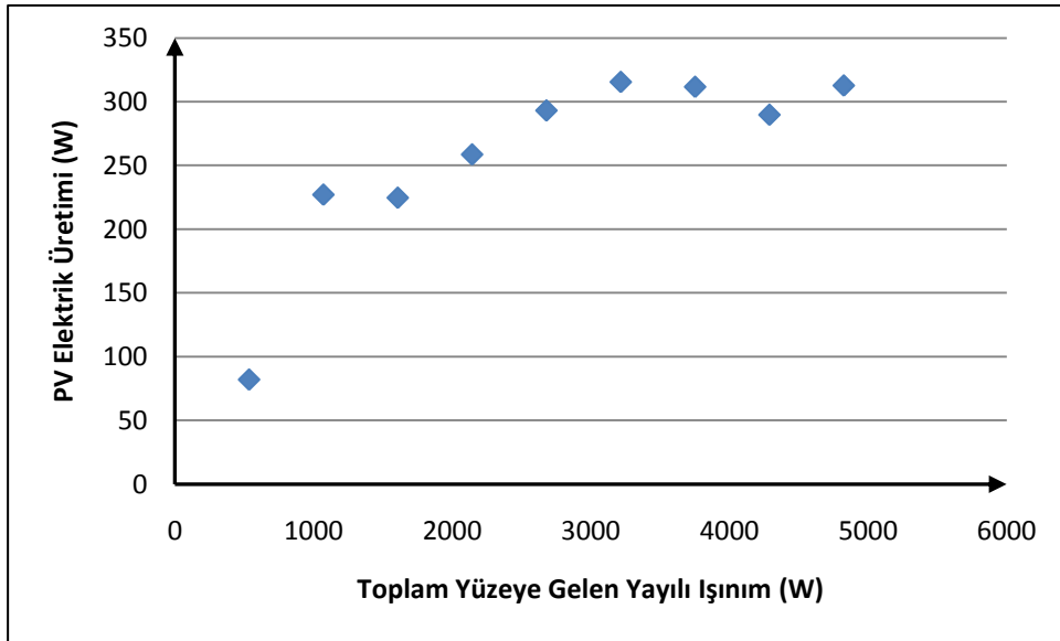
Şekil B.2 : Mart ayında toplam yüzeye gelen yayılı ışınım ve PV elektrik üretimi ilişkisi.
