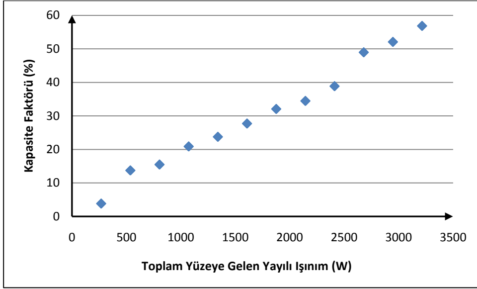
Şekil 4.76 : Şubat ayında toplam yüzeye gelen yayılı ışınım ve kapasite faktörü ilişkisi.
