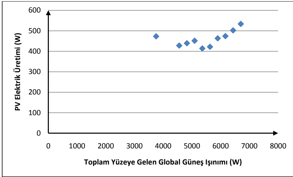
Şekil B.97 : Nisan '10 ayında ortalamadan 1.5 standart sapma büyük PV elektrik üretimi ve toplam yüzeye gelen global güneş ışıınımlı ilişkisi.
