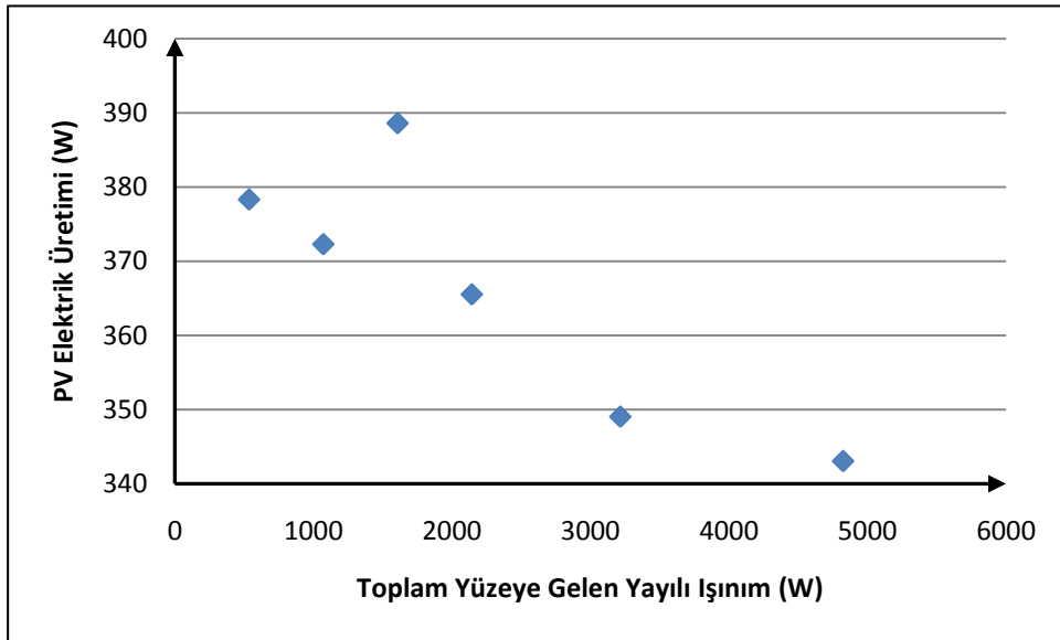
Şekil B.14 : Mart ayında ortalamadan 1.5 standart sapma büyük PV elektrik üretimi ve toplam yüzeye gelen yayılı ışıınımlı ilişkisi.
