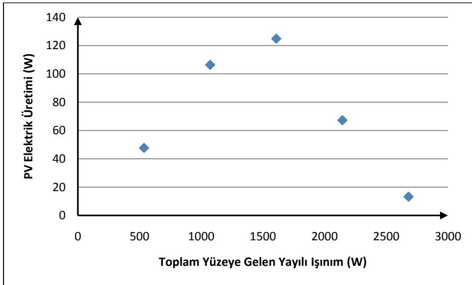
Şekil B.122 : Mayıs '10 ayında ortalamadan 0.5 standart sapma düşük PV elektrik üretimi ve toplam yüzeye gelen yayılı ışıınımlı ilişkisi.
