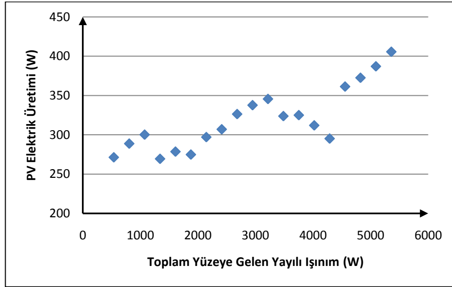
Şekil B.68 : Temmuz '09 ayında ortalamadan 1 standart sapma büyük PV elektrik üretim değerleri ile toplam yüzeye gelen yayılı ışıınımlı ilişkisi.
