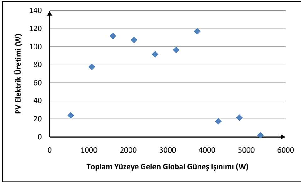
Şekil B.121 : Mayıs '10 ayında ortalamadan 0.5 standart sapma düşük PV elektrik üretimi ve toplam yüzeye gelen global güneş ışıınımlı ilişkisi.
