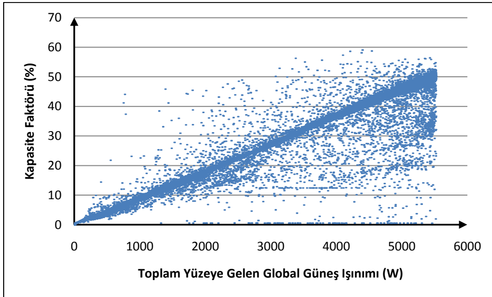
Şekil 4.33 : Toplam yüzeye gelen global güneş ışıını ve kapasite faktörü arasındaki saçılma diyagramı.
