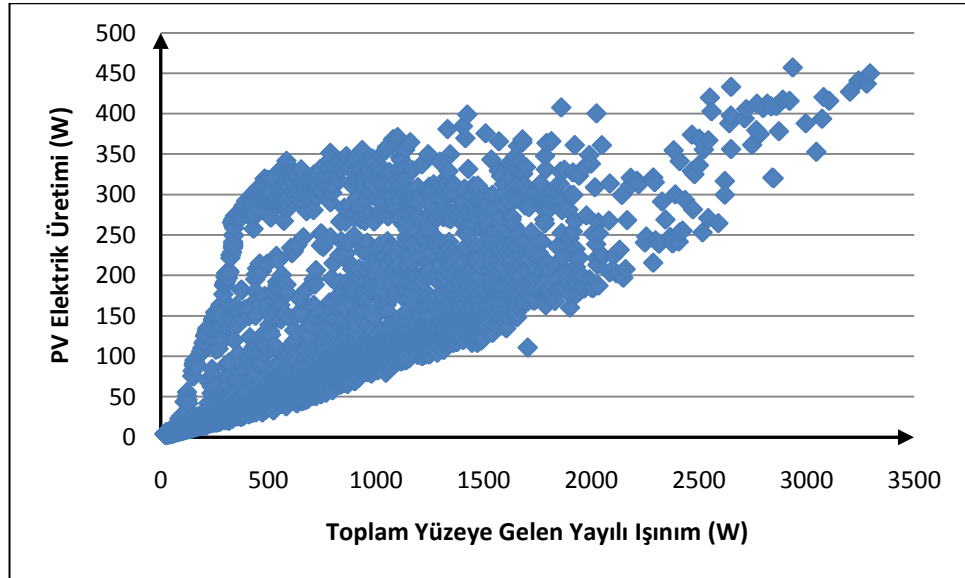
Şekil 4.51 : Şubat ayında toplam yüzeye gelen yayılı ışıını ve PV elektrik üretimi arasındaki saçılma diyagramı.
