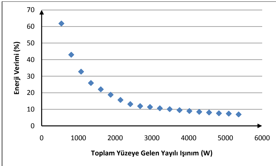
Şekil 4.43 : Ortalamadan 1 standart sapma büyük verilere karşılık gelen enerji verimliliği ve toplam yüzeye gelen yayılı ışıınımlı ilişkisi.
