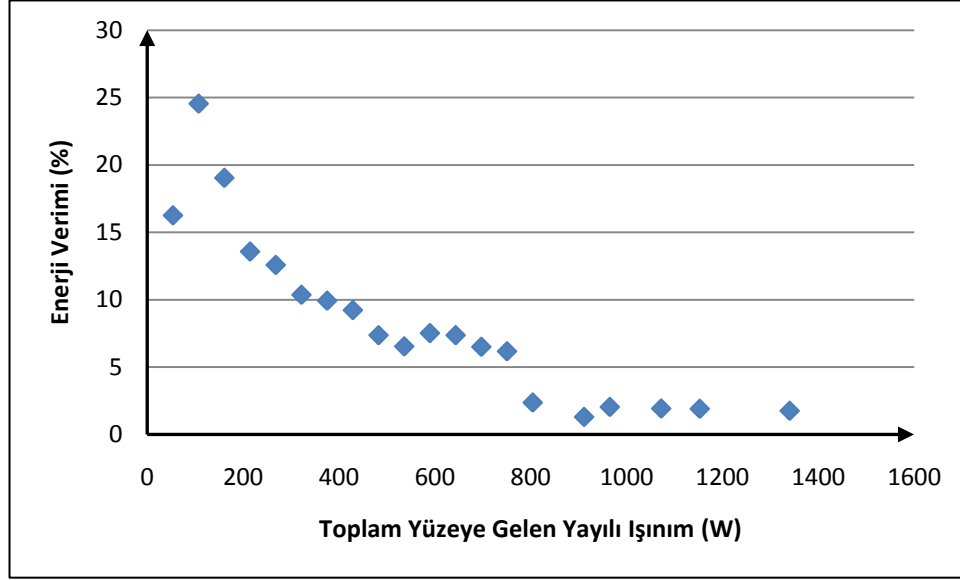
Şekil 4.47 : Ortalamadan 0.5 standart sapma düşük verilere karşılık gelen enerji verimliliği ve toplam yüzeye gelen yayılı ışıınım ilişkisi.
