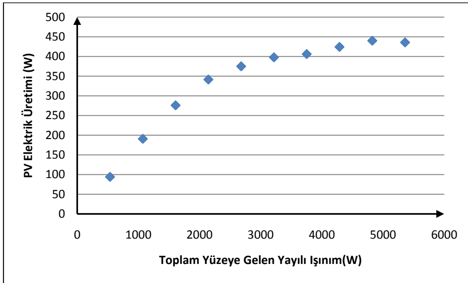
Şekil B.86 : Nisan '10 ayında toplam yüzeye gelen yayılı ışınlım ve PV elektrik üretimi arasındaki saçılma diyagramı.
