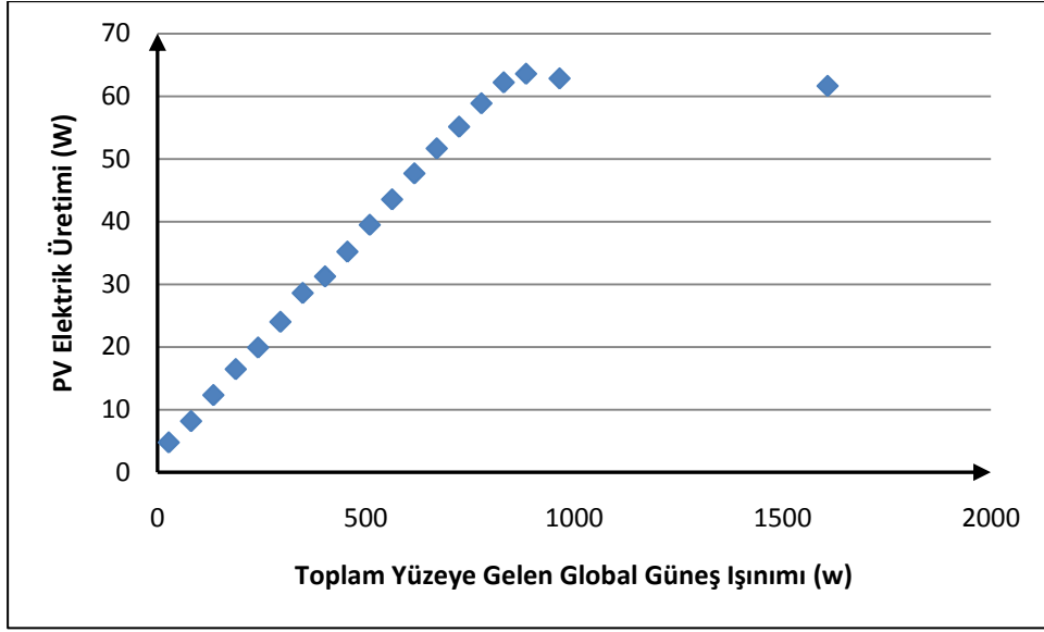
Şekil B.19 : Mart ayında ortalamadan 0.5 standart sapma düşük PV elektrik üretimi ve toplam yüzeye gelen global güneş ışınımı ilişkisi.
