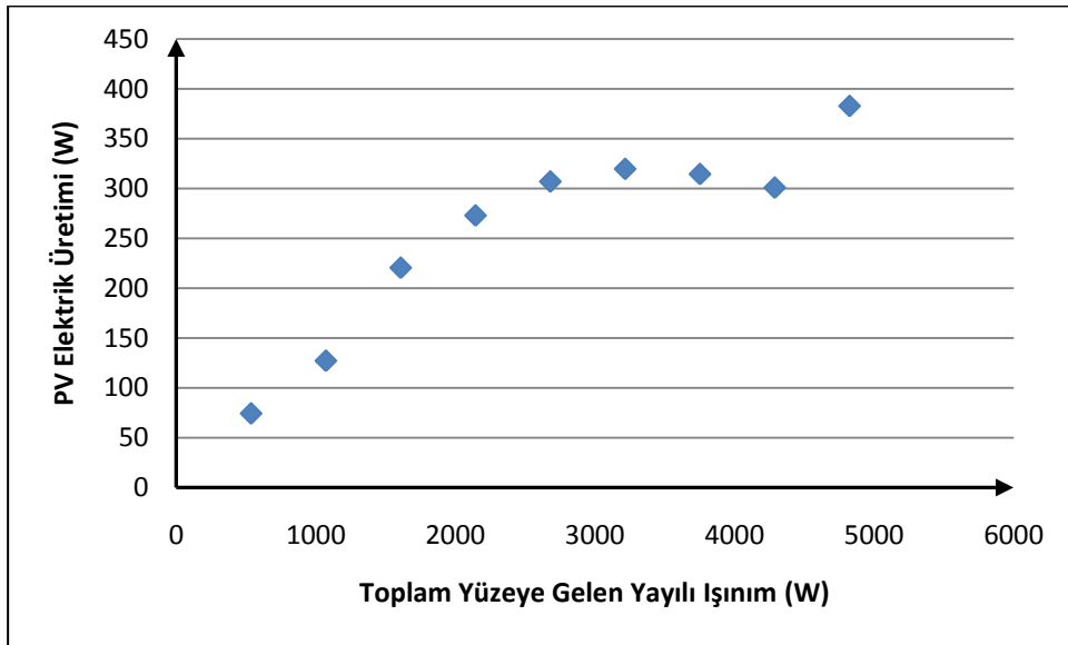
Şekil B.62 : Temmuz '09 ayında toplam yüzeye gelen yayılı ışıını ve PV elektrik üretimi ilişkisi.
