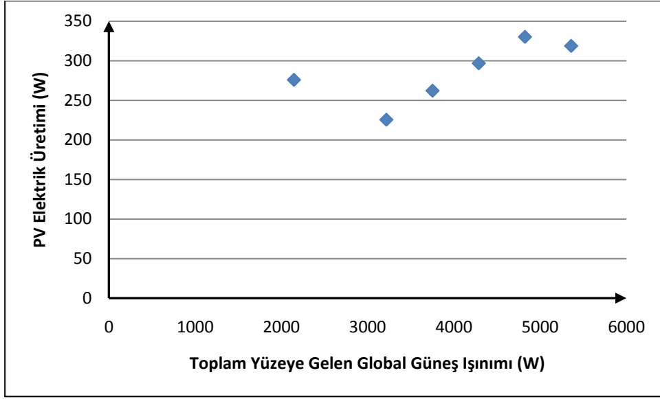
Şekil B.31 : Nisan '09 ayında ortalamadan 1 standart sapma büyük PV elektrik üretim değerleri ile toplam yüzeye gelen global güneş ışıınımlı ilişkisi.
