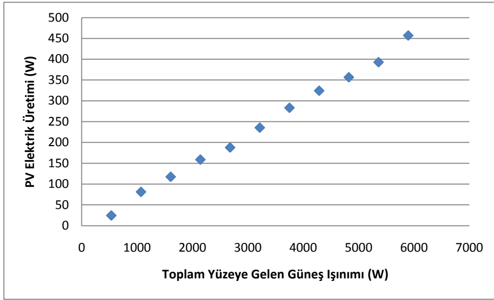
Şekil B.1 : Mart ayında toplam yüzeye gelen güneş ışınımı ve PV elektrik üretimi ilişkisi.
