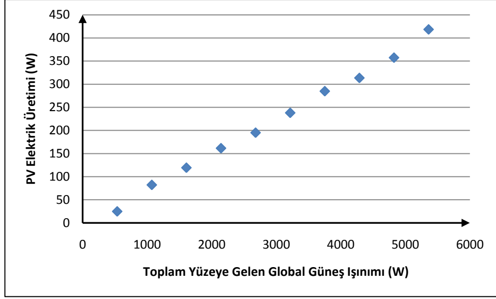
Şekil 4.50 : Şubat ayında toplam yüzeye gelen ortalama global güneş ışıını ve ortalama PV elektrik üretimi arasındaki ilişki.
