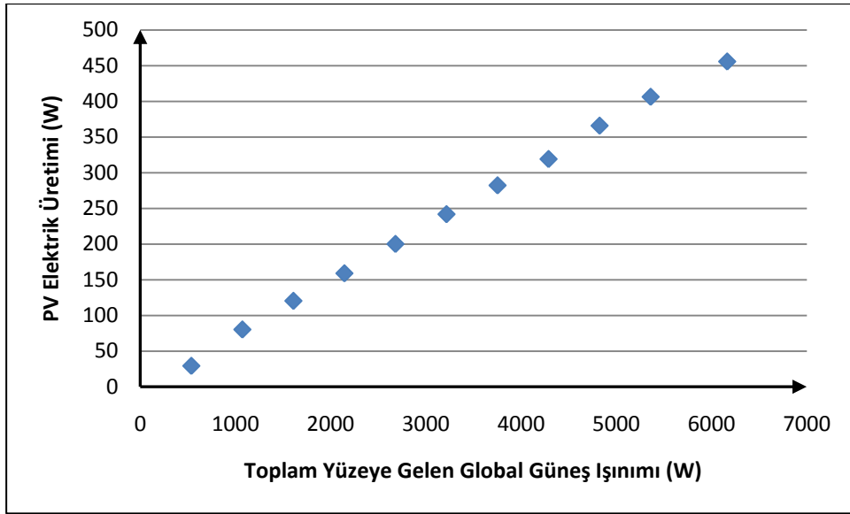
Şekil B.85 : Nisan '10 ayında toplam yüzeye gelen global güneş ışınlımı ve PV elektrik üretimi ilişkisi.
