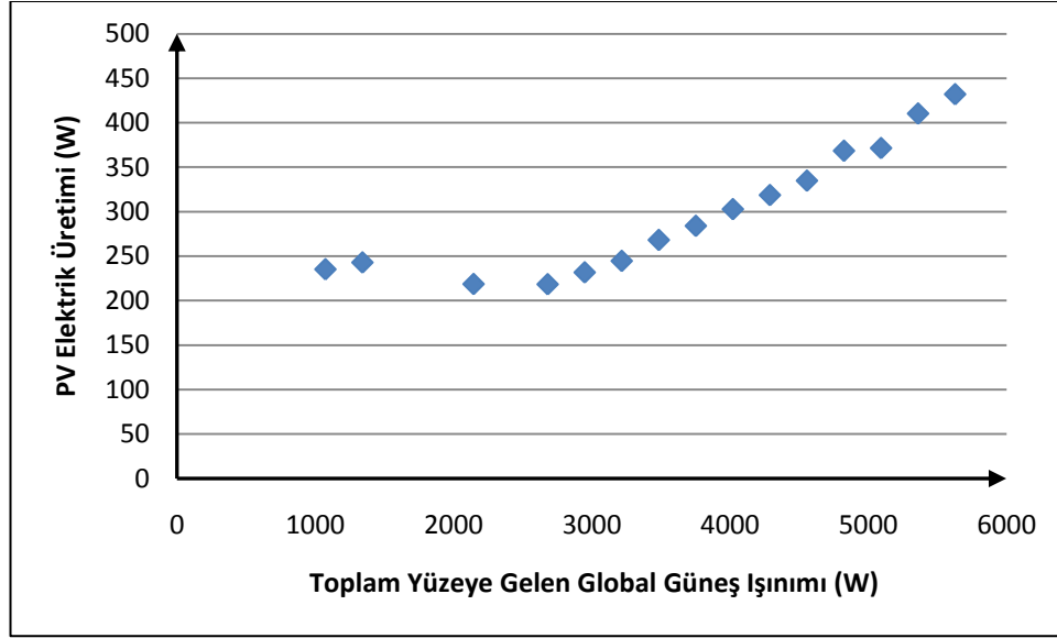
Şekil 4.57 : Şubat ayında ortalamadan 1 standart sapma büyük PV elektrik üretim değerleri ile toplam yüzeğe gelen global güneş ışınımı ilişkisi.
