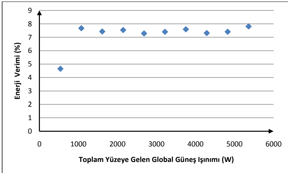
Şekil 4.77 : Şubat ayında toplam yüzeye gelen global güneş ışınımı ve enerji verimliliği ilişkisi.
