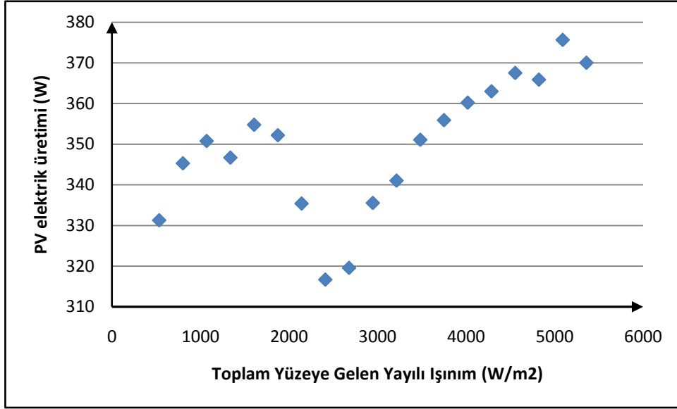
Şekil 4.18 : Ortalamadan 1 standart sapma yukarı ve gruplara ayrılmış PV elektrik üretimi ile toplam yüzeye gelen yayılı ışıını ilişkisi.
