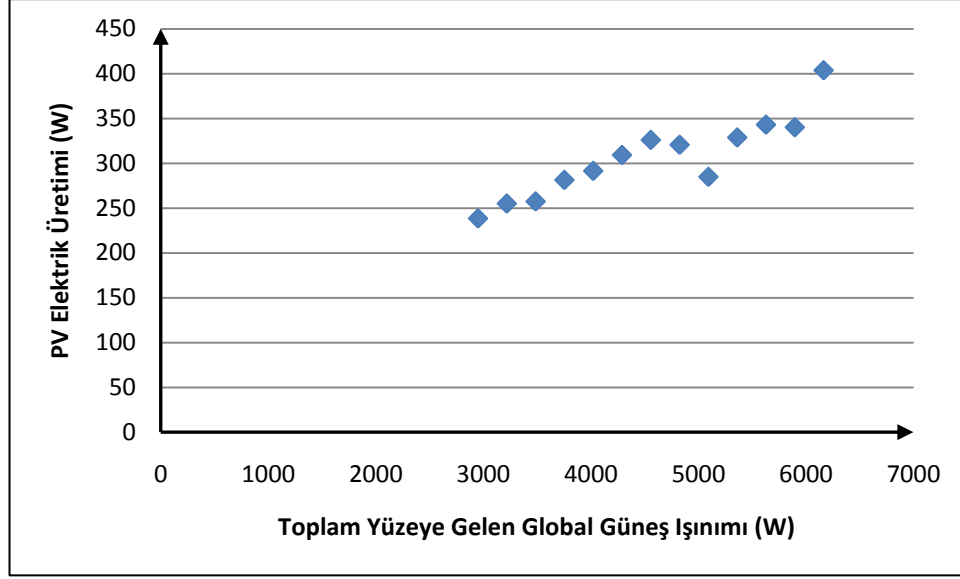
Şekil B.67 : Temmuz '09 ayında ortalamadan 1 standart sapma büyük PV elektrik üretim değerleri ile toplam yüzeye gelen global güneş ışıınımlı ilişkisi.
