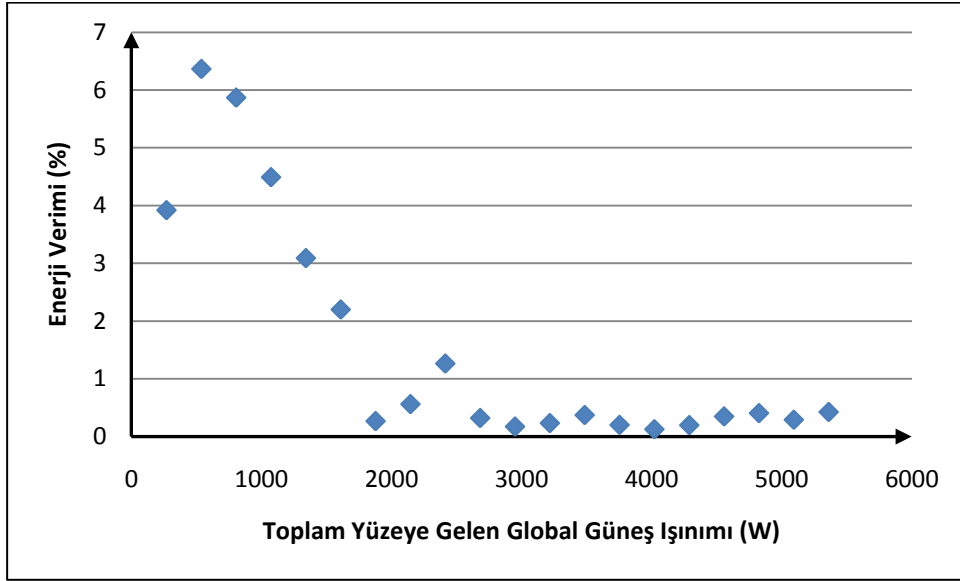
Şekil 4.46 : Ortalamadan 0.5 standart sapma düşük verilere karşılık gelen enerji verimliliği ve toplam yüzeye gelen global güneş ışıınımlı ilişkisi.
