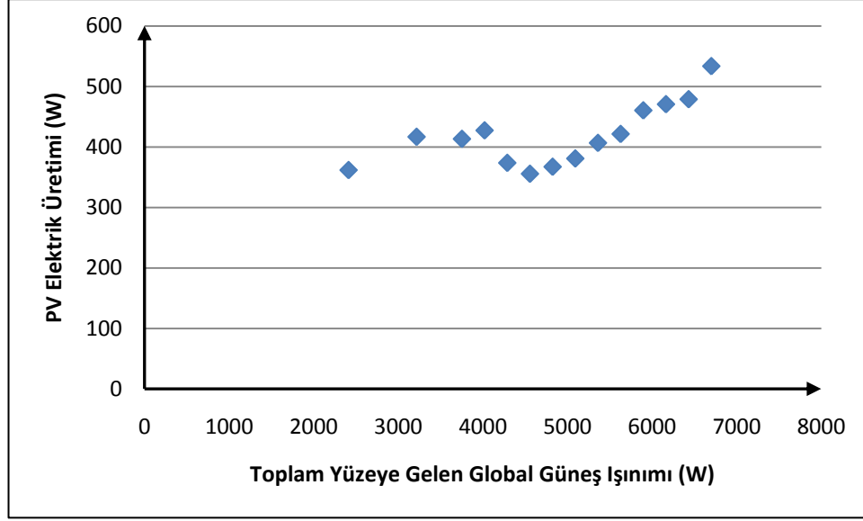
Şekil B.91 : Nisan '10 ayında ortalamadan 1 standart sapma büyük PV elektrik üretim değerleri ile toplam yüzeye gelen global güneş ışıınımlı ilişkisi.
