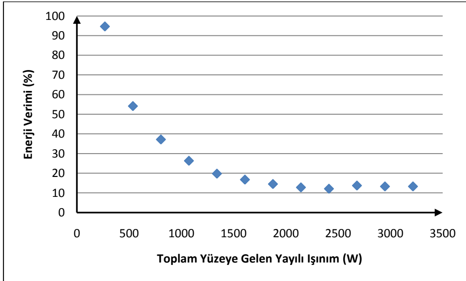
Şekil 4.80 : Şubat ayında ortalamadan 1 standart sapma yukarı PV enerji verimlilikleri ve toplam yüzeye gelen yayılı ışıınımlı ilişkisi.
