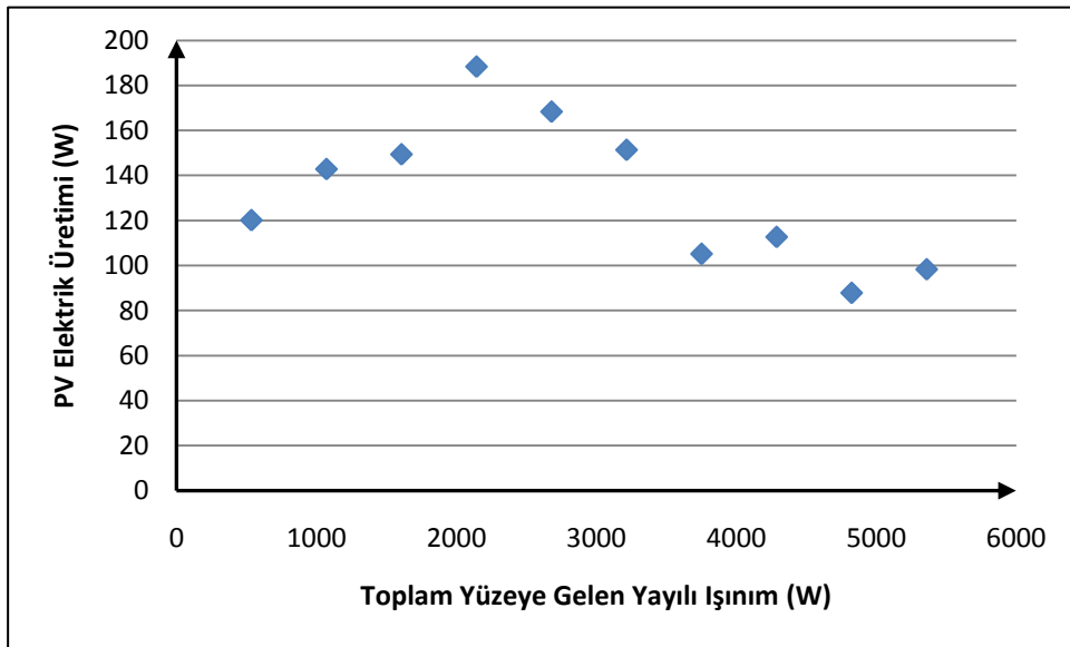
Şekil B.38 : Mayıs '09 ayında toplam yüzeye gelen yayılı ışınlm ve PV elektrik üretimi ilişkisi.
