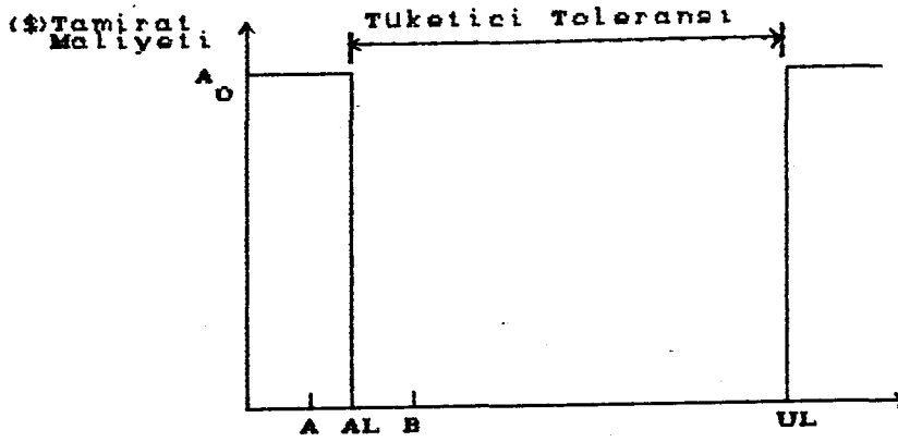
Sekil 2-9; Geleneksel Toleranslama Grafığı [5,4]
