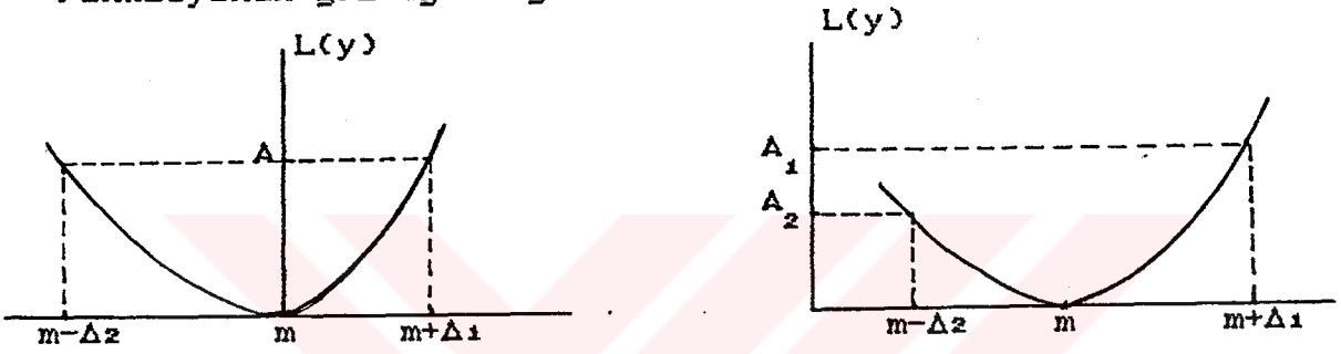
Sekil 2-13; Tolerans Limitleri Farklı İken Kayıp Fonksiyonunun Grafiđi
