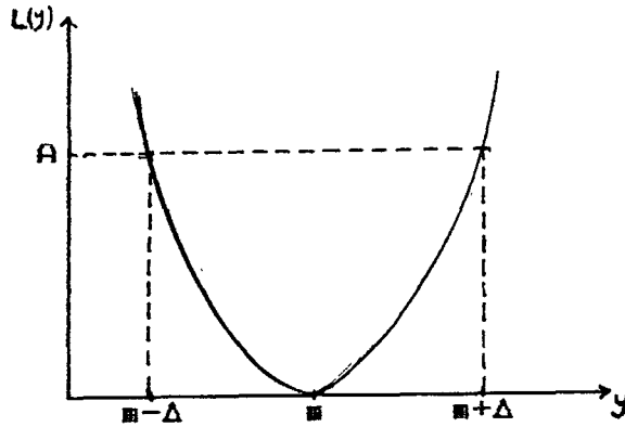
Sekil 2-10; Kayıp Fonksiyonunun Grafığı
