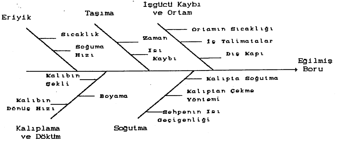
Şekil 3-2 ; Problemin Kılçık Diyagramı
