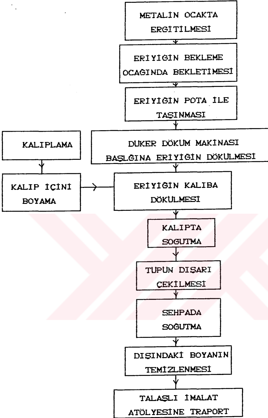
Şekil 3-1 İş Akışı Seması
