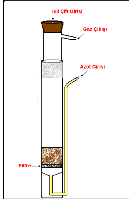
Şekil 3.2 Akışkan yataklı reaktör
