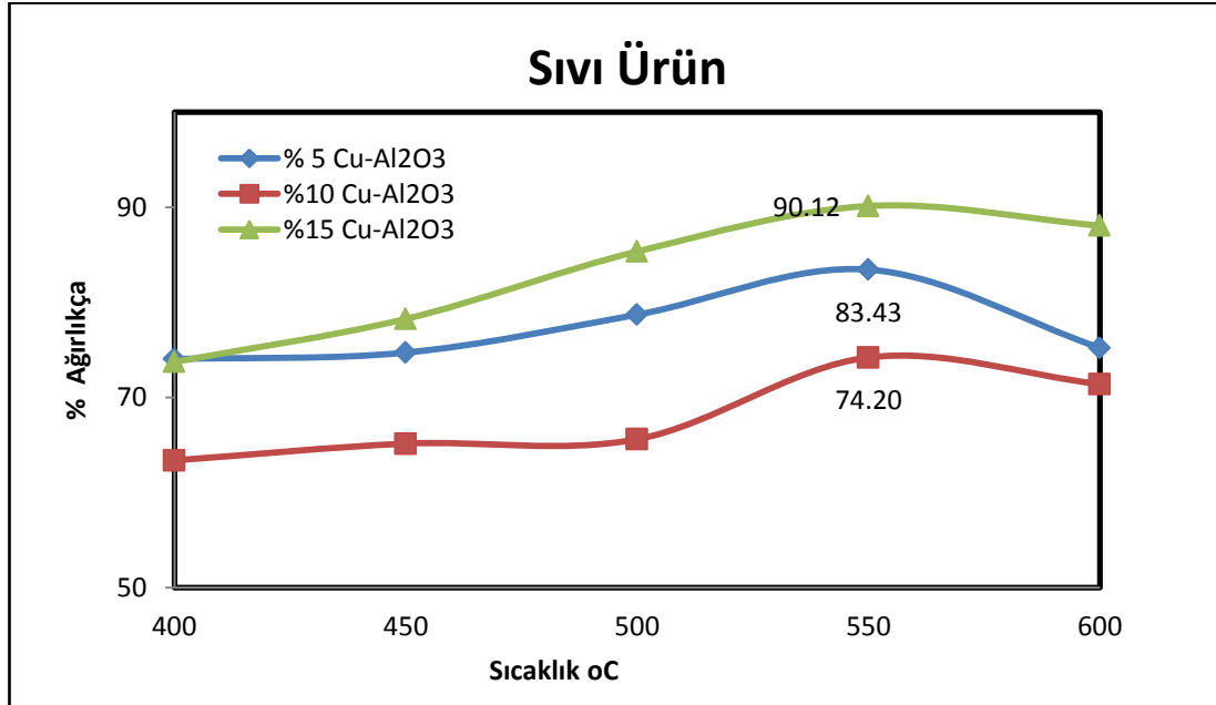
Şekil 4.1 PS'in Cu-Al 2 O 3 katalizörü ile ısı pirolizinde sıvı ürün miktarının sıcaklık ile değişimi
