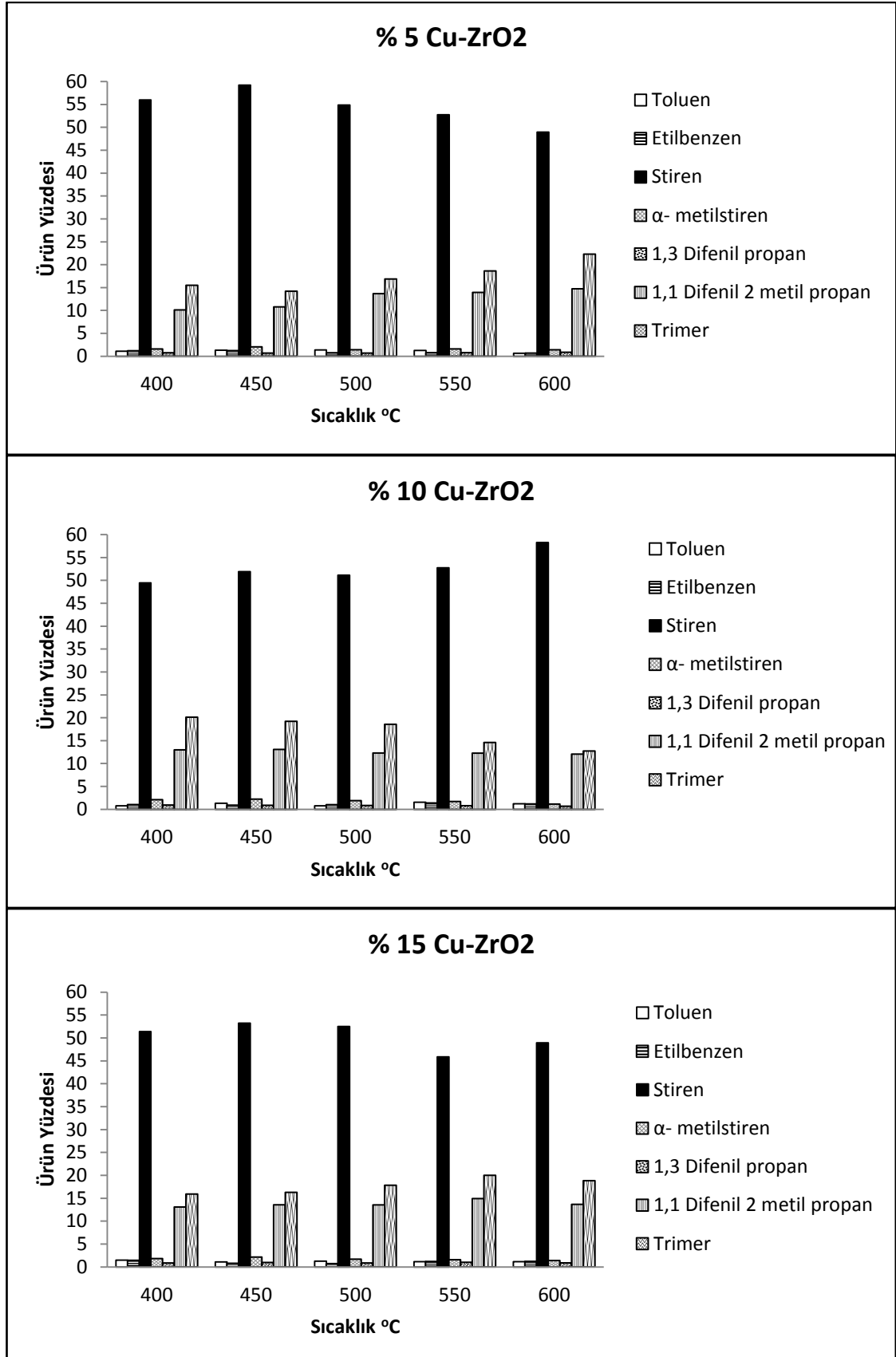
Şekil 4.26 Cu-ZrO 2 katalizörü ile elde edilen sıvı ürün bileşiminin sıcaklıkla değişimi
