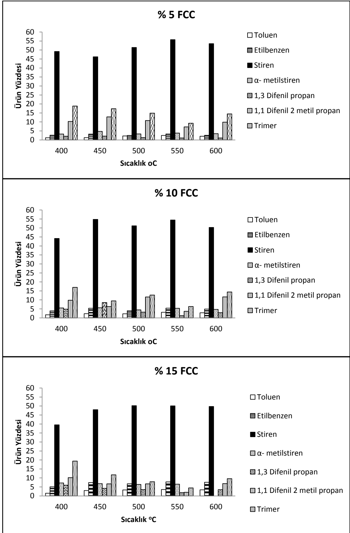
Şekil 4.27 FCC katalizörü ile elde edilen sıvı ürün bileşiminin sıcaklıkla değişimi
