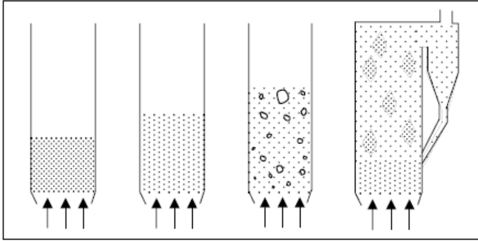
Şekil 2.4 Sabit yatak, minimum akışkanlaşma konumu, kabarcıklı ve dolaşimli akışkan yatak (Oymak ve Batu 2010).
