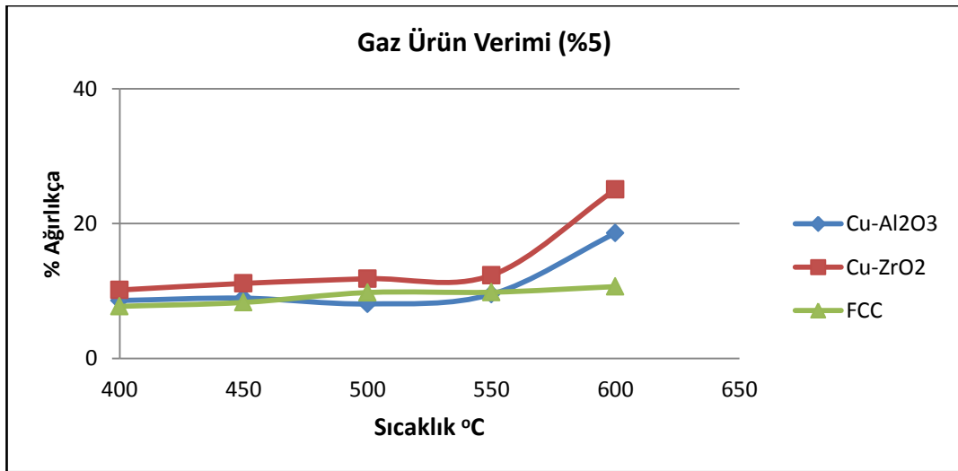
Şekil 4.5 % 5 Katalizör/PS oranında gaz ürün veriminin karşılaştırılması
