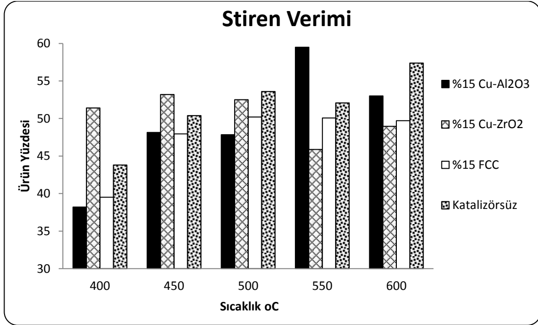
Şekil 4.30 Stiren veriminin %15 katalizör/PS oranı için sıcaklık ile değişimi
