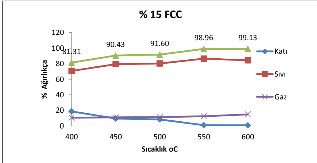
Şekil 4.10 FCC katalizörü varlığında katı-sıvı ve gaz ürünlerin sıcaklıkla değişimi
