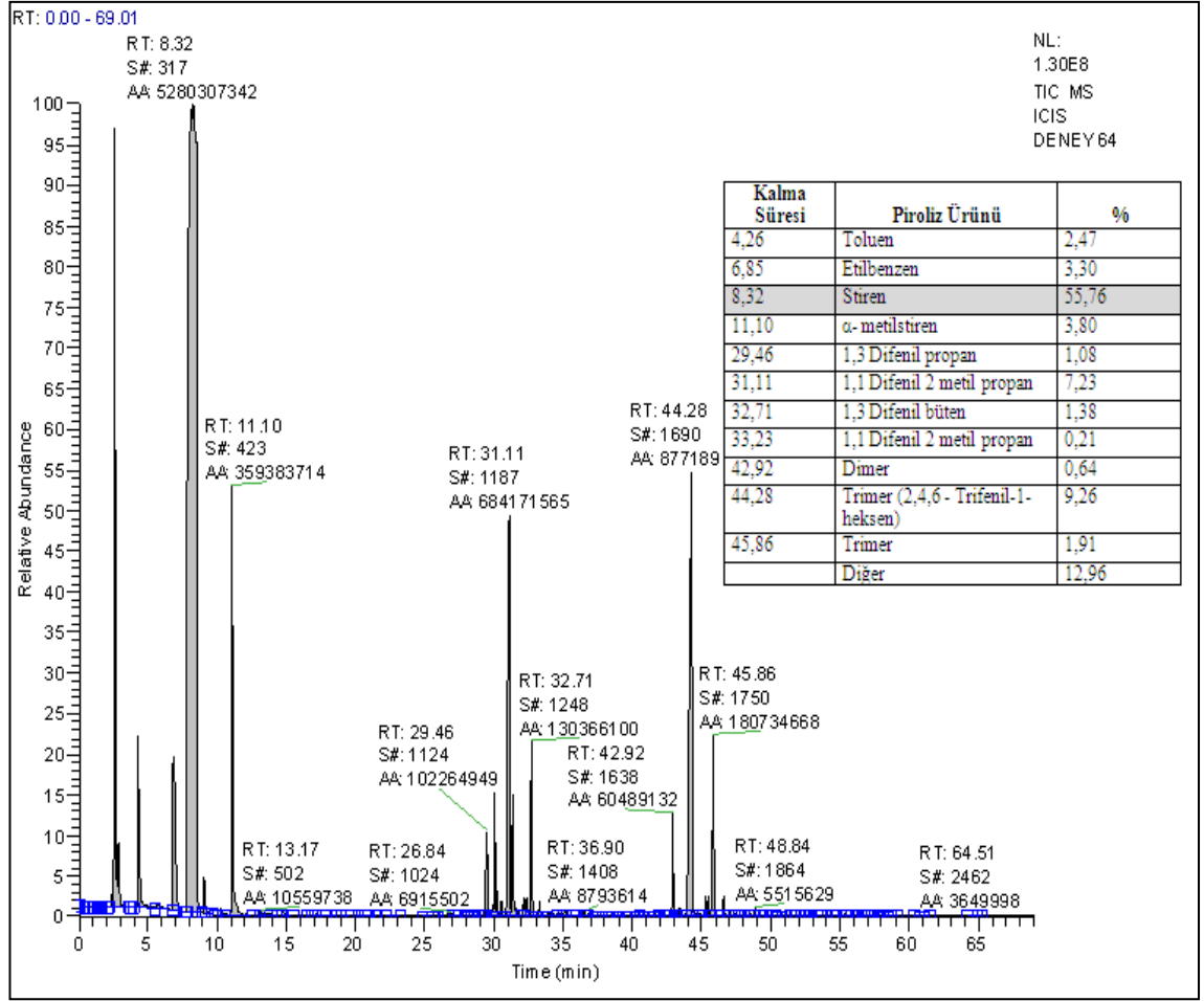
Şekil 4.21 550 °C sıcaklık ve % 5 FCC katalizörü ile gerçekleştirilen deney için sıvı ürünlerin GS/MS kromatogramı
