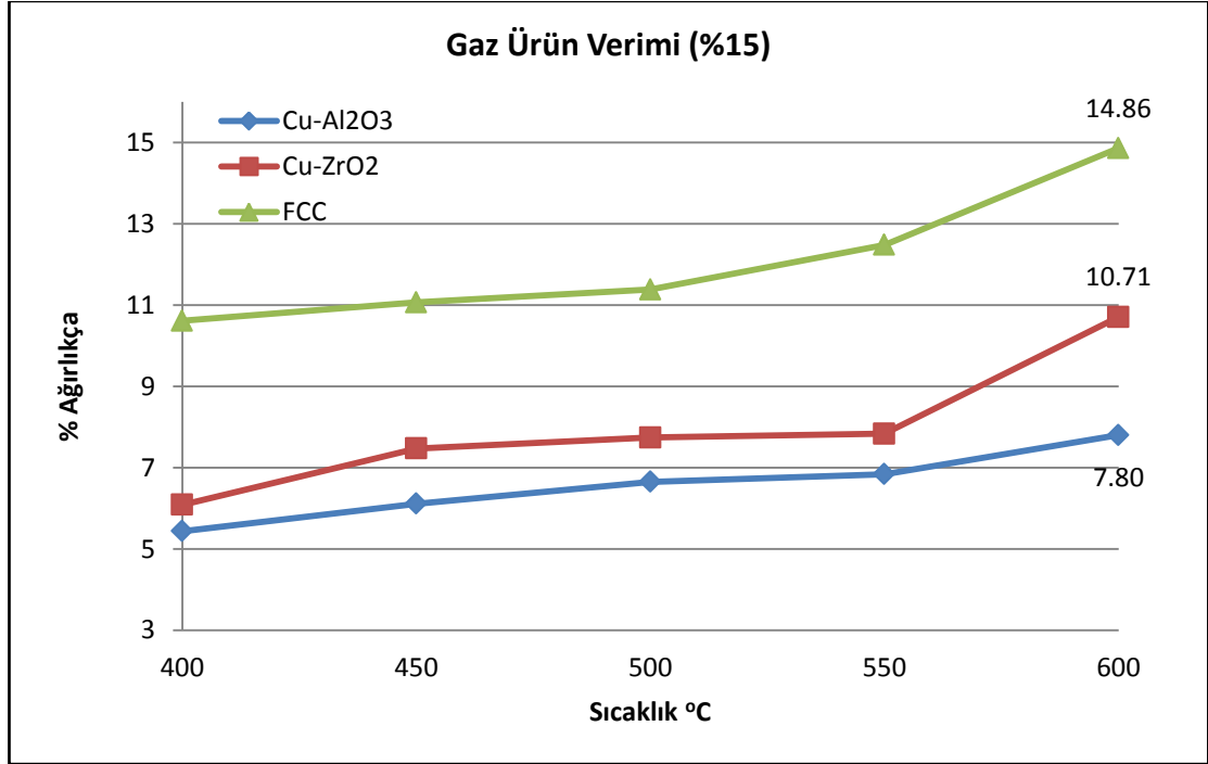
Şekil 4.7 % 15 Katalizör/PS oranında gaz ürün veriminin karşılaştırılması
