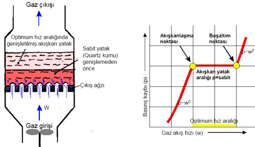
Şekil 2.5 Akışkan yataklı reaktörün çalışma prensibi
