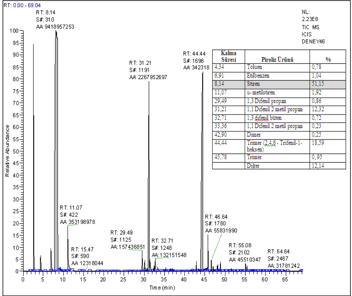
Şekil 4.18 500 °C sıcaklık ve % 10 Cu-ZrO 2 katalizörü ile gerçekleştirilen deneyin sıvı ürünlerin GC-MS kromatogramları
