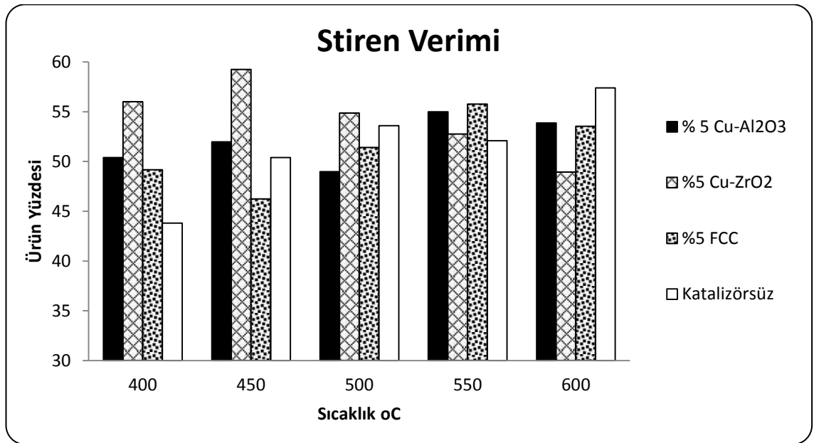
Şekil 4.28 Stiren veriminin %5 katalizör/PS oranı için sıcaklık ile değişimi
