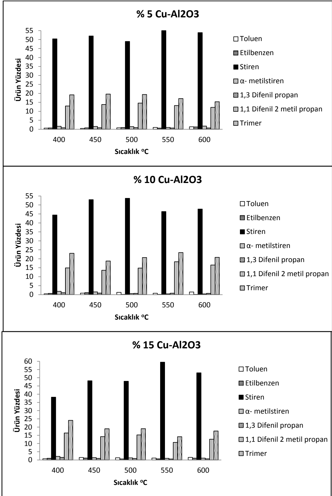
Şekil 4.25 Cu-Al 2 O 3 katalizörü ile elde edilen sıvı ürün bileşiminin sıcaklıkla değişimi
