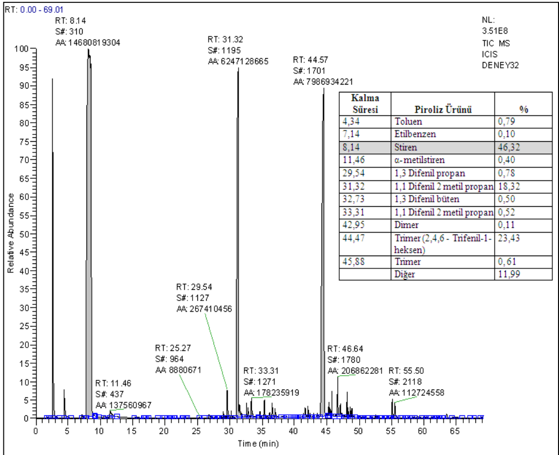
Şekil 4.14 550 °C sıcaklık ve % 10 Cu-Al 2 O 3 katalizörü ile gerçekleştirilen deney için sıvı ürünlerin GS/MS kromatogramı
