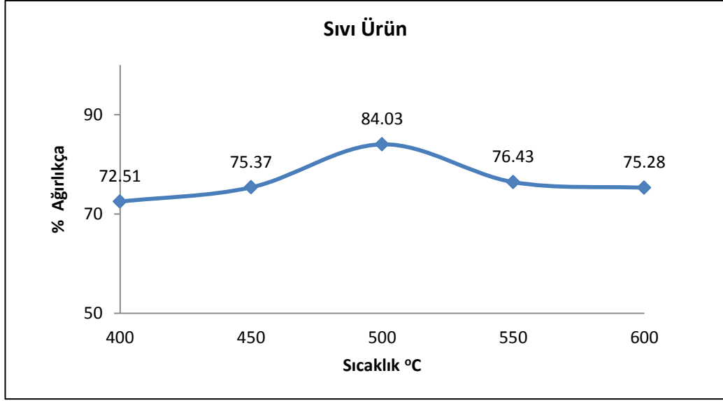
Şekil 4.4 PS'in katalizörsüz olarak ısıtılmasında sıvı ürün veriminin sıcaklık ile değişimi
