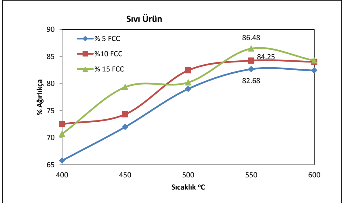
Şekil 4.3 PS'in FCC katalizörü ile ısı pirolizinde sıvı ürün veriminin sıcaklık ile değişimi
