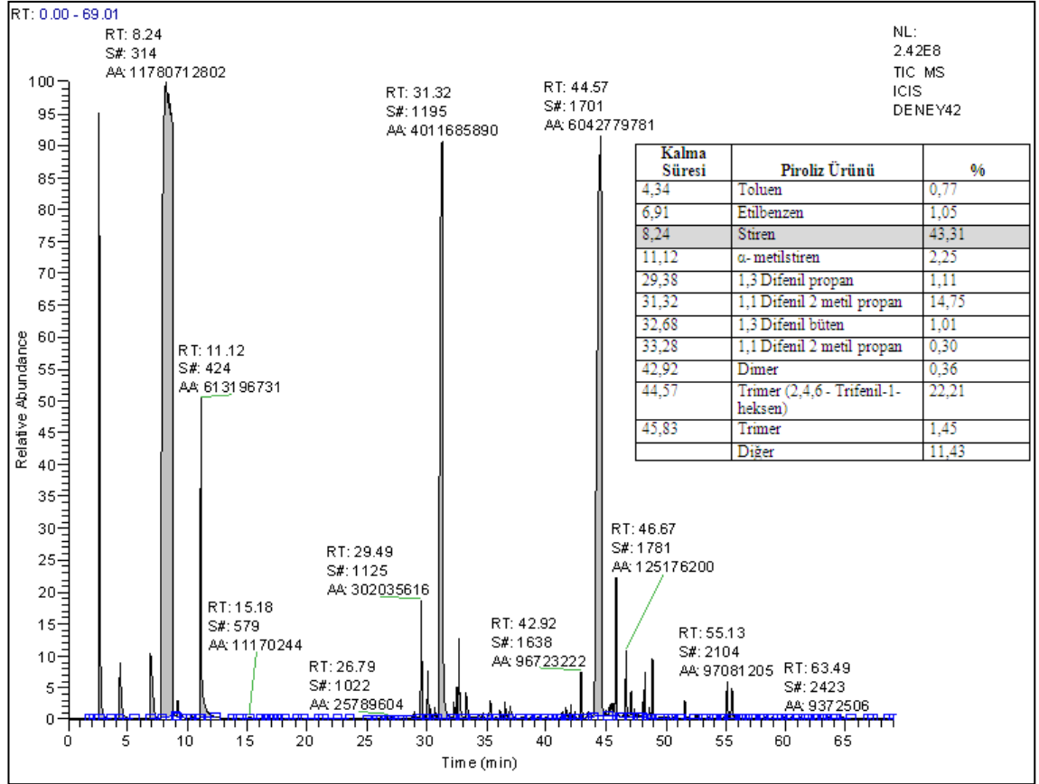
Şekil 4.17 550 °C sıcaklık ve % 5 Cu-ZrO 2 katalizörü ile gerçekleştirilen deney için sıvı ürünlerin GS/MS kromatogramı
