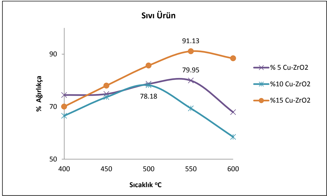
Şekil 4.2 PS'in \text{Cu-ZrO}_2 katalizörü ile ısıl pirolizinde sıvı ürün veriminin sıcaklık ile değişimi
