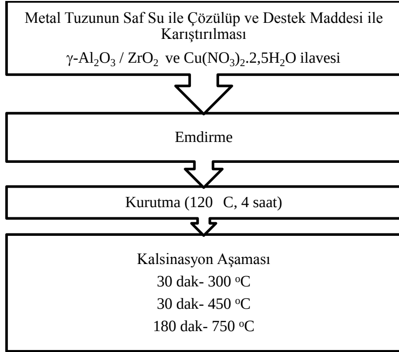
Şekil 3.1 Katalizör hazırlama aşamaları
