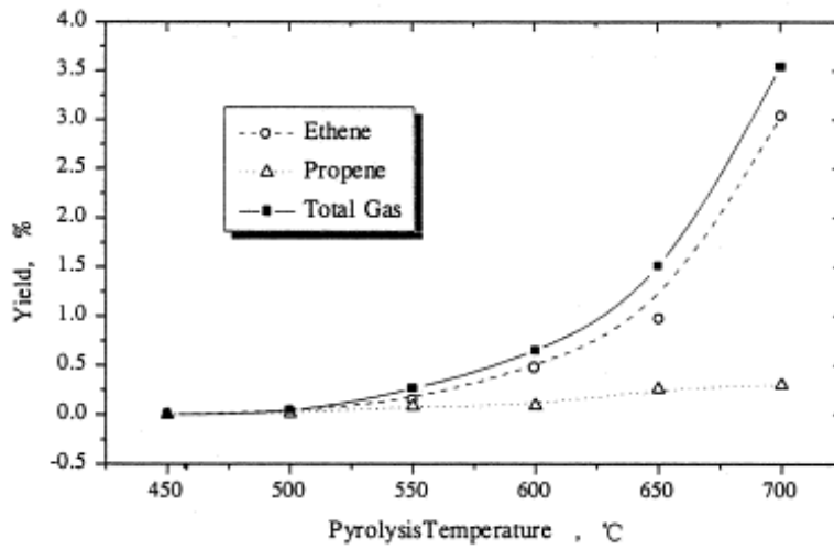
Şekil 2.6 Gaz ürün veriminin piroliz sıcaklığı ile değişimi (Liu vd. 2000)
