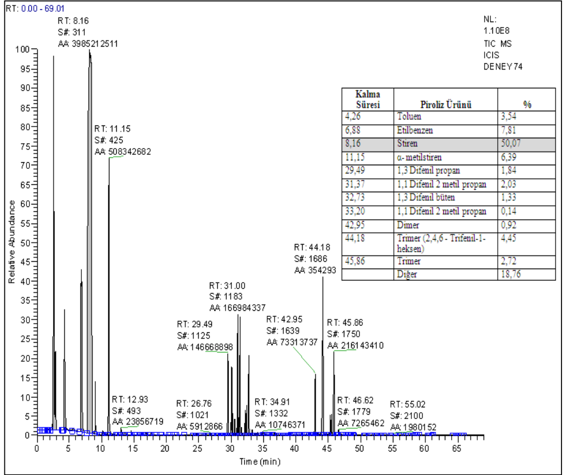
Şekil 4.23 550 °C sıcaklık ve % 15 FCC katalizörü ile gerçekleştirilen deney için sıvı ürünlerin GS/MS kromatogramı
