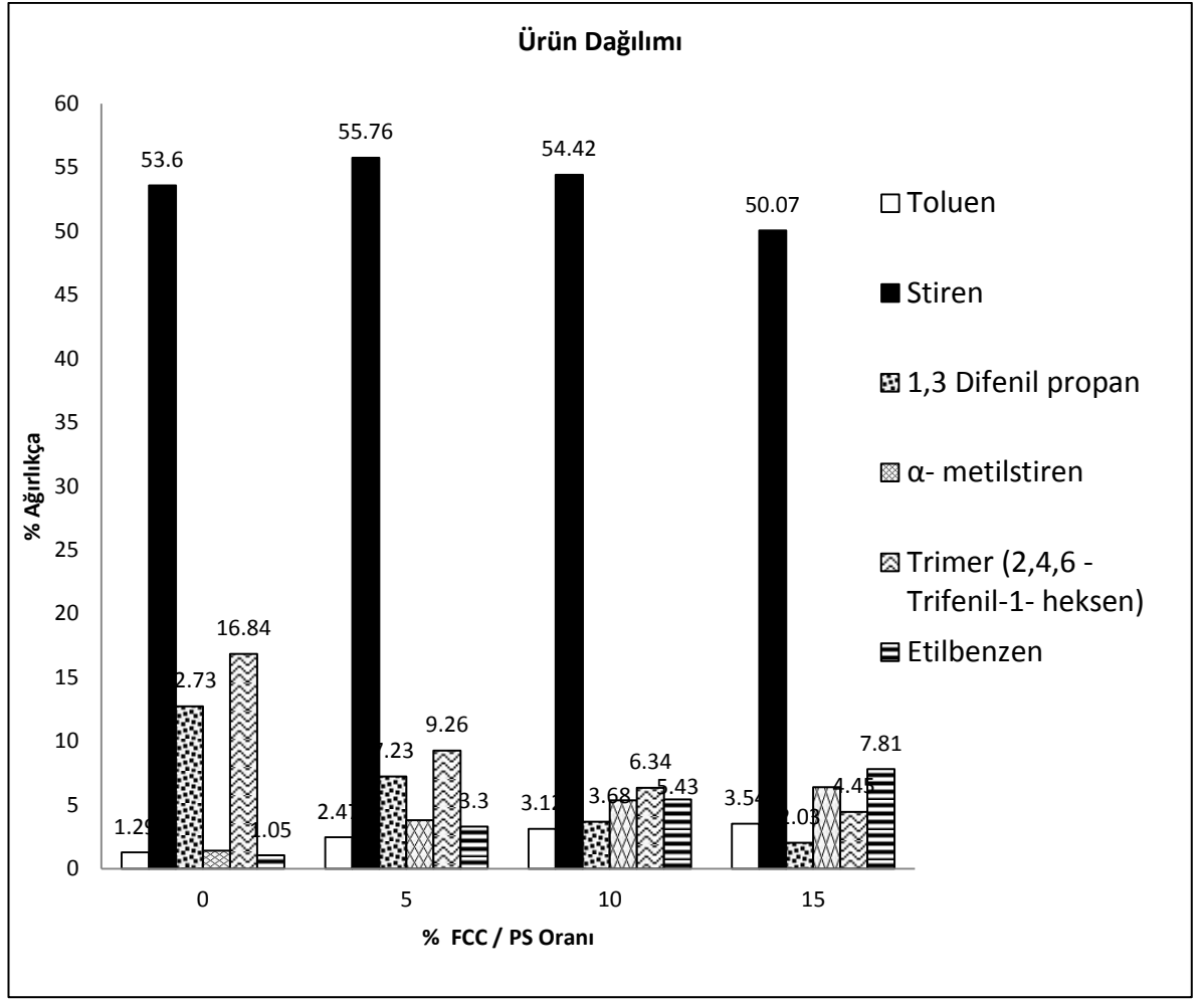
Şekil 4.20 FCC katalizörü için sıvı ürün dağılımı
