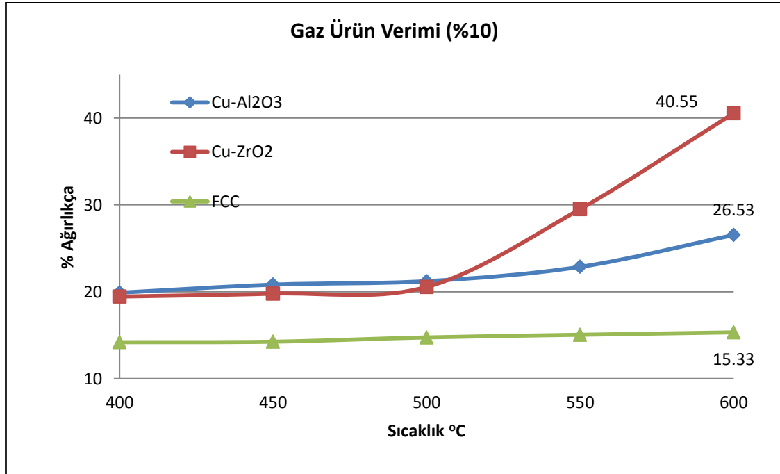
Şekil 4.6 % 10 Katalizör/PS oranında gaz ürün veriminin karşılaştırılması
