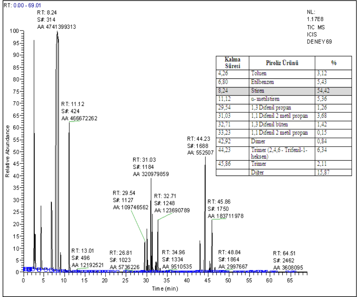
Şekil 4.22 550 °C sıcaklık ve % 10 FCC katalizörü ile gerçekleştirilen deney için sıvı ürünlerin GS/MS kromatogramı
