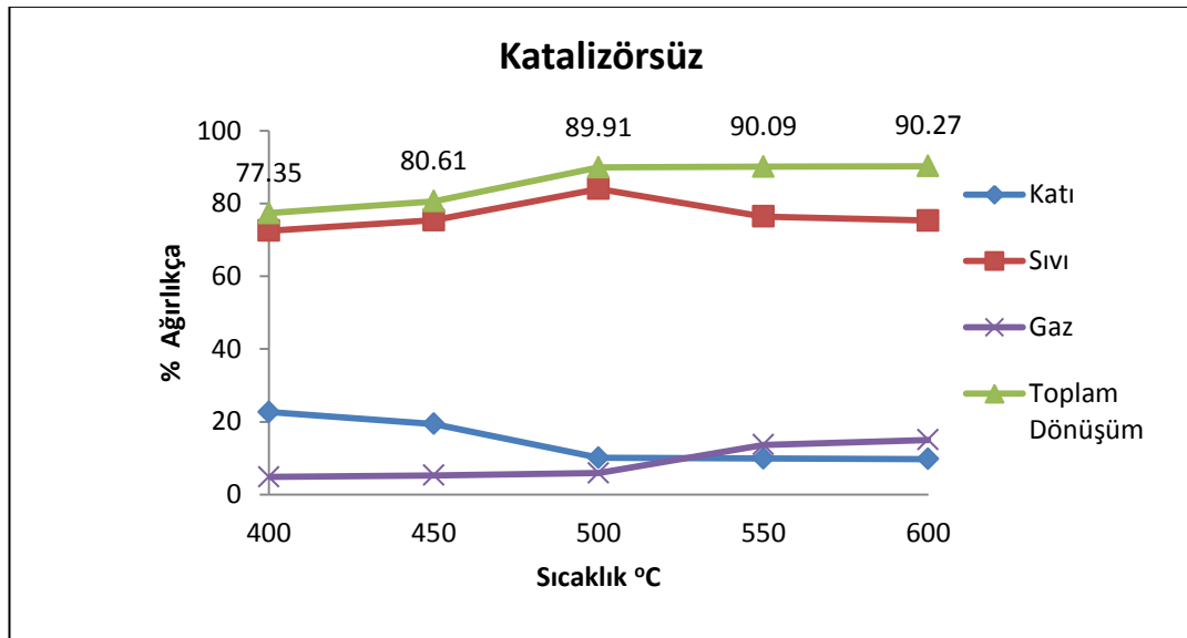
Şekil 4.11 Katalizörsüz ortamda sıvı, gaz, katı kalıntı ve toplam dönüşümün sıcaklıkla değişimi
