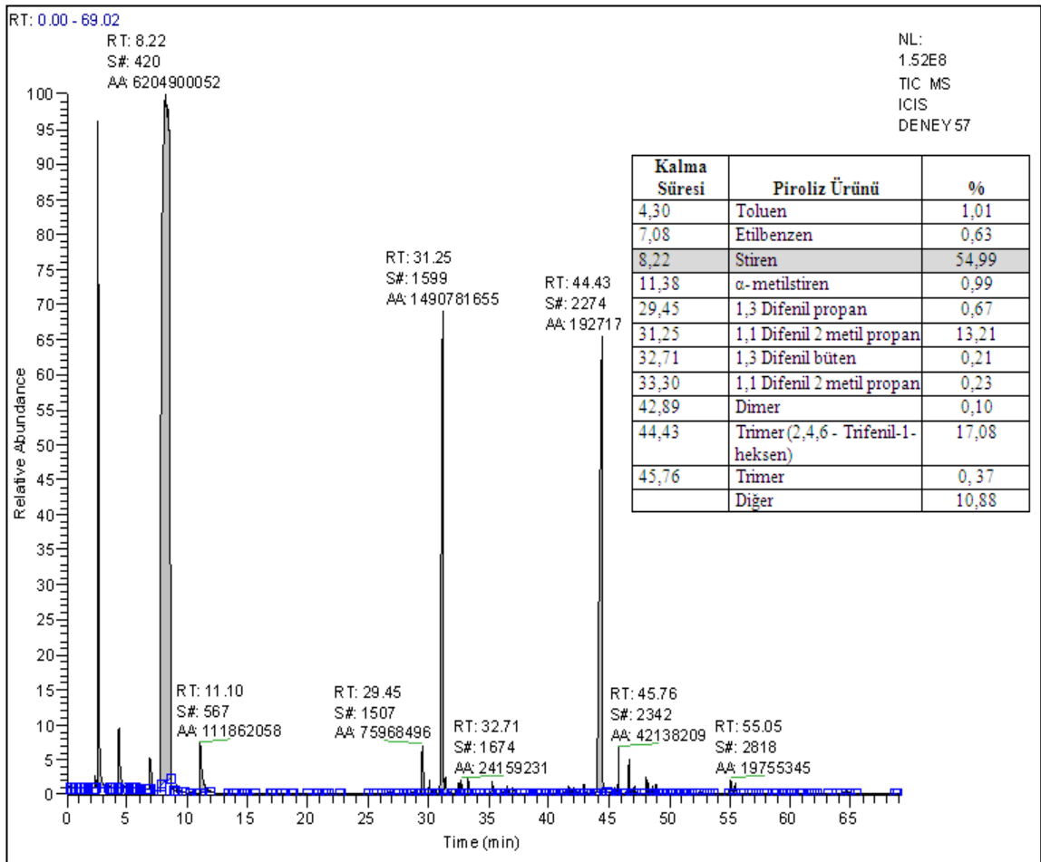
Şekil 4.13 550 °C sıcaklık ve % 5 Cu-Al 2 O 3 katalizörü ile gerçekleştirilen deney için sıvı ürünlerin GS/MS kromatogramı
