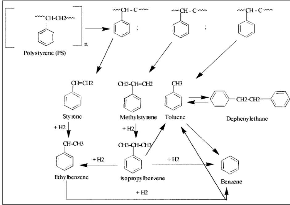
Şekil 2.7 PS'in pirolizinden elde edilen sıvı ürünlerin oluşum aşamaları (Karaduman 2002)
