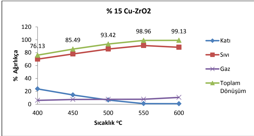
Şekil 4.9 Cu-ZrO 2 katalizörü varlığında katı-sıvı ve gaz ürünlerin sıcaklıkla değişimi
