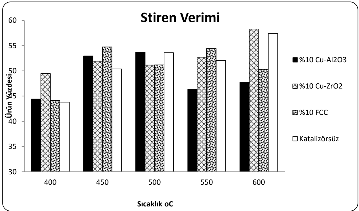
Şekil 4.29 Stiren veriminin %10 katalizör/PS oranı için sıcaklık ile değişimi
