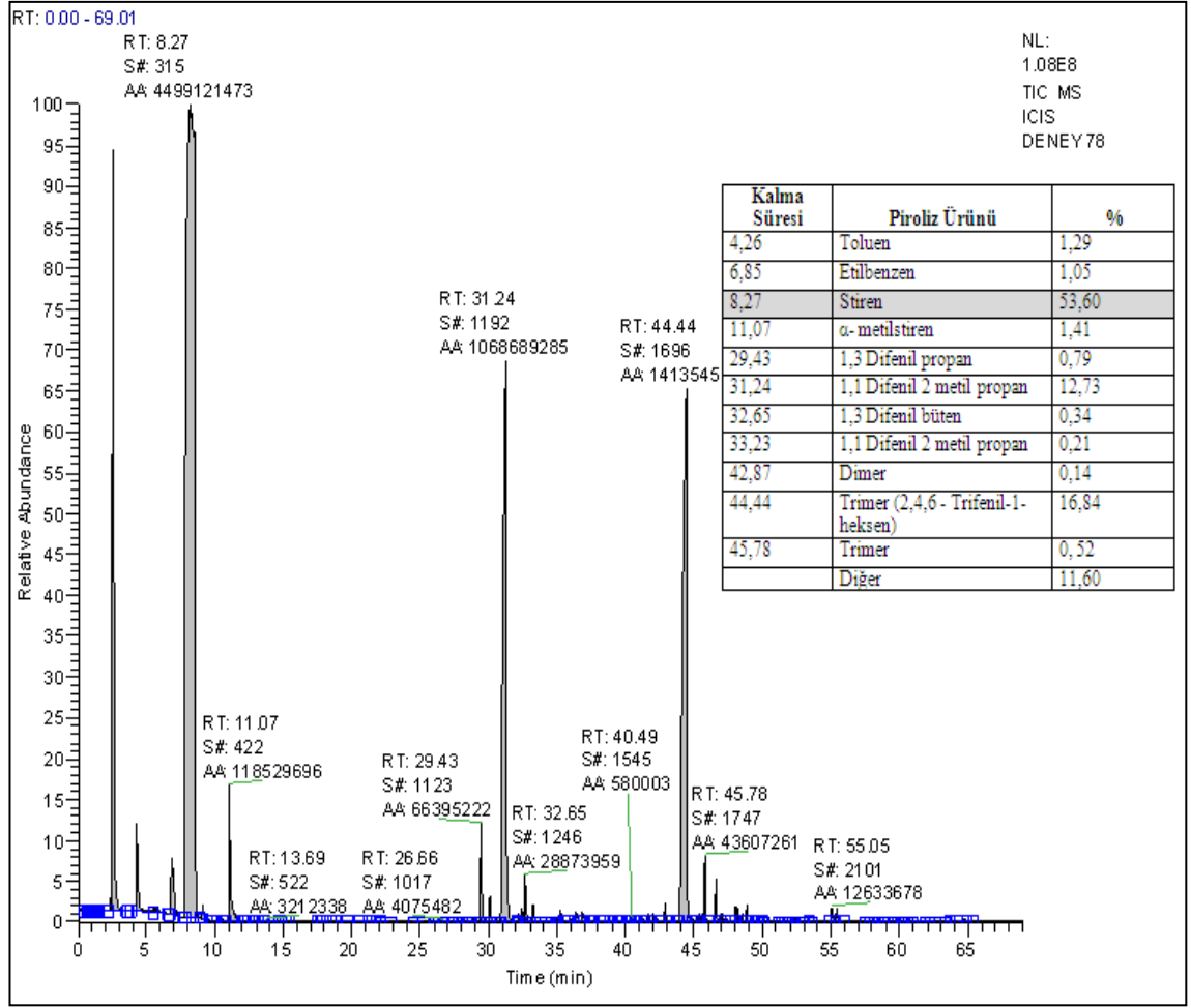
Şekil 4.24 500 °C sıcaklıkta katalizörsüz gerçekleştirilen deneyin sıvı ürünlerin GC-MS kromatogramları
