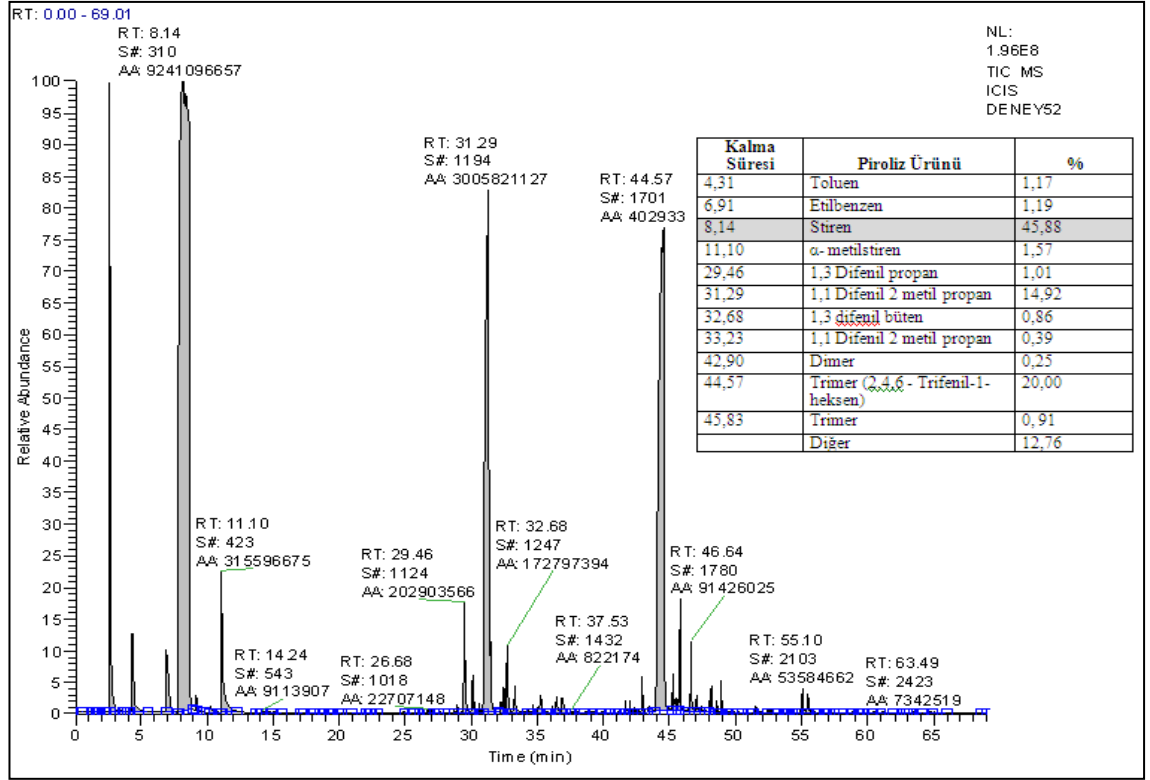
Şekil 4.19 550 °C sıcaklık ve % 15 Cu-ZrO 2 katalizörü ile gerçekleştirilen deney için sıvı ürünlerin GS/MS kromatogramı
