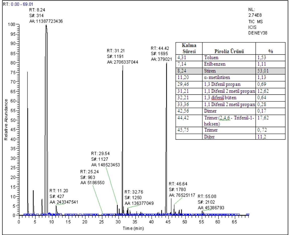
Şekil 4.15 550 °C sıcaklık ve % 15 Cu-Al 2 O 3 katalizörü ile gerçekleştirilen deney için sıvı ürünlerin GS/MS kromatogramı
