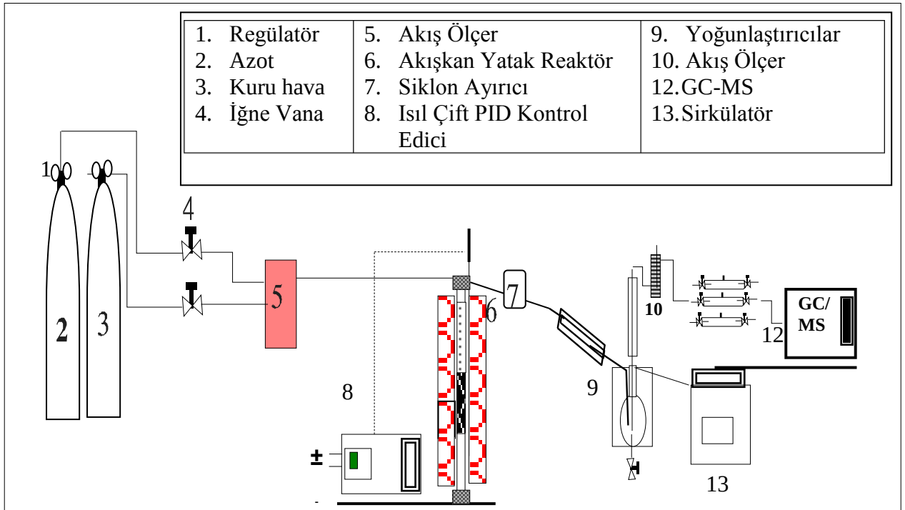
Şekil 3.3 Akışkan yataklı deney sistemi
