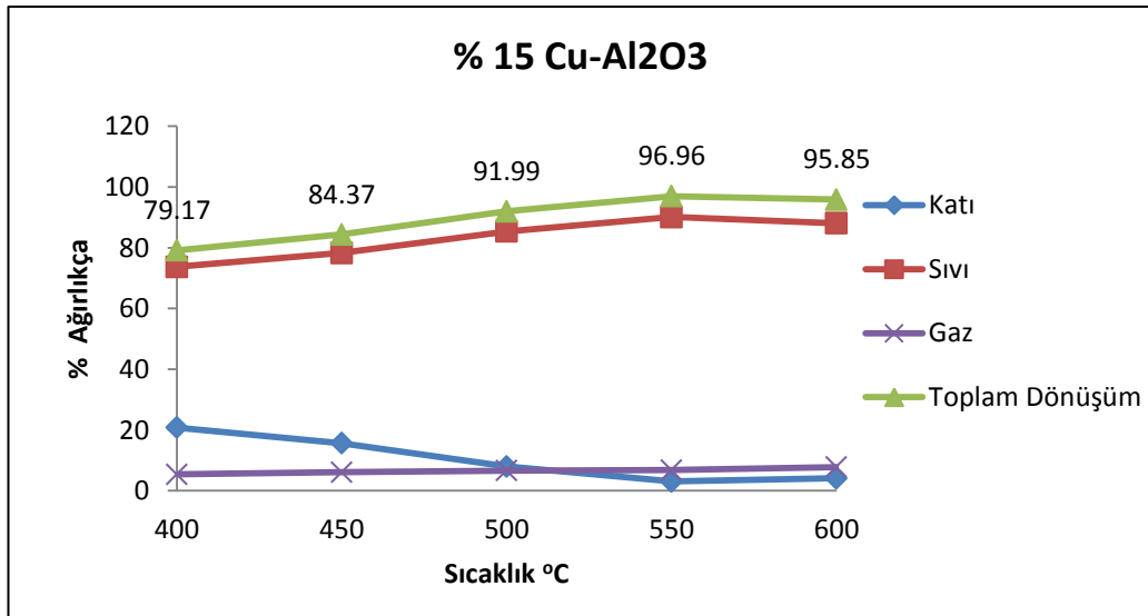
Şekil 4.8 Cu-Al 2 O 3 katalizörü varlığında katı-sıvı ve gaz ürünlerin sıcaklıkla değişimi
