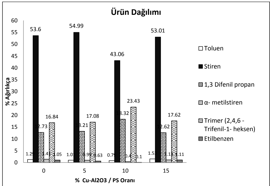
Şekil 4.12 Cu-Al 2 O 3 katalizörü için 550 °C sıcaklıkta sıvı ürün dağılımının katalizör/PS oranı ile değişimi
