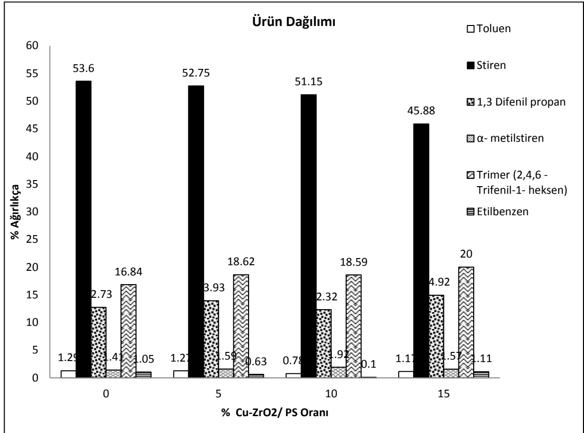
Şekil 4.16 Cu-ZrO 2 katalizörü için sıvı ürün dağılımı
