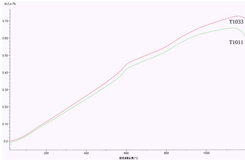
Şekil 6.56. T1011 ve T1033 kodlu numuneler için dilatometre eğrisi
