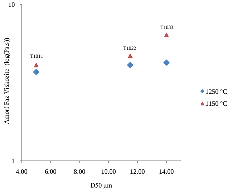
Şekil 6.33. Porselen bünne çamur D50 değerinin amorf faz viskozitesine olan etkisi
