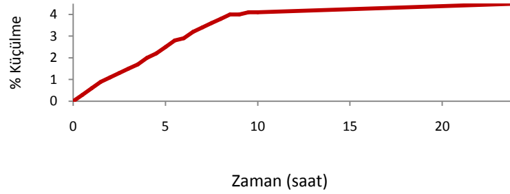
Şekil 6.10. Kaolen-2 için küçülme hız grafiği
