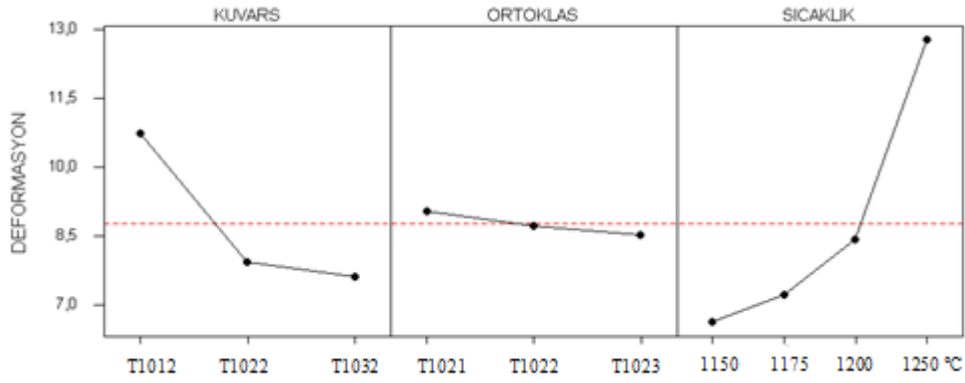
Şekil 6.51. Kuvars, ortoklas ve sıcaklık için deformasyon değişimi temel etki grafiği
