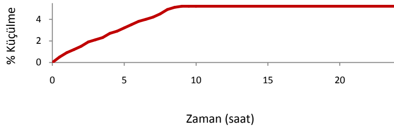
Şekil 6.9. Halloysit için küçülme hız grafiği
