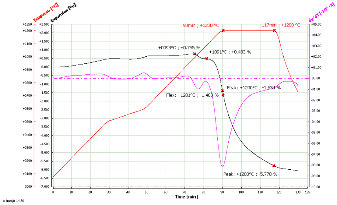
Şekil 6.24. T1033 kodlu numune için dilatometre eğrisi
