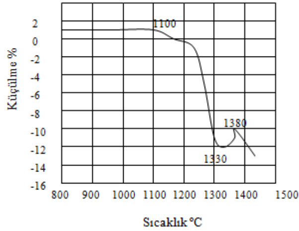
Şekil 3.8. Potasyum Feldispat için küçülme-genleşme eğrisi (Fortuna, 2000)
