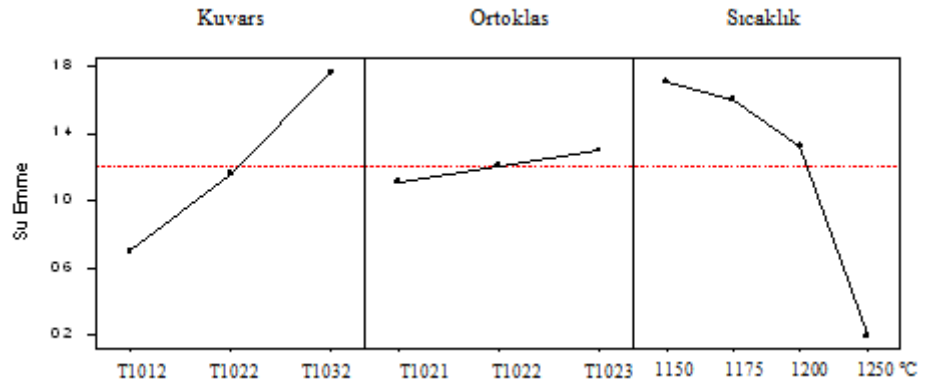
Şekil 6.41. Kuvars, ortoklas ve sıcaklık için su emme değişimi temel etki grafiği
