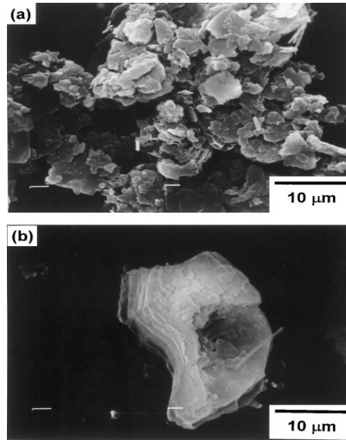
řekil 3.1. Kaolen partik÷llerinin morfolojisi (a)Tabakalı yapı, (b) Tabakaların birbirine yapıřarak aglomere olması (Chen ve ark., 2000)
