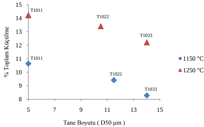
Şekil 6.45. Toplam küçülme değeri ve tane boyutu (D50) ilişkisi
