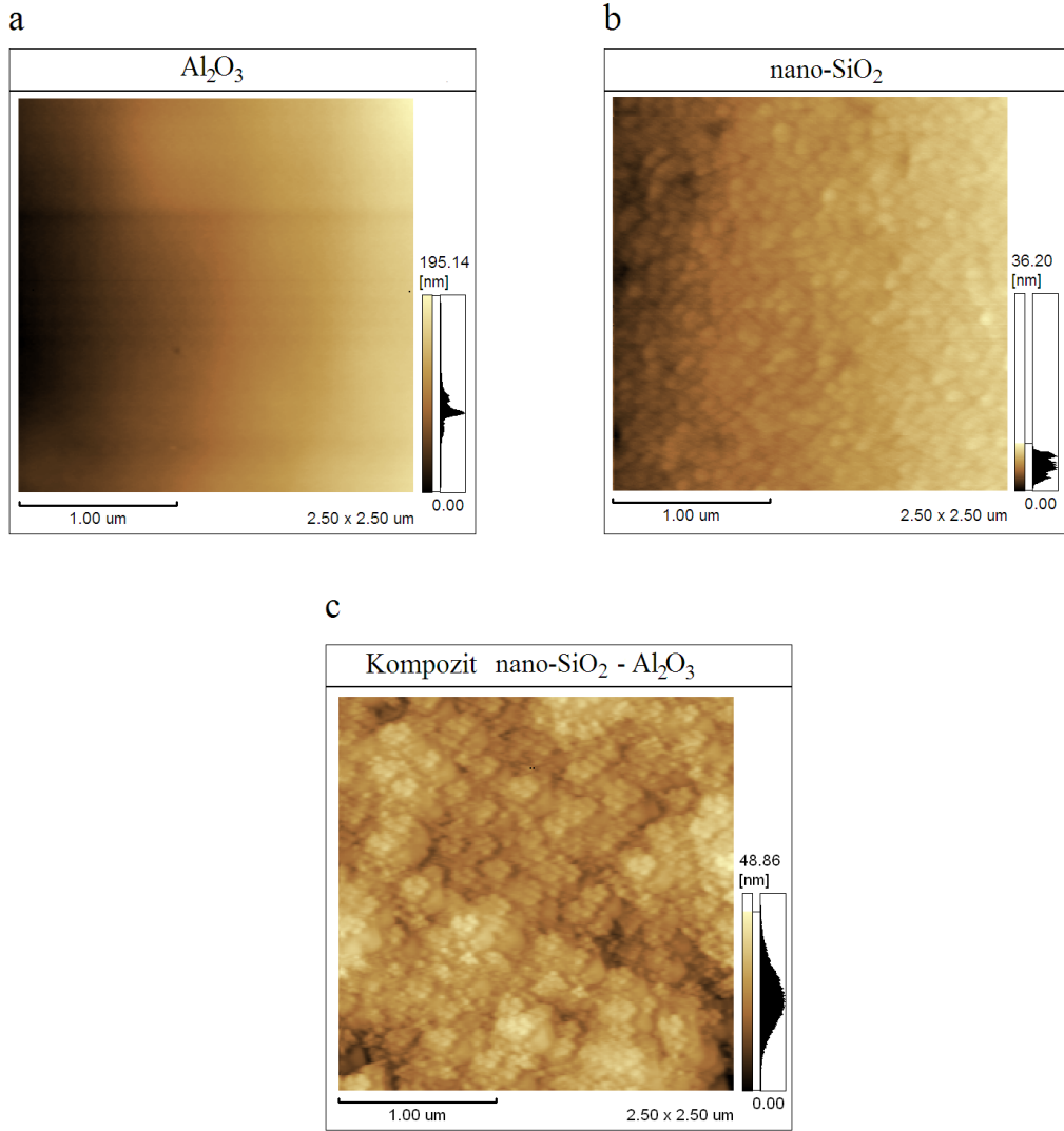
Şekil 5.38 : 450°C sıcaklıkta ısıtılmış ve ısıtılma tabii tutulmuş olan (a) \text{Al}_2\text{O}_3 film, (b) nano- \text{SiO}_2 film ( \text{NH}_3/\text{TEOS} oranı=1:32), (c) nano- \text{SiO}_2 - \text{Al}_2\text{O}_3 kompozit filmin ( \text{NH}_3/\text{TEOS} oranı=1:32) AFM ile çekilmiş yüzey görüntüleri.
