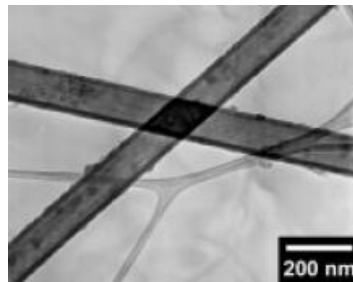
Şekil 4.9 : Silisyumdioksit nanotübün TEM görüntüsü.
