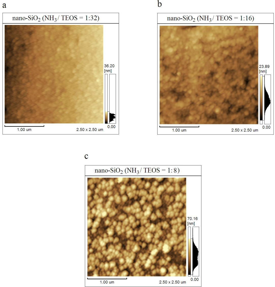
Şekil 5.1 : Farklı \text{NH}_3 /TEOS oranlarında hazırlanmış olan nano-SiO 2 sollerinin 450°C sıcaklıkta kurutulması ile oluşan ince filmlerin AFM resimleri.
