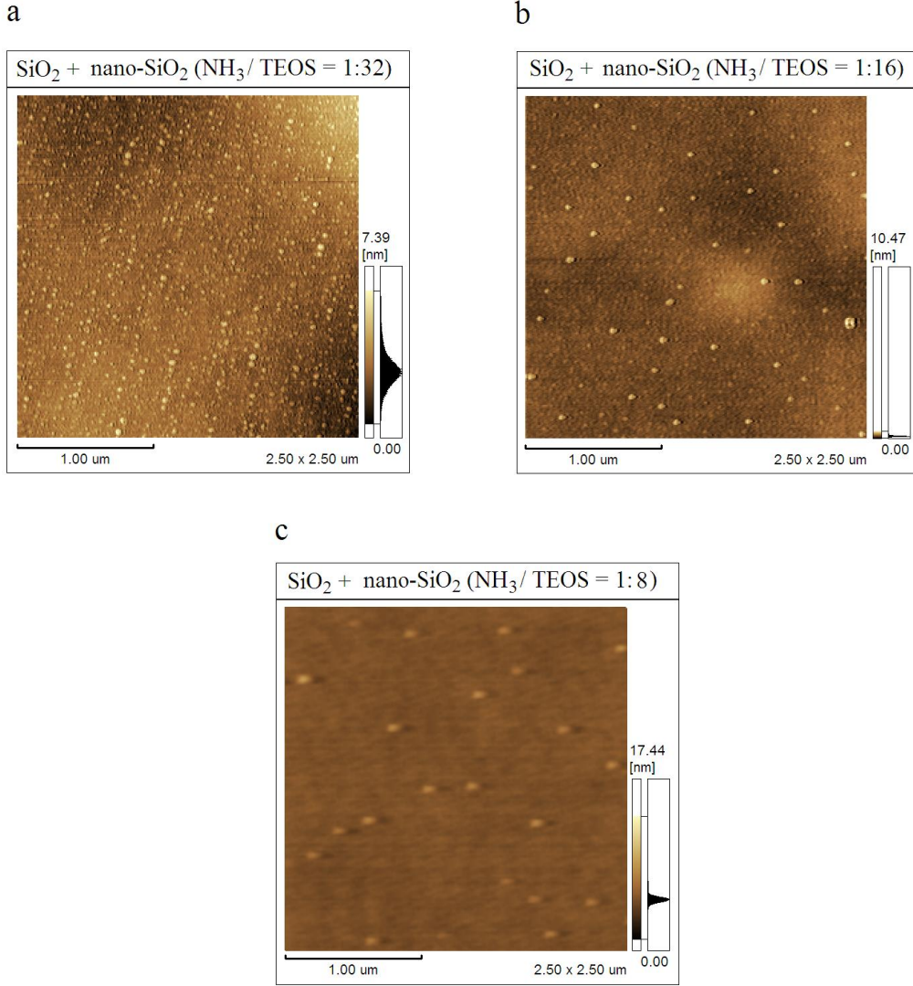
Şekil 5.16 : \text{SiO}_2 solünün içine farklı nano \text{SiO}_2 sollarının 1/10 oranında karıştırılması ile oluşan sollar kullanılarak hazırlanan 450^\circ\text{C} 'de ısıtılma tabi tutulan filmlerin AFM ile çekilmiş görüntüleri.
