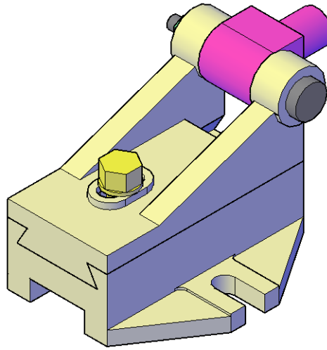
Şekil 4.8 Bağlantı kızağı üç boyutlu montaj modelinin görüntüsü.
