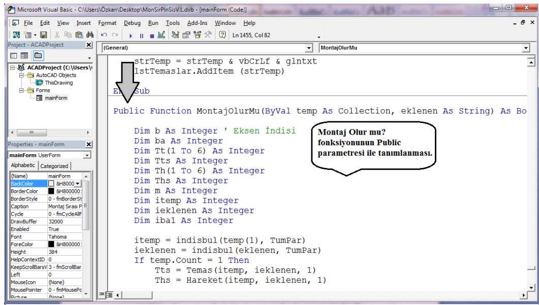
Şekil 3.5 Program içerisinde public parametresinin kullanımı.
