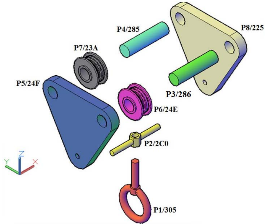
Şekil 4.2 Palanga yük aparatı üç boyutlu demontaj görüntüsü.
