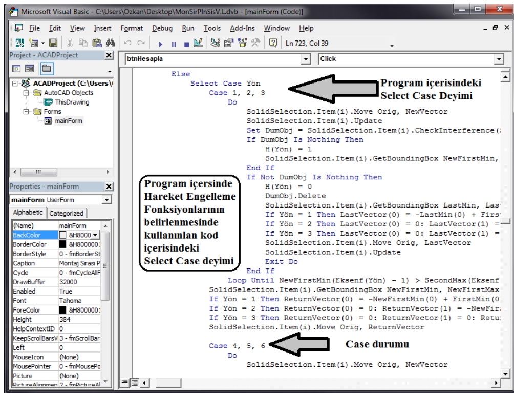
Şekil 3.13 Select case deyiminin program içerisinde kullanımı.
