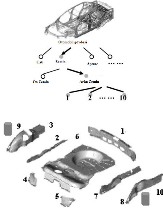
Şekil 1.7 Araba gövdesi montaj işlemi ve arka zeminin ana parçaları.
