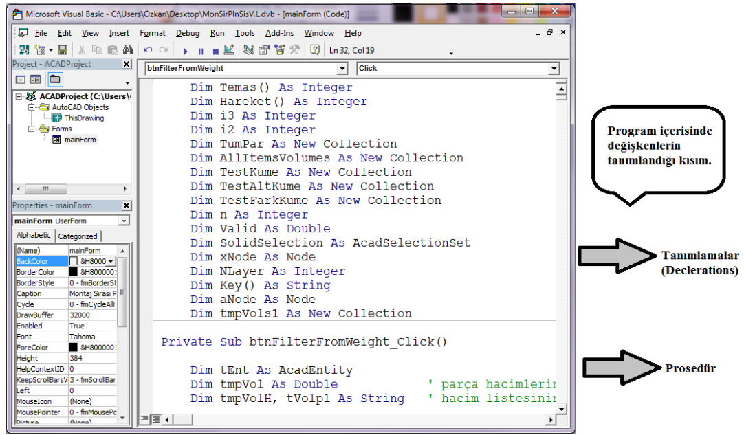
Şekil 3.2 Geliştirilen program içerisindeki tanımlamalar kısmı.
