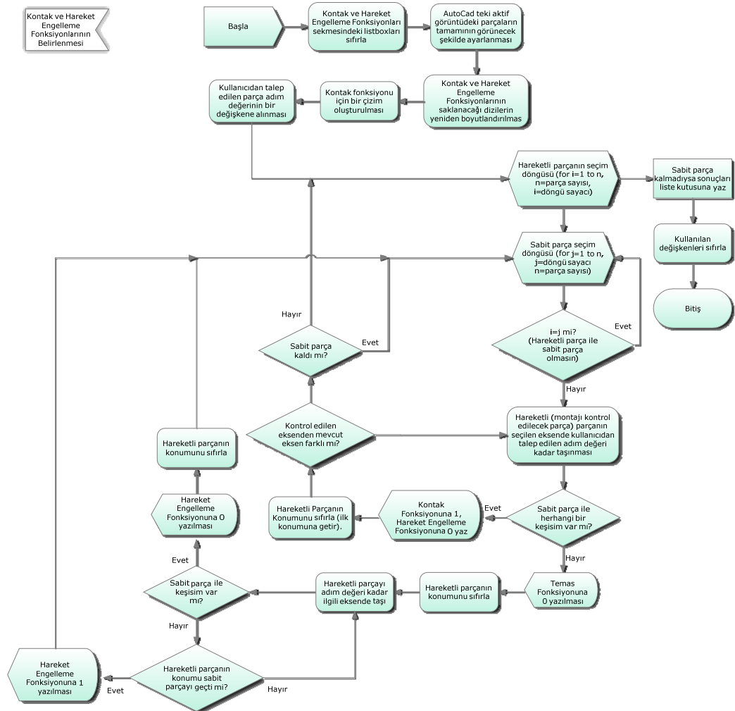
Şekil 3.27 K-H fonksiyonlarının oluşturulması için akış şeması [39].
