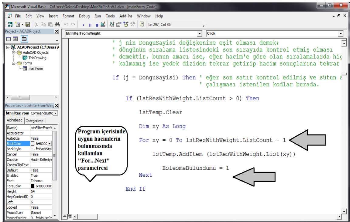
Şekil 3.15 For...Next döngüsünün program içerisinde kullanımı.
