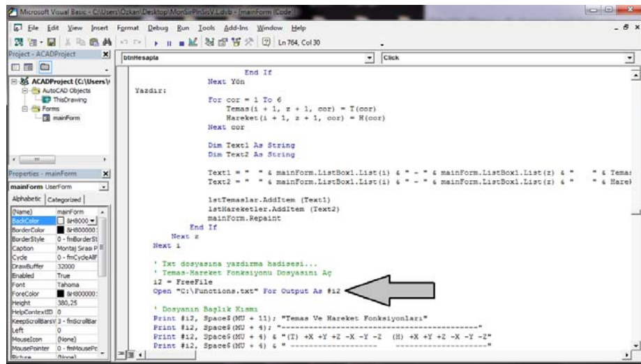
Şekil 3.21 Program içerisindeki open parametresinin kullanılması.
