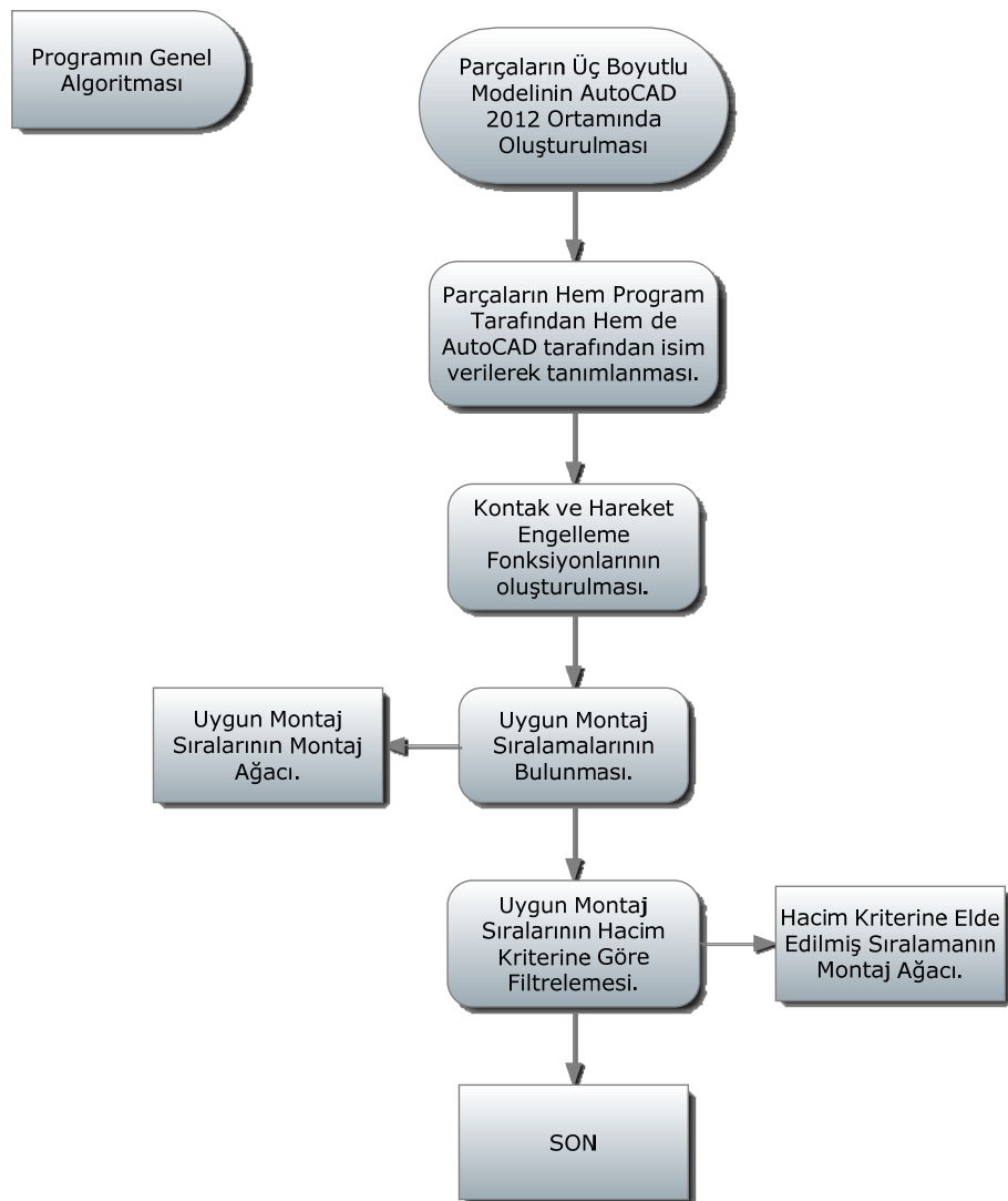
Şekil 3.32 Programın genel algoritması.
