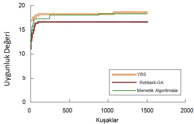
Şekil 1.11 YBS, rehberli-ga ve memetik algoritmaların karşılaştırılması.
