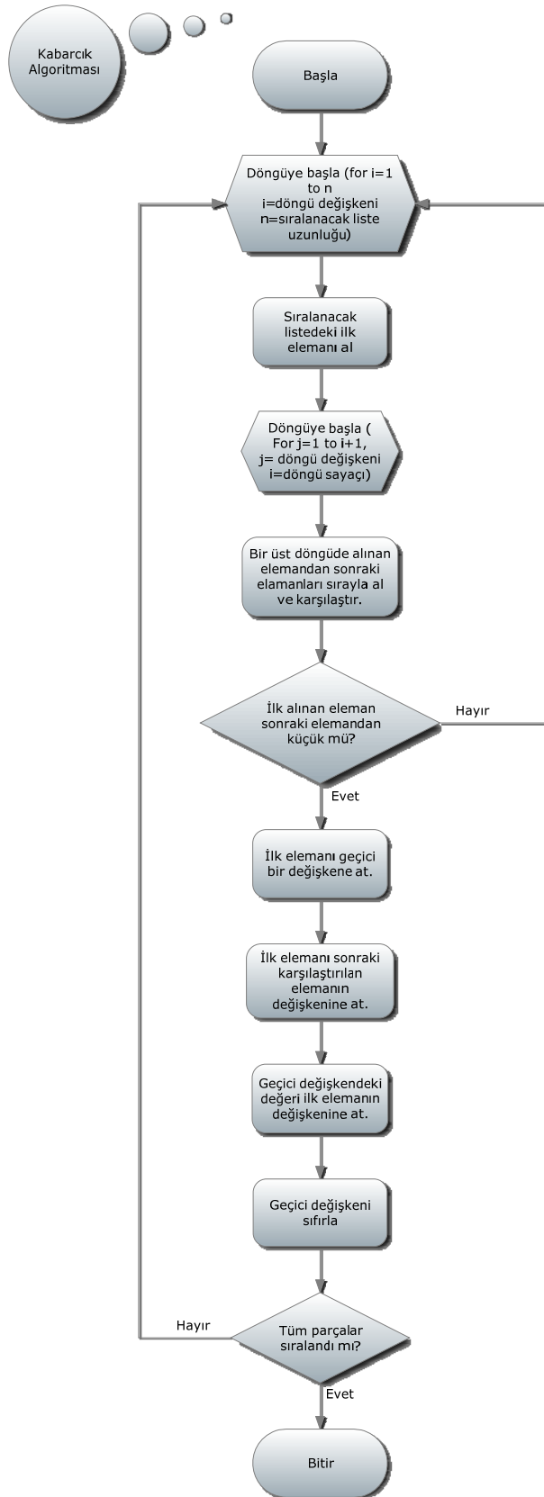
Şekil 3.29 Kabarcık algoritmasının şematik gösterimi.
