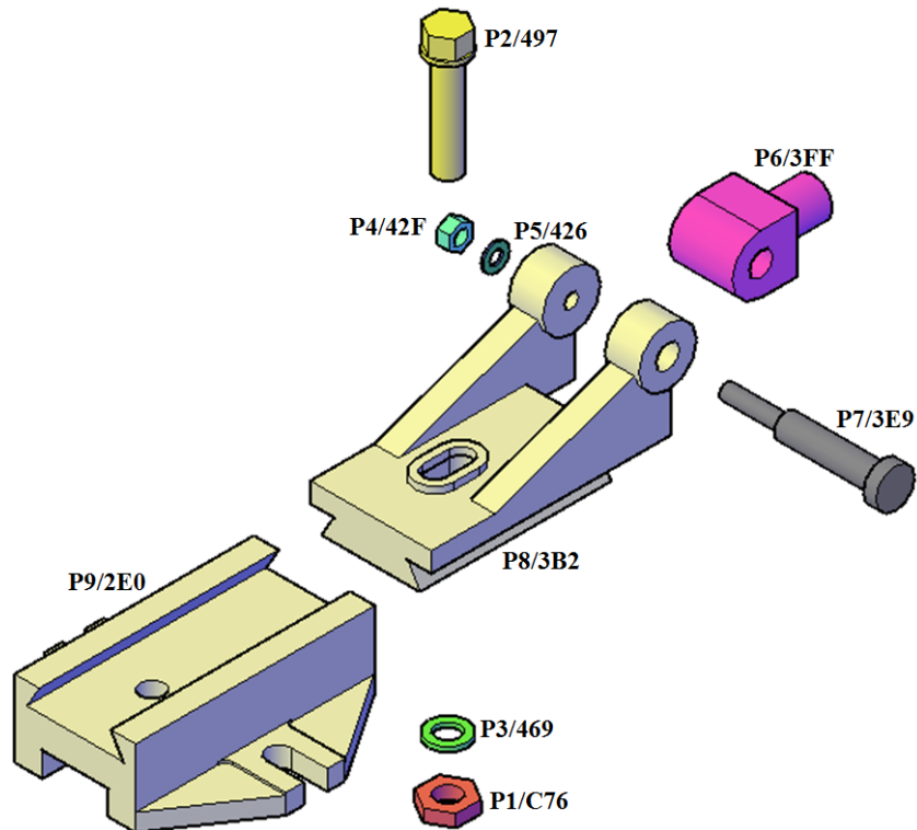
Şekil 4.9 Bağlantı kızağı üç boyutlu patlatılmış görüntüsü.
