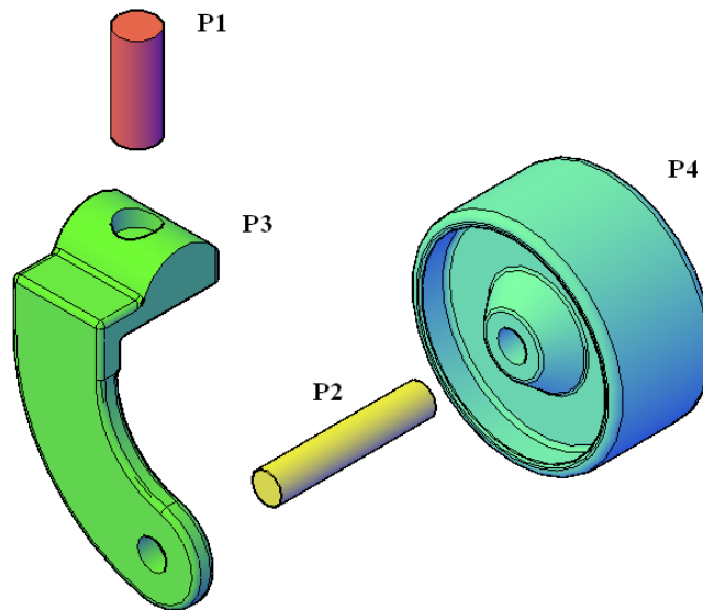
Şekil 3.38 Örnek montaj sisteminin demontaj hali.
