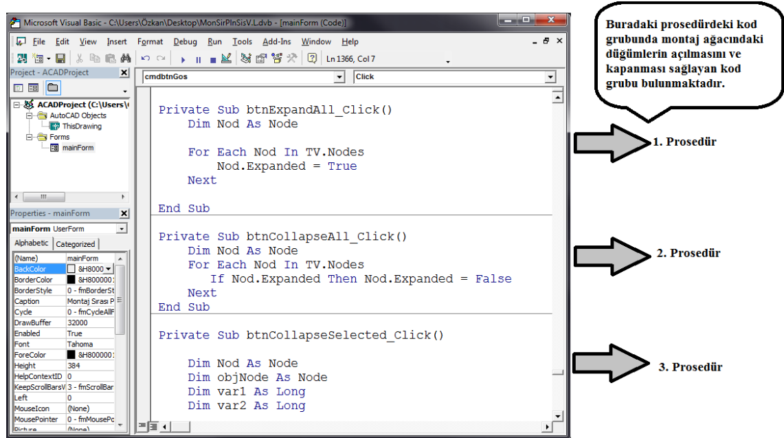
Şekil 3.1 Geliştirilen program içerisinde prosedür örnekleri.
