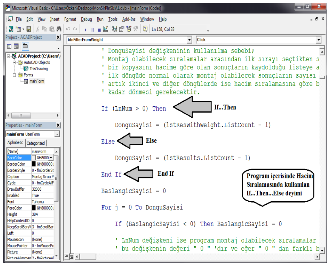
Şekil 3.14 If...Then...Else deyim grubunun program içerisinde kullanımı.
