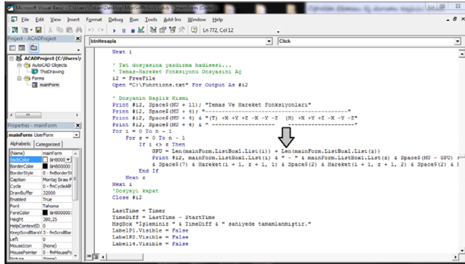
Şekil 3.20 Program içerisindeki len deyiminin kullanılması.
