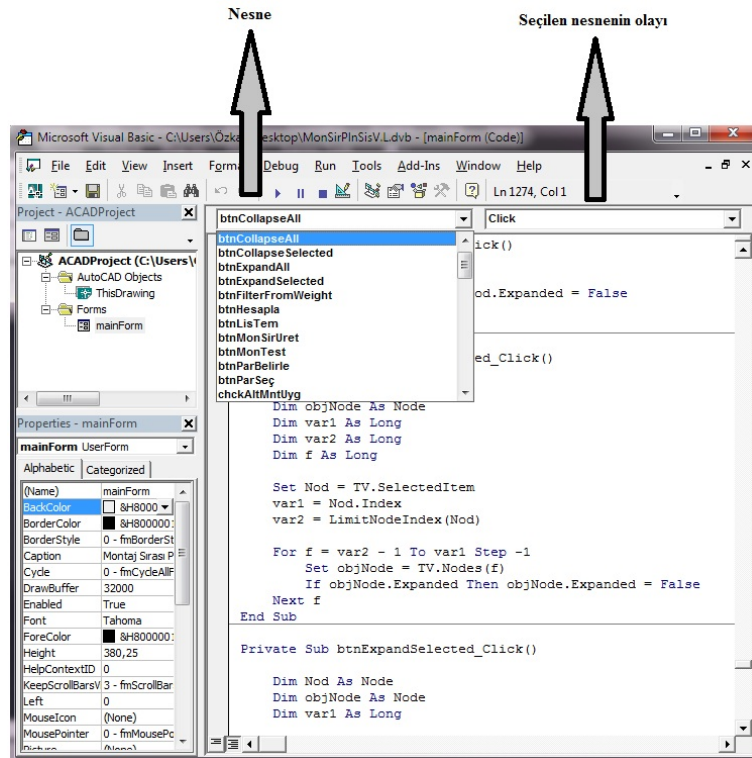
Şekil 3.3 VBA' da nesne ve olay kavramları.
