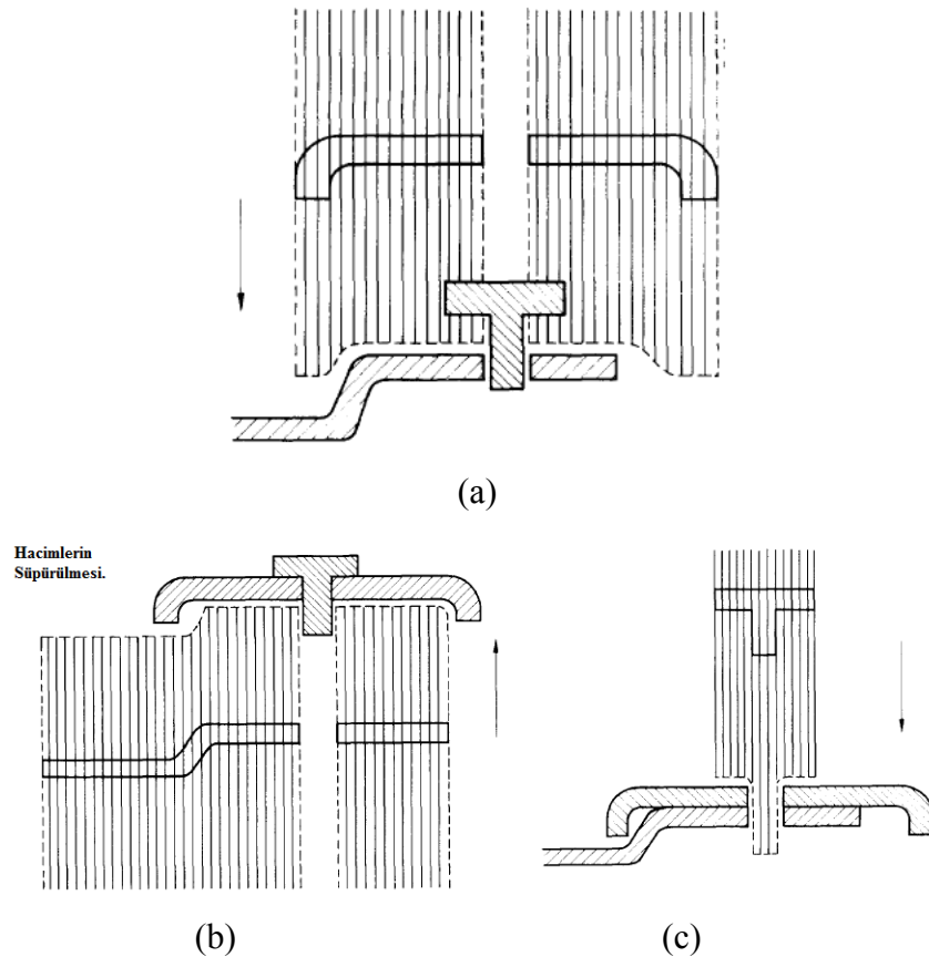
Şekil 1.3 Başlık, alt destek parçası, pin için çakışma kontrolleri a) Başlığın süpürülmesi, b) Alt destek parçasının süpürülmesi, c) Pin' in süpürülmesi.
