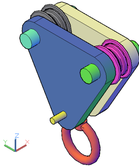
Şekil 4.1 Palanga yük aparatı üç boyutlu montaj modelinin görüntüsü.
