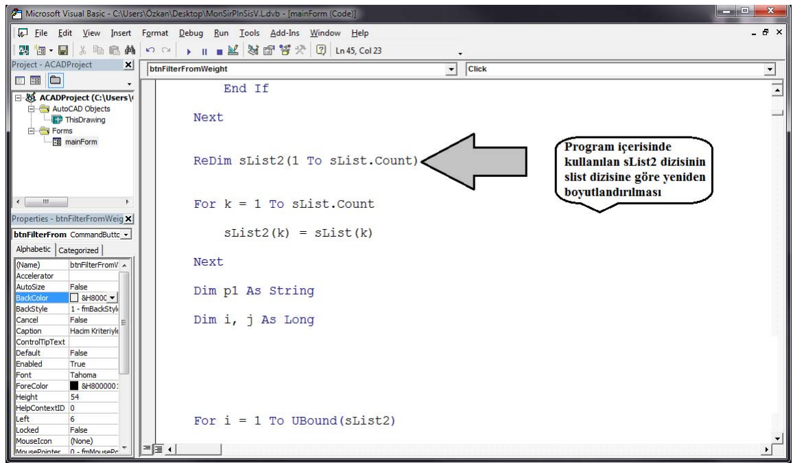
Şekil 3.17 Program içerisindeki dinamik dizi tanımlanması.
