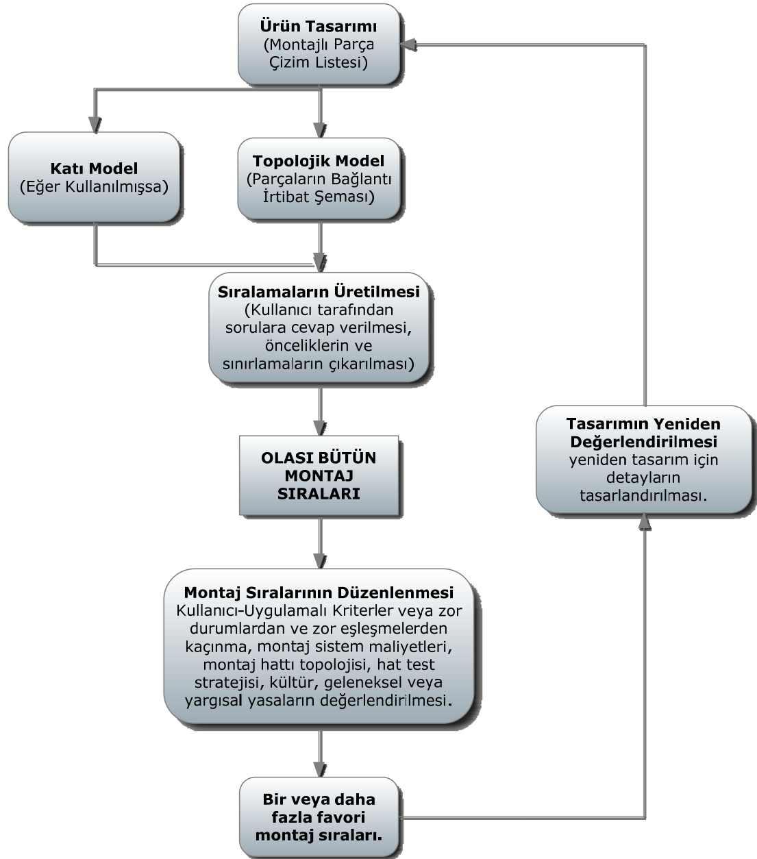
Şekil 1.1 Erken ürün tasarımında montaj sırası tasarımı ve değerlendirme rolleri [11].
