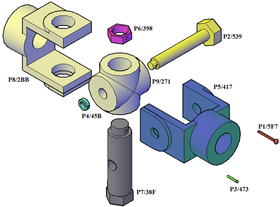
Şekil 4.16 Mafsal parçalarının üç boyutlu demontaj modeli görüntüsü.
