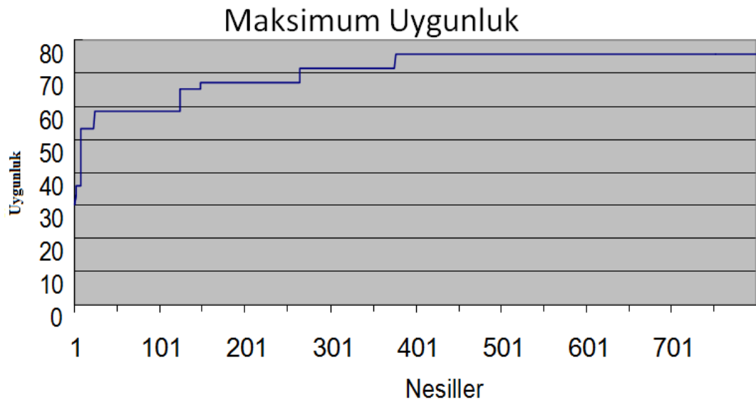
Şekil 1.12 İki boyutlu montajda genetik algoritma tabanlı hibrit modelin maksimum uygunluğa karşı popülasyon grafiği.
