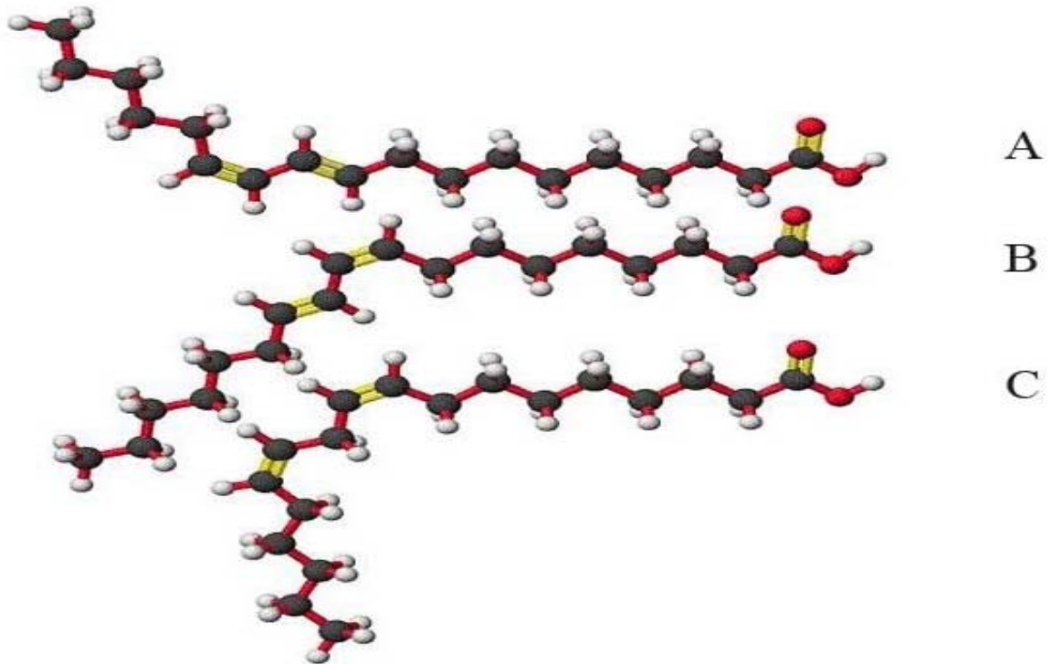
Şekil 2.1. Linoleik asitin bazı izomerleri
