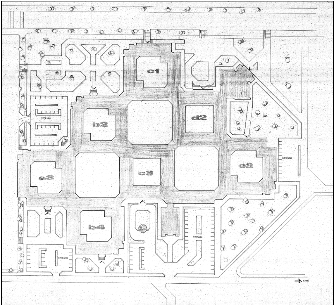
Şekil 6.37. Müh.-Mim. Fakültesi (Fen Fakültesi) vaziyet planı, 1993 (Arşiv, 2011)
