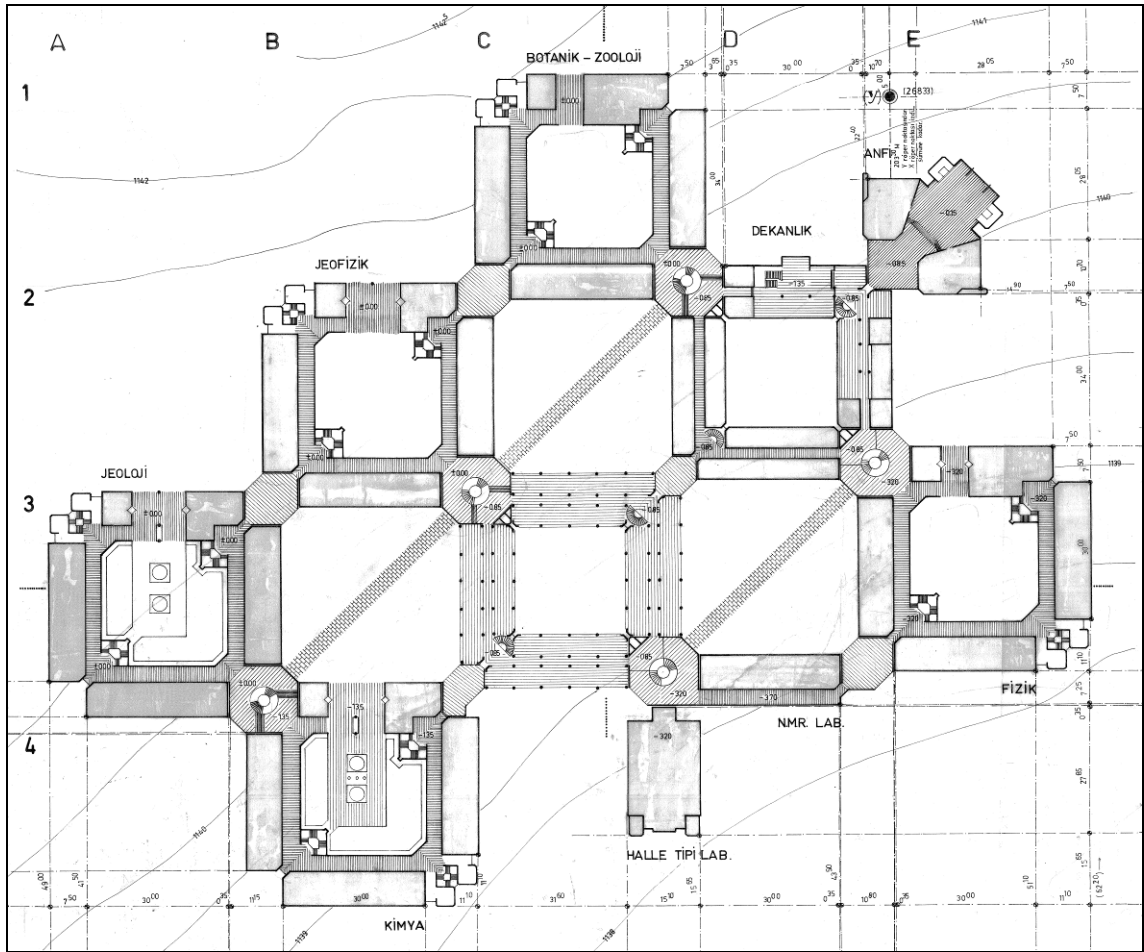
Şekil 6.36. Müh.-Mim. Fakültesi (Fen Fakültesi) yerleşim planı, 1981 (Arşiv, 2011)
