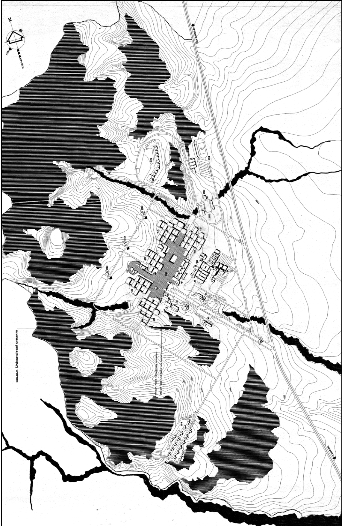
Şekil 6.2. S.Ü. Alaeddin Keykubat Kampüsü genel yerleşim planı, fikir projesi Aralık-1980 (Arşiv, 2011)
