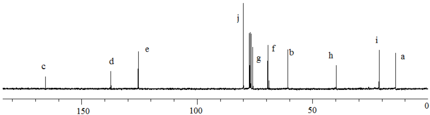
Figure A.8. 13 C-NMR spectra of monomer A5 .
