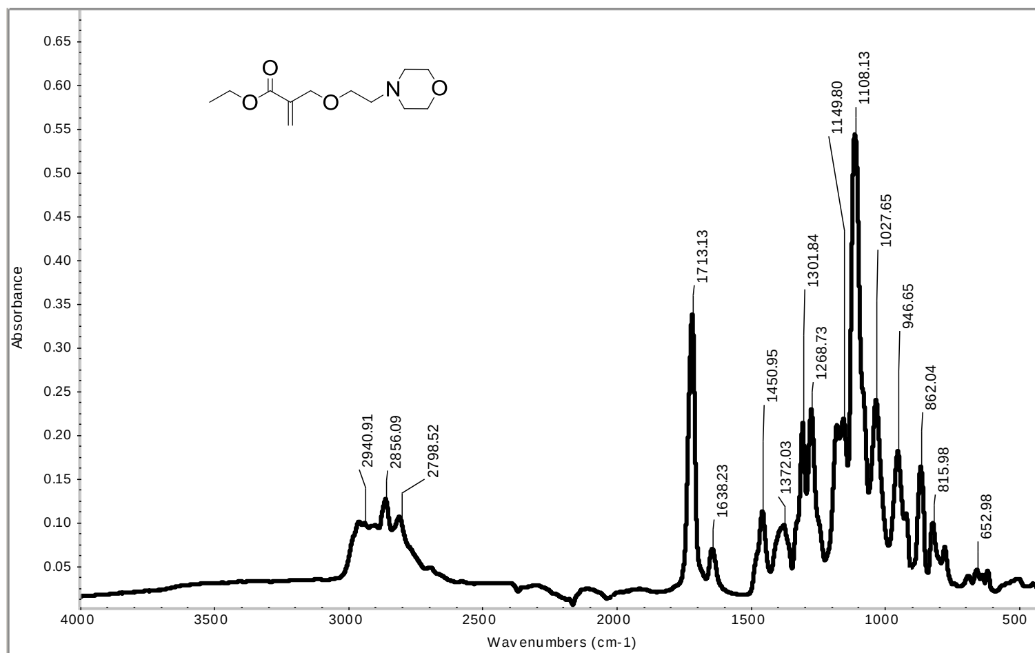
Figure A.23. FTIR spectra of monomer A1 .
