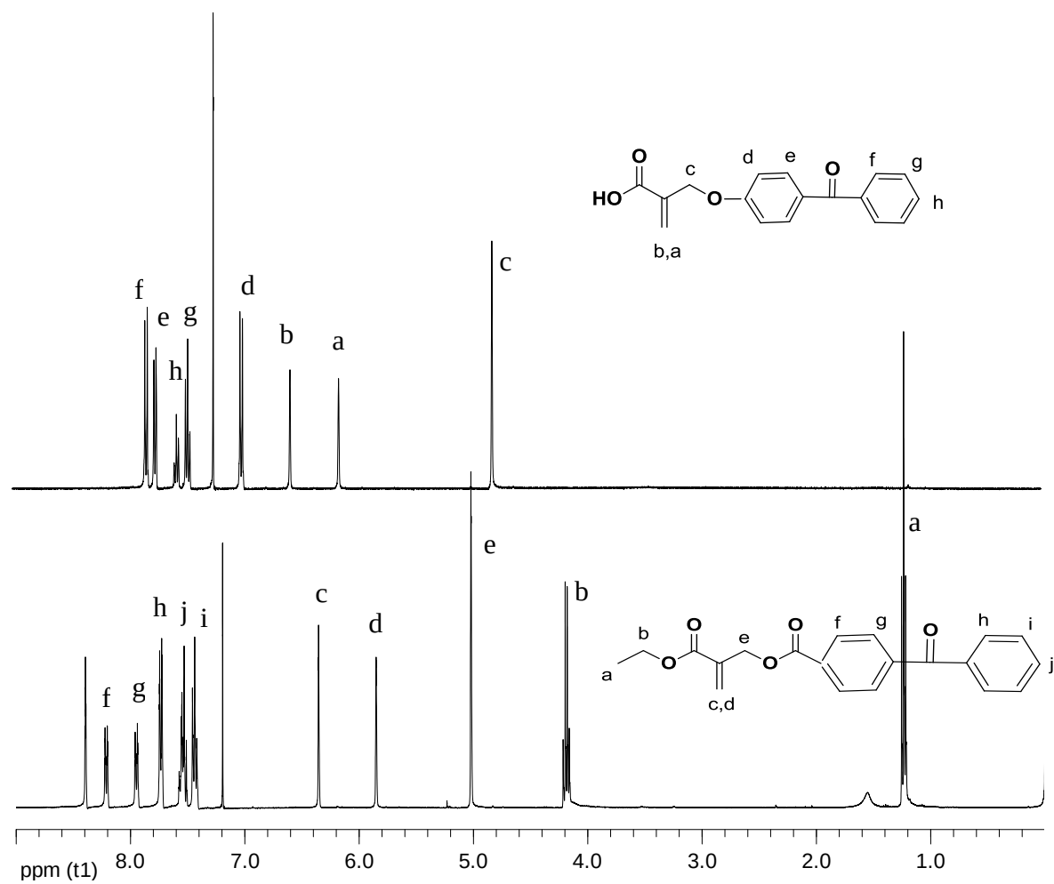
Figure 7.4. ^1\text{H} NMR spectra of E2 and E3 .
