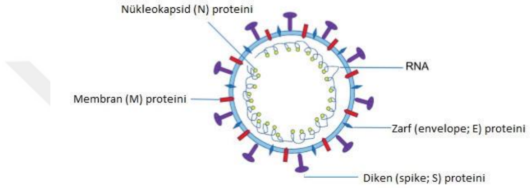
Şekil 5: Koronavirüsün şematik yapısı (TC Sağlık Bakanlığı COVID-19 Genel Bilgiler, Epidemiyoloji ve Tanı,2020,7)
