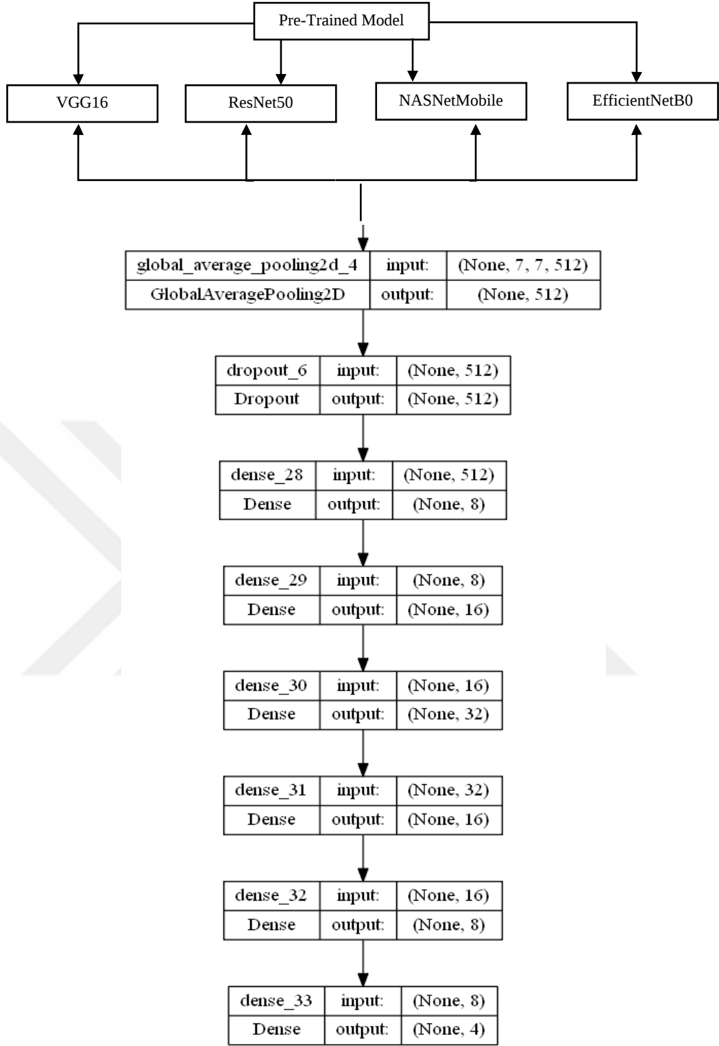
Şekil 38 Bu Tezde Önerilen Önceden Eğitilmiş Modellerin Araştırılması Yöntemi.
