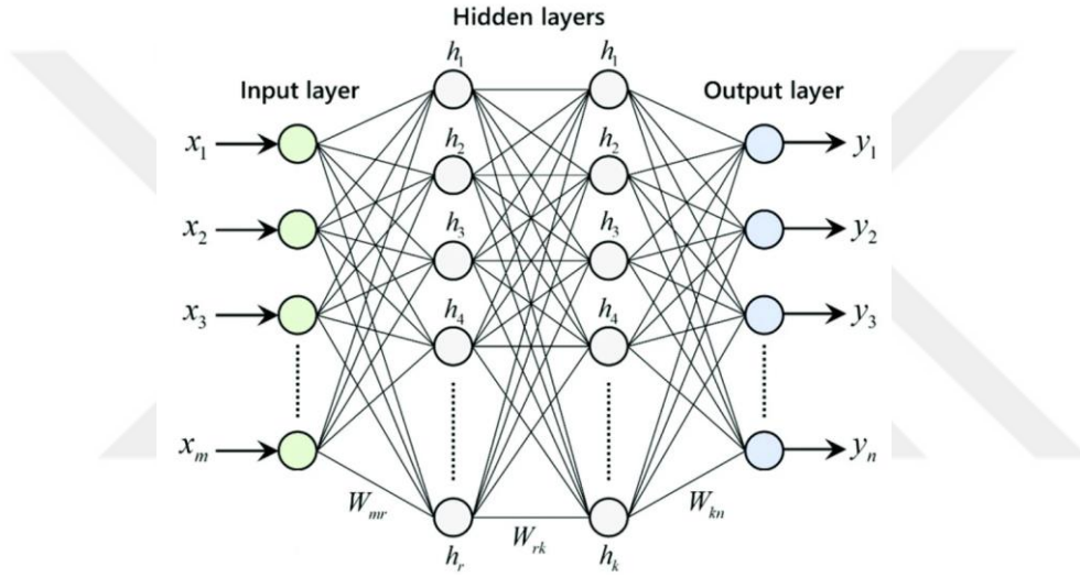
Şekil 23 İki Gizli Katman İçeren DNN Mimarisi Örneği. Oklar Ağırlıkları Temsil Ederken, Döğümler Girdi, Gizli ve Çıktı Değişkenlerini Temsil Eder. Değiştirilmiş Resim
