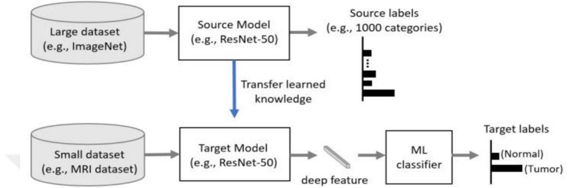
Şekil 14 Transfer Öğrenme Kavramı
