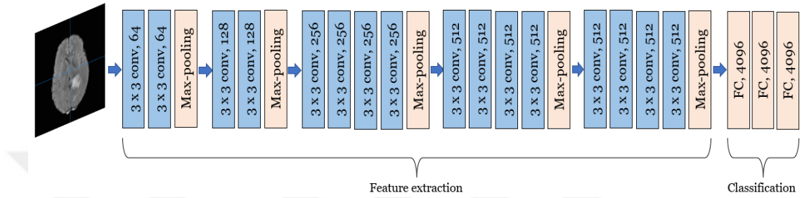
řekil 37 VGG-19 Modelinin Temel Mimari Yapısı.
