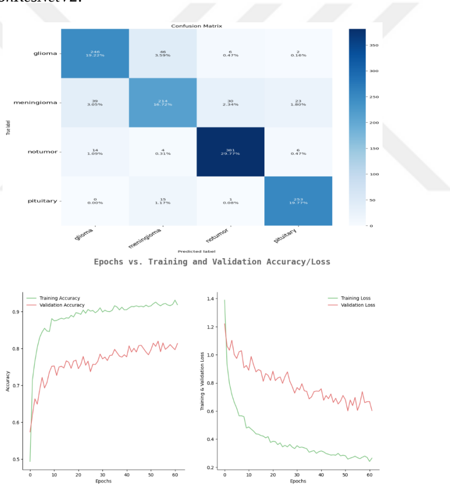
Şekil 41 InceptionResnetv2 Sonuçları Metrikleri ve Karışıklık Matrisi
