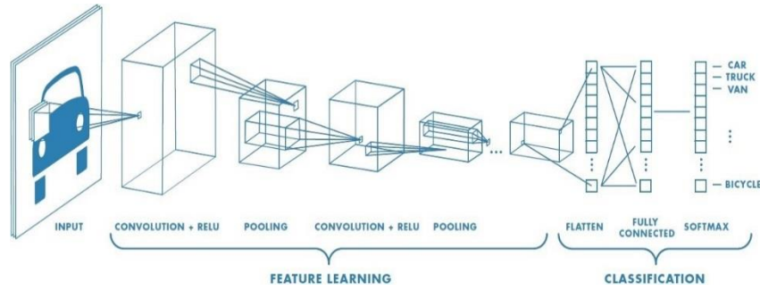
Şekil 24 CNN'nin Mimarisi.
