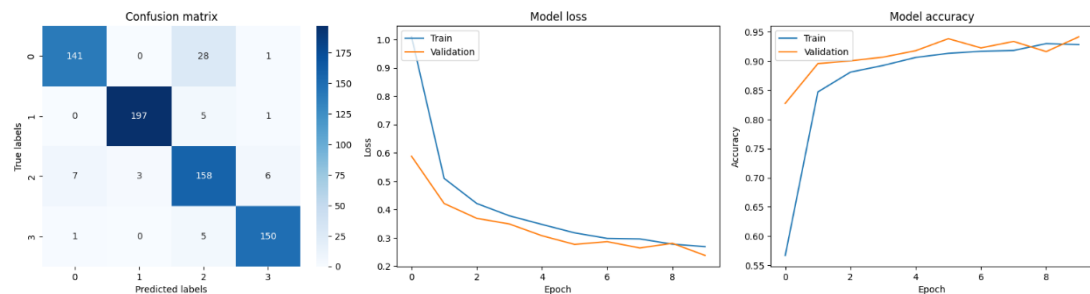
Şekil 39 EfficientNetB0 Sonuçları
