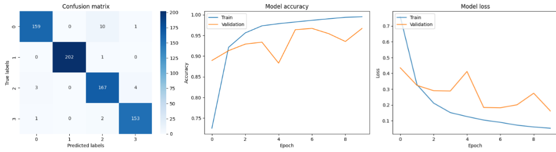
Şekil 40 Resnet50 Sonuçları
