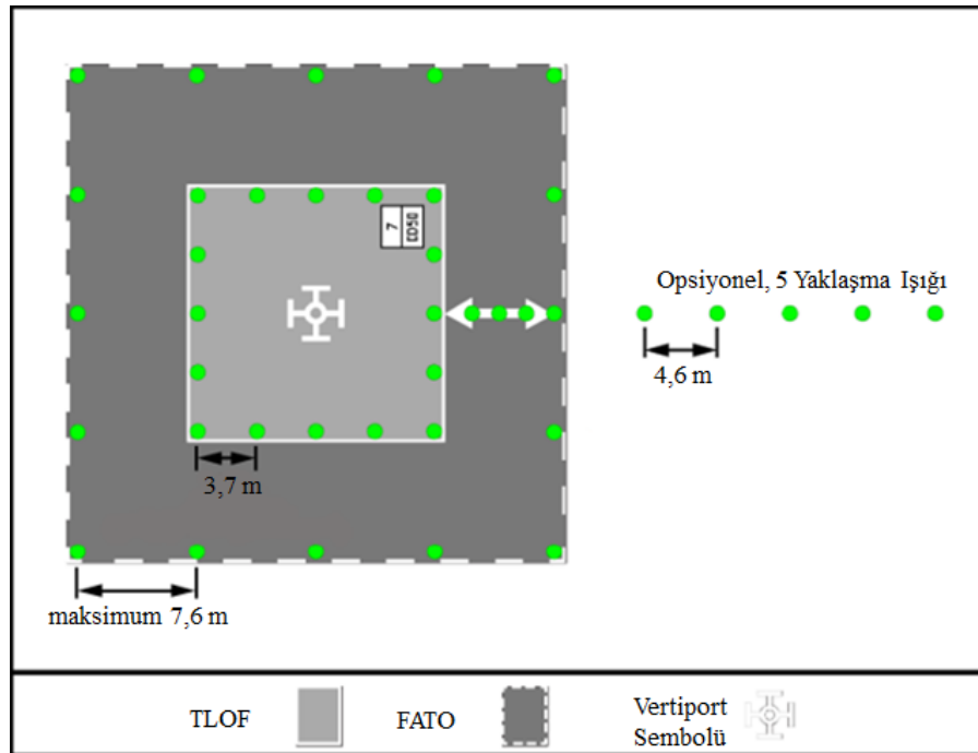
Şekil 4.10. TLOF/FATO çevre ışıklandırması (Federal Aviation Administration, 2022)
