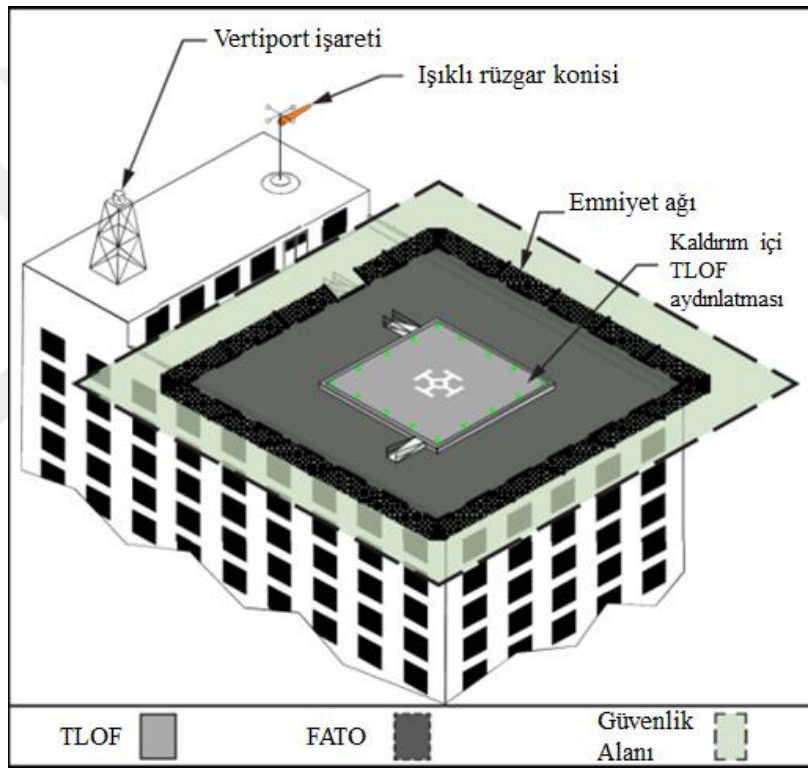
Şekil 4.11. Yükseltilmiş vertiport yapılandırma örneği (Federal Aviation Administration, 2022)
