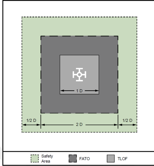
Şekil 4.2. TLOF, FATO ve SA ilişkisi ve boyutları (Federal Aviation Administration, 2022)
