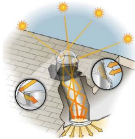
Şekil 26 Gün ışığı tüpünün kullanım prensibinin şematik gösterimi
