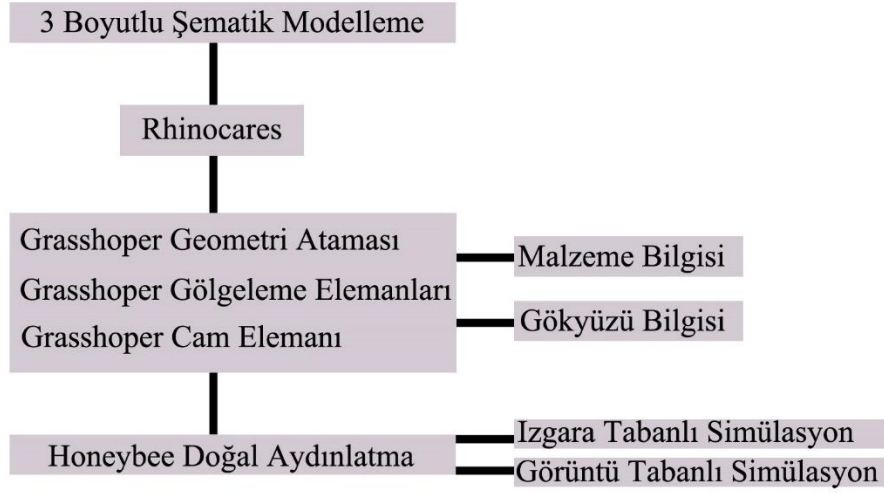
Şekil 47 Simülasyon Akış Şeması (Kaynak: Yazar, 2022))
