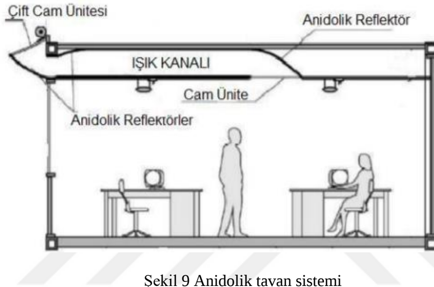
Şekil 9 Anidolik tavan sistemi
