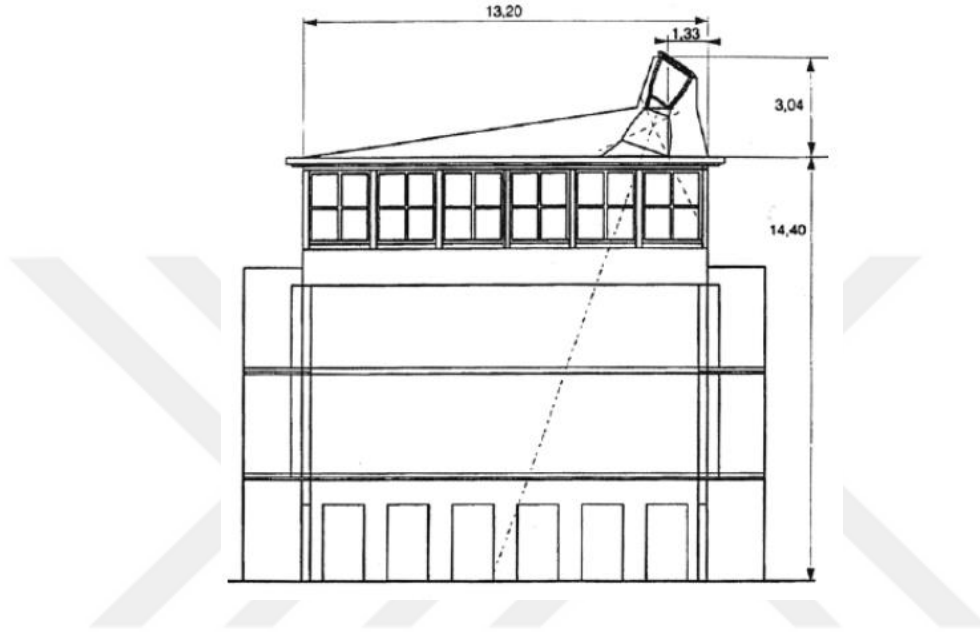
Şekil 12 Tessin Kantonu Arşivleri binasının anidolik tepe açıklığı sisteminin de eklendiği atrium kesiti
