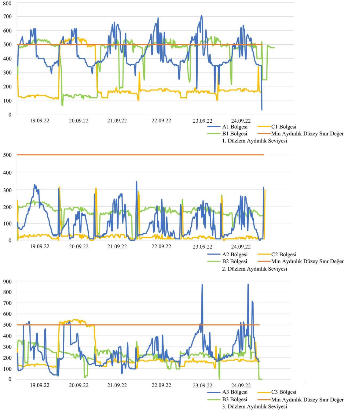
Şekil 51 Gençlik Salonu Aydınlik Düzeyi Ölçüm Sonuçları Grafiği
