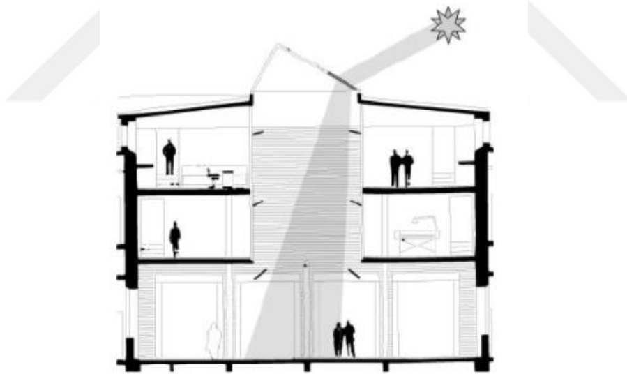
Şekil 40 Bir binanın atriumuna yerleştirildiğinde, ışık yönlendirici camın davranışını gösteren kesit
