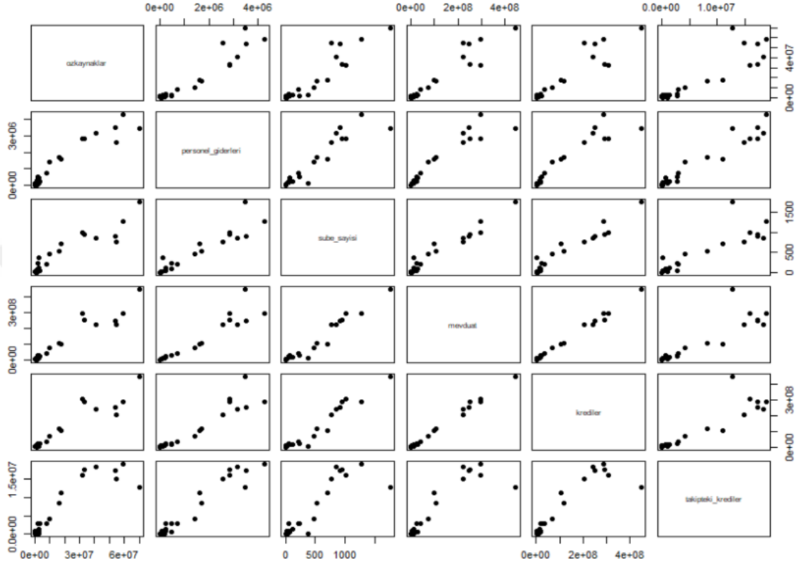
Şekil 16: Mevduat Bankaları'nın Girdi-Çıktı Değişkenlerine Yönelik Saçılım Grafiği
