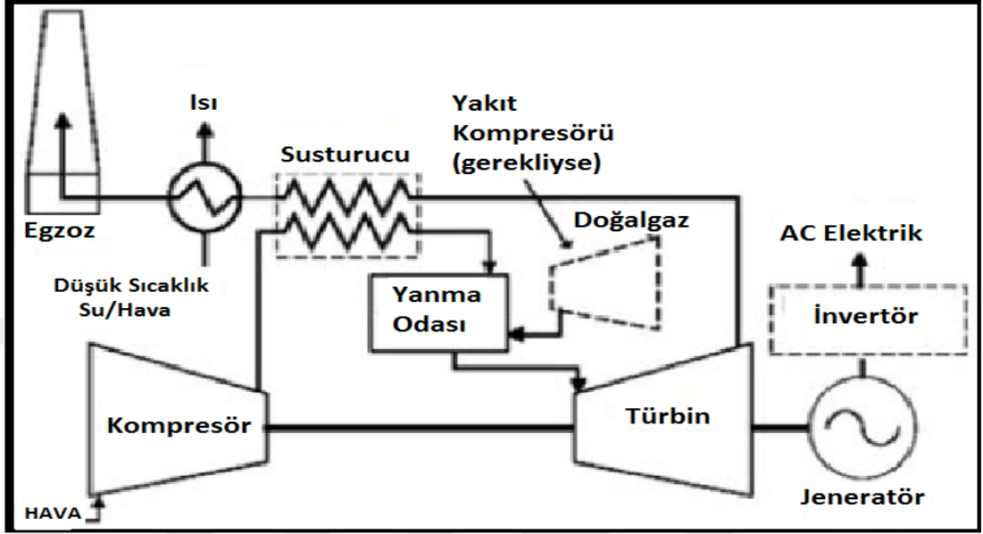
Şekil 2.8 : Biyogaz mikro-türbin yapısı (Al Seadi, vd. 2008).
