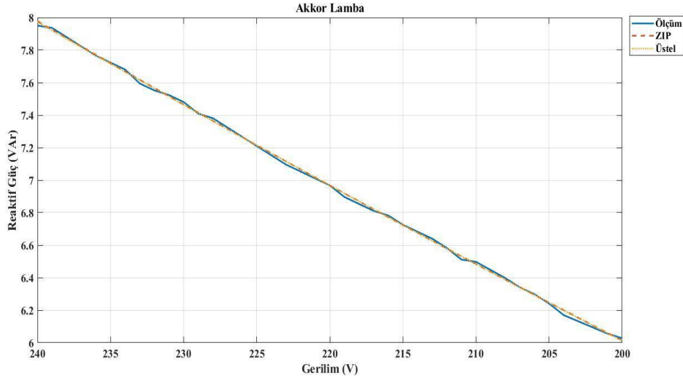
řekil 4.2. Akkor lamba gerilim - reaktif g eęrisi.
