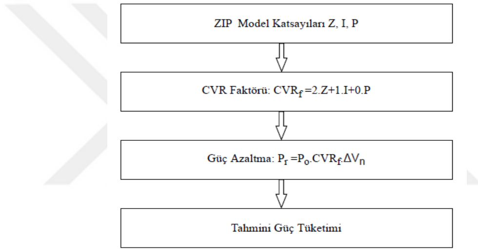
Şekil 3.1. Tahmini güç tüketimi akış şeması.
