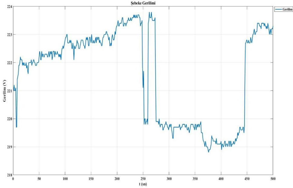
Şekil 4.34. Şebeke geriliminin zamana değişimi.
