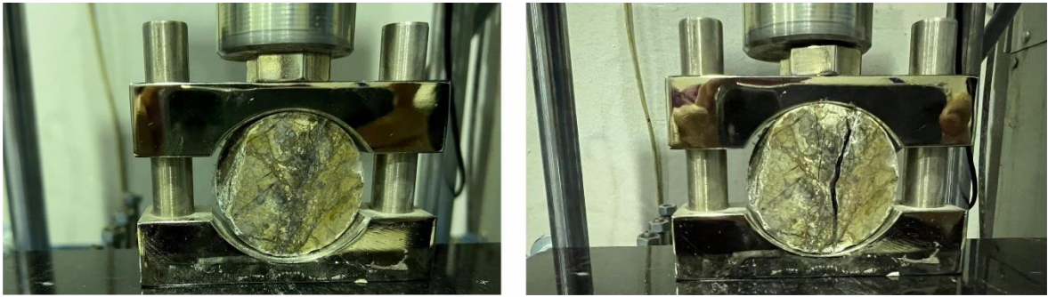
Şekil 4.11: İndirekt çekme deneyinin deneyi uygulanması
