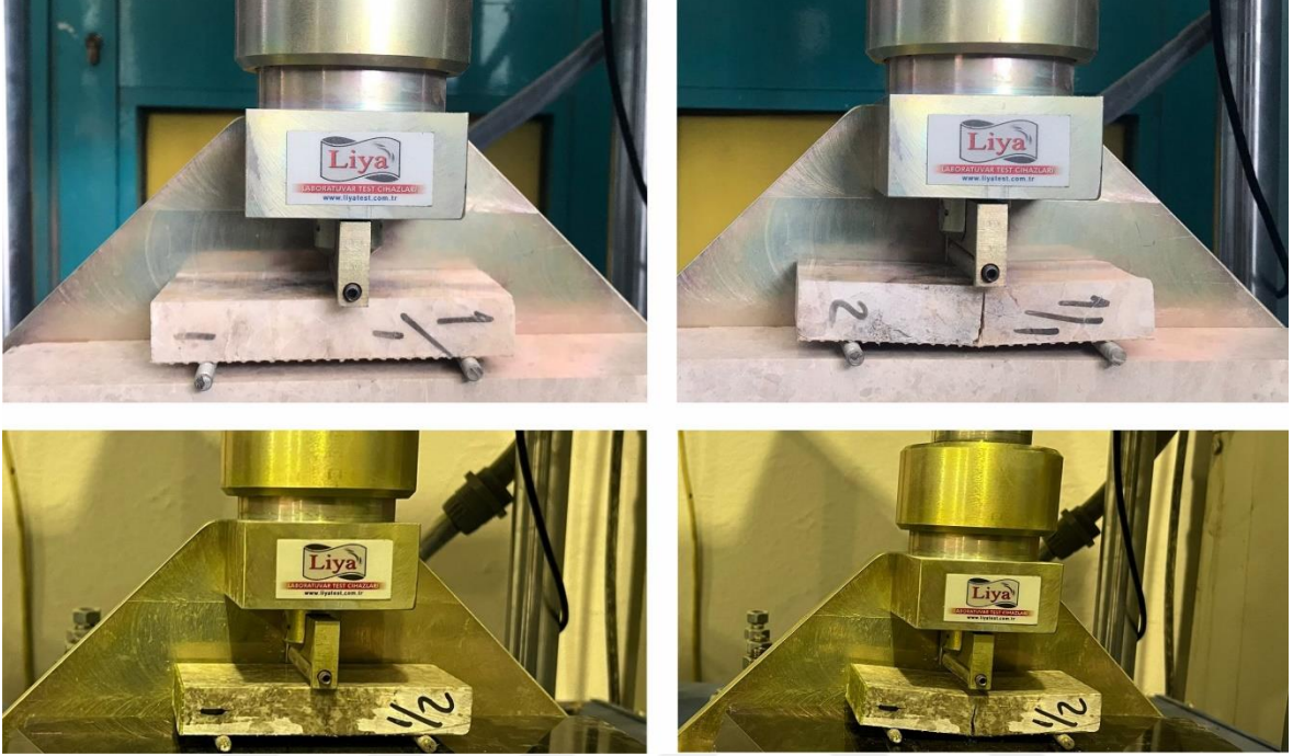
Şekil 4.12: Eğilme dayanımı deneyi öncesi ve sonrası görünüm.
