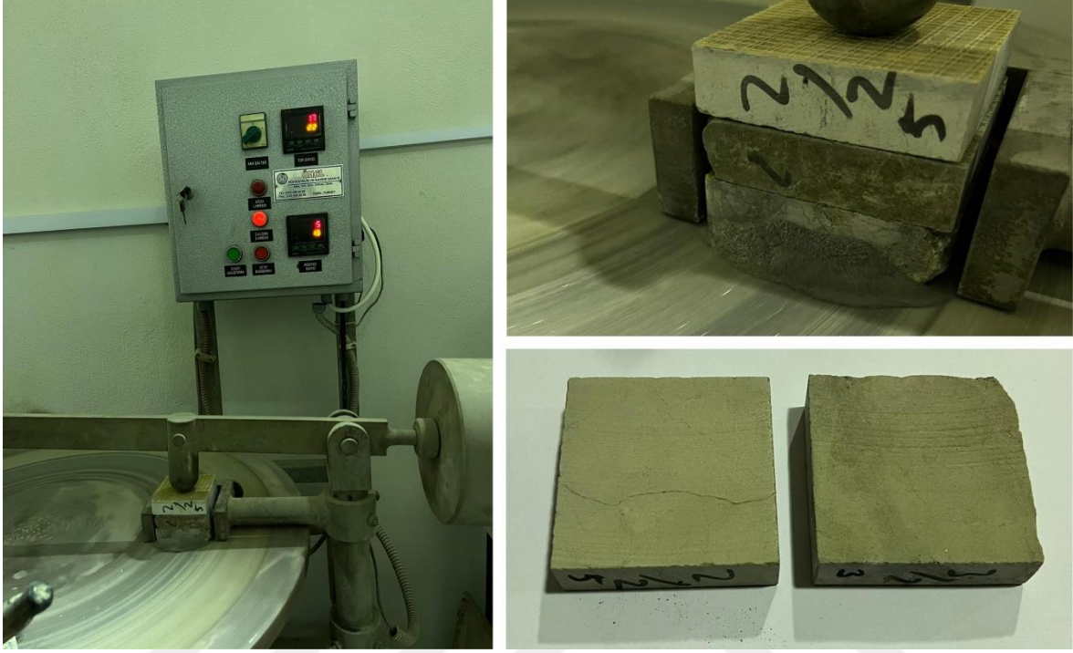
Şekil 4.7: Böhme aşınma deneyi
