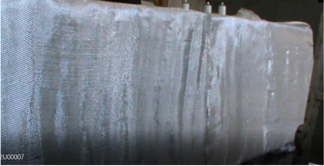
Şekil 1.16: Tamamı cam elyaf file ile sarılmış bohcalanmış blok örneği.
