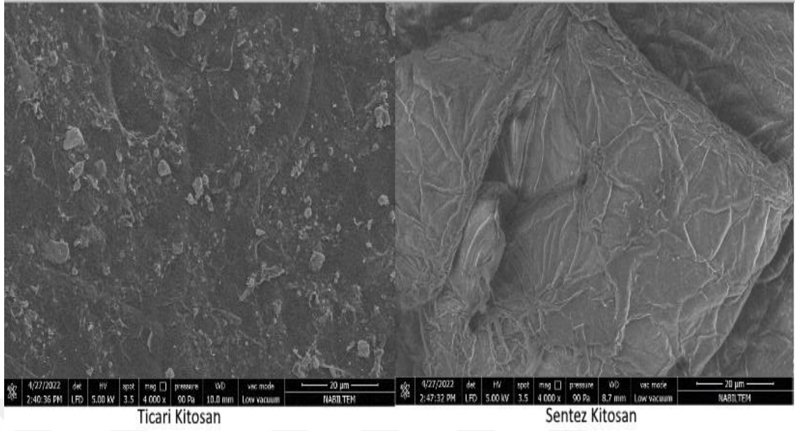
Şekil 7.12. Ticari Kitosan (Solda) ve Sentez Kitosana (Sağda) Ait 4000x Yaklaşırma-20 µm Boyutta SEM Görüntüleri
