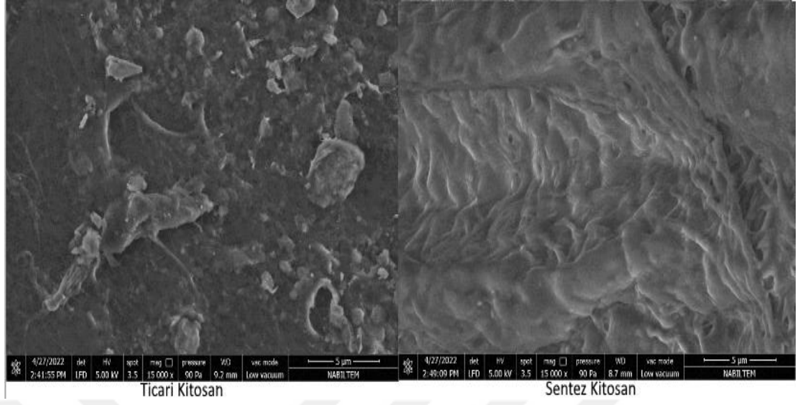
Şekil 7.14. Ticari Kitosan (Solda) ve Sentez Kitosana (Sağda) Ait 15000x Yaklaşırma-5 µm Boyutta SEM Görüntüleri
