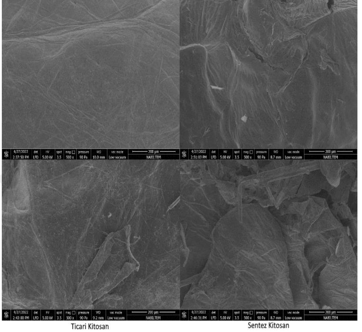
Şekil 7.9. Ticari Kitosan (Solda) ve Sentez Kitosana (Sağda) Ait 500x Yaklaşdırma-200 µm Boyutta SEM Görüntüleri
