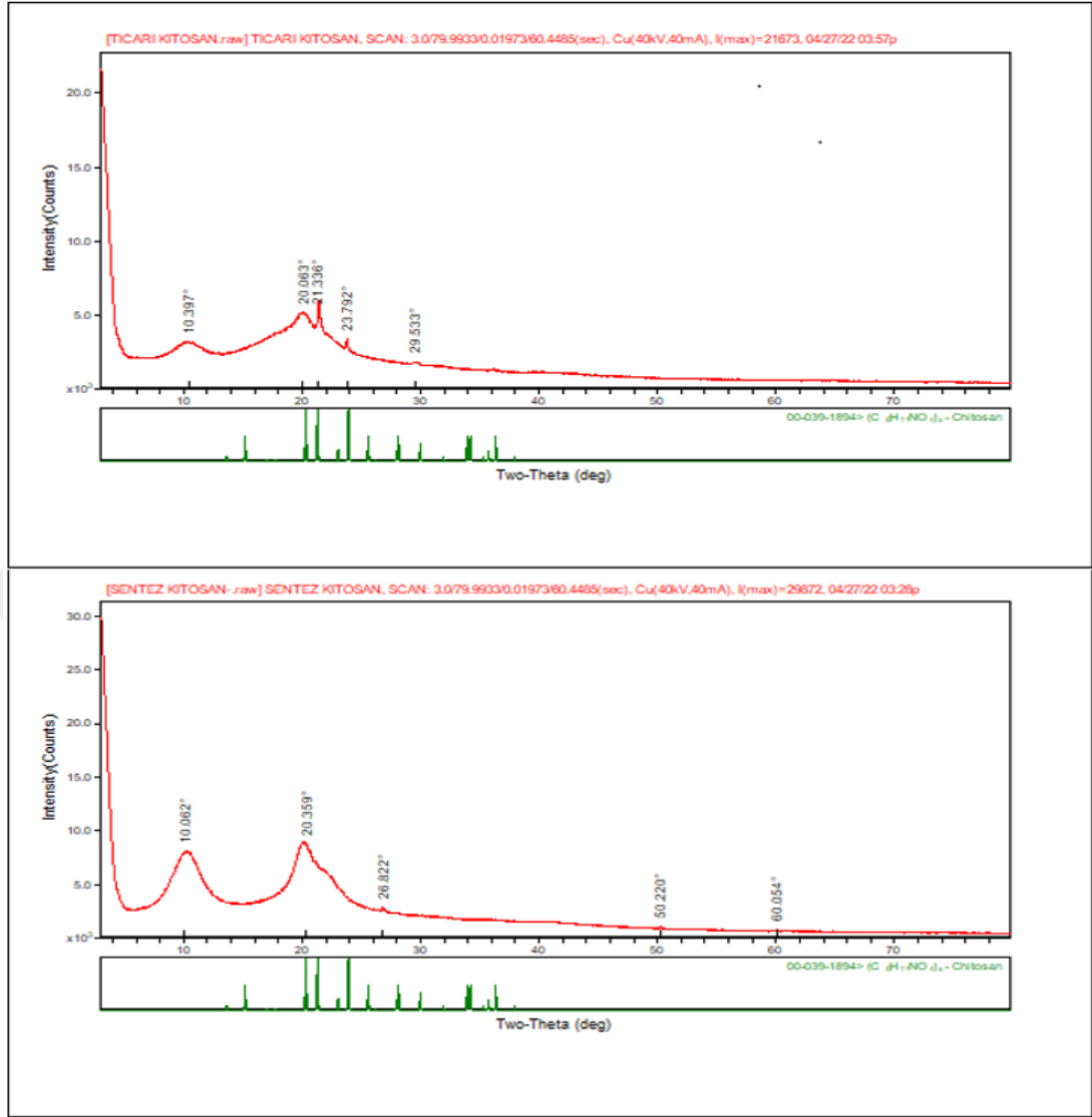
Şekil 7.6. Ticari Kitosana ve Sentez Kitosana Ait XRD Analiz Sonuç Grafiği
