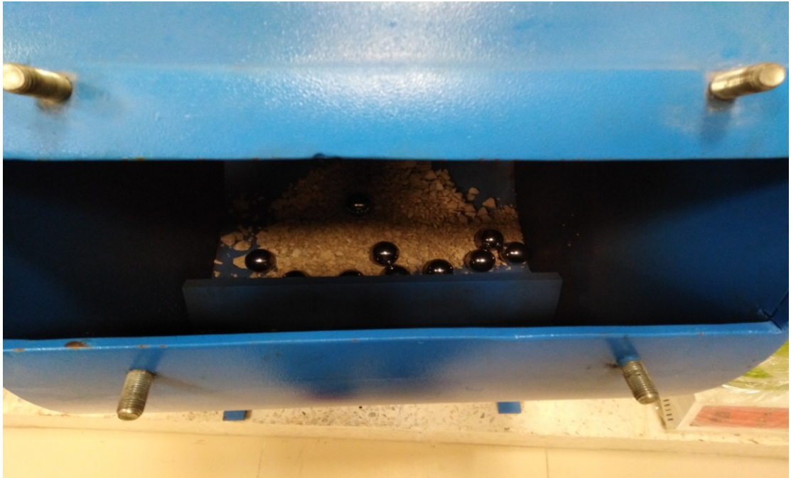
Şekil 3.7. Los Angeles Aşındırma Cihazı Tamburu
