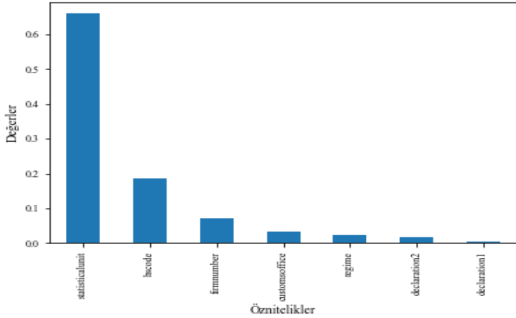
Şekil 41. Birim Modelinde Öz niteliklerin Ağırlığı
