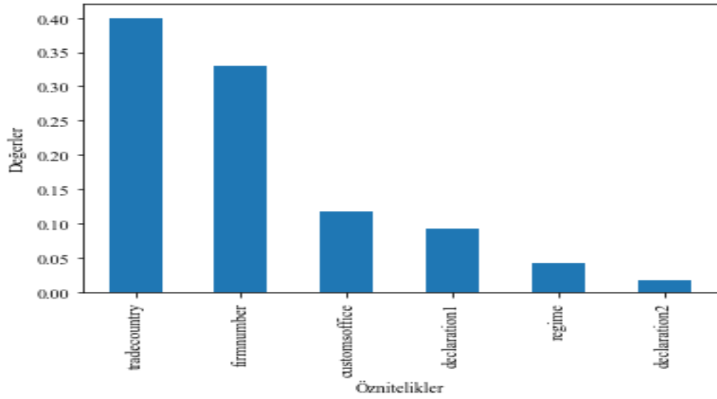
Şekil 39. Döviz Türü Modelinde Öz niteliklerin Ağırlığı
