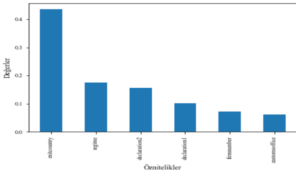
Şekil 42. Uluslararası Anlaşma Modelinde Öz niteliklerin Ağırlığı
