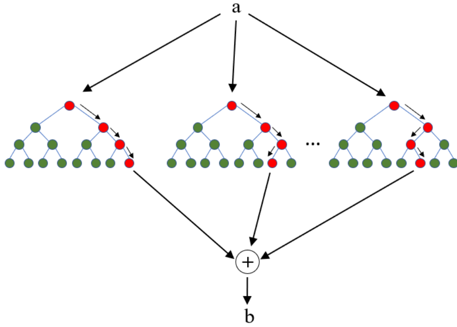
Şekil 19. Random Forest Mimarisi
