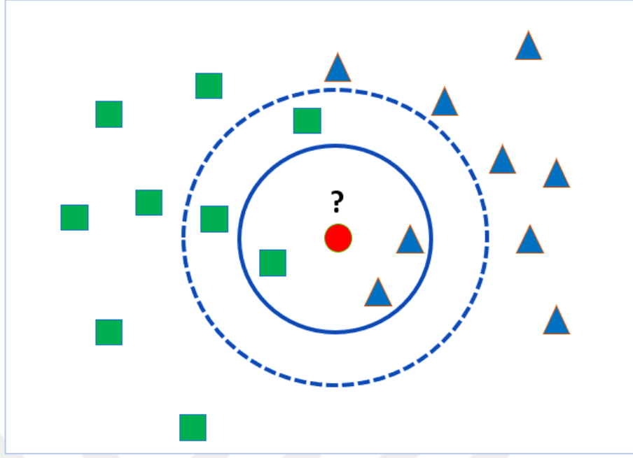
Şekil 16. KNN Algoritması Örneği
