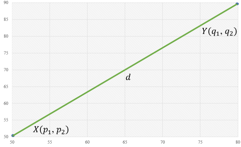
Şekil 17. Euclidean Uzaklığı
