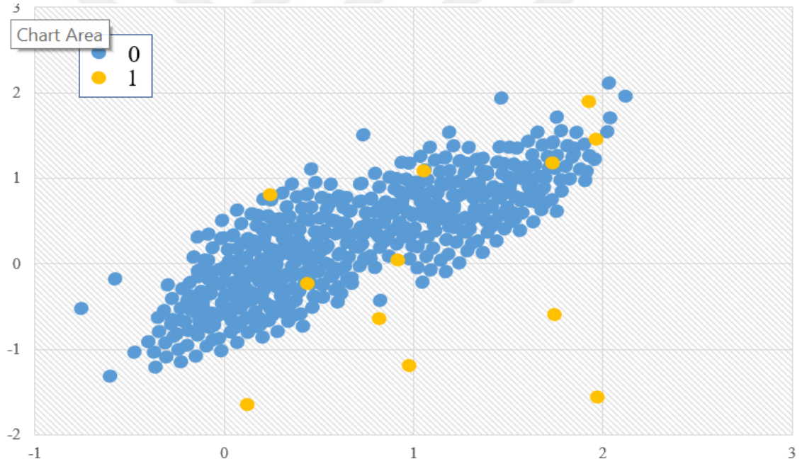
Şekil 12. Imbalanced Sınıflandırma
