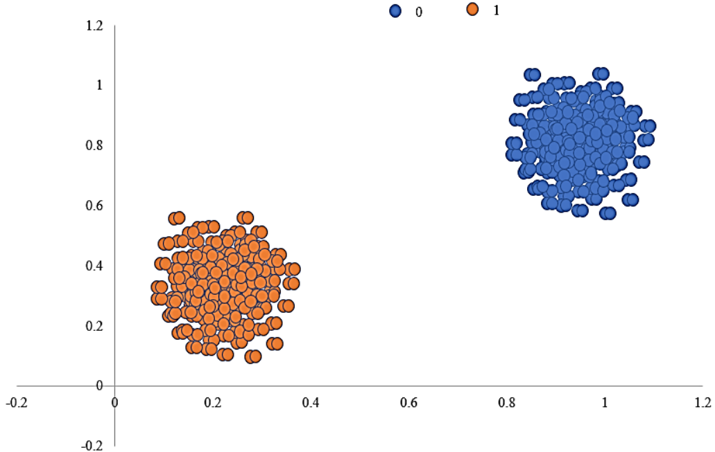
Şekil 10. Binary Sınıflandırma
