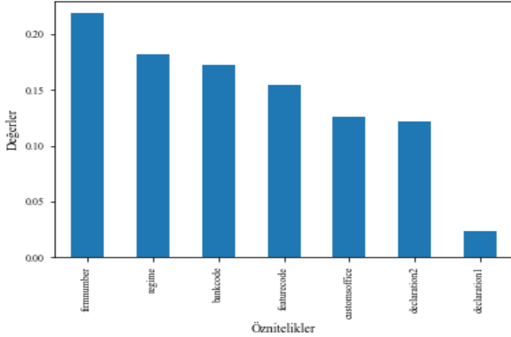
Şekil 43. Ödeme Şekli Modelinde Öz niteliklerin Ağırlığı
