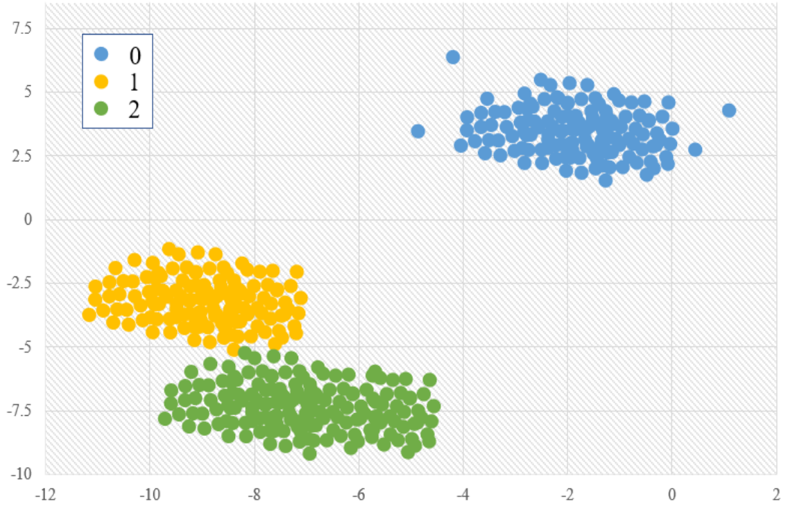
Şekil 11. Multi-Class Sınıflandırma
