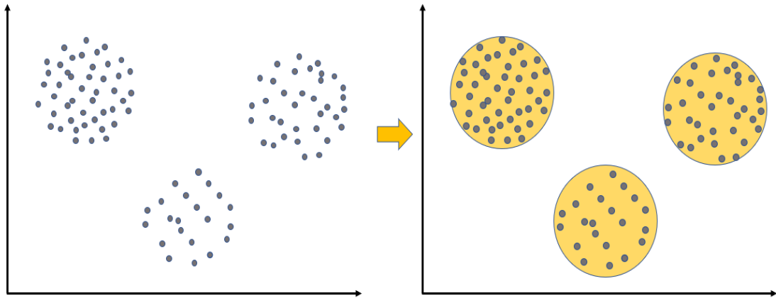
Şekil 13. Clustering
