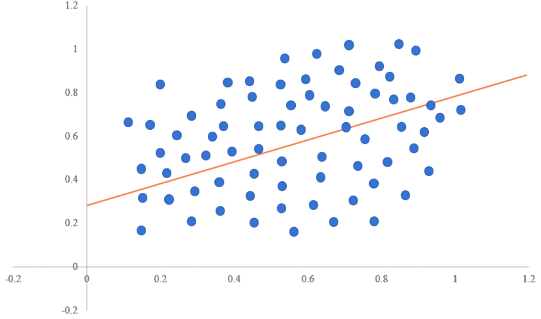
Şekil 9. Linear Regresyon Modeli
