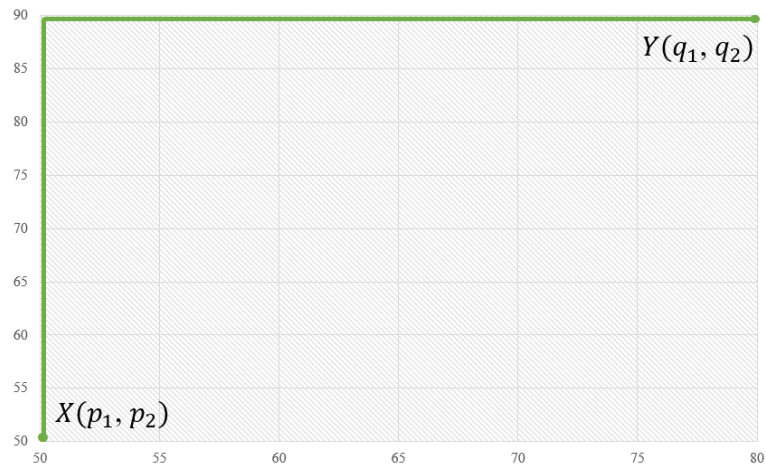
Şekil 18. Manhattan Uzaklığı
