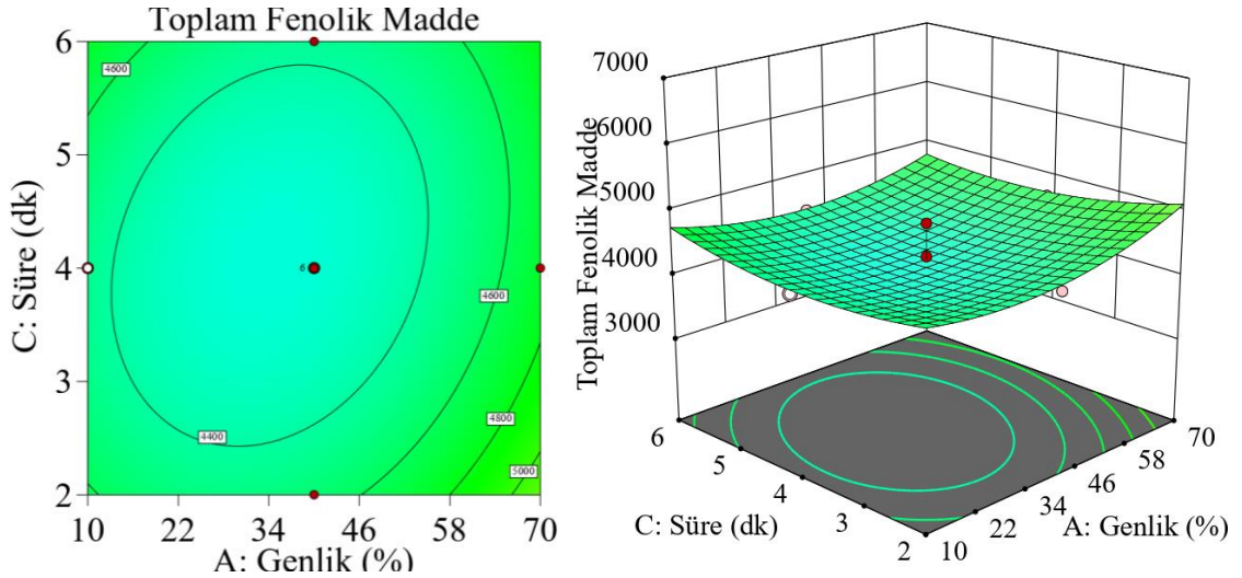
Şekil 4.4. Sabit sıcaklık ve etanol konsantrasyonunda, süre ve genlik değişkenlerinin ekstraktlardaki toplam fenolik madde miktarına etkisinin izohips ve yanıt yüzey grafiği (Sıcaklık 20 °C, Etanol konsantrasyonu %40, Süre 2-6 dk, Genlik %10-70)
