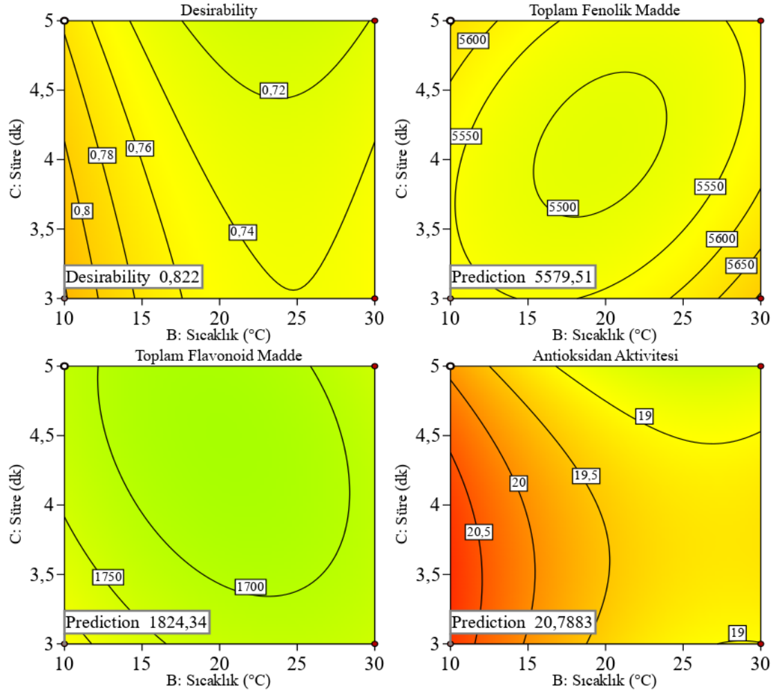
Şekil 4.29. Optimum koşullarda süre ve sıcaklık faktör etkileşiminin toplam fenolik madde miktarı, toplam flavonoid madde miktarı ve antioksidan aktivitesi üzerine etkisi ile istenebilirlik değerleri arasındaki ilişkiyi gösteren izohips grafikleri
