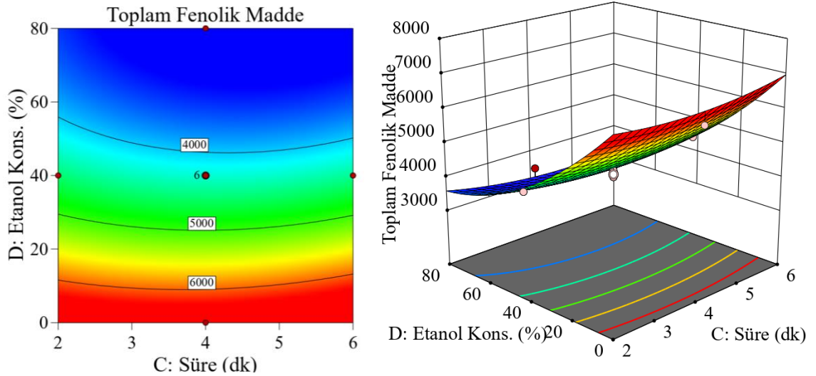
Şekil 4.8. Sabit sıcaklık ve genlikte, süre ve etanol konsantrasyonu değişkenlerinin ekstraktlardaki toplam fenolik madde miktarına etkisinin izohips ve yanıt yüzey grafiği (Sıcaklık 20 °C, Genlik %40, Süre 2-6 dk, Etanol konsantrasyonu %0-80)
