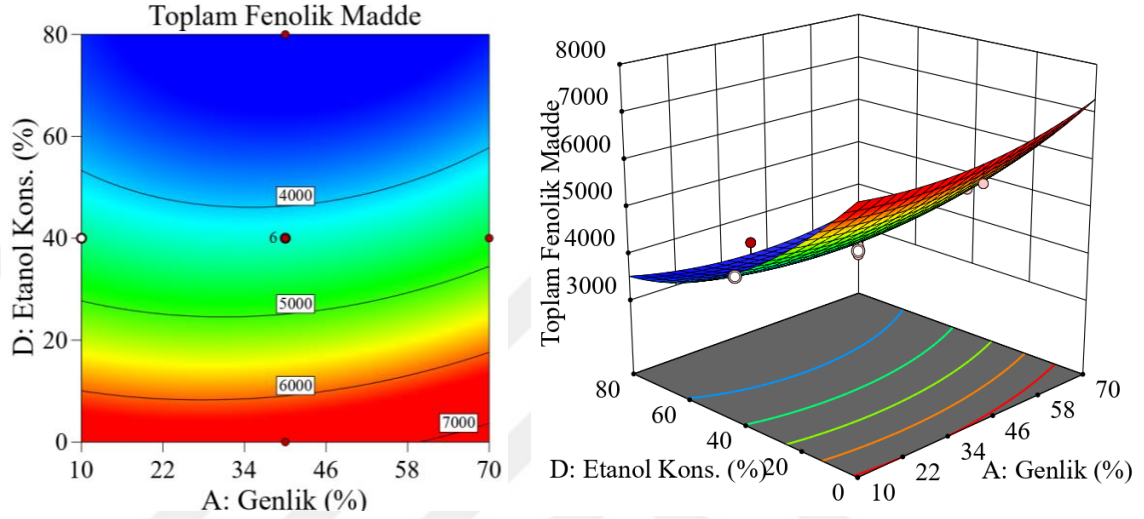
Şekil 4.6. Sabit sıcaklık ve sürede, etanol konsantrasyonu ve genlik değişkenlerinin ekstraktlardaki toplam fenolik madde miktarına etkisinin izohips ve yanıt yüzey grafiği (Sıcaklık 20 °C, Süre 4 dk, Etanol konsantrasyonu %0-80, Genlik %10-70)
