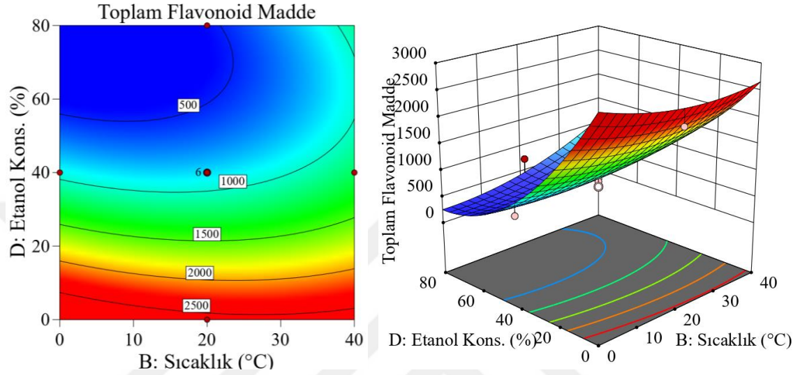
Şekil 4.15. Sabit süre ve genlikte, etanol konsantrasyonu ve sıcaklık değişkenlerinin ekstraktlardaki toplam flavonoid madde miktarına etkisinin izohips ve yanıt yüzey grafiği (Süre 4 dk, Genlik %40, Sıcaklık 0-40 °C, Etanol konsantrasyonu %0-80)
