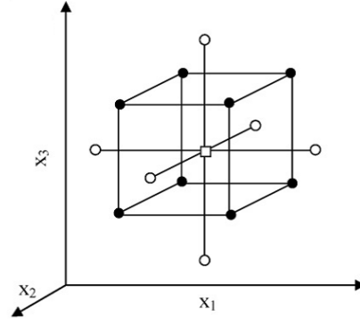
Şekil 2.9. Merkez nokta (□), faktöriyel noktaları (●) ve yıldız noktalarını (○) içeren 3 faktörlü bir deneme için oluşturulan merkezi kompozit tasarım (Bezerra vd., 2008)
