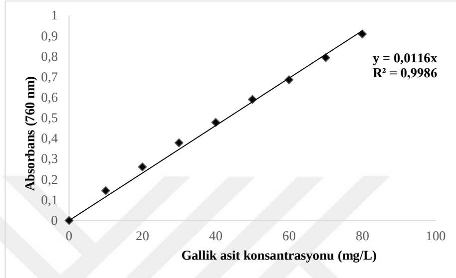
Şekil 3.3. Gallik asit kalibrasyon eğrisi
