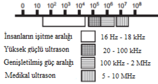
Şekil 2.2. Ses dalgası tipleri (Yağcıoğlu, 2015).
