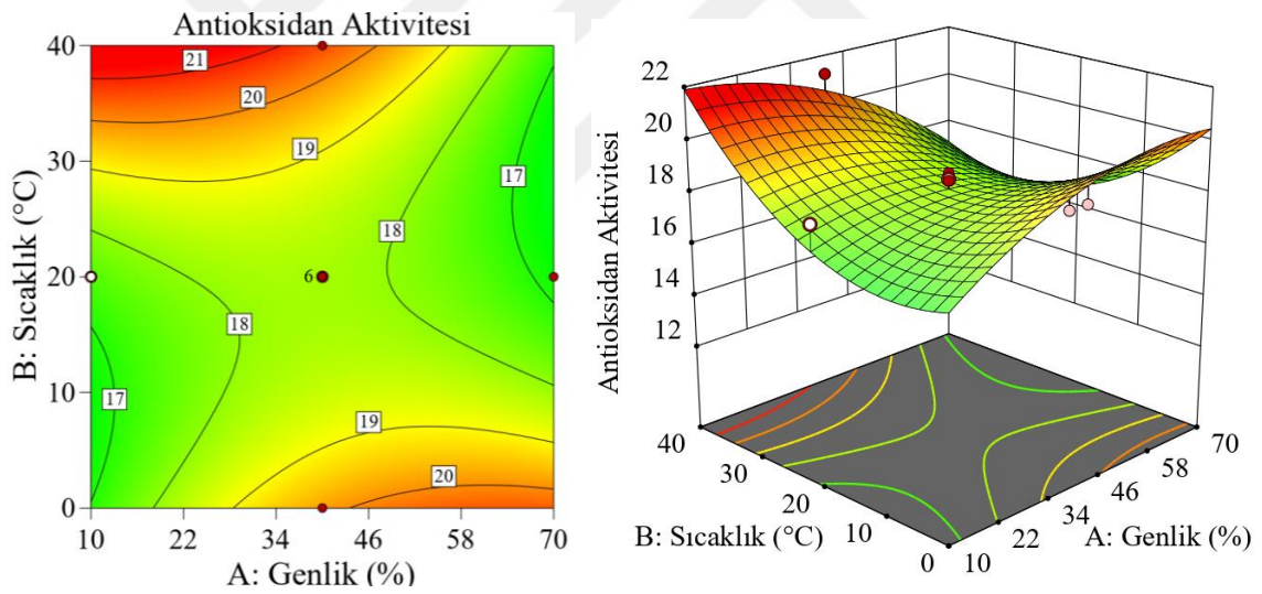
Şekil 4.19. Sabit etanol konsantrasyonu ve sürede, sıcaklık ve genlik değişkenlerinin ekstraktlardaki antioksidan aktiviteye etkisinin izohips ve yanıt yüzey grafiği (Süre 4 dk, Etanol konsantrasyonu %40, Sıcaklık 0-40 °C, Genlik %10-70)
