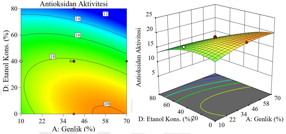
Şekil 4.22. Sabit süre ve sıcaklıkta, etanol konsantrasyonu ve genlik değişkenlerinin ekstraktlardaki antioksidan aktiviteye etkisinin izohips ve yanıt yüzey grafiği (Süre 4 dk, Sıcaklık 20 °C, Genlik %10-70, Etanol konsantrasyonu %0-80)
