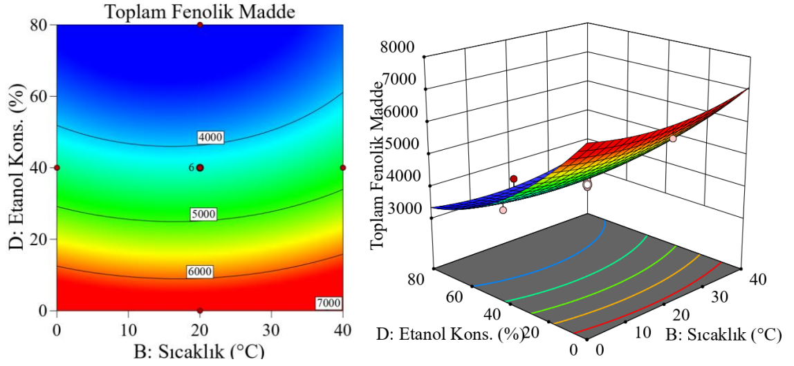
Şekil 4.7. Sabit süre ve genlikte, sıcaklık ve etanol konsantrasyonu değişkenlerinin ekstraktlardaki toplam fenolik madde miktarına etkisinin izohips ve yanıt yüzey grafiği (Süre 4 dk, Genlik %40, Sıcaklık 0-40 °C, Etanol konsantrasyonu %0-80)
