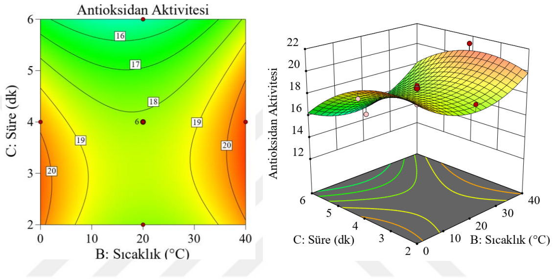
Şekil 4.21. Sabit etanol konsantrasyonu ve genlikte, süre ve sıcaklık değişkenlerinin ekstraktlardaki antioksidan aktiviteye etkisinin izohips ve yanıt yüzey grafiği (Genlik %40, Etanol konsantrasyonu %40, Süre 2-6 dk, Sıcaklık 0-40 °C)
