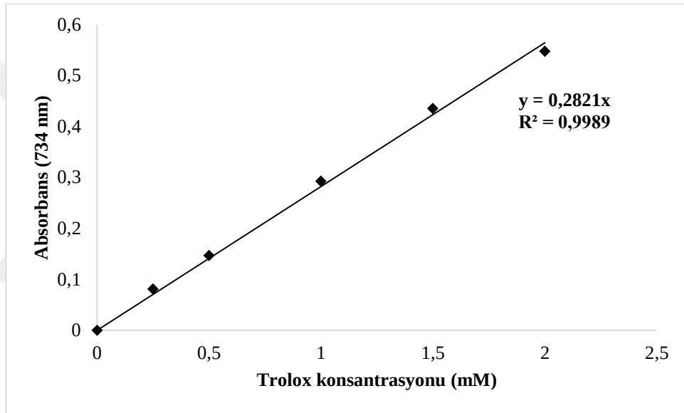
Şekil 3.5. Trolox kalibrasyon eğrisi
