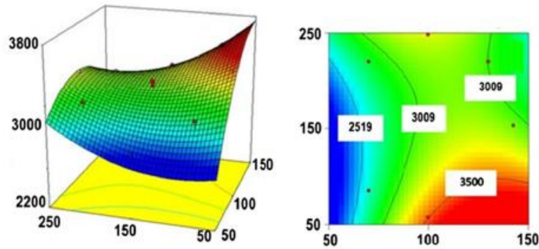
Şekil 2.10. Tahmin edilen örnek model denkleminin yanıt yüzeyi (sol) ve kontur (sağ) çizimleri (Yolmeh vd., 2017)
