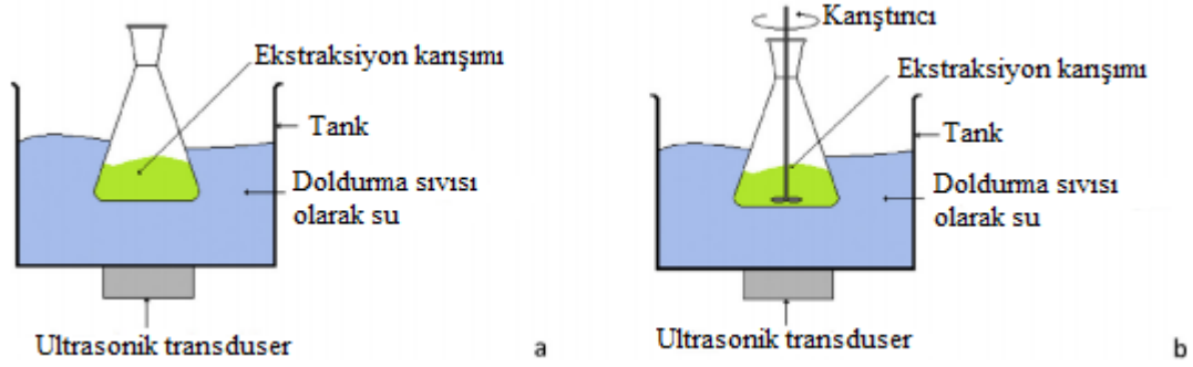
Şekil 2.7. Dolaylı sonikasyon için tankta ekstraksiyon kabı konumlandırma. a: karıştırılmamış ekstraksiyon; b: karıştırılmış ekstraksiyon (Vinatoru vd., 2017)
