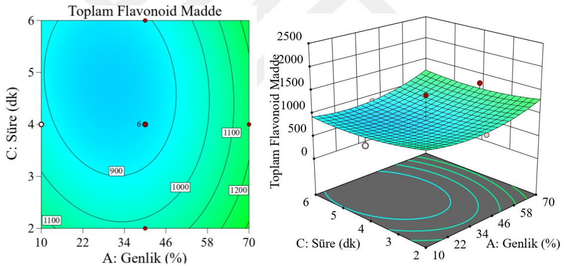
Şekil 4.12. Sabit etanol konsantrasyonu ve sıcaklıkta, süre ve genlik değişkenlerinin ekstraktlardaki toplam flavonoid madde miktarına etkisinin izohips ve yanıt yüzey grafiği (Etanol konsantrasyonu %40, Sıcaklık 20 °C, Süre 2-6 dk, Genlik %10-70)
