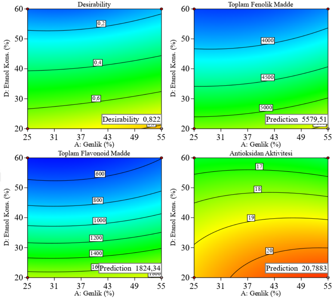
Şekil 4.28. Optimum koşullarda etanol konsantrasyonu ve genlik faktör etkileşiminin toplam fenolik madde miktarı, toplam flavonoid madde miktarı ve antioksidan aktivitesi üzerine etkisi ile istenebilirlik değerleri arasındaki ilişkiyi gösteren izohips grafikleri
