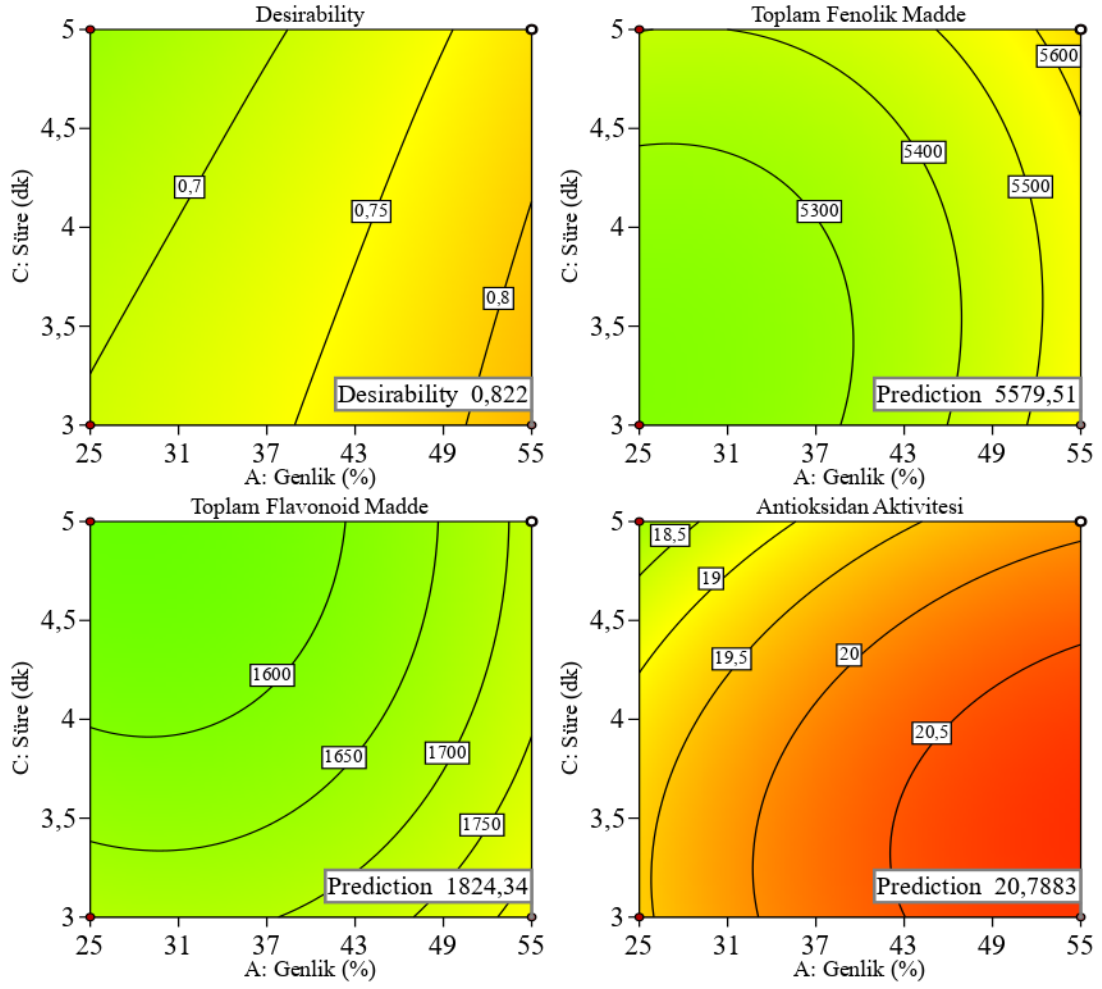
Şekil 4.27. Optimum koşullarda süre ve genlik faktör etkileşiminin toplam fenolik madde miktarı, toplam flavonoid madde miktarı ve antioksidan aktivitesi üzerine etkisi ile istenebilirlik değerleri arasındaki ilişkiyi gösteren izohips grafikleri
