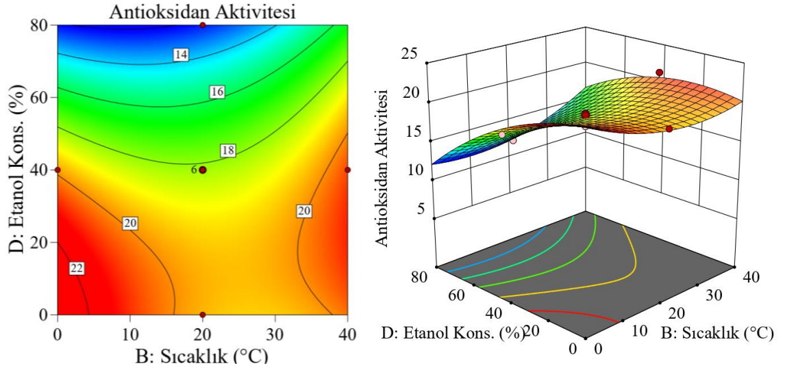
Şekil 4.23. Sabit süre ve genlikte, etanol konsantrasyonu ve sıcaklık değişkenlerinin ekstraktlardaki antioksidan aktiviteye etkisinin izohips ve yanıt yüzey grafiği (Süre 4 dk, Genlik %40, Sıcaklık 0-40 °C, Etanol konsantrasyonu %0-80)
