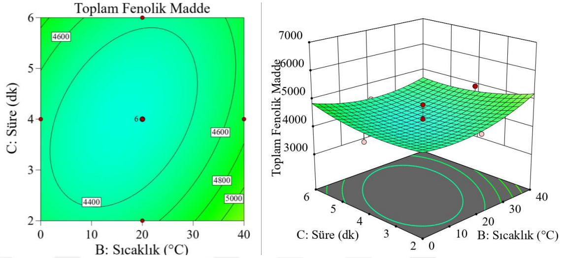
Şekil 4.5. Sabit etanol konsantrasyonu ve genlikte, sıcaklık ve süre değişkenlerinin ekstraktlardaki toplam fenolik madde miktarına etkisinin izohips ve yanıt yüzey grafiği (Etanol konsantrasyonu %40, Genlik %40, Sıcaklık 0-40 °C, Süre 2-6 dk)
