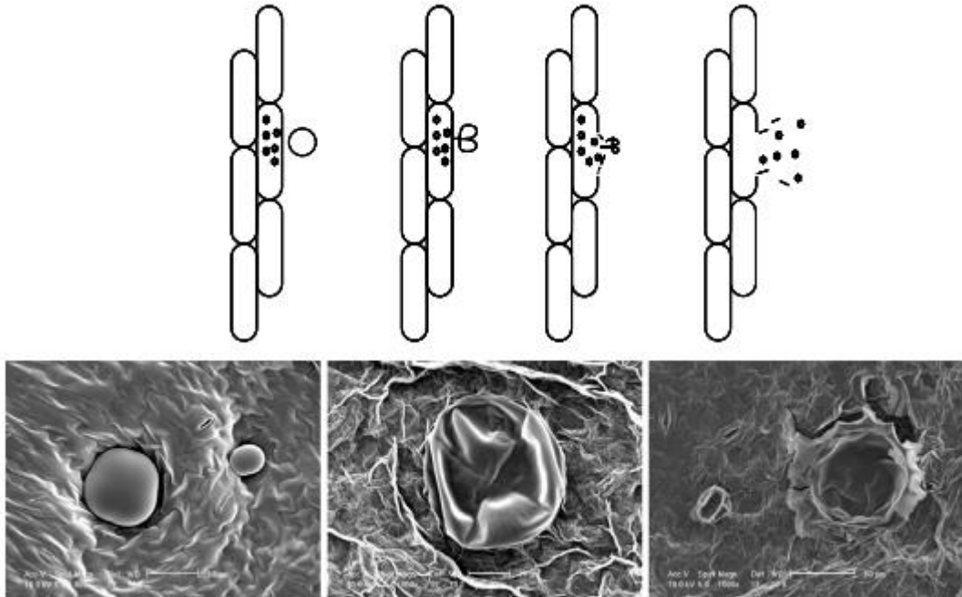
Şekil 2.5. Kavitasyon kabarcığı çökmesi ve bitki materyalinin serbest bırakılması (Chemat vd., 2011)
