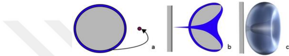
Şekil 2.4. Parçacıklara çarpan jetlerin mekanik etkileri, çöken baloncukların (a) simetrik ve (b) asimetrik gösterimi ve (c) halka şeklinin çizimi (Vinatoru vd., 2017)
