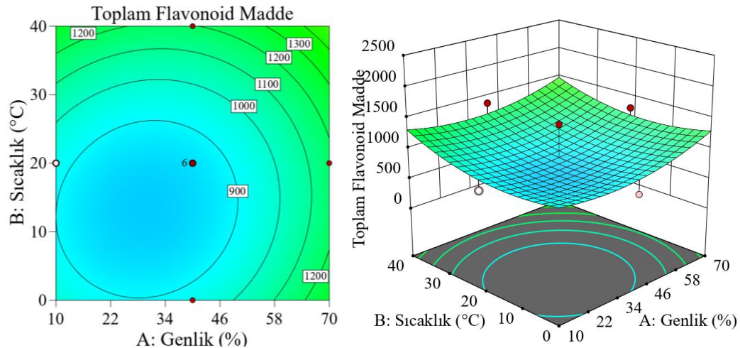
Şekil 4.11. Sabit etanol konsantrasyonu ve sürede, sıcaklık ve genlik değişkenlerinin ekstraktlardaki toplam flavonoid madde miktarına etkisinin izohips ve yanıt yüzey grafiği (Etanol konsantrasyonu %40, Süre 4 dk, Sıcaklık 0-40 °C, Genlik %10-70)
