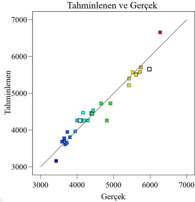
Şekil 4.1. Ekstraktların karesel model üzerinde toplam fenolik madde yanıtı için tahminlenen ve gerçek verileri
