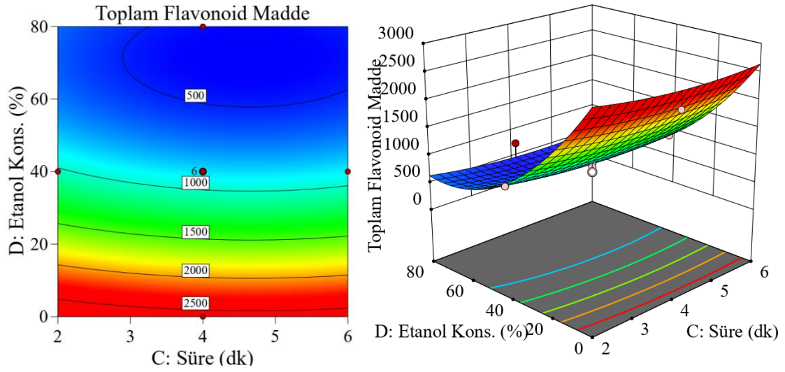
Şekil 4.16. Sabit sıcaklık ve genlikte, etanol konsantrasyonu ve süre değişkenlerinin ekstraktlardaki toplam flavonoid madde miktarına etkisinin izohips ve yanıt yüzey grafiği (Sıcaklık 20 °C, Genlik %40, Süre 2-6 dk, Etanol konsantrasyonu %0-80)
