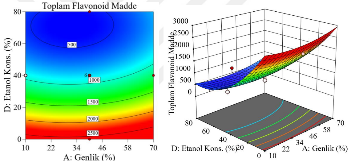
Şekil 4.14. Sabit süre ve sıcaklıkta, etanol konsantrasyonu ve genlik değişkenlerinin ekstraktlardaki toplam flavonoid madde miktarına etkisinin izohips ve yanıt yüzey grafiği (Süre 4 dk, Sıcaklık 20 °C Etanol konsantrasyonu %0-80, Genlik %10-70)
