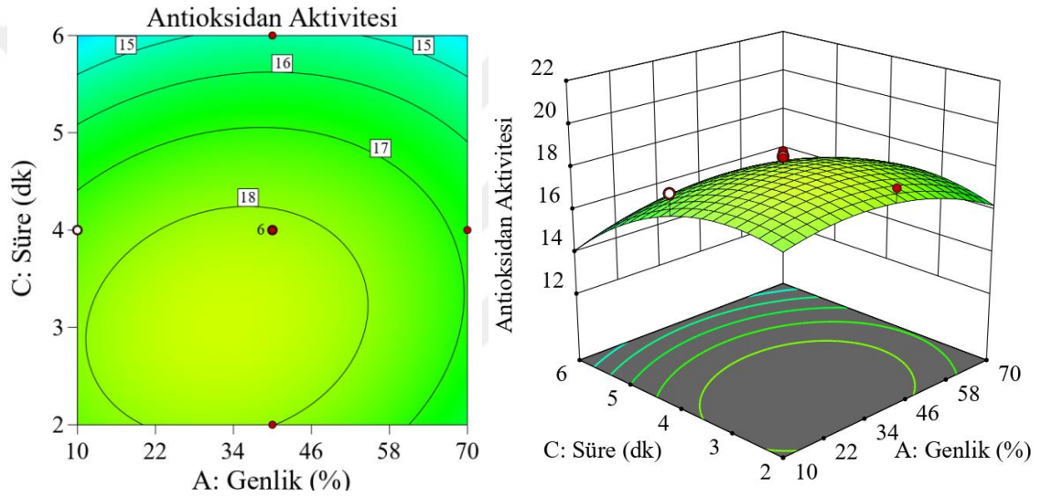
Şekil 4.20. Sabit etanol konsantrasyonu ve sıcaklıkta, süre ve genlik değişkenlerinin ekstraktlardaki antioksidan aktiviteye etkisinin izohips ve yanıt yüzey grafiği (Sıcaklık 20 °C, Etanol konsantrasyonu %40, Süre 2-6 dk, Genlik %10-70)
