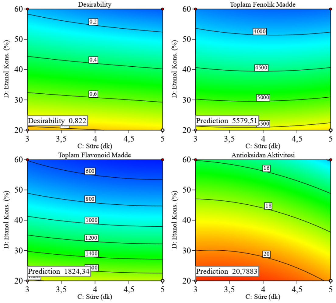
Şekil 4.31. Optimum koşullarda etanol konsantrasyonu ve süre faktör etkileşiminin toplam fenolik madde miktarı, toplam flavonoid madde miktarı ve antioksidan aktivitesi üzerine etkisi ile istenebilirlik değerleri arasındaki ilişkiyi gösteren izohips grafikleri
