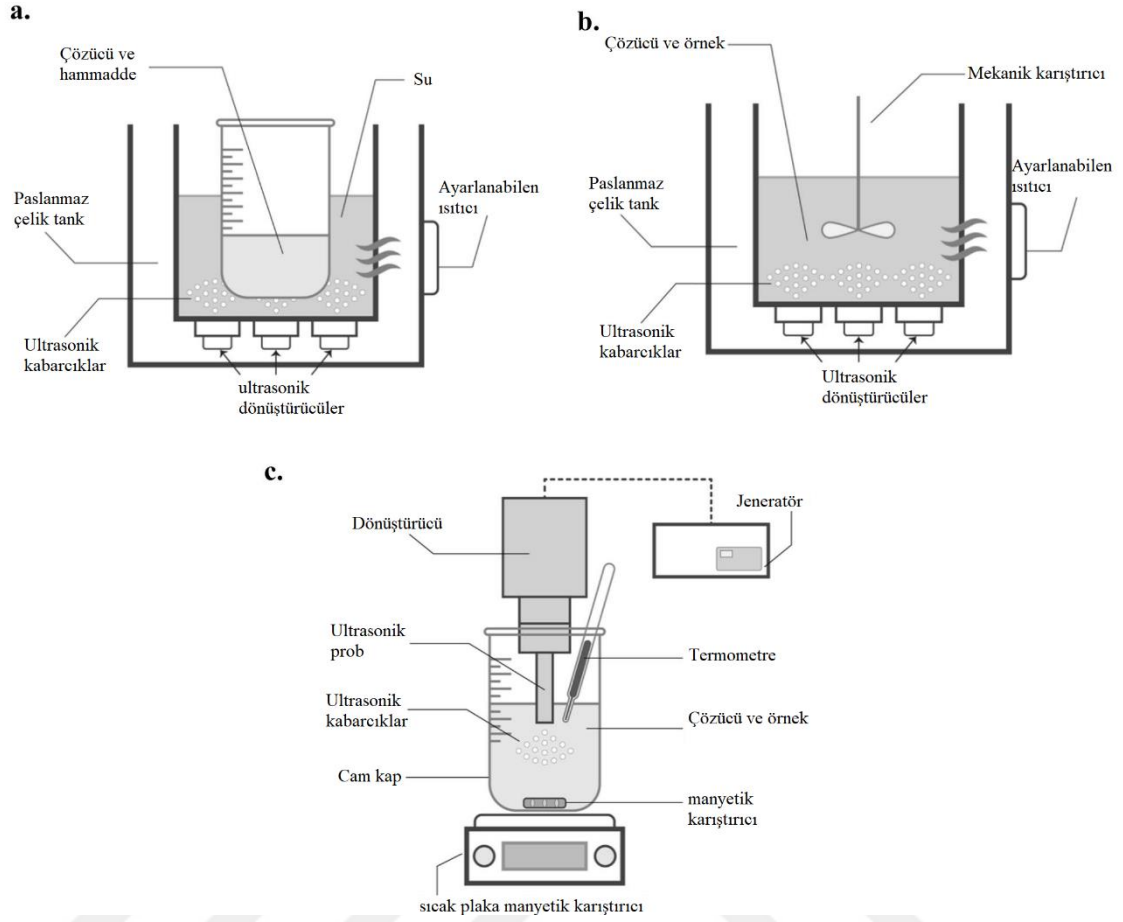
Şekil 2.8. a) Dolaylı ekstraksiyon için ultrasonik temizleme banyosu b) Doğrudan ekstraksiyon için temizleme banyosu c) Doğrudan ekstraksiyon için ultrasonik prob (Martinez-Solano vd., 2021)
