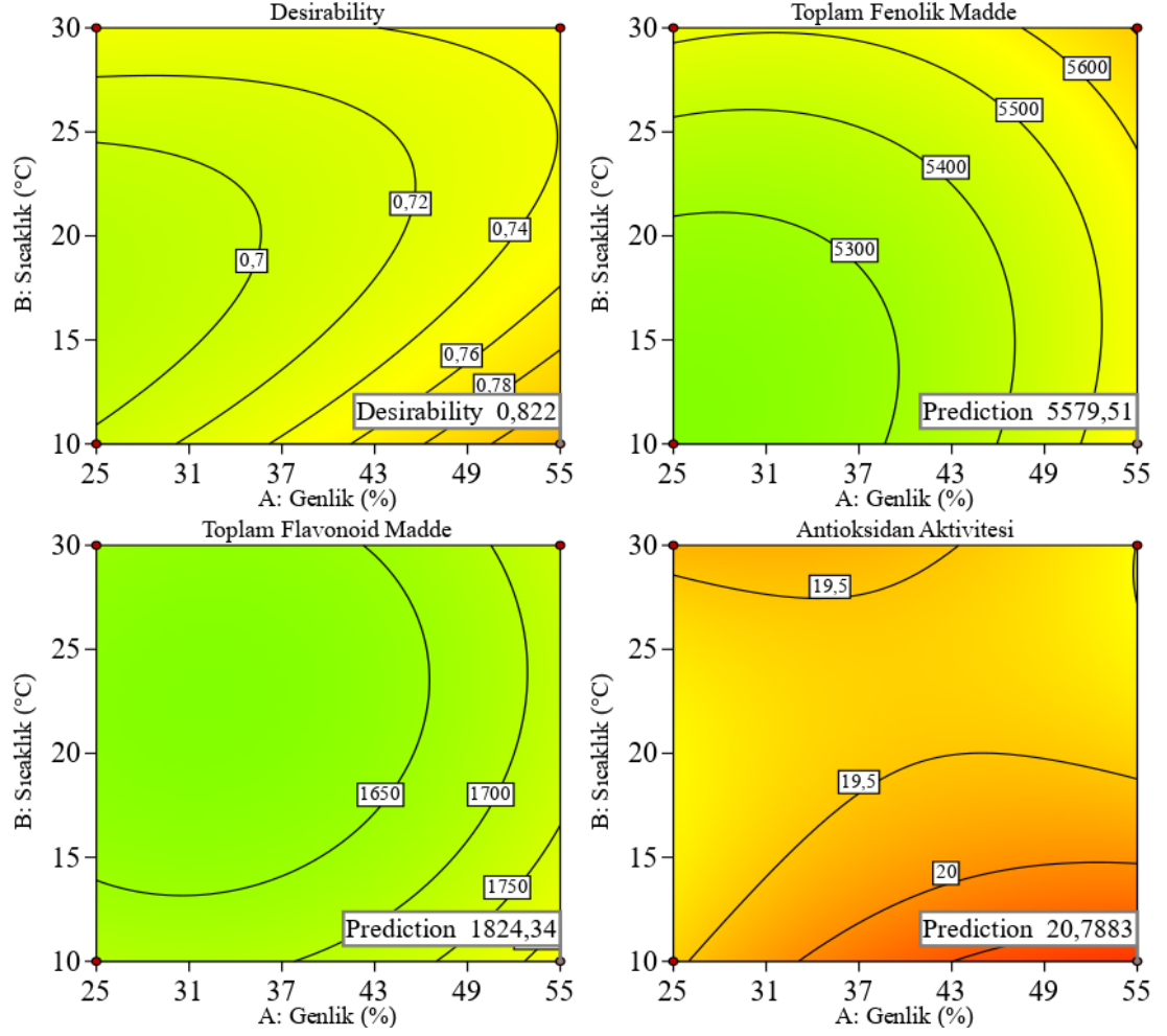
Şekil 4.26. Optimum koşullarda sıcaklık ve genlik faktör etkileşiminin toplam fenolik madde miktarı, toplam flavonoid madde miktarı ve antioksidan aktivitesi üzerine etkisi ile istenebilirlik değerleri arasındaki ilişkiyi gösteren izohips grafikleri
