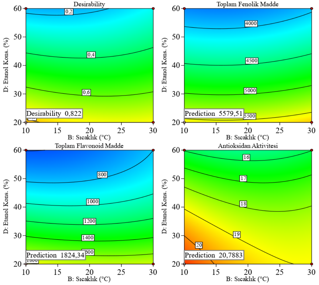
Şekil 4.30. Optimum koşullarda etanol konsantrasyonu ve sıcaklık faktör etkileşiminin toplam fenolik madde miktarı, toplam flavonoid madde miktarı ve antioksidan aktivitesi üzerine etkisi ile istenebilirlik değerleri arasındaki ilişkiyi gösteren izohips grafikleri
