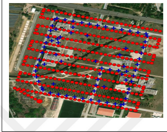
Şekil 4.23: Pix4D Mapper YKN noktaları
