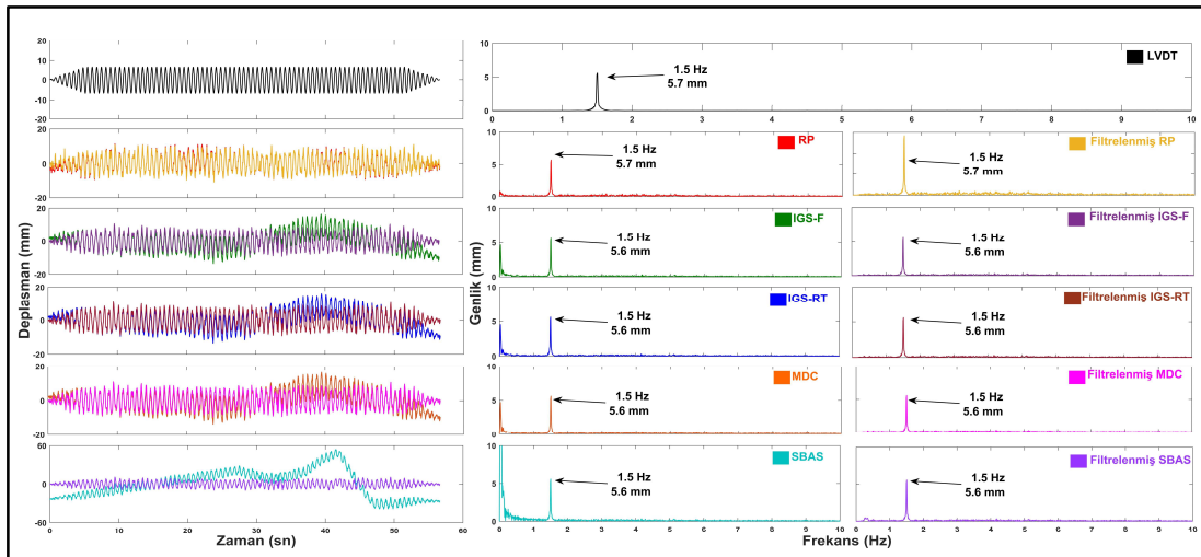
Şekil 7.13: Durum 11 için deplasman zaman serisi (sol) ve FFT spektrumu (sağ).
