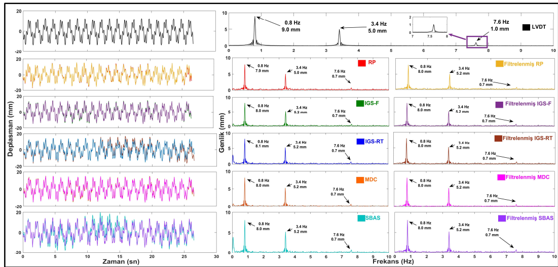
Şekil 7.14: Durum 17 için deplasman zaman serisi (sol) ve FFT spektrumu (sağ).
