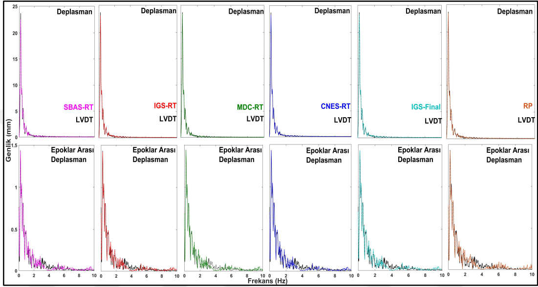
Şekil 7.8: Düzce depremi için çalışmada tartışılan tüm sensörlerden elde edilen deplasman ve epoklar arası deplasman zaman serilerinin FFT spektrumları.
