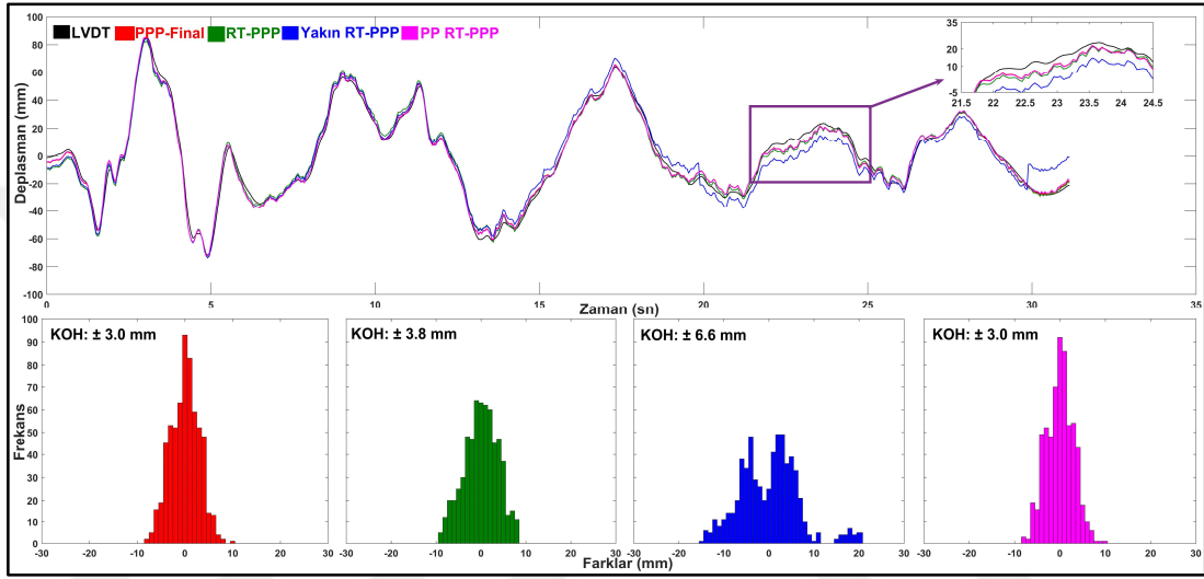
Şekil 7.50: El Centro depremi simülasyonunun neden olduğu deplasman zaman serileri (üst) ve LVDT ile PPP-tabanlı yöntemler arasındaki farkların histogramları ve KOH değerleri (alt).
