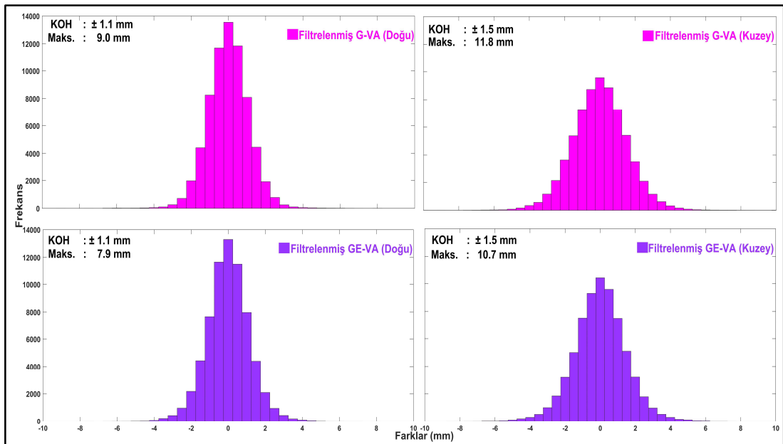
Şekil 7.27: Filtrelenmiş RP ve VA arasındaki deplasman farklarının histogramları.
