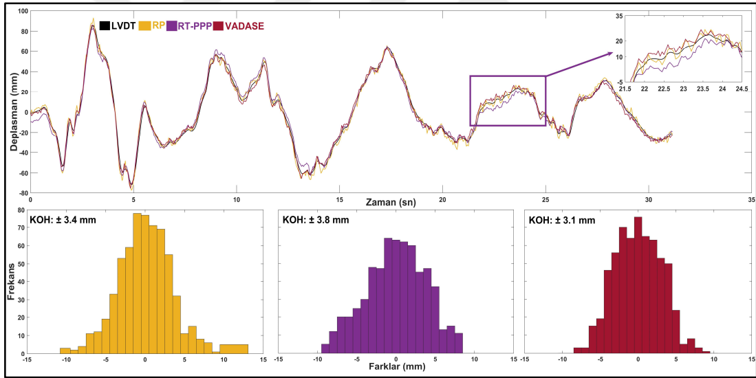
Şekil 7.40: El Centro deprem simülasyonunda LVDT, RP, RT-PPP ve VADASE'den türetilen deplasmanların karşılaştırılması (üst) ve GPS-tabanlı deplasmanlar ile LVDT arasındaki farkların histogramları (alt).
