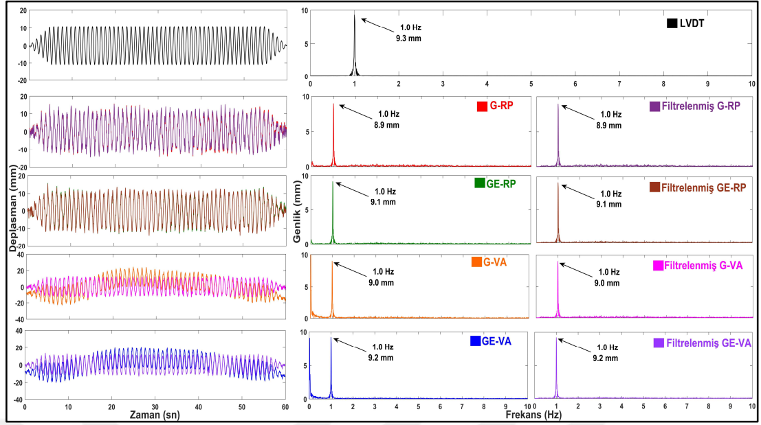
Şekil 7.28: Durum 4 için deplasman zaman serisi (sol) ve FFT spektrumu (sağ).
