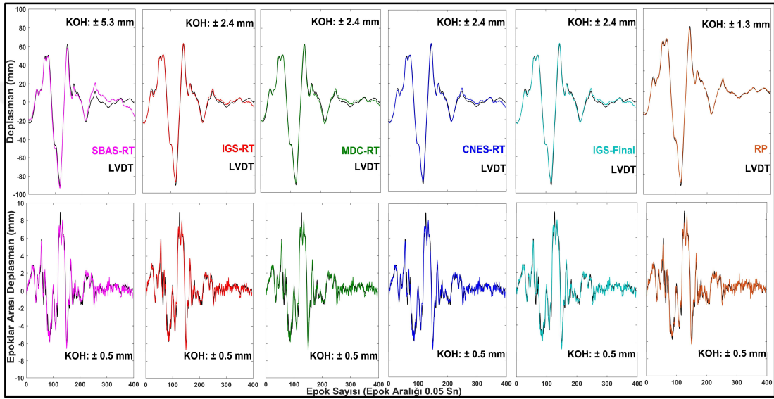
Şekil 7.7: Düzce depremi için tüm yöntemlerden elde edilen deplasman (üst) ve epoklar arası deplasman (alt) zaman serileri ve her iki zaman alanı için tartışılan tüm yöntemler ve LVDT sensörü arasındaki KOH değerleri
