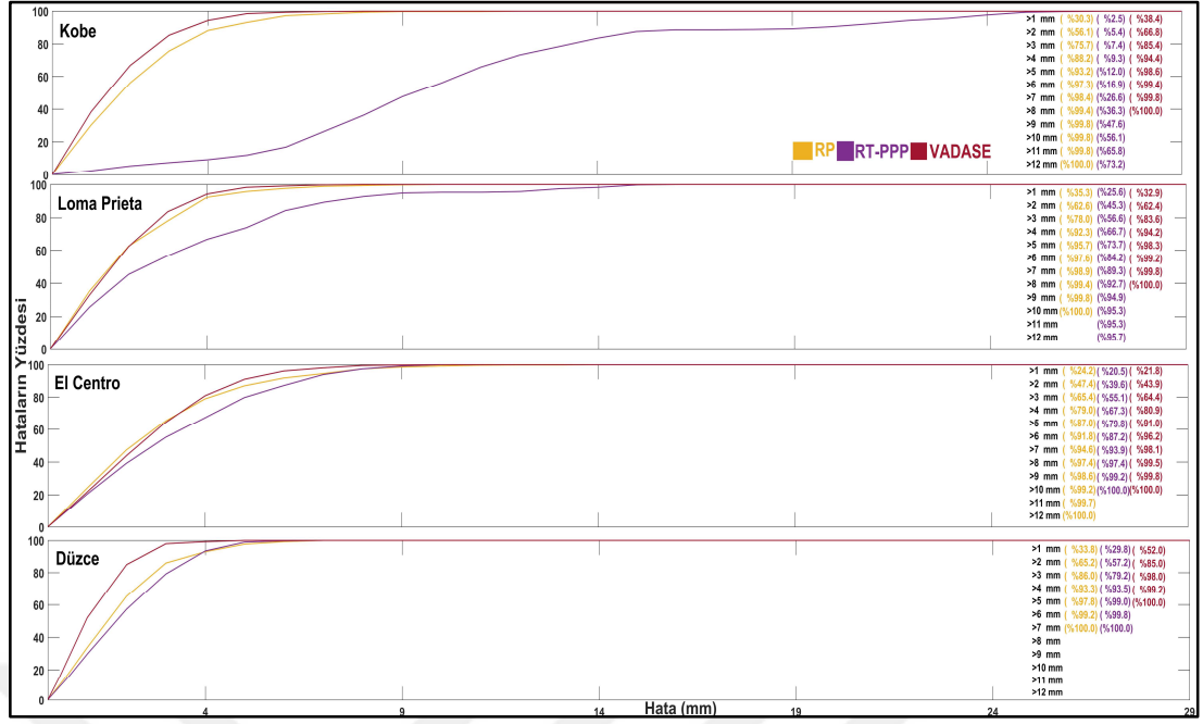
Şekil 7.42: Tüm deprem simülasyonları için GPS-tabanlı çözümlerden elde edilen deplasmanların LVDT'den olan farklarının yüzde dağılımı.
