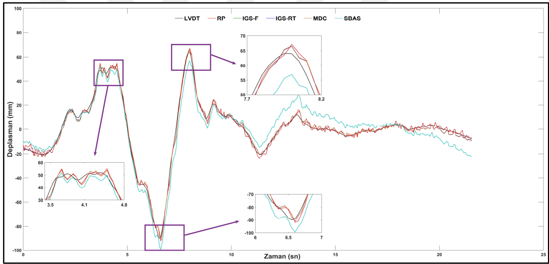
Şekil 7.17: Düzce depremi simülasyonunda farklı ürünlere dayalı SF-PPP, SF-RP ve LVDT kaynaklı yer değiştirmelerin karşılaştırılması.
