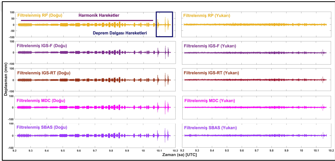
Şekil 7.12: Filtrenmiş SF-RP ve SF-PPP den türetilen deplasmanlar.
