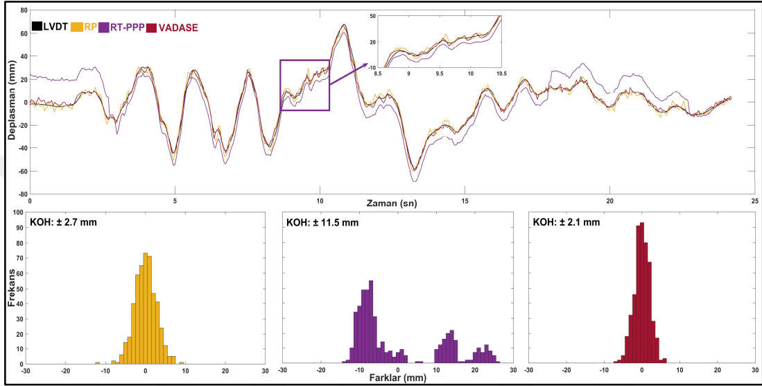
Şekil 7.38: Kobe deprem simülasyonunda LVDT, RP, RT-PPP ve VADASE'den türetilen deplasmanların karşılaştırılması (üst) ve GPS-tabanlı deplasmanlar ile LVDT arasındaki farkların histogramları (alt).
