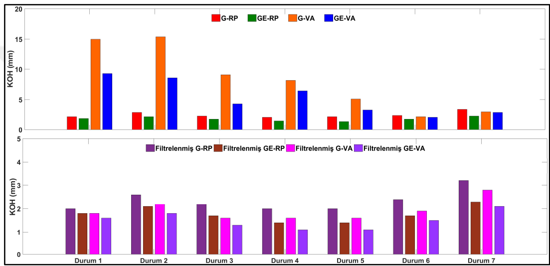
Şekil 7.30: Tüm durumlar için RP, VA ve LVDT arasındaki deplasman farklarının KOH değerleri.
