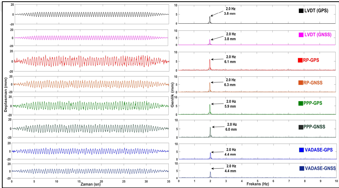
Şekil 7.54: Örnek durum zaman serileri (sol) ve FFT spektrumları (sağ).
