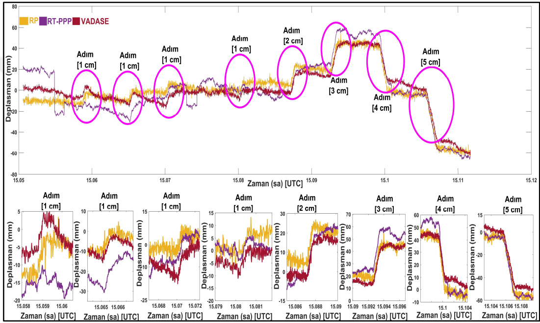
Şekil 7.43: Adım fonksiyonu deneylerinde RP-, RT-PPP- ve VADASE-den türetilen deplasmanların karşılaştırılması.
