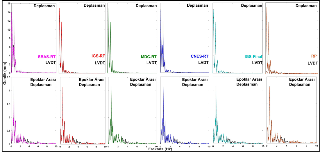
Şekil 7.10: Kobe depremi için çalışmada tartışılan tüm sensörlerden elde edilen deplasman ve epoklar arası deplasman zaman serilerinin FFT spektrumları.
