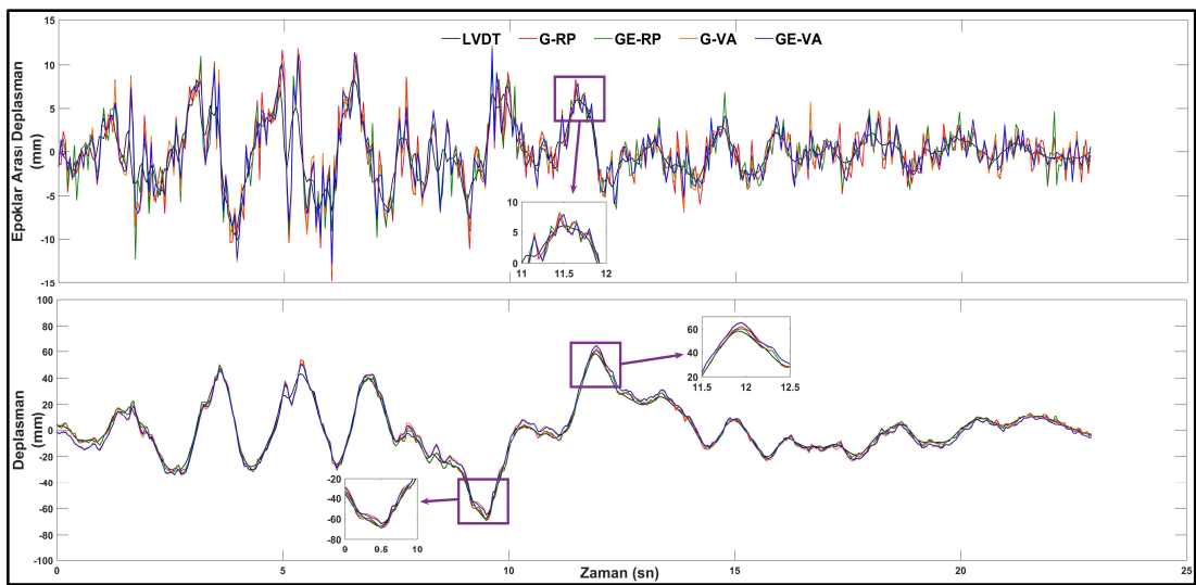
Şekil 7.32: Kobe depremi simülasyonundan elde edilen RP, VA ve LVDT sensörlerine ait epoklar arası deplasman ve deplasman zaman serilerinin karşılaştırılması.
