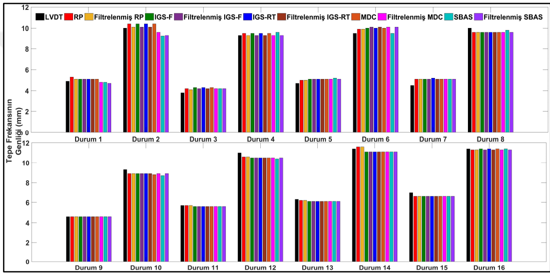
Şekil 7.15: Deplasman değerlerinden elde edilen tepe frekansına karşılık gelen genlik değerleri
