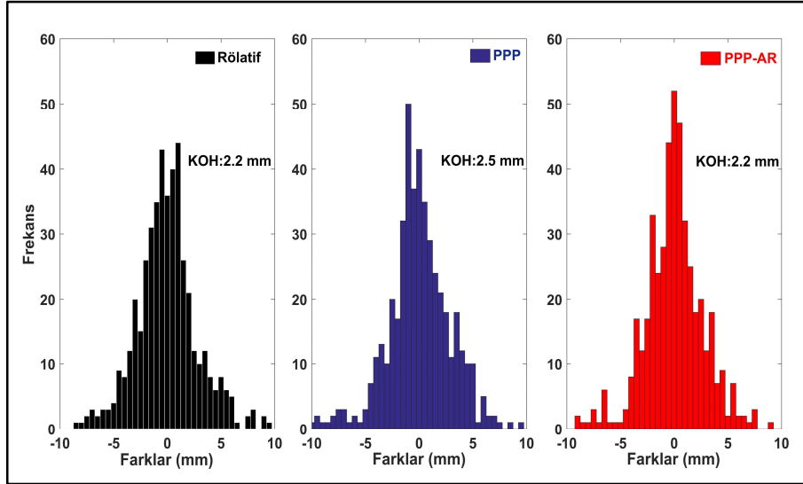
Şekil 7.64: Kobe deprem simülasyonu için LVDT ve GNSS tabanlı yöntemler arasındaki deplasman farklarının histogramları.
