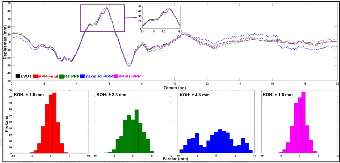
Şekil 7.51: Düzce depremi simülasyonunun neden olduğu deplasman zaman serileri (üst) ve LVDT ile PPP-tabanlı yöntemler arasındaki farkların histogramları ve KOH değerleri (alt).
