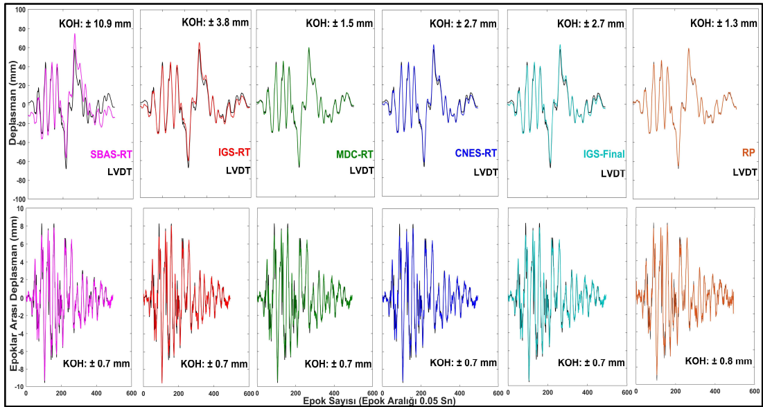
Şekil 7.9: Kobe depremi için tüm yöntemlerden elde edilen deplasman (üst) ve epoklar arası deplasman (alt) zaman serileri ve her iki zaman alanı için tartışılan tüm yöntemler ve LVDT sensörü arasındaki KOH değerleri
