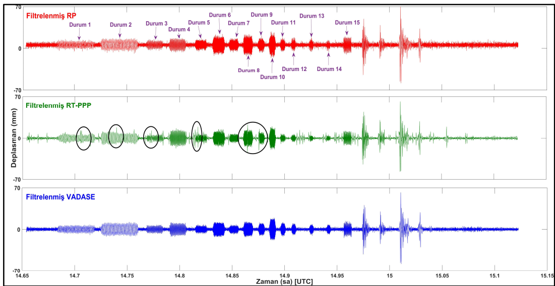
Şekil 7.35: Tüm GPS tabanlı yaklaşımların filtrelenmiş deplasman zaman serileri.
