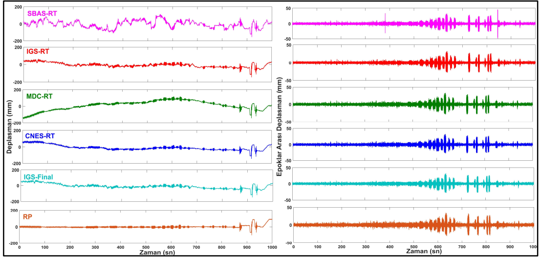
Şekil 7.1: Tüm GPS tabanlı yöntemlerden türetilen deplasman (sol) ve epoklar arası deplasman zaman serileri (sağ).
