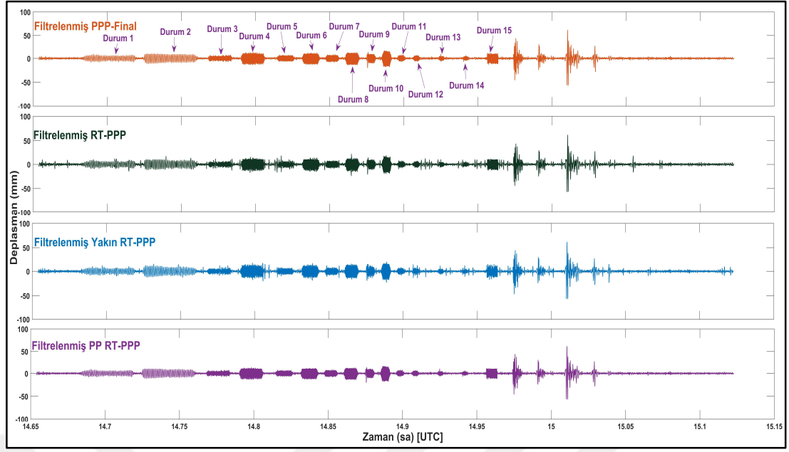
Şekil 7.45: PPP-Final, RT-PPP, Yakın RT-PPP ve PP RT-PPP'den türetilen filtrelenmiş deplasman zaman serileri.
