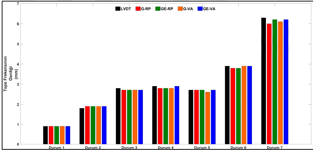
Şekil 7.22: Tüm durumlar için tepe frekansına karşılık gelen genlik değerleri.
