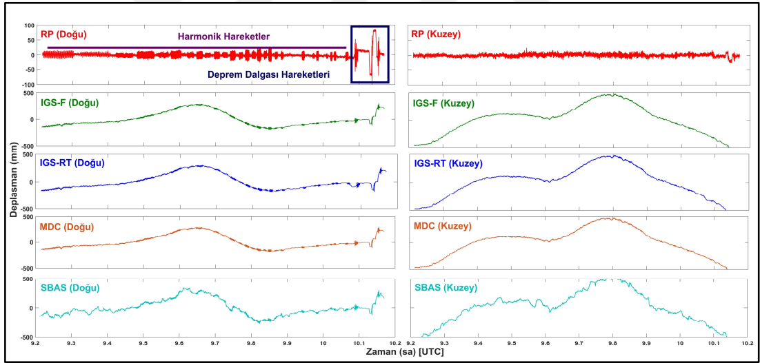
Şekil 7.11: SF-RP- (kırmızı), IGS Final tabanlı SF-PPP- (yeşil), IGS-RT tabanlı SF-PPP- (lacivert), MDC tabanlı SF-PPP- (turuncu) ve İkinci-Nesil destekli SF-PPP- (gökyüzü- mavisi)-den elde edilen deplasmanlar.
