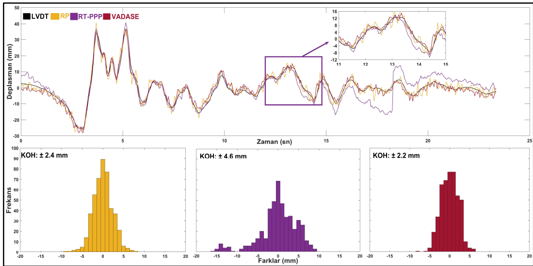
Şekil 7.39: Loma Prieta deprem simülasyonunda LVDT, RP, RT-PPP ve VADASE'den türetilen deplasmanların karşılaştırılması (üst) ve GPS-tabanlı deplasmanlar ile LVDT arasındaki farkların histogramları (alt).
