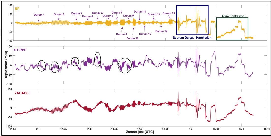
Şekil 7.34: Çalışmada tasarlanan tüm deneyler için RP- (üst panel), RT-PPP- (üstten ikinci panel) ve VADASE- (üstten üçüncü panel) den elde edilen deplasmanlar.
