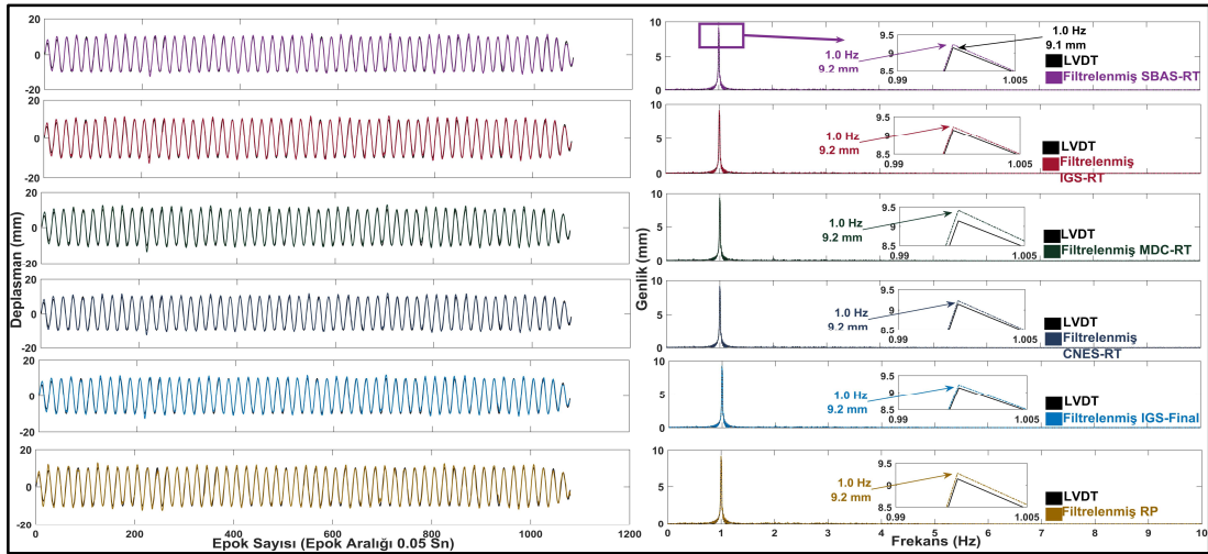
Şekil 7.5: Dördüncü durum için GPS tabanlı yöntemlerden elde edilen filtrelenmiş deplasman zaman serileri (sol) ve FFT spektrumları (sağ).
