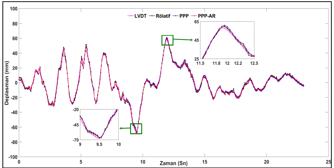
Şekil 7.63: Kobe deprem simülasyonunda geleneksel-PPP, PPP-AR, rölatif konum belirleme ve LVDT'den türetilen deplasmanların karşılaştırılması.
