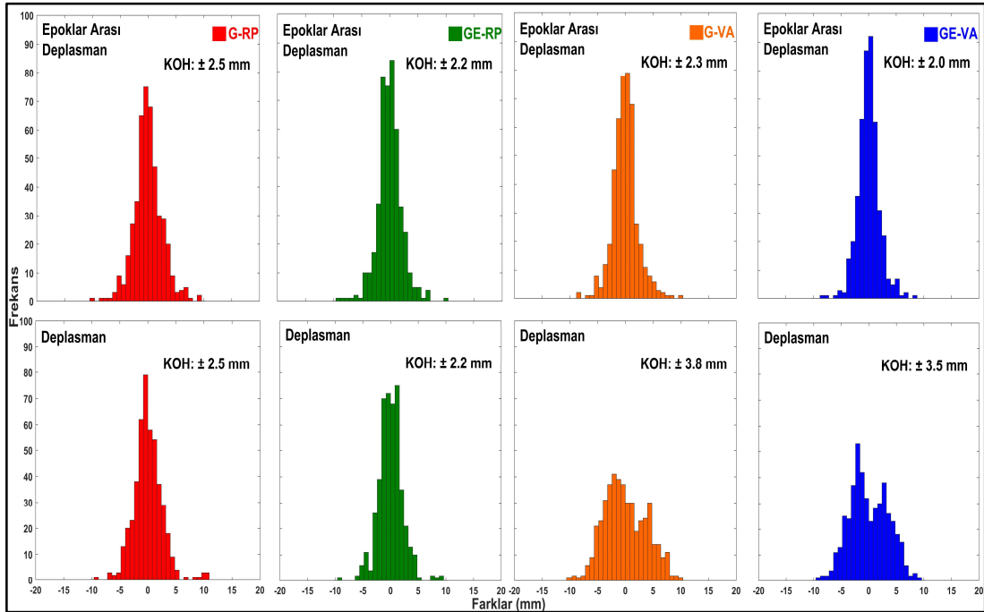
Şekil 7.33: Kobe deprem simülasyonu için LVDT ile RP ve VA sensörleri arasındaki epoklar arası deplasman ve deplasman farklarının histogramları.
