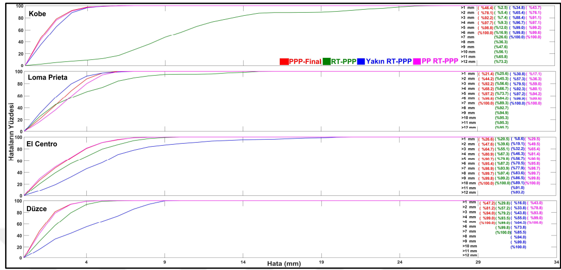
Şekil 7.52: Tüm deprem simülasyonları için PPP tabanlı yaklaşımlarından elde edilen deplasmanların LVDT'den olan farklarının yüzde dağılımı.
