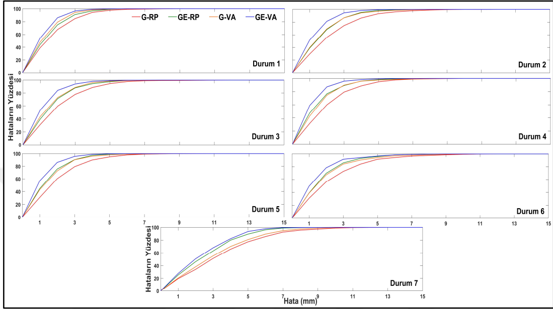
Şekil 7.24: Tüm durumlar için KOH değerleri.
