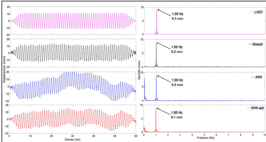
Şekil 7.60: Durum 5 için LVDT, rölatif konum belirleme, geleneksel-PPP ve PPP-AR tekniklerinden elde edilen deplasman zaman serileri ve FFT spektrumları.
