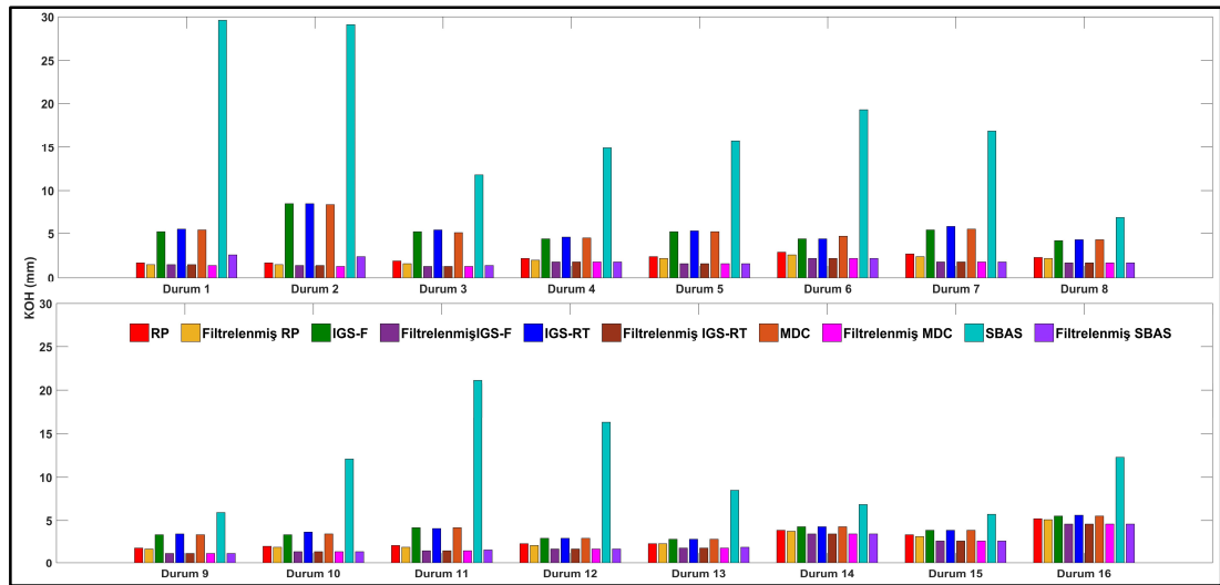
Şekil 7.16: Tüm durumlar için KOH değerleri.
