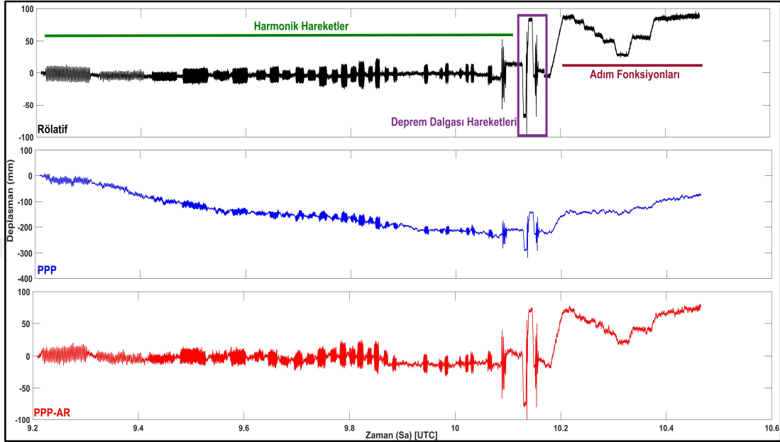
Şekil 7.58: Rölatif konum belirleme, geleneksel-PPP ve PPP-AR tekniklerinden elde edilen deplasmanlar.
