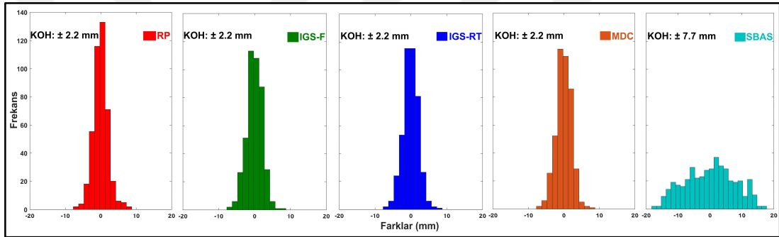
Şekil 7.18: Düzce deprem simülasyonu için LVDT ile SF-RP (kırmızı), IGS-Final tabanlı SF-PPP (yeşil), IGS-RT tabanlı SF-PPP (lacivert), MDC tabanlı SF-PPP (turuncu) ve SBAS tabanlı SF-PPP (gök mavisi) yöntemleri arasındaki farkların histogramları.
