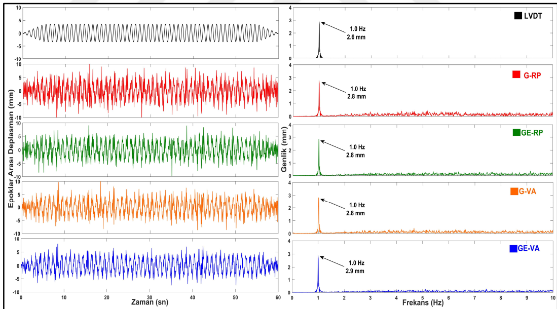
Şekil 7.21: Durum 4 için LVDT, RP ve VA çözümlerinin epoklar arası deplasman zaman serisi (sol) ve FFT spektrumu (sağ).
