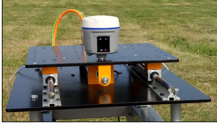
Şekil 6.2: 1 nolu deney anından bir görünüm.
