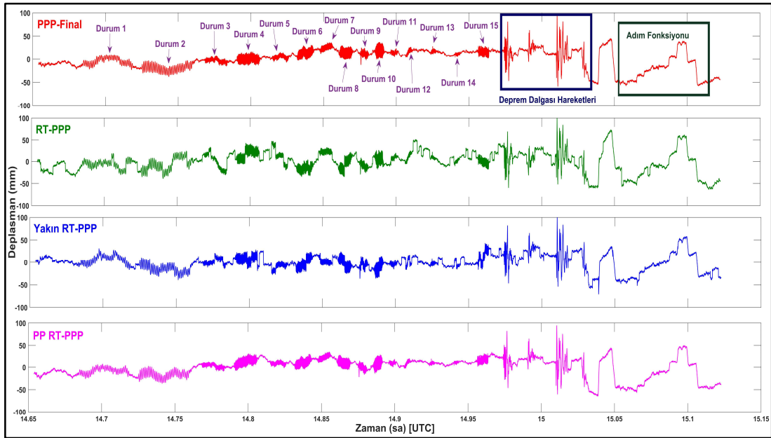
Şekil 7.44: PPP-Final, RT-PPP, Yakın RT-PPP ve PP RT-PPP'den türetilen deplasman zaman serileri.
