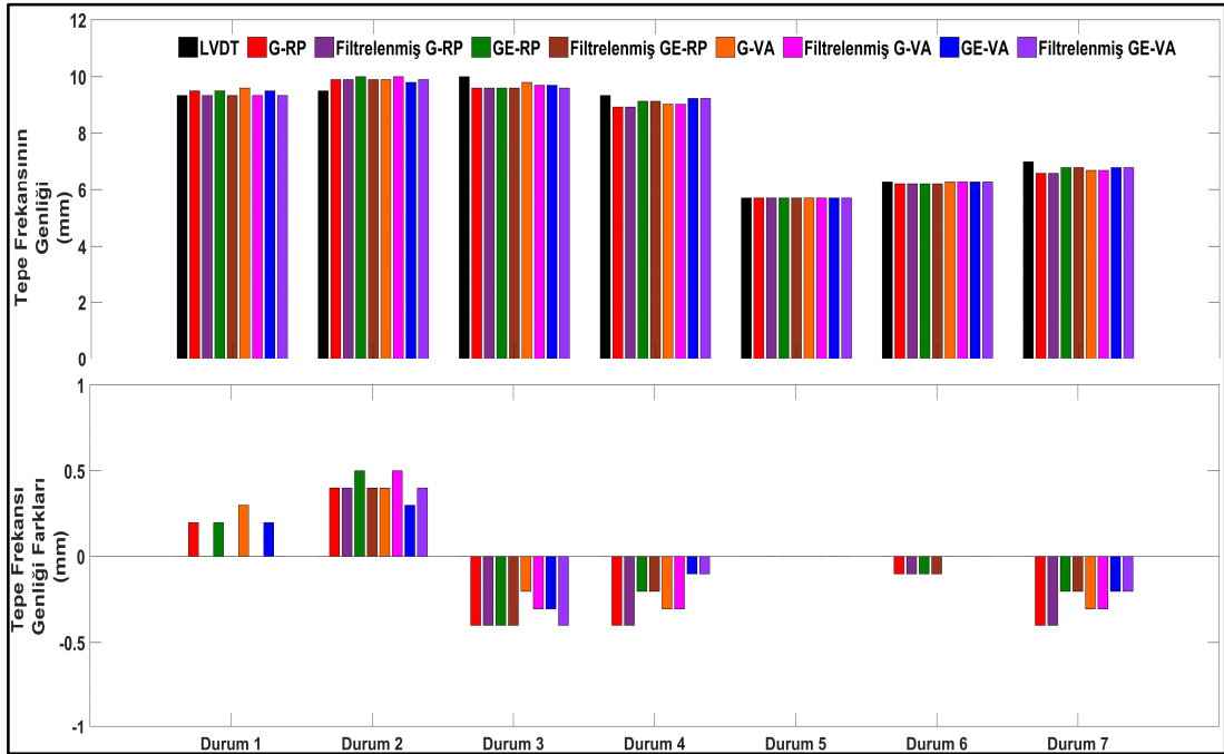
Şekil 7.29: Tepe frekansına deplasman genliği ve LVDT ile filtrelenmemiş/filtrelenmemiş sonuçlar arasındaki farklar.
