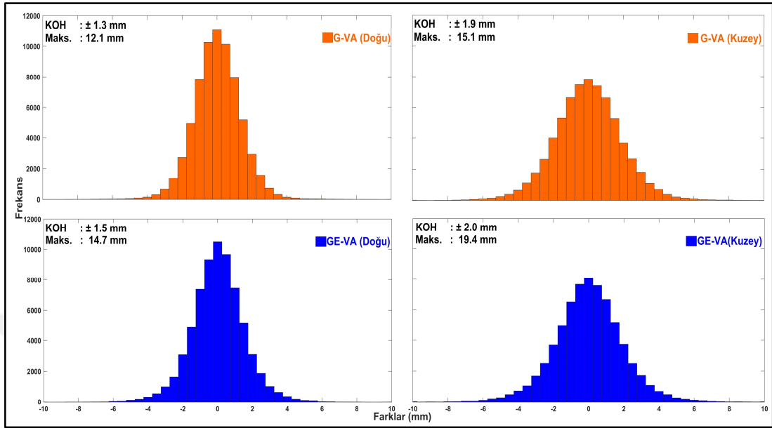
Şekil 7.20: RP ve VA teknikleri arasındaki farkların histogramı.
