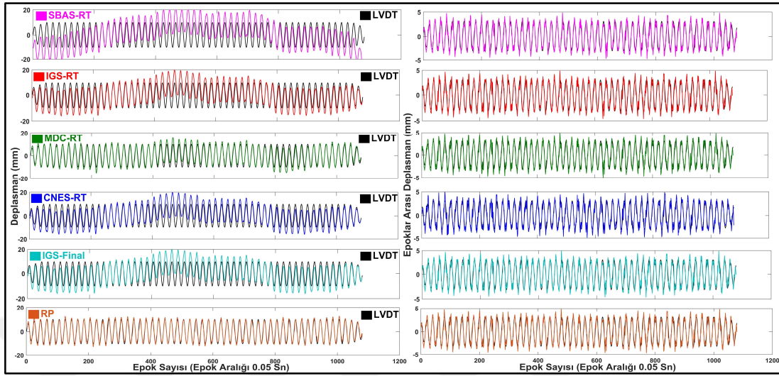
Şekil 7.3: Dördüncü durum için tüm GPS tabanlı yöntemlerden türetilen deplasman ve epoklar arası deplasman zaman serileri.
