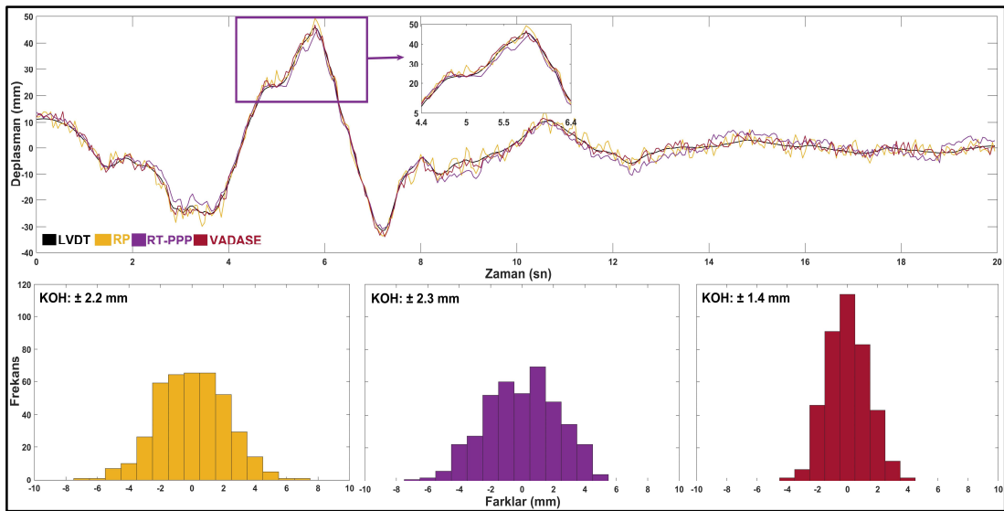
Şekil 7.41: Düzce deprem simülasyonunda LVDT, RP, RT-PPP ve VADASE'den türetilen deplasmanların karşılaştırılması (üst) ve GPS-tabanlı deplasmanlar ile LVDT arasındaki farkların histogramları (alt).
