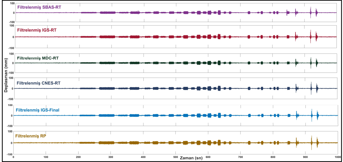
Şekil 7.2: Tüm GPS tabanlı yöntemlerden türetilen filtrelenmiş deplasman zaman serileri.
