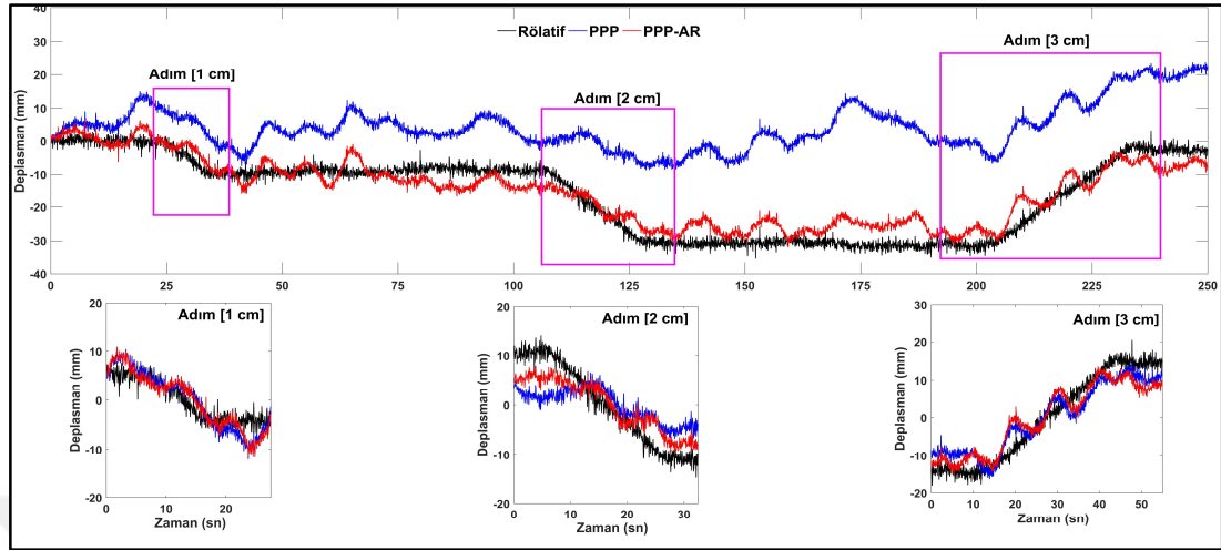
Şekil 7.65: Adım fonksiyon testlerinde rölatif konum belirleme, geleneksel-PPP ve PPP AR tekniklerinden türetilen deplasmanların karşılaştırılması.
