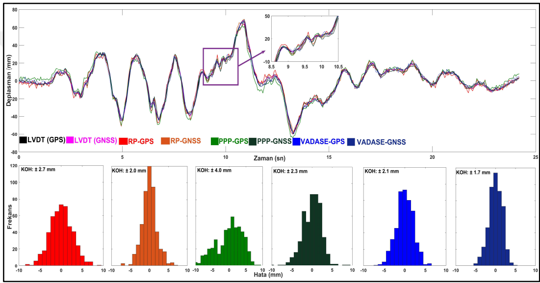
Şekil 7.56: Kobe depremi simülasyondan elde edilen zaman serileri (üst) ve LVDT ile GNSS sensörleri arasındaki hataların histogram ve KOH değerleri (alt).
