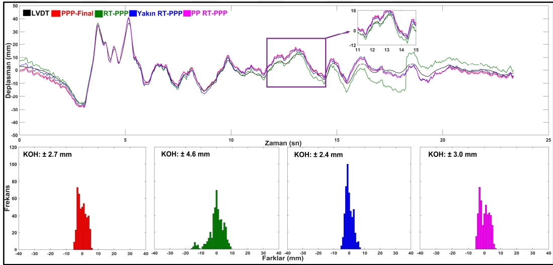
Şekil 7.49: Loma Prieta depremi simülasyonunun neden olduğu deplasman zaman serileri (üst) ve LVDT ile PPP-tabanlı yöntemler arasındaki farkların histogramları ve KOH değerleri (alt).
