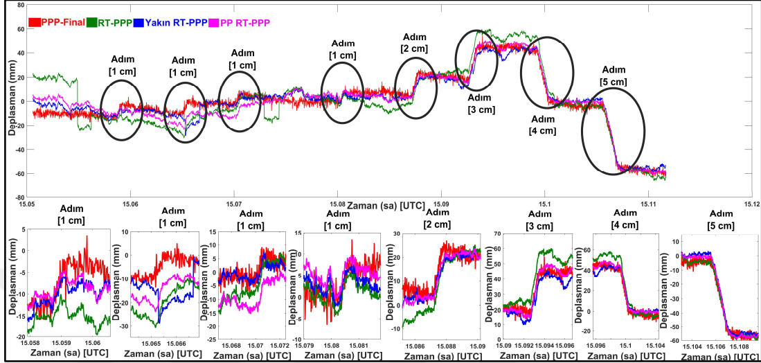
Şekil 7.53: Adım fonksiyonu deneylerinde PPP-Final, RT-PPP, Yakın RT-PPP ve PP RT-PPP'den türetilen kalıcı deplasmanların karşılaştırılması.
