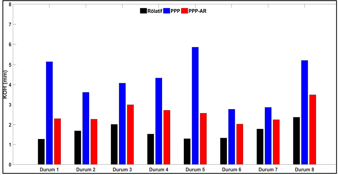
Şekil 7.62: Tüm durumlar için LVDT ve GNSS tabanlı yöntemlerin farkları arasındaki KOH değerleri.
