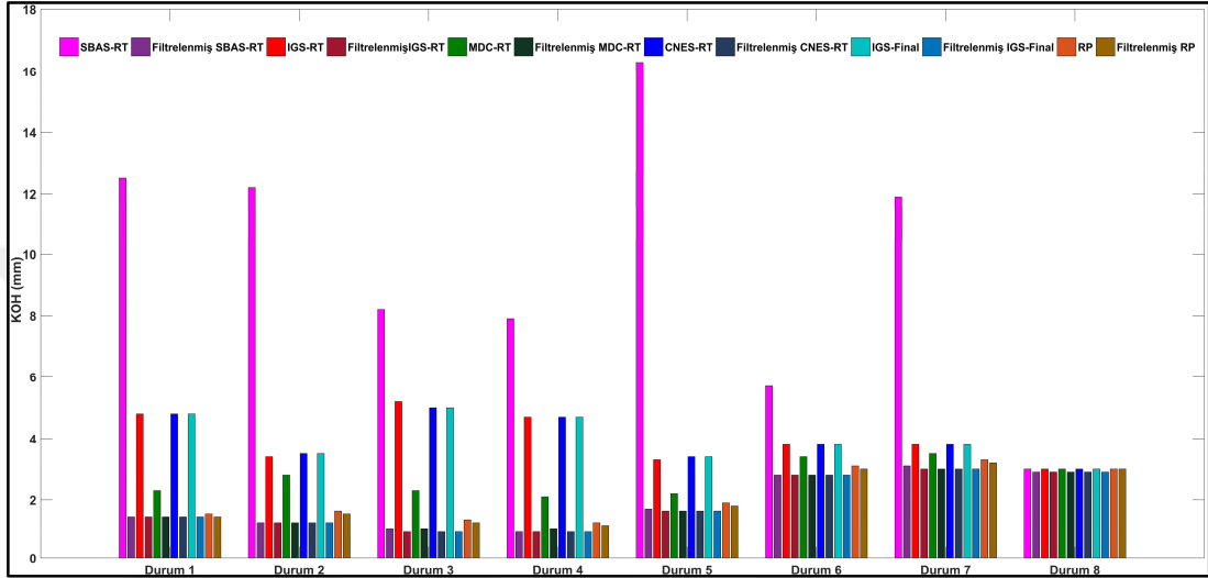
Şekil 7.6: Filtrelenmiş ve filtrelenmemiş sonuçlar için deplasman alanında GPS tabanlı yöntemler ve LVDT arasındaki farkların KOH değerleri.
