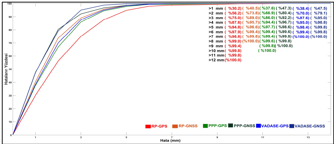
Şekil 7.57: Kobe depremi için LVDT ile GNSS sensörleri arasındaki hataların yüzdesel dağılımı.
