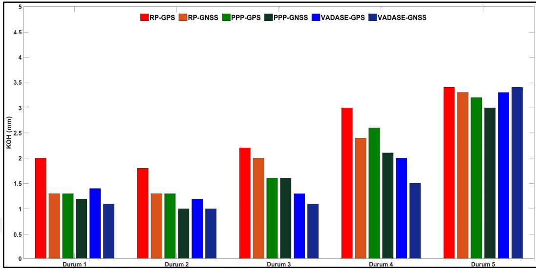
Şekil 7.55: Tüm durumlar için GNSS tabanlı yöntemler ve LVDT arasındaki farkların KOH değerleri.
