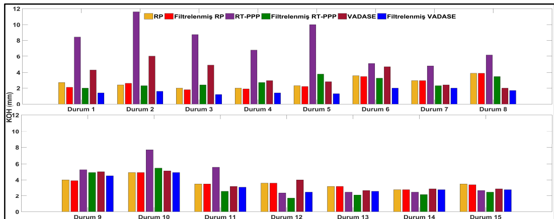
Şekil 7.37: GPS-tabanlı teknikler ve LVDT arasındaki deplasman farklarının KOH değerleri.
