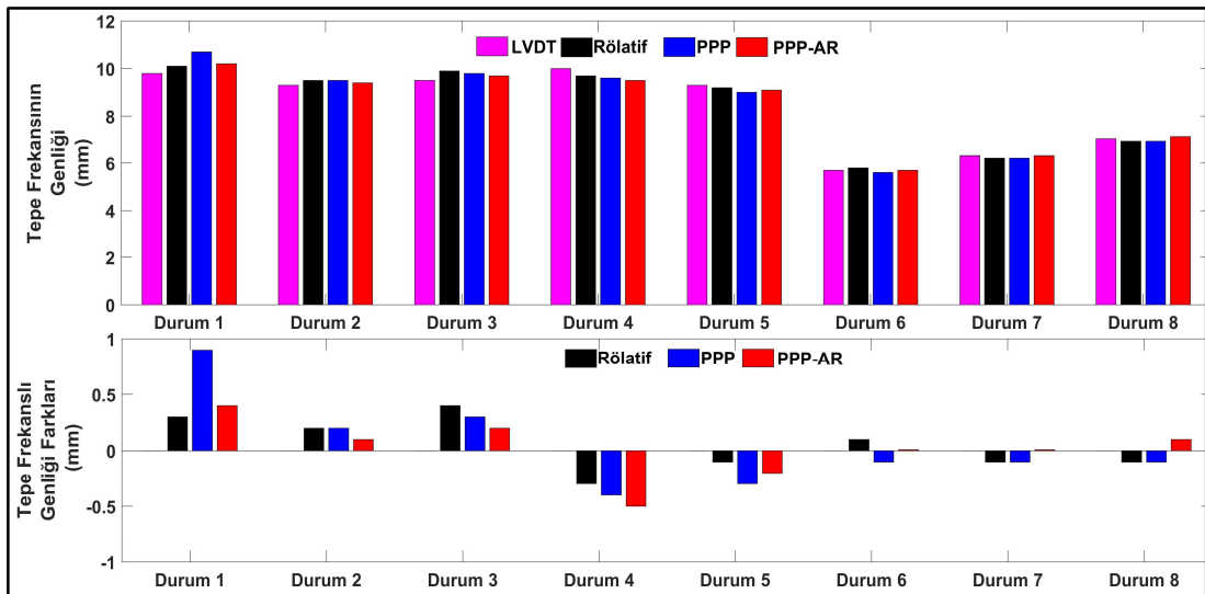
Şekil 7.61: LVDT ve GNSS çözümleri için FFT spektrumlarından elde edilen tepe frekanslarının genliği ve LVDT ile GNSS tabanlı yöntemler arasındaki farklılıklar.
