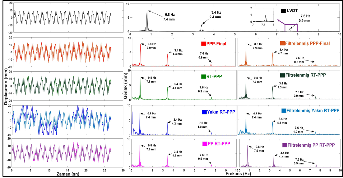
Şekil 7.46: Durum 15 için LVDT, filtrelenmemiş ve filtrelenmiş RT-PPP tabanlı yaklaşımlardan elde edilen deplasman zaman serileri ve FFT spektrumları.
