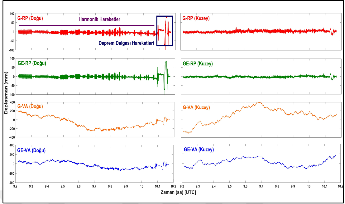
Şekil 7.25: VA ve RP'den türetilmiş deplasmanlar.
