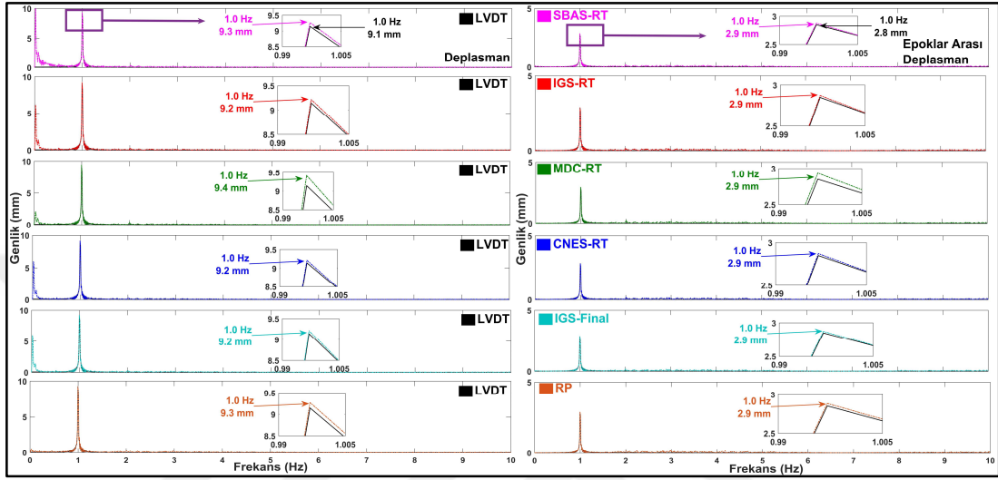
Şekil 7.4: Dördüncü durum için tüm GPS tabanlı yöntemlerden elde edilen deplasman ve epoklar arası deplasman FFT spektrumları.
