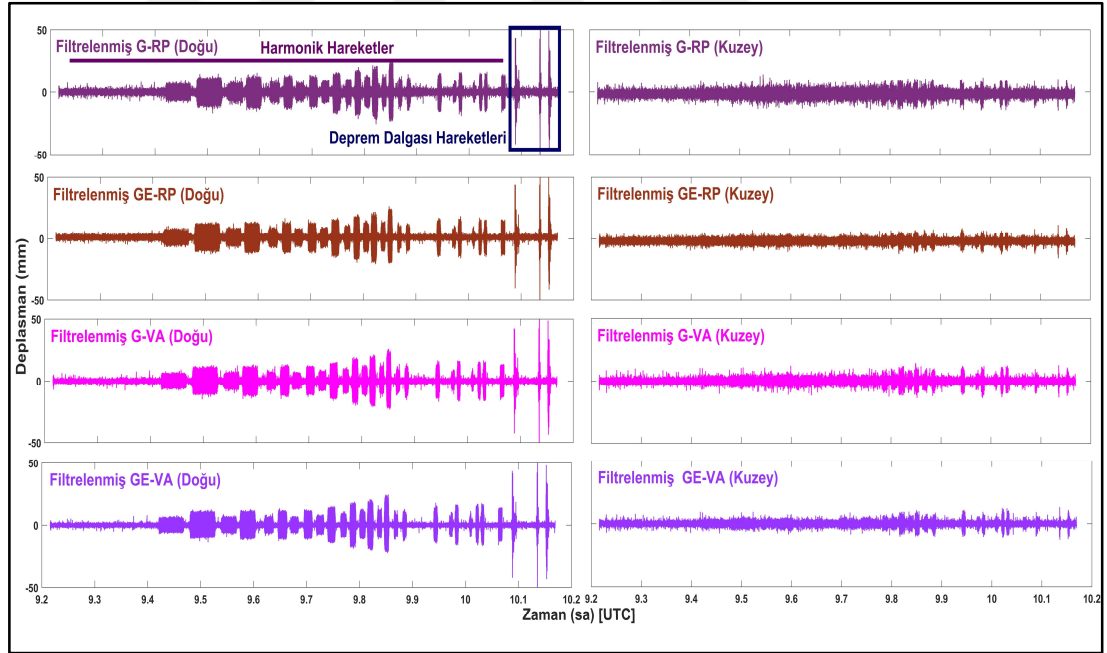
Şekil 7.26: VA ve RP'den türetilmiş ve filtrelenmiş deplasmanlar.
