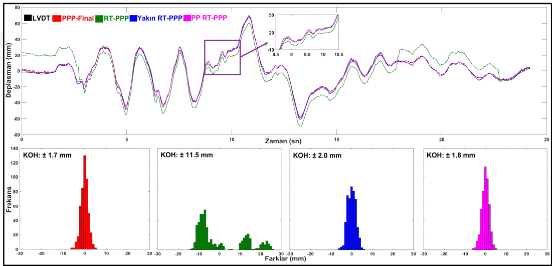
Şekil 7.48: Kobe depremi simülasyonunun neden olduğu deplasman zaman serileri (üst) ve LVDT ile PPP-tabanlı yöntemler arasındaki farkların histogramları ve KOH değerleri (alt).
