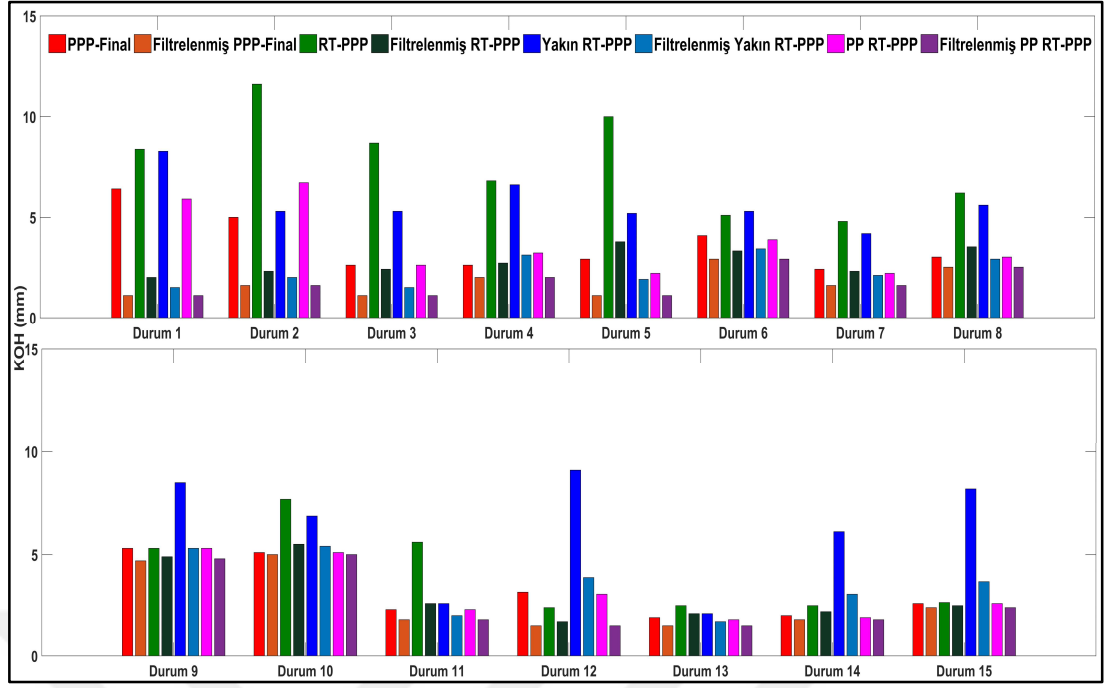
Şekil 7.47: Tüm durumlardan elde edilen LVDT ve PPP tabanlı yaklaşımlar arasındaki farkların KOH değerleri.
