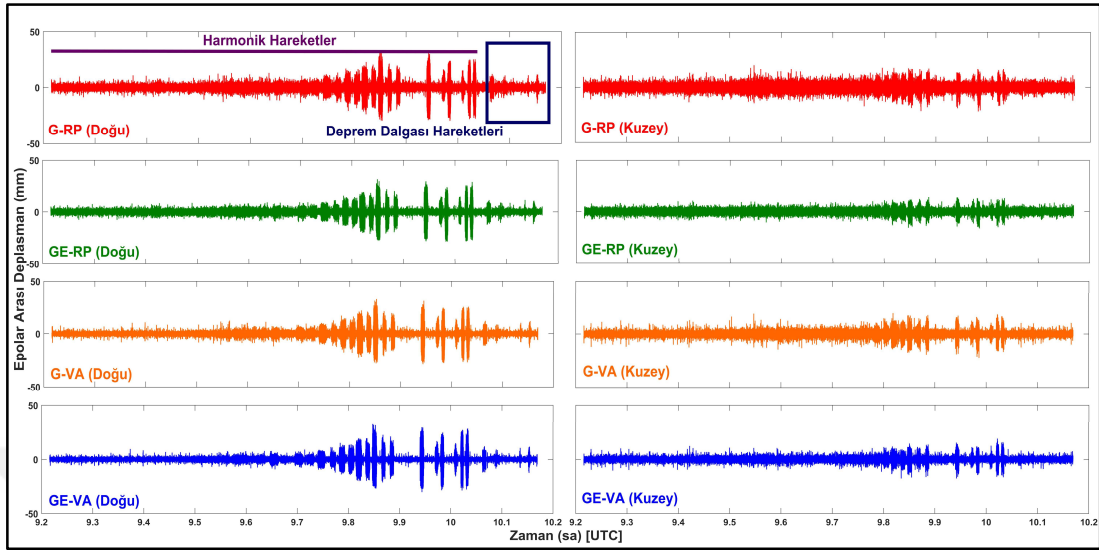
Şekil 7.19: RP ve VA tekniklerinden elde edilen epoklar arası deplasman değerleri.
