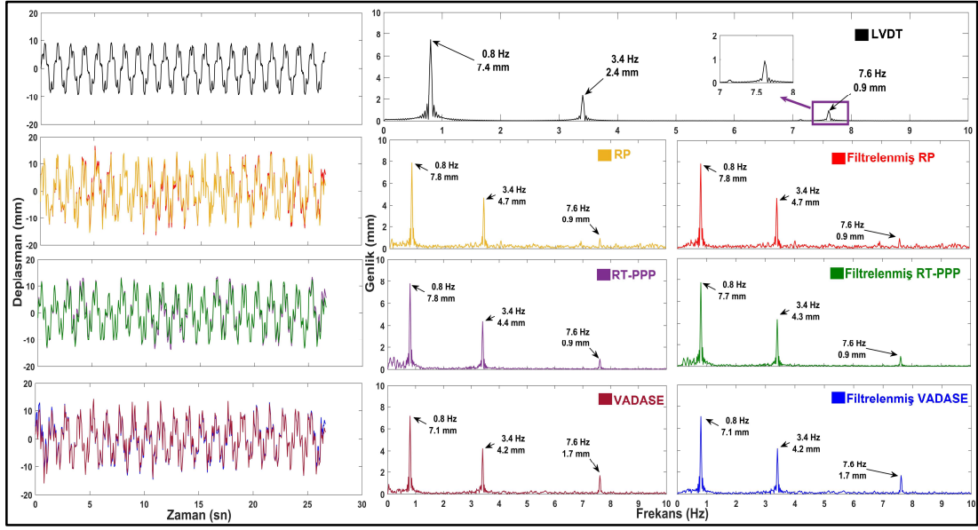
Şekil 7.36: Durum 15 için deplasman zaman serisi (sol) ve FFT spektrumu (sağ).
