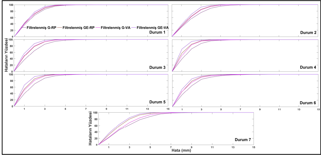
Şekil 7.31: Tüm durumlar için RP, VA ve LVDT arasındaki deplasman farkı hatalarının yüzde dağılımı.
