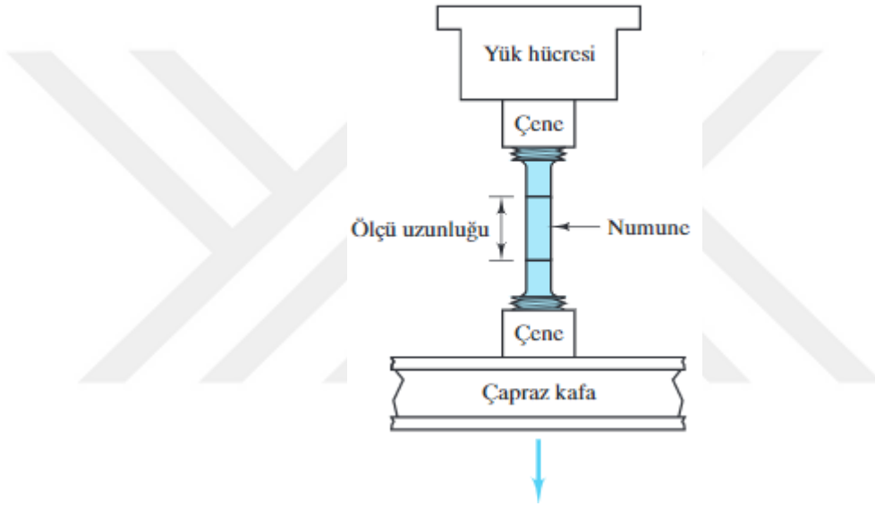
Şekil 3.10. Çekme deney düzeneği [37].
