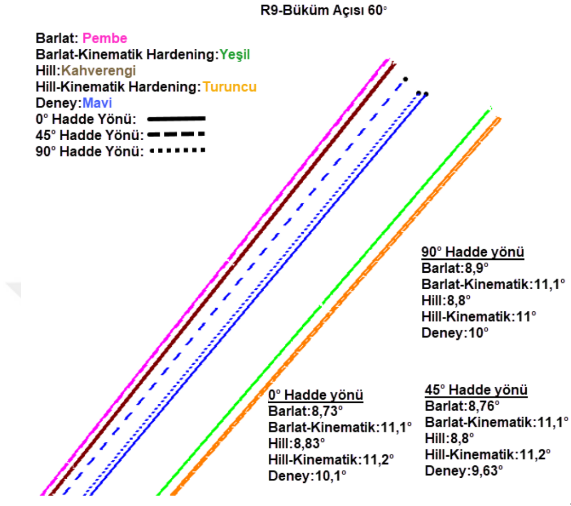
Şekil 7.23. Zımba yarıçapı R9, büküm açısı 60° olduğu durumda malzeme modellerine göre A detayının geri yaylanmaların gösterimi.
