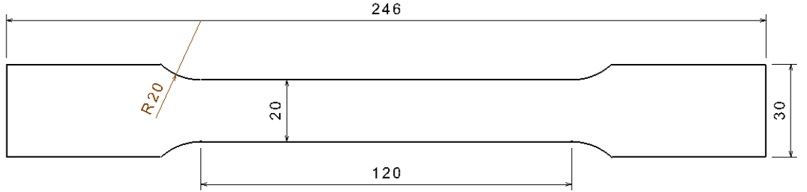
Şekil 6.1. Çekme test numune ölçüleri.
