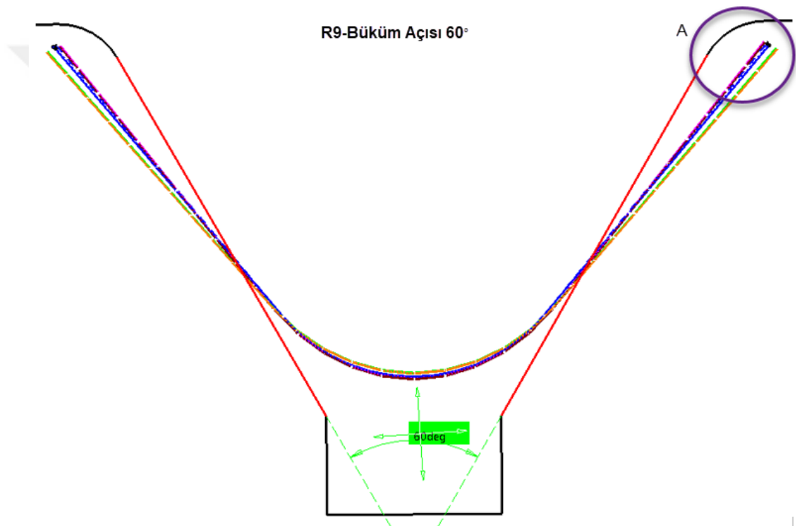
Şekil 7.22. Zimba yarıçapı R9, büküm açısı 60^\circ olduğu durumda malzeme modellerine göre geri yaylanmaların gösterimi.
