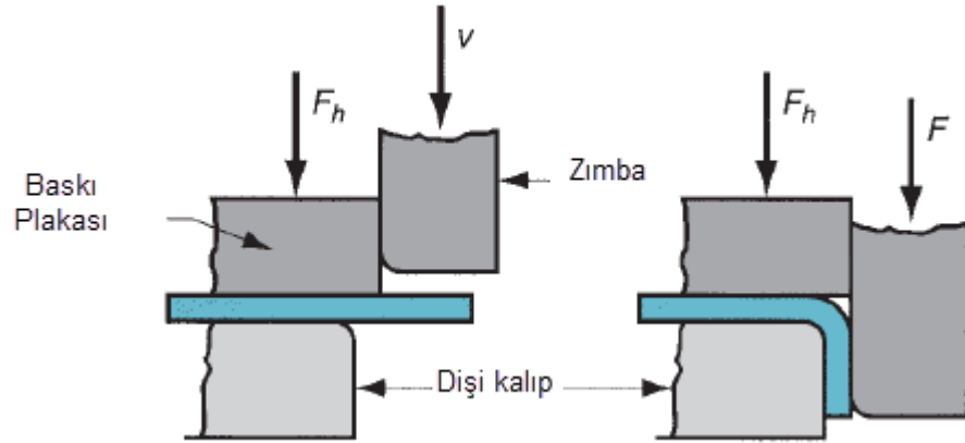
Şekil 3.6. Kenar bükme [35].
