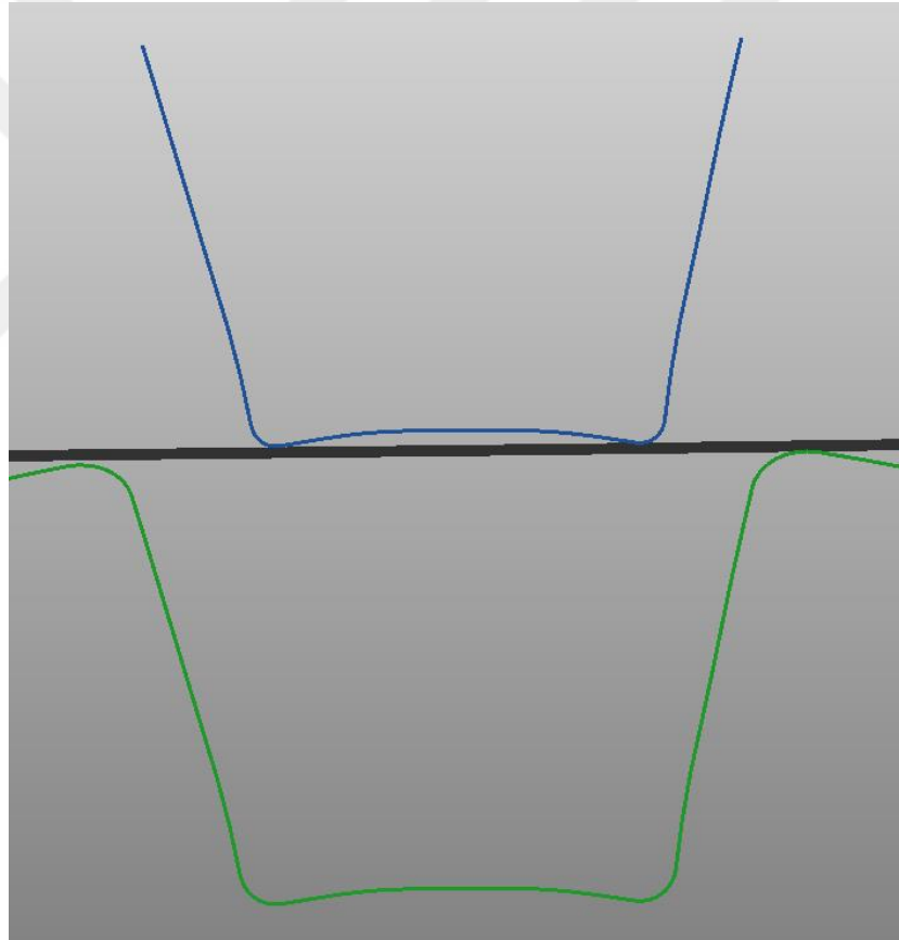
Şekil 7.44. R3 zimba yarıçapında Barlat kinematik pekleşme model telafili yüzey.
