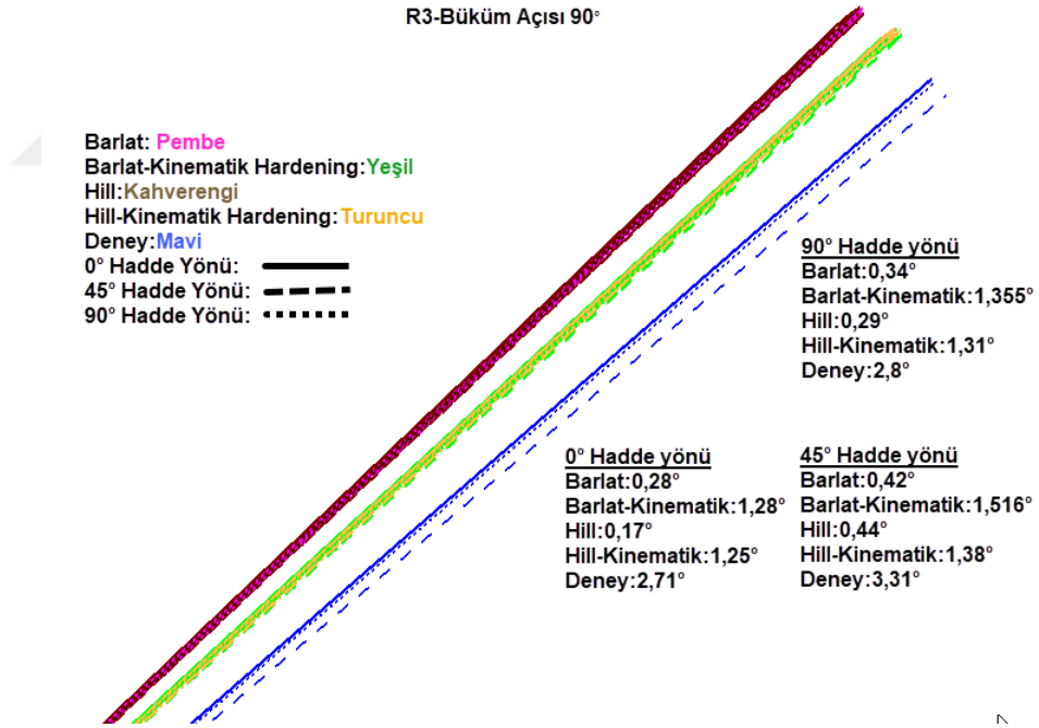
Şekil 7.13. Zımba yarıçapı R3, büküm açısı 90° olduğu durumda malzeme modellerine göre geri yaylanmaların A detay gösterimi.
