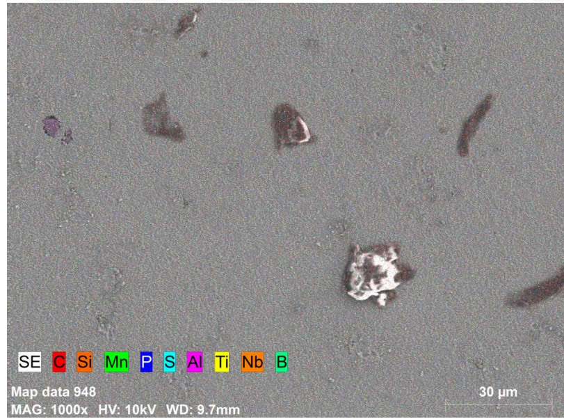
Şekil 6.10. SCGADUB1180 malzemesinin element dağılımı.
