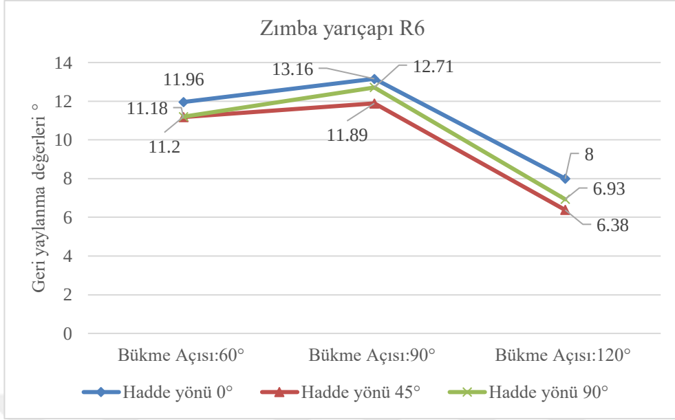
Şekil 7.3. R6 zimba yarıçapındaki geri yaylanma değerleri.
