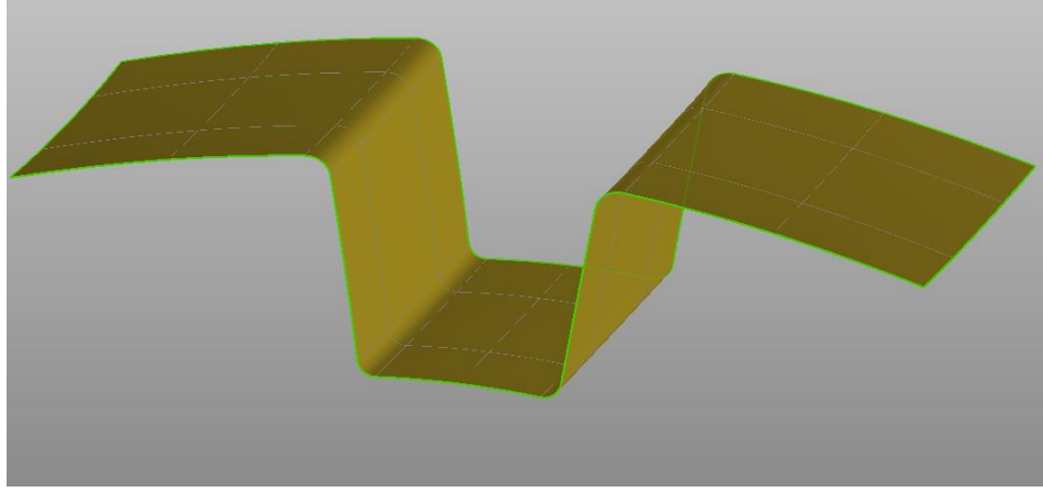
Şekil 7.44. R3 zimba yarıçapında Barlat kinematik pekleşme model telafili yüzey.
