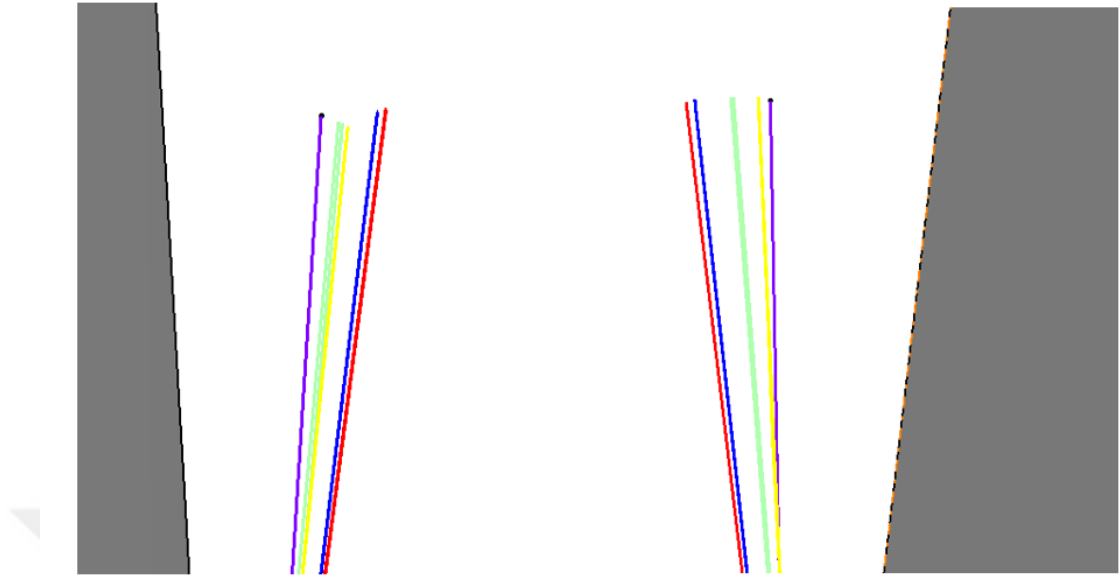
Şekil 7.29. Zımba yarıçapı R3 durumunda geri-ileri yaylanma değerlerinin gösterimi (a) Duvar açısı 93° (b) Duvar açısı 97°.
