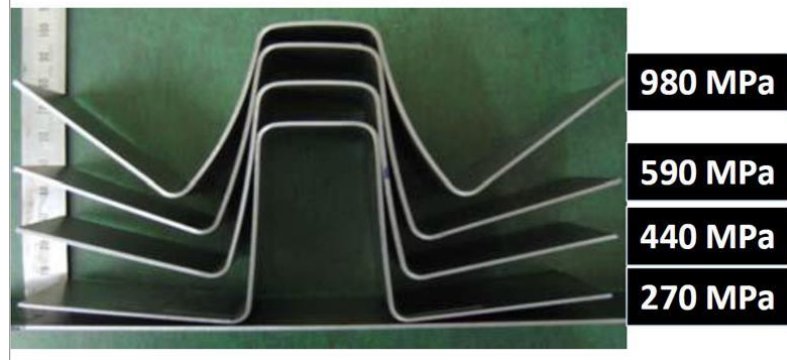
Şekil 4.2. Farklı mukavemet değerlerindeki parçaların geri yaylanma değerleri [49].
