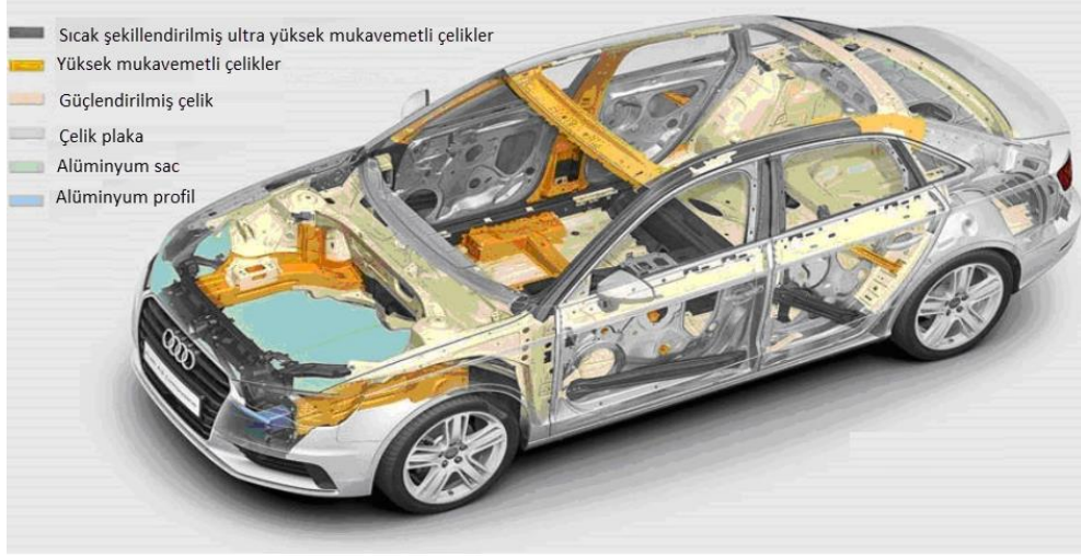
Şekil 1.2. Araçtaki metallerin kullanım yerlerinin gösterimi [6].
