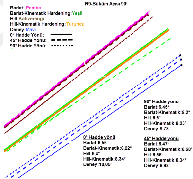
Şekil 7.25. Zımba yarıçapı R9, büküm açısı 90^\circ olduğu durumda malzeme modellerine göre A detayının geri yaylanmaların gösterimi.
