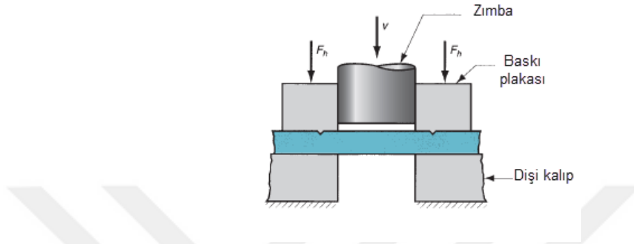
Şekil 3.2. Kesme işlemi
