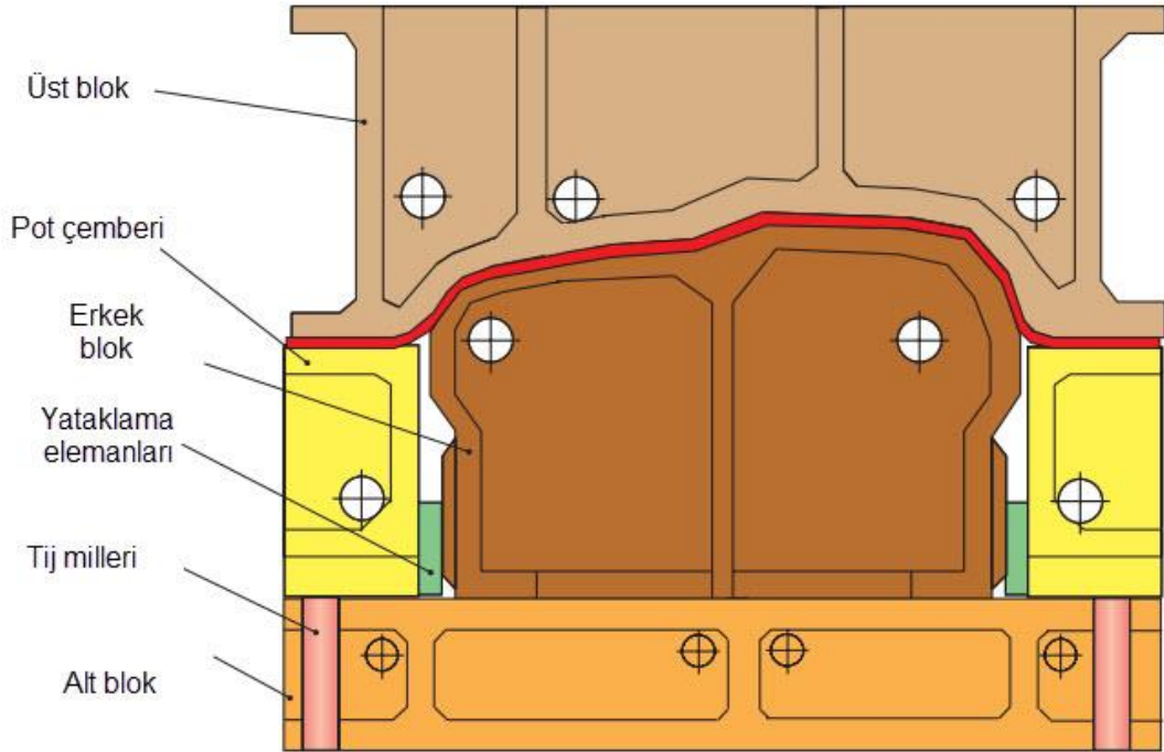
Şekil 3.1. Çekme kalıbı parçaları [33].
