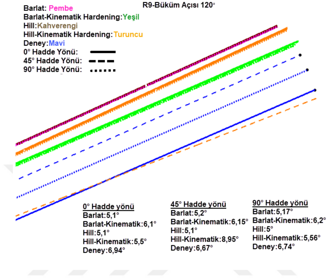
Şekil 7.27. Zımba yarıçapı R9, büküm açısı 120° olduğu durumda malzeme modellerine göre A detayının geri yaylanmaların gösterimi.
