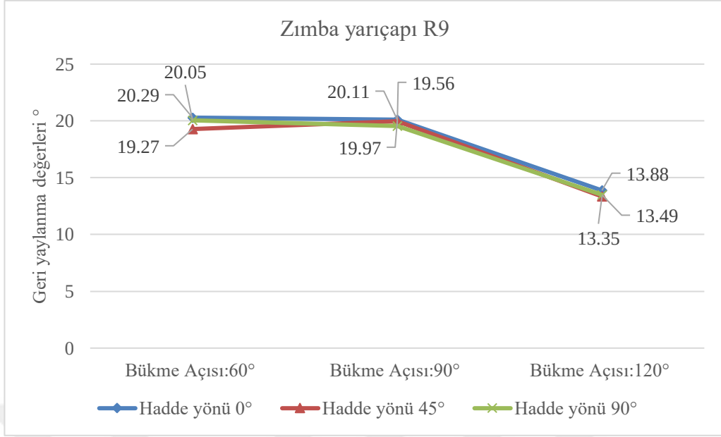
Şekil 7.4. R9 zimba yarıçapındaki geri yaylanma değerleri.
