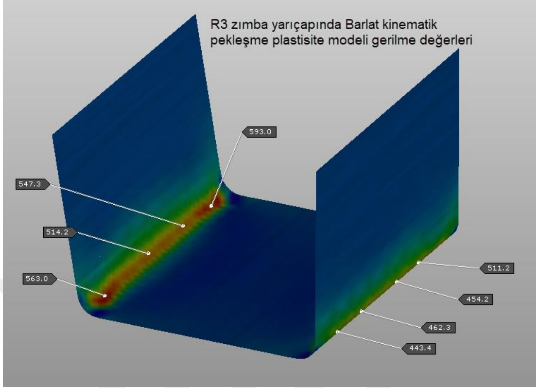
Şekil 7.37. R3 zımba yarıçapında Barlat-kinematik pekleşme malzeme modeline göre gerilme değerleri.
