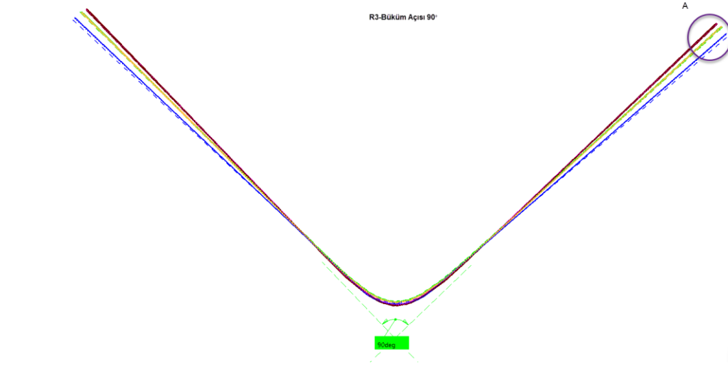
Şekil 7.12. Zımba yarıçapı R3, büküm açısı 90° olduğu durumda malzeme modellerine göre geri yaylanmaların gösterimi.
