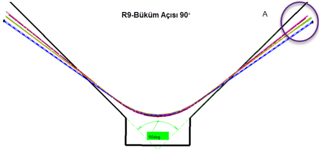
Şekil 7.24. Zımba yarıçapı R9, büküm açısı 90^\circ olduğu durumda malzeme modellerine göre geri yaylanmaların gösterimi.
