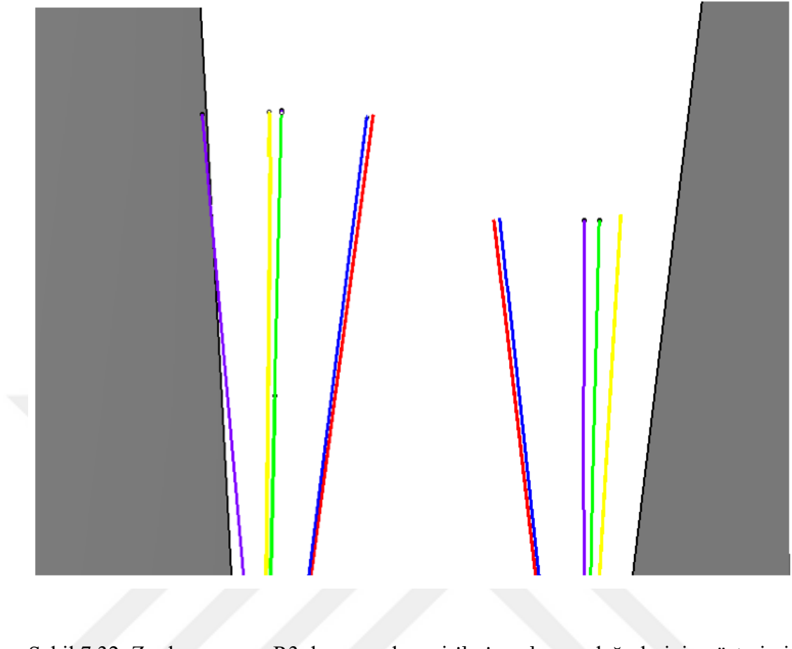
Şekil 7.32. Zımba yarıçapı R3 durumunda geri-ileri yaylanma değerlerinin gösterimi (a) Duvar açısı 93° (b) Duvar açısı 97°.
