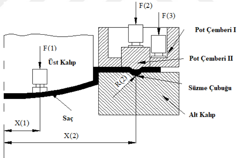
Şekil 4.3. Şekillendirme parametreleri.
