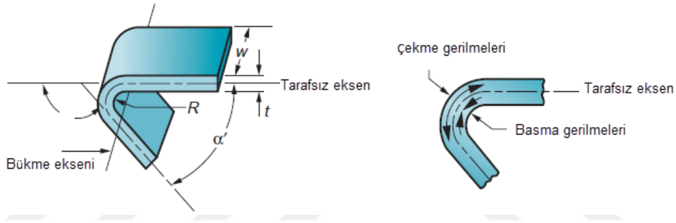
Şekil 3.4. Bükme işleminin incelenmesi [35].
