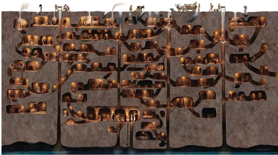
Şekil 21. Derinkuyu Yeraltı Şehri Şematik Kesit (URL-11).
