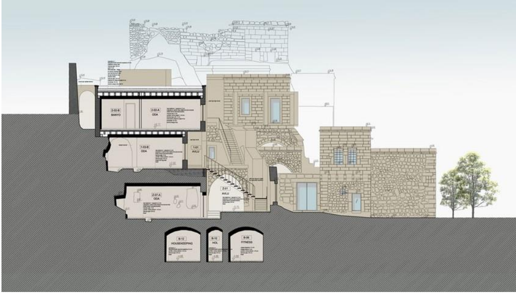
Şekil 54.Millstone Cave Suites-Kesit 2 (URL-49).
