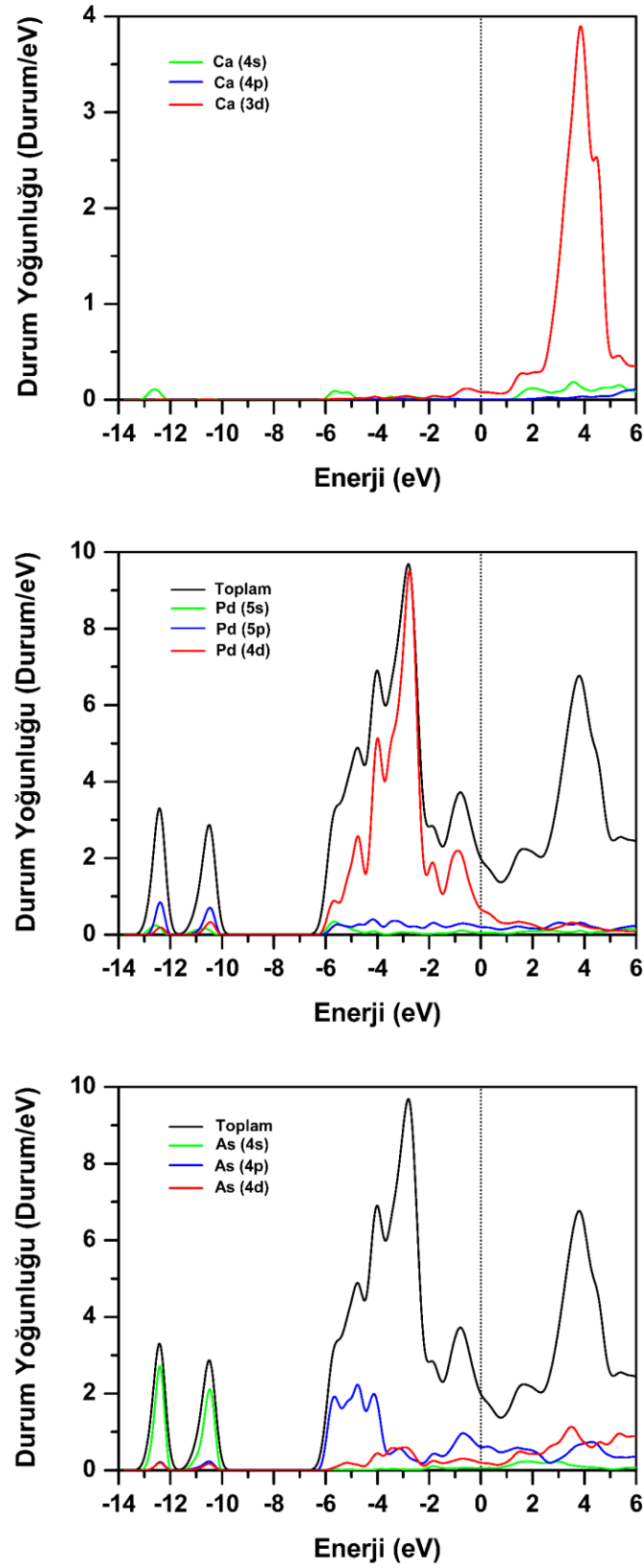
Şekil 5.15. \text{CaPd}_2\text{As}_2 malzemesi için toplam (siyah) ve kısmi (renkli) elektronik durum yoğunluğu. Fermi enerjisi 0 eV olarak alınmıştır.
