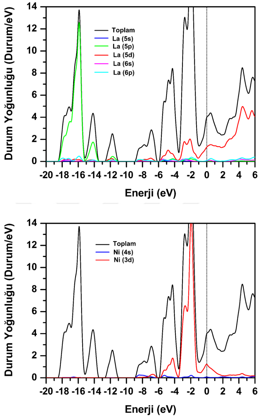
Şekil 5.65. \text{La}_3\text{Ni}_2\text{B}_2\text{N}_3 malzemesi için toplam ve kısmi (La,Ni) elektronik durum yoğunluğu. Fermi enerjisi 0 eV olarak alınmıştır.
