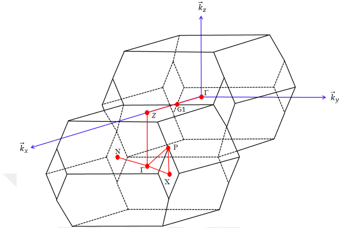
Şekil 2.9. BCT yapı için I.Brillouin bölgesi ve ana simetri noktalarının temsili gösterimi
