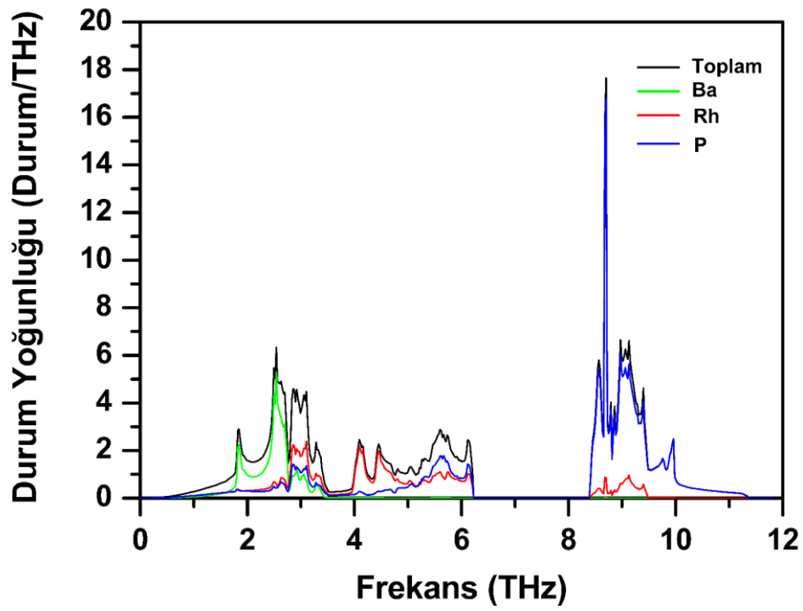
Şekil 5.41. BaRh 2 P 2 malzemesi için a-) fonon modlarının farklı yüksek simetri doğrultularında dağılımlarının gösterilmesi b-) fonon durum yoğunluğuna atomların katkısına göre gösterimi
