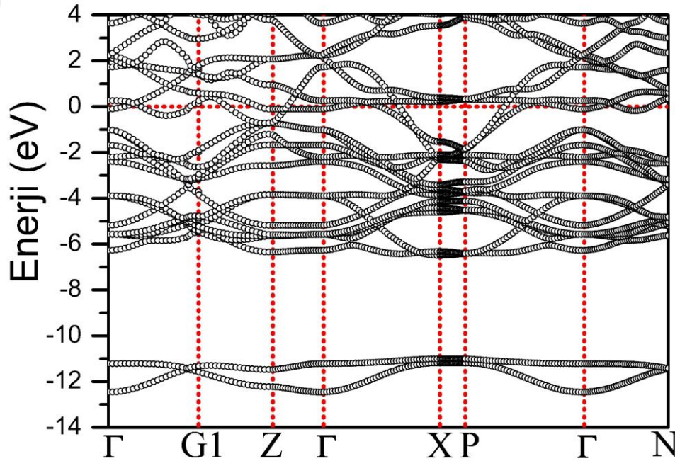
řekil 5.38. BaRh 2 P 2 malzemesi iin yksek simetri boyunca elektronik enerji band yapısı. Fermi enerjisi 0 eV olarak alınmıřtır.
