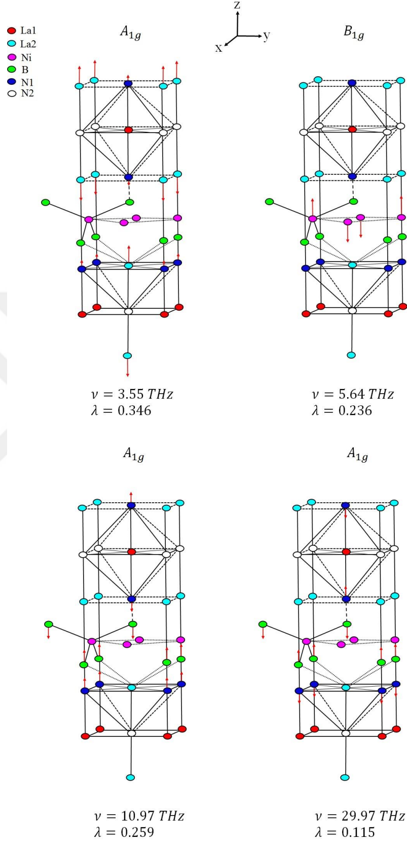
Şekil 5.67. \text{La}_3\text{Ni}_2\text{B}_2\text{N}_3 malzemesi için elektron-fonon etkileşim parametresine en yüksek katkısı yapan üç tane A_{1g} ve bir tane B_{1g} modunun özvektörler ile atomik yer değiştirmelerin gösterimi.
