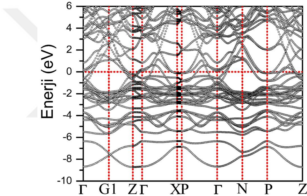
Şekil 5.64. La 3 Ni 2 B 2 N 3 malzemesi için yüksek simetri boyunca elektronik enerji band yapısı. Fermi enerjisi 0 eV olarak alınmıştır.
