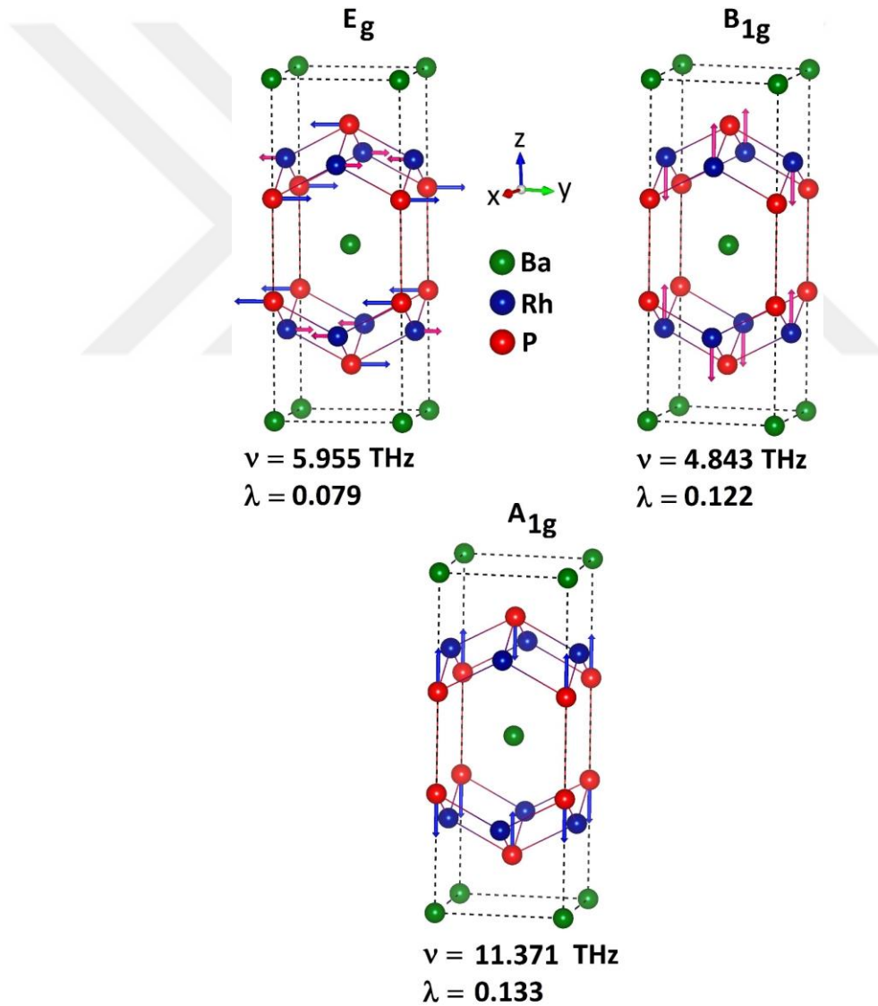
Şekil 5.40. BaRh_2P_2 malzemesi için elektron-fonon etkileşim parametresine en yüksek katkıyı yapan E_g , B_{1g} ve A_{1g} modlarının özvektörler ile atomik yer değiştirmelerin gösterimi.
