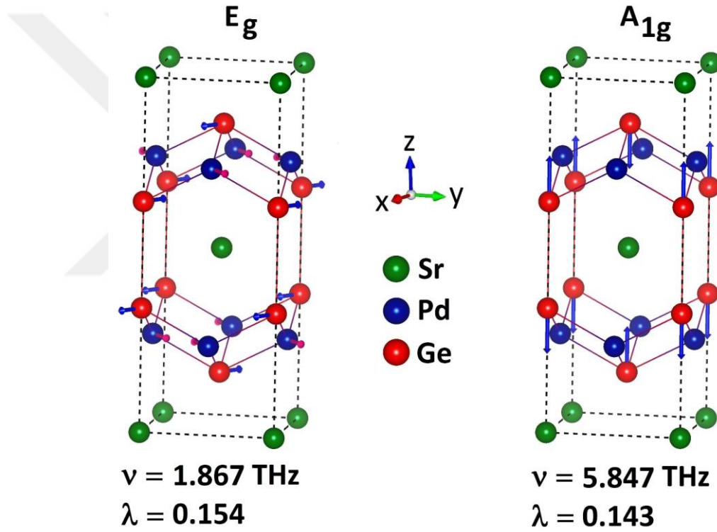
Şekil 5.4. \text{SrPd}_2\text{Ge}_2 malzemesi için elektron-fonon etkileşim parametresine en yüksek katkıyı yapan E_g ve A_{1g} optik fonon modlarının özvektörler ile atomik yer değiştirmelerin gösterimi.
