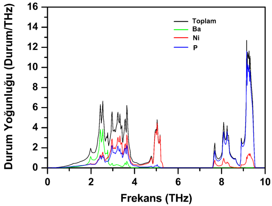
Şekil 5.35. \text{BaNi}_2\text{P}_2 malzemesi için a-) fonon modlarının farklı yüksek simetri doğrultularında dağılımlarının gösterilmesi b-) fonon durum yoğunluğuna atomların katkısına göre gösterimi
