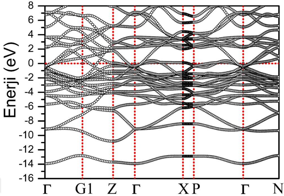
Şekil 5.57. \text{ScNi}_2\text{B}_2\text{C} malzemesi için yüksek simetri boyunca elektronik enerji band yapısı. Fermi enerjisi 0 eV olarak alınmıştır
