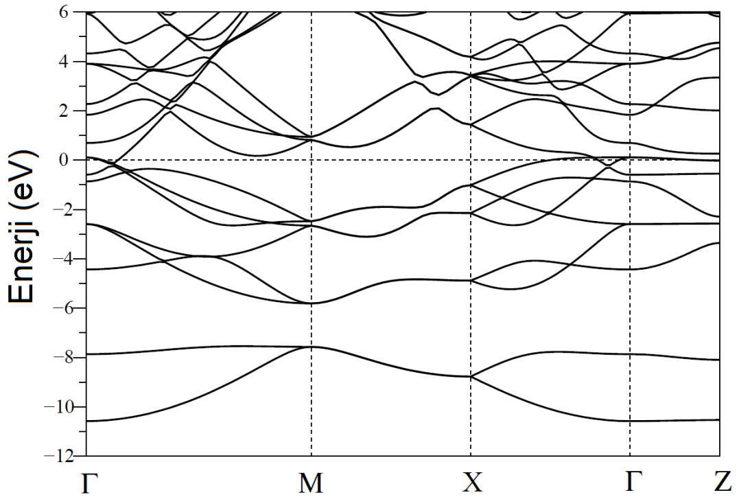
Şekil 4.3. NaAlSi malzemesi için yüksek simetri boyunca elektronik enerji band yapısı. Fermi enerjisi 0 eV olarak alınmıştır.
