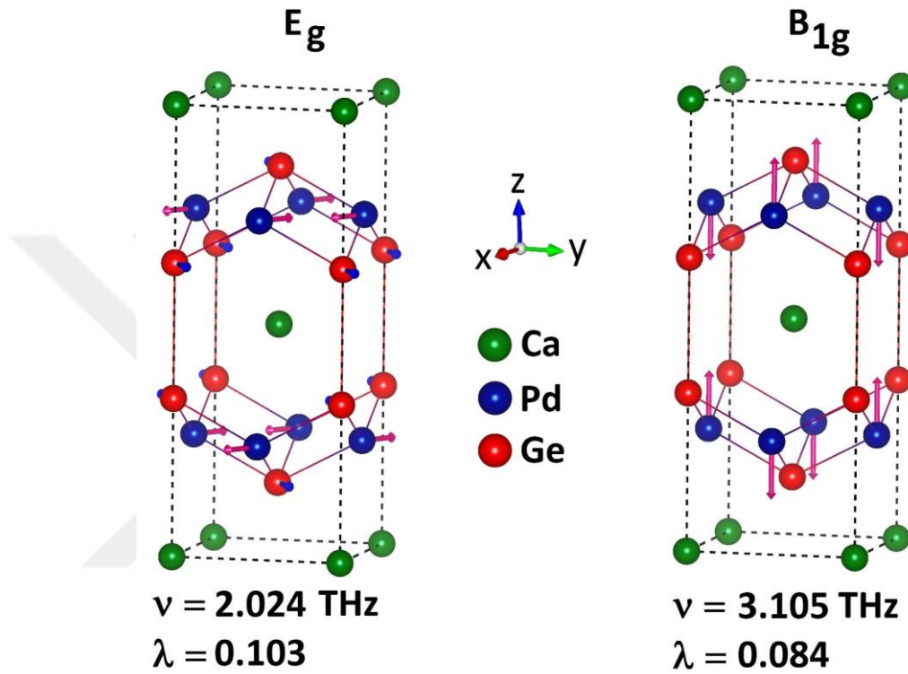
Şekil 5.22. CaPd 2 Ge 2 malzemesi için elektron-fonon etkileşim parametresine en yüksek katkıyı yapan E_g ve B_{1g} modlarının özvektörler ile atomik yer değiştirmelerin gösterimi.
