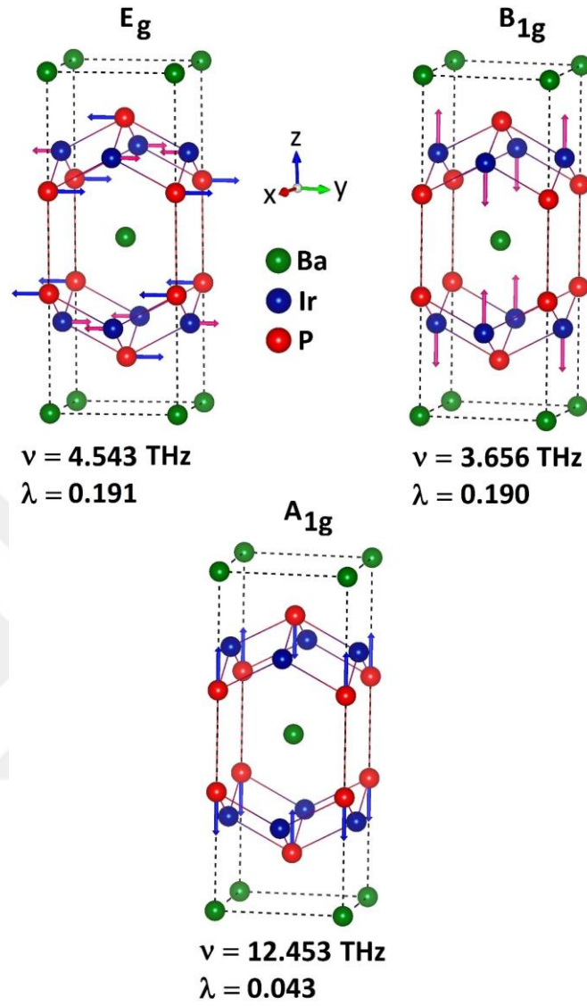
Şekil 5.46. BaIr 2 P 2 malzemesi için elektron-fonon etkileşim parametresine en yüksek katkısı yapan E g , B 1g ve A 1g modlarının özvektörler ile atomik yer değiştirmelerin gösterimi.
