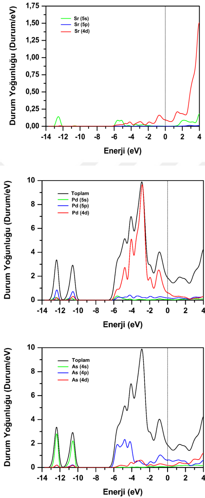
Şekil 5.9. \text{SrPd}_2\text{As}_2 malzemesi için toplam (siyah) ve kısmi (renkli) elektronik durum yoğunluğu. Fermi enerjisi 0 eV olarak alınmıştır.
