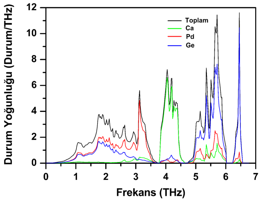
Şekil 5.23. \text{CaPd}_2\text{Ge}_2 malzemesi için a-) fonon modlarının farklı yüksek simetri doğrultularında dağılımlarının gösterilmesi b-) fonon durum yoğunluğuna atomların katkısına göre gösterimi
