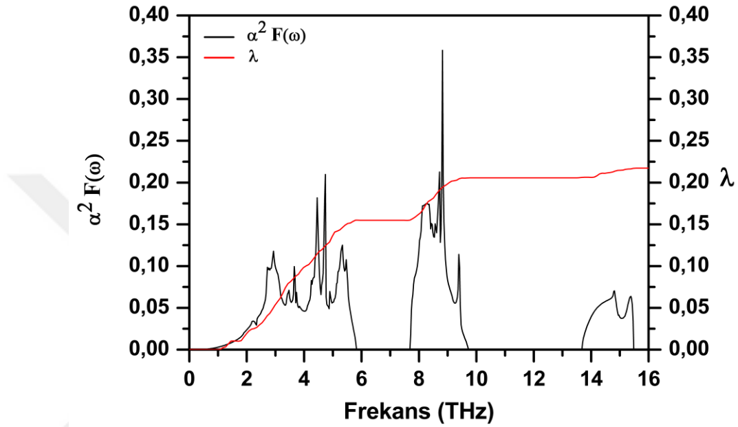
Şekil 5.30. \text{LiCu}_2\text{P}_2 malzemesi için Eliashberg spektral fonksiyonunun elektron-fonon etkileşim parametresine göre değişimi
