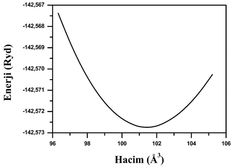
Şekil 5.7. \text{SrPd}_2\text{As}_2 malzemesi için a-) kristal yapının gösterimi b-) hesaplamalar sonucu elde edilen Enerji-Hacim grafiği
