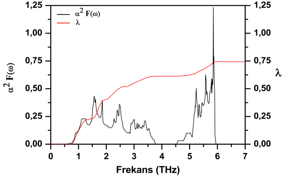
Şekil 5.6. \text{SrPd}_2\text{Ge}_2 malzemesi için Eliashberg spektral fonksiyonunun elektron-fonon etkileşim parametresine göre değişimi
