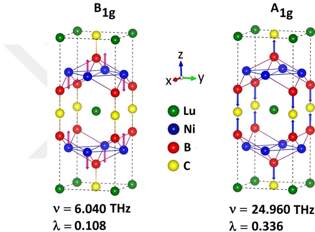
Şekil 5.52. LuNi_2B_2C malzemesi için elektron-fonon etkileşim parametresine en yüksek katkıyı yapan B_{1g} ve A_{1g} modlarının özvektörler ile atomik yer değiştirmelerin gösterimi.
