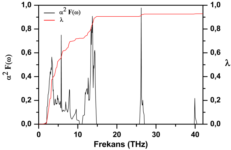
Şekil 5.62. ScNi 2 B 2 C malzemesi için Eliashberg spektral fonksiyonunun elektron-fonon etkileşim parametresine göre değişimi
