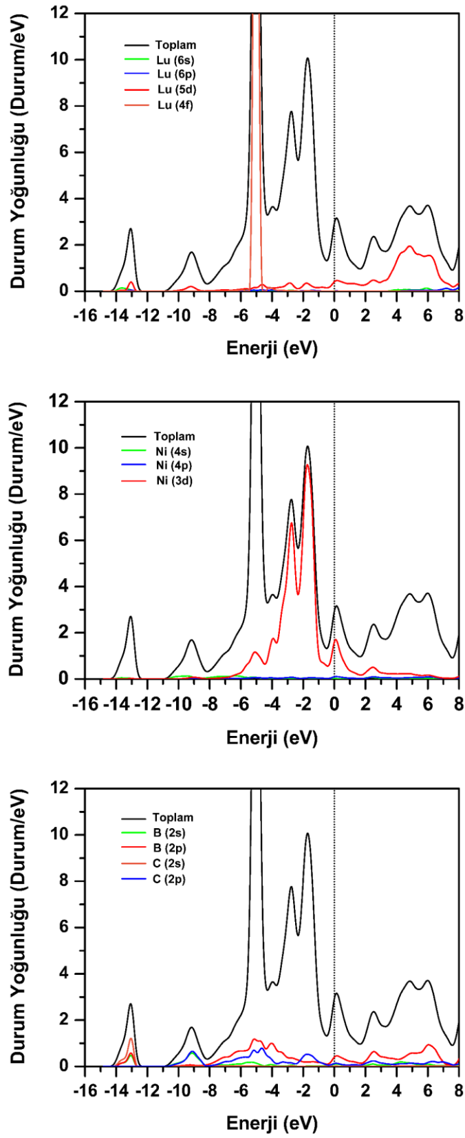
Şekil 5.51. \text{LuNi}_2\text{B}_2\text{C} malzemesi için toplam ve kısmi elektronik durum yoğunluğu. Fermi enerjisi 0 eV olarak alınmıştır.
