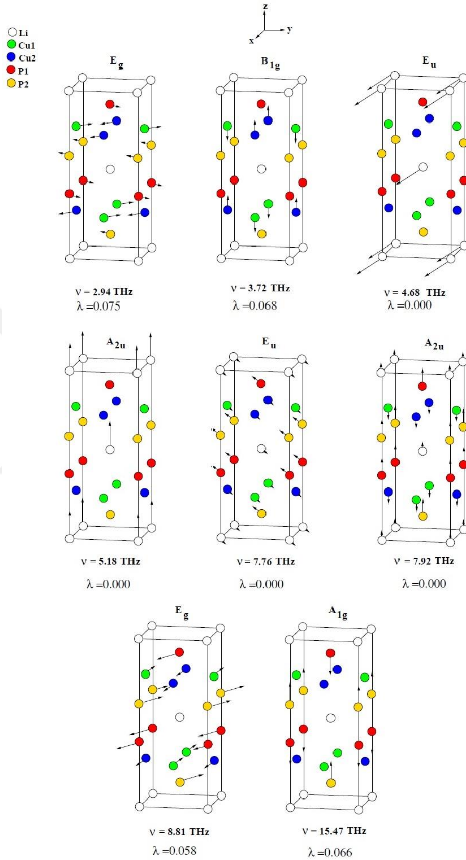
Şekil 5.28. LiCu 2 P 2 malzemesinin optik modlara ait özvektörler ile atomik yer değiştirmelerin gösterimi.
