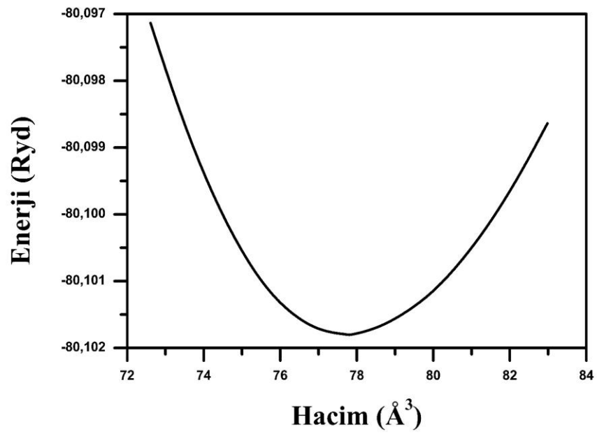
Şekil 5.70. \text{Bi}_2\text{Pd} malzemesi için a-) kristal yapının gösterimi b-) hesaplamalar sonucu elde edilen Enerji-Hacim grafiği
