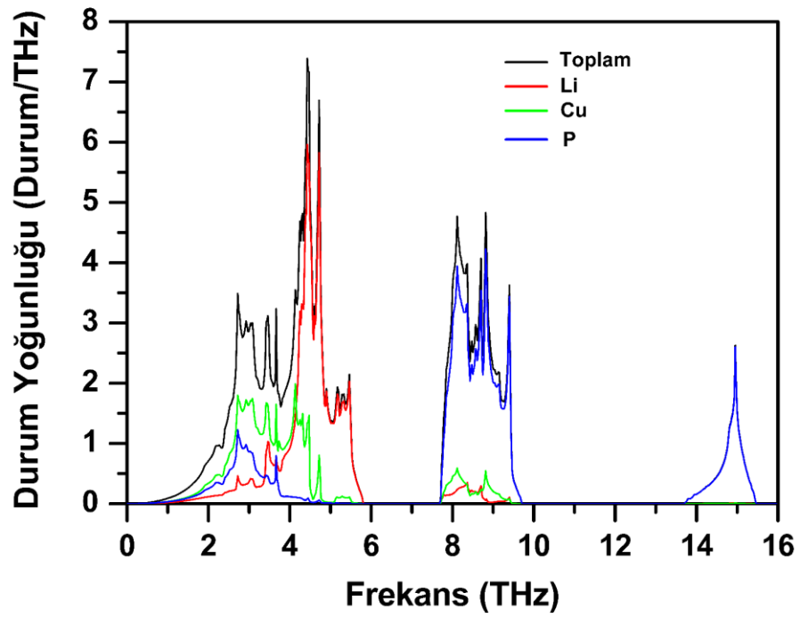
Şekil 5.29. \text{LiCu}_2\text{P}_2 malzemesi için a-) fonon modlarının farklı yüksek simetri doğrultularında dağılımlarının gösterilmesi b-) fonon durum yoğunluğuna atomların katkısına göre gösterimi
