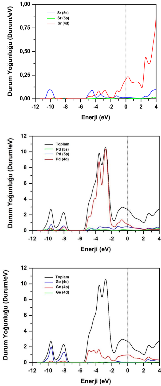
Şekil 5.3. \text{SrPd}_2\text{Ge}_2 malzemesi için toplam (siyah) ve kısmi (renkli) elektronik durum yoğunluğu. Fermi enerjisi 0 eV olarak alınmıştır.
