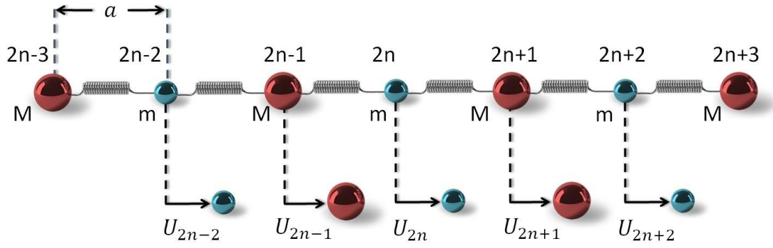
Şekil 3.5. Denge durumundan küçük yer değıştirmeler yapan bir boyutta iki atomlu örgü.
