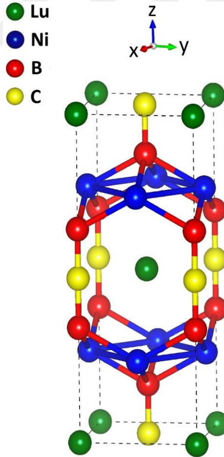
Şekil 2.8. \text{LuNi}_2\text{B}_2\text{C} malzemesinin kristal yapısının şematik gösterimi.
