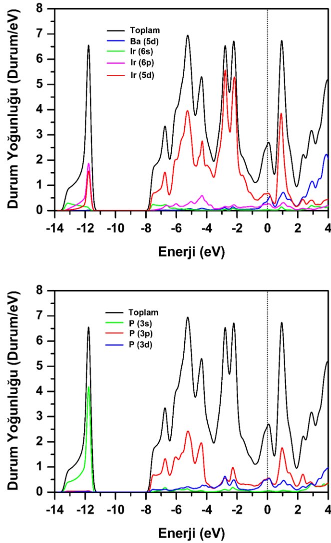
Şekil 5.45. BaIr 2 P 2 malzemesi için toplam ve kısmi elektronik durum yoğunluğu. Fermi enerjisi 0 eV olarak alınmıştır.
