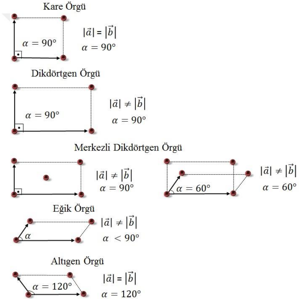
Şekil 2.4. İki boyutta örgü türleri
