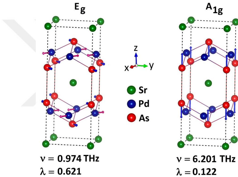
Şekil 5.10. \text{SrPd}_2\text{As}_2 malzemesi için elektron-fonon etkileşim parametresine en yüksek katkıyı yapan E_g ve A_{1g} modlarının özvektörler ile atomik yer değiştirmelerin gösterimi.
