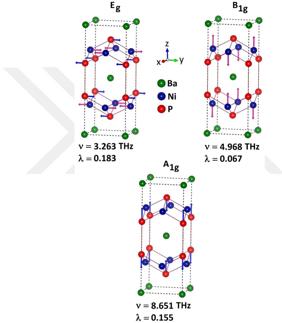
Şekil 5.34. BaNi 2 P 2 malzemesi için elektron-fonon etkileşim parametresine en yüksek katkısı yapan E_g , B_{1g} ve A_{1g} modlarının özvektörler ile atomik yer değiştirmelerinin gösterimi.
