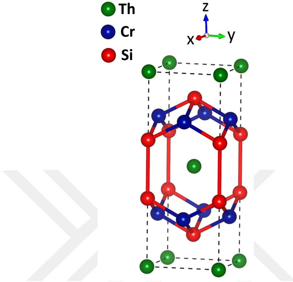
Şekil 2.7. ThCr 2 Si 2 malzemesinin kristal yapısının şematik gösterimi.
