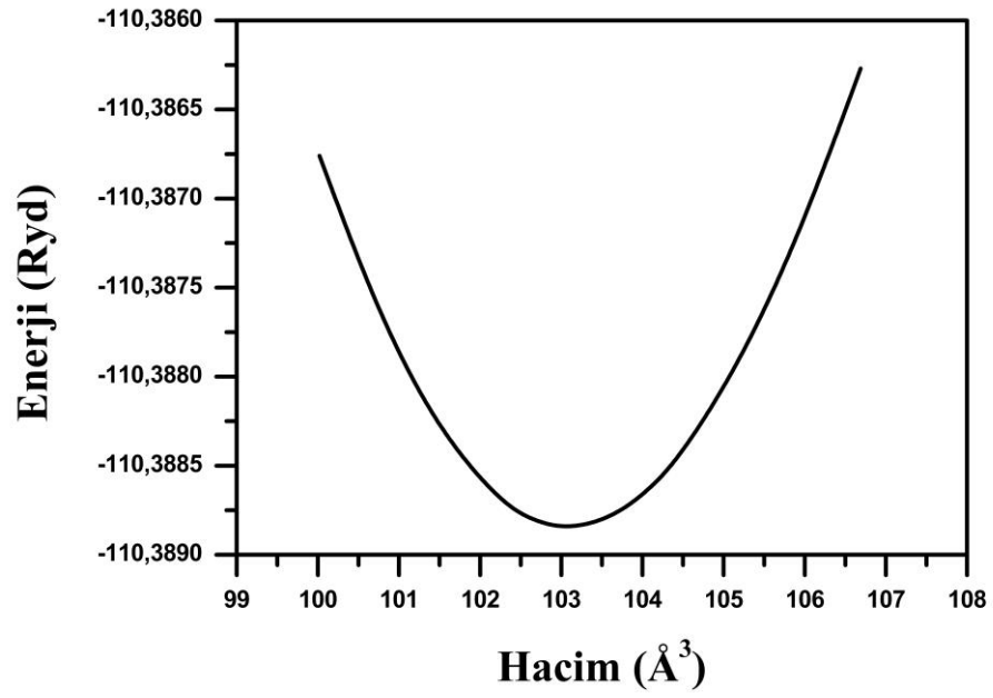
Şekil 5.43. BaIr 2 P 2 malzemesi için a-) kristal yapının gösterimi b-) hesaplamalar sonucu elde edilen Enerji-Hacim grafiği
