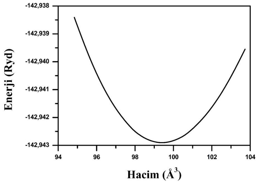
Şekil 5.13. \text{CaPd}_2\text{As}_2 malzemesi için a-) kristal yapının gösterimi b-) hesaplamalar sonucu elde edilen Enerji-Hacim grafiği
