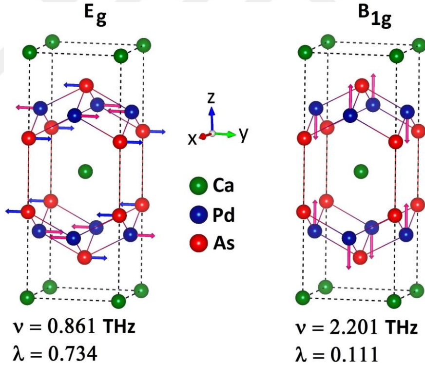
Şekil 5.16. \text{CaPd}_2\text{As}_2 malzemesi için elektron-fonon etkileşim parametresine en yüksek katkıyı yapan E_g ve B_{1g} modlarının özvektörler ile atomik yer değiştirmelerin gösterimi.
