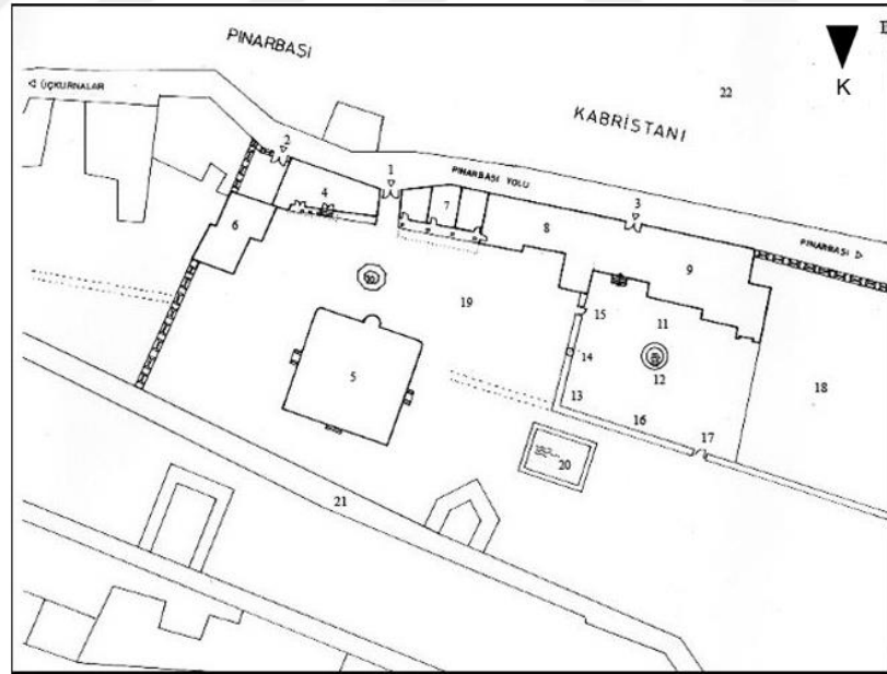
Şekil 3.177. Bursa Mevlevihanesi vaziyet planı, 1. Cümle kapısı, 2. Matbah girişi, 3. Hareme sokaktan girişi, 4. Türbe, 5. Semahane (Mihrap yönü hatalı çizilmiş), 6. Matbah-ı şerif ve hizmet odaları, 7. Dedegan hücreleri, 8. Selamlık, 9. Harem, 10. Şadırvan, 11. Harem bahçesi, 12. Havuz etrafından gezinti yolları ve meyve bahçeleri, 13. Harem bahçesini selamlıktan ayıran duvar, 14. Matbah-Harem dönme dolabı, 15. Geçiş kapısı, 16. Duvar, 17. Büyük bahçeye açılan kapı, 18. Çamaşır bahçesi, 19. Ana avlu, 20. Büyük havuz, 21. Kale surları, 22. Pınarbaşı kabristanı, (BVBMA).
