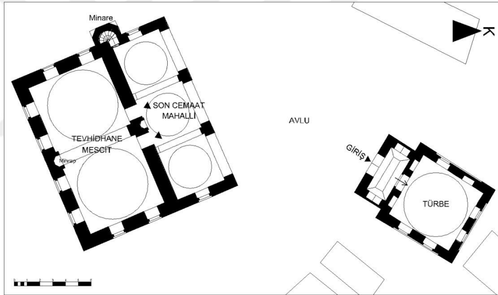
Şekil 3.1. Abdal Mehmet Tekkesi kat planı, Demirtaşpaşa Mh./Bursa, 15.yy., Kadiriyye (Gabriel.'den düzeltilerek çizilmiştir, Osmanoğlu İ., Taşkın C., 2015), [89].
