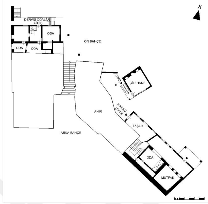
Şekil 3.100. Üftâde Tekkesi birinci kat planı, Molla Fenari Mh./Bursa, 16.yy., Celvetiyye (İşlenerek yeniden çizilmiştir, Osmanoglu İ., Taşkın C., 2014), [212].
