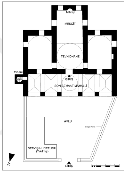
Şekil 3.21. Ebu İshak Kâzeruni Tekkesi planı, Ebu İshak Mh./Bursa, 15.yy., Kâzeruniyye (Gabriel' den düzeltilerek çizilmiştir, Osmanoğlu İ., Taşkın C., 2015), [89].
