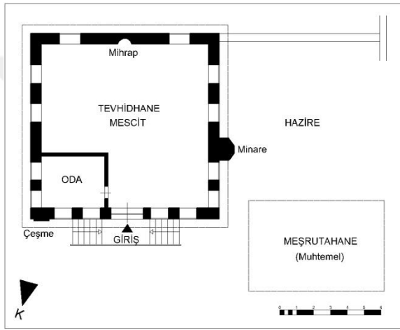
Şekil 3.70. Veli Şemseddin Tekkesi kat planı, Maksem Mh./Bursa, (Rölöve, Osmanoğlu İ., Taşkın C., 2015), [15].
