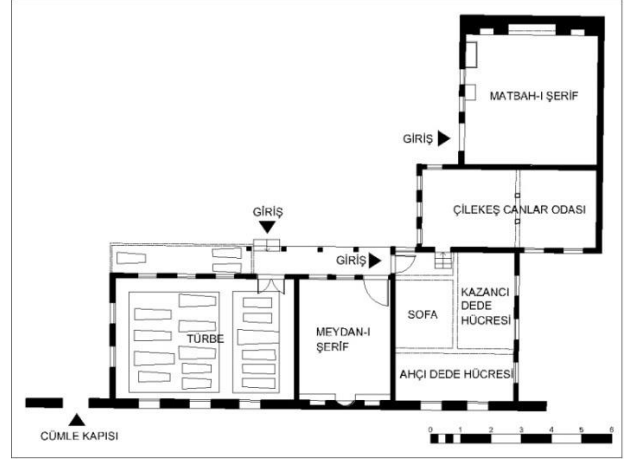
Şekil 3.179. Bursa Mevlevihanesi Türbe, Matbah-ı Şerif, Meydan-ı Şerif kat planı (B. Tanrıkorur 1994, BVBMA.'den düzeltilerek çizilmiştir, Osmanoğlu İ., Taşkın C., 2015).
