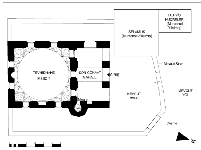
Şekil 3.40. Karakadi Tekkesi planı, Alacamescit Mh./Bursa, 15.yy., Halvetiyye, Kadiriyye, Celvetiyye, (Rölöve, Osmanoğlu İ., Taşkın C., 2015).
