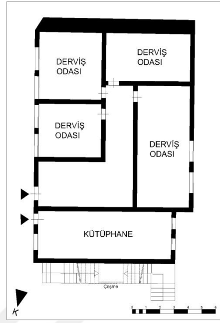
Şekil 3.146. İsmail Hakkı Tekkesi zemin kat planı, Tuzpazarı Mh./Bursa, 18. yy. (Gabriel'den ve rölöve ile düzeltilerek çizilmiştir, Osmanoğlu İ., Taşkın C., 2015), [89].
