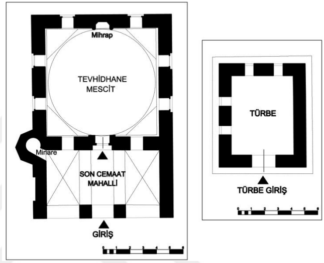
Şekil 3.8. Akbıyık Sultan Tekkesi planı, Nalbantoğlu Mh./Bursa, 15.yy., Bayramiyye (Rölöve, Osmanoğlu İ., Taşkın C., 2014).
