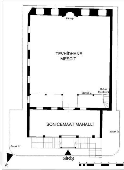
Şekil 3.145. İsmail Hakkı Tekkesi tevhidhane kat planı, Tuzpazarı Mh./Bursa, 18. yy. (Gabriel'den ve rölöve ile düzeltilerek çizilmiştir, Osmanoğlu İ., Taşkın C., 2015), [89].
