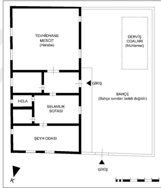
Şekil 3.81. Būdelâ Bey Tekkesi selamlık ve tevhidhane planı, Kocanaib Mh./Bursa, Halvetiyye, Rifaiyye, Bektaşîyye, Nakşibendiyye, 16. yy. (BVBMA'den ve yerinde rölöve ile düzeltilerek çizilmiştir, Osmanoğlu İ., Taşkın C., 2015).
