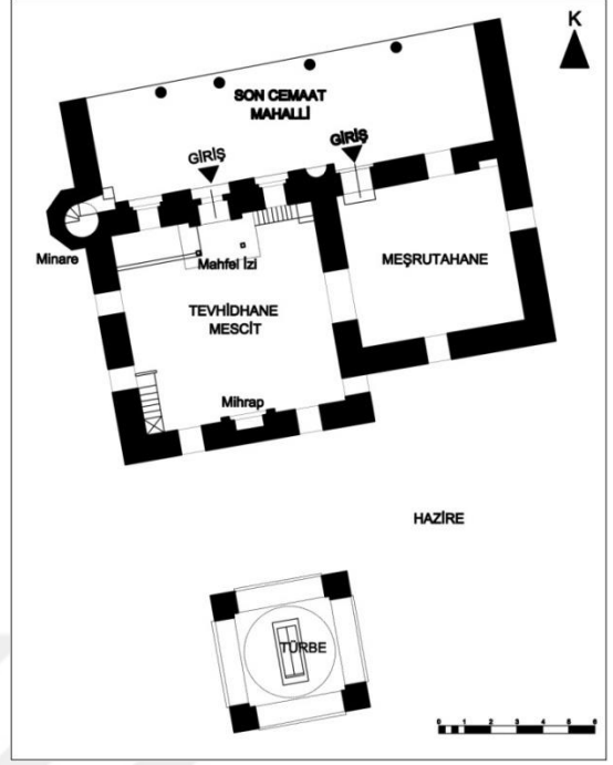
Şekil 3.65. Umur Bey Tekkesi kat planı, Umur Bey Mh./Bursa, 15. yy. (Gabriel'den düzeltilerek çizilmiştir, Osmanoğlu İ., Taşkın C., 2015).
