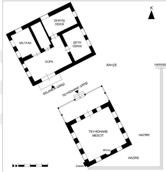
Şekil 3.92. Nakkaş Ali Tekkesi, Tevhidhane ve selamlık zemin kat planı, Osmangazi Mh./Bursa, 16. yy., Nakşibendiyye (BVBMA'den ve yerinde rölöve ile düzeltilerek çizilmiştir, Osmanoglu İ., Taşkın C., 2015).
