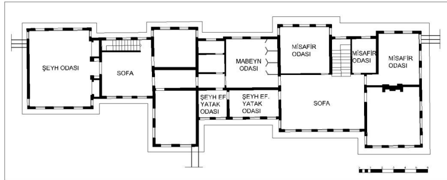
Şekil 3.181. Bursa Mevlevihanesi harem ve selamlık birinci kat planı (B. Tanrıkorur 1994, BVBMA.'den düzeltilerek çizilmiştir, Osmanoğlu İ., Taşkın C., 2015)
