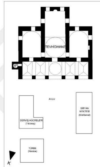
Şekil 3.22. Ebu İshak Kâzeruni Tekkesi mekan şeması, Restitüsyon denemesi [15,89,100].
