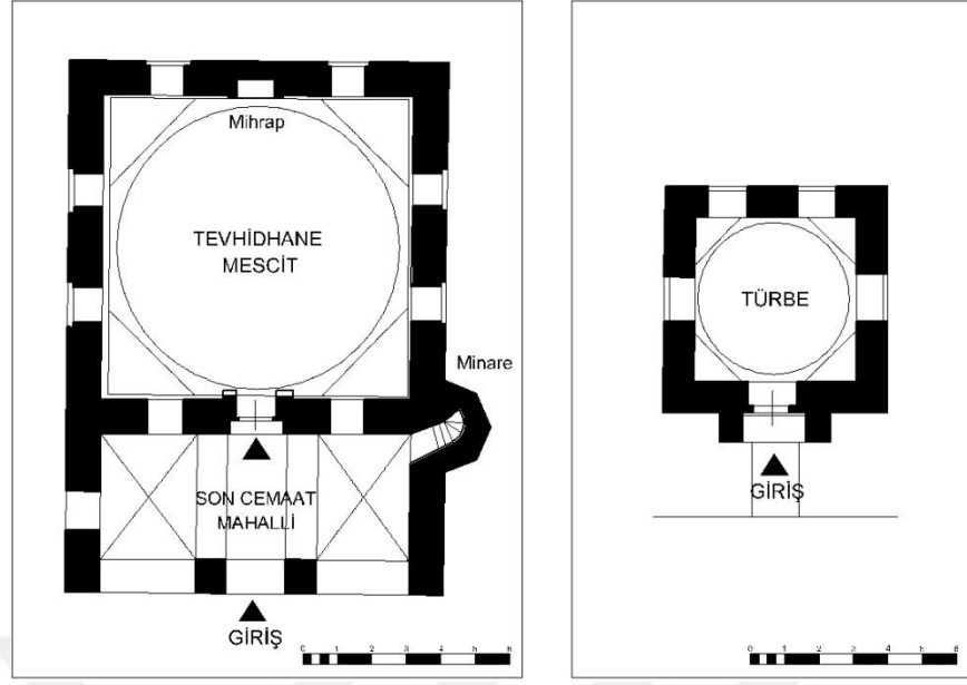
Şekil 3.73. Zeyniler Tekkesi, Solda Tevhidhane (Cami) planı, Sağda Türbe planı Umur Emir Sultan Mh./Bursa, 15. yy. (Gabriel'den ve rölöve ile düzeltilerek çizilmiştir, Osmanoğlu İ., Taşkın C., 2015), [198].
