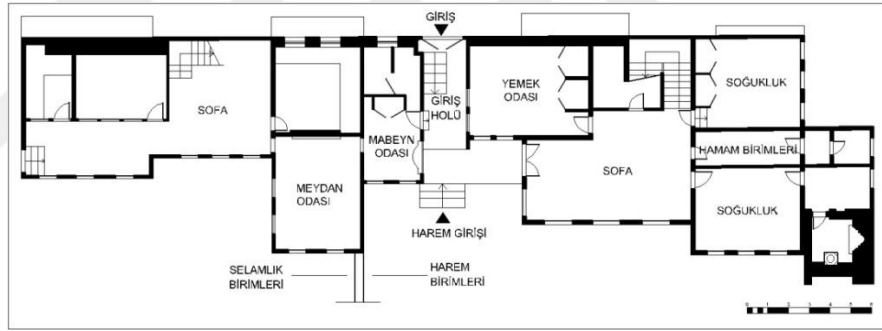
Şekil 3.180. Bursa Mevlevihanesi harem ve selamlık zemin kat planı (B. Tanrıkorur 1994, BVBMA.'den düzeltilerek çizilmiştir, Osmanoğlu İ., Taşkın C., 2015).
