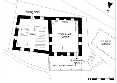
Şekil 3.114. Hüsameddin Tekke zemin kat planı, (Piray Mimarlık ve BVBMA.'den düzeltilerek çizilmiştir, Osmanoğlu İ., Taşkın C., 2015).
