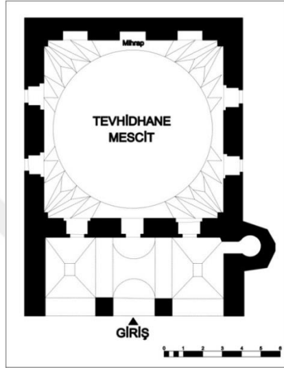
Şekil 3.15. Bedreddin Pars Bey Tekkesi tevhidhane planı, Şehreküstü Mh./Bursa, 15.yy., Nakşibendiyye (Kökten B.'den düzeltilerek çizilmiştir, Osmanoğlu İ., Taşkın C., 2015), [100].
