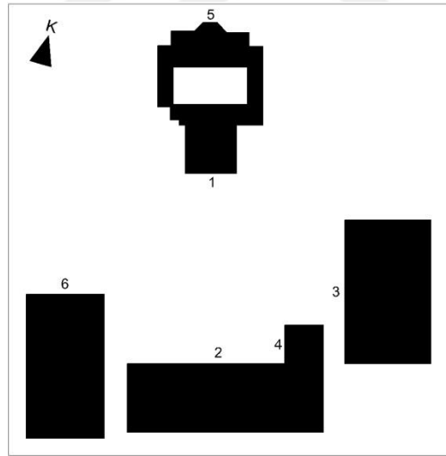
Şekil 3.25. Emir Buhari Tekkesi vaziyet planı şeması, 1.Tevhidhane, 2.Harem, 3. Muhtemel Selamlık, 4.Çilehane, 5.Türbe, 6.Hamam, (Osmanoğlu İ., Taşkın C.,2015) [15,89].
