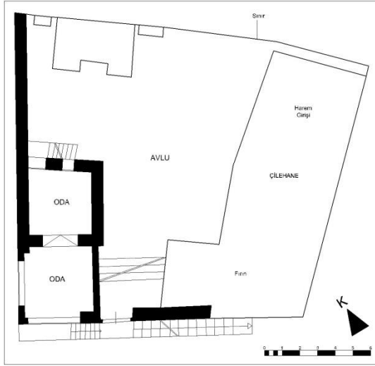
Şekil 3.58. Somuncu Baba Tekkesi birinci kat planı, Molla Fenari Mh./Bursa, 15. yy. (BVBMA.'den düzeltilerek çizilmiştir, Osmanoğlu İ., Taşkın C., 2015).
