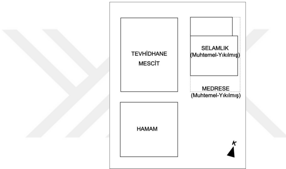
Şekil 3.43. Mecnun Dede Tekkesi plan şeması, Restitüsyon denemesi, Tahtakale Mh./Bursa, 15.yy., (Osmanoğlu İ., Taşkın C., 2015), [201].
