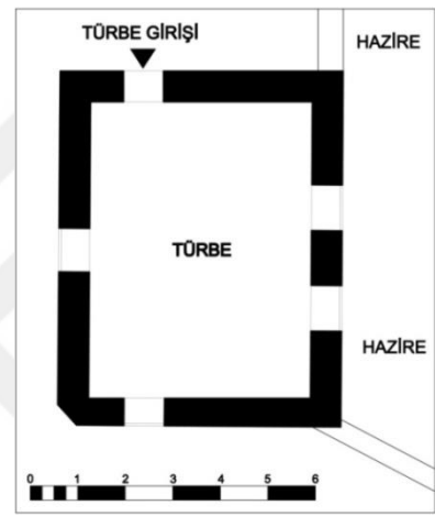
Şekil 3.129. Üçkozlar Tekkesi türbe planı, Molla Fenari Mh./Bursa (Rölöve, Osmanoğlu İ., Taşkın C., 2015).
