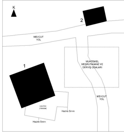
Şekil 3.46. Seyyid Nasır Tekkesi vaziyet planı şeması, Restitüsyon denemesi, 1.Tevhidhane, 2.Türbe, Molla Fenari Mh./Bursa, 15.yy. (Osmanoğlu İ., Taşkın C., 2015), [15,100].
