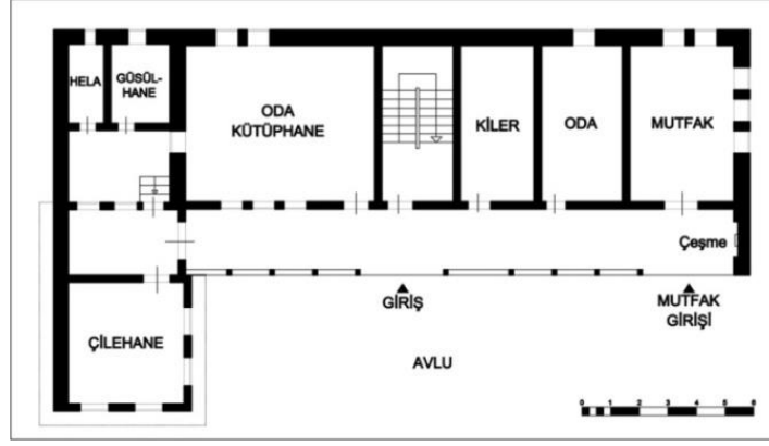
Şekil 3.26. Emir Buhari Tekkesi haremi zemin kat planı, Emirsultan Mh. /Bursa, 15. yy., Kübreviyye, Celvetiyye, Nakşibendiyye, (Rölöve, Osmanoğlu İ., Taşkın C., 2015).
