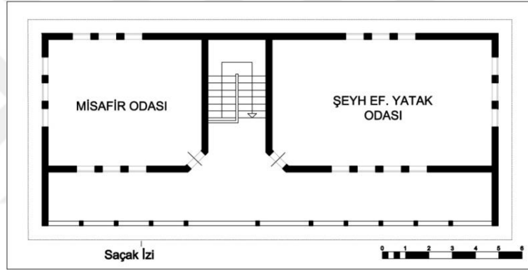
Şekil 3.27. Emir Buhari Tekkesi haremi birinci kat planı, Emirsultan Mh. /Bursa, 15. yy., Kübreviyye, Celvetiyye, Nakşibendiyye, (Rölöve, Osmanoğlu İ., Taşkın C., 2015).
