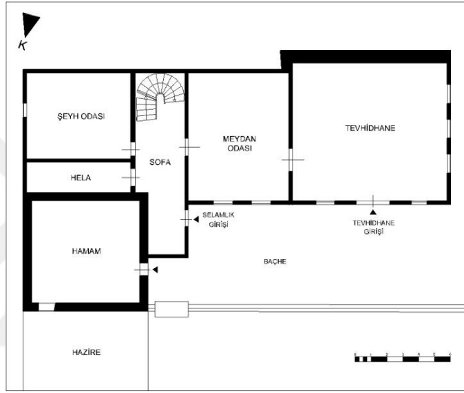
Şekil 3.151. İsmail Rumi Tekkesi zemin kat planı, Ali Paşa Mh./Bursa, 19.yy., Sadiyye Rifaiyye, Kadiriyye, Şabaniyye (BVBMA.'den düzeltilerek çizilmiştir, Osmanoglu İ., Taşkın C., 2015).
