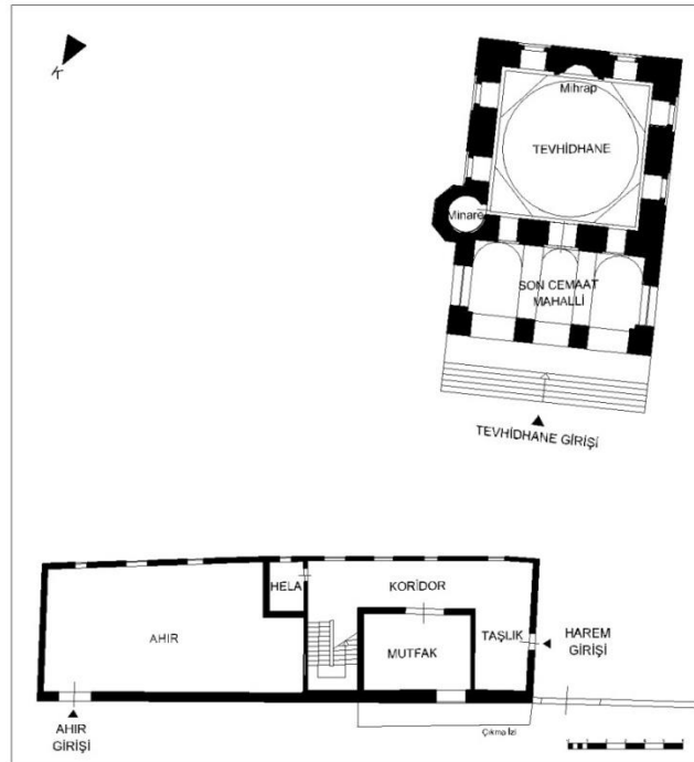
Şekil 3.78. Bahri Dede Tekkesi tevhidhane ve harem planı, Muradiye Mh./Bursa, Halvetiyye, 16. yy. (BVBMA'den ve yerinde rölöve ile düzeltilerek çizilmiştir, Osmanoglu İ., Taşkın C., 2015).
