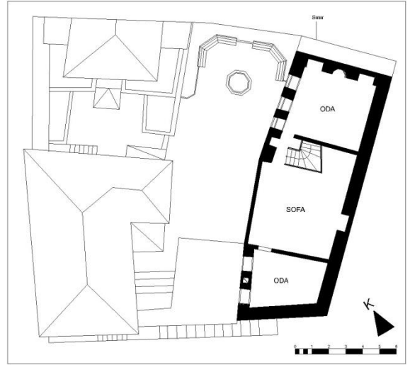
Şekil 3.59. Somuncu Baba Tekkesi ikinci kat planı, Molla Fenari Mh./Bursa, 15. yy. (BVBMA.'den düzeltilerek çizilmiştir, Osmanoğlu İ., Taşkın C., 2015).
