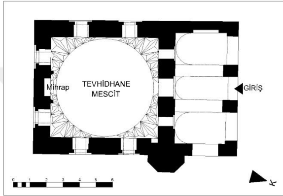
Şekil 3.19. Düstürhan Tekkesi'nde tevhidhane olarak kullanılan Düstürhan Cami planı, Pınarbaşı Mh./Bursa, 15.yy., Halvetiyye (Kökten B.'den düzeltilerek çizilmiştir, Osmanoğlu İ., Taşkın C., 2015), [100].
