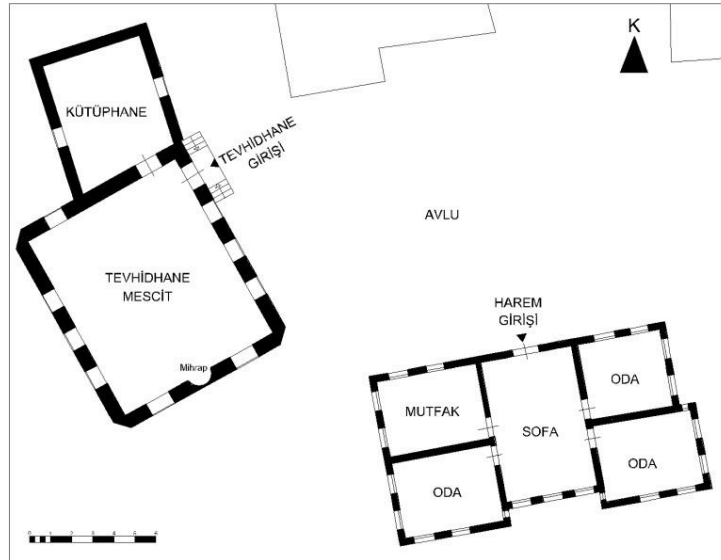
Şekil 3.137. Cizyedarzâde Tekkesi tevhidhane, kütüphane ve harem zemin kat planları, Kavaklı Mh./Bursa, 18.yy., Nakşibendiyye (BVBMA.'den düzeltilerek çizilmiştir, Osmanoğlu İ., Taşkın C., 2015).
