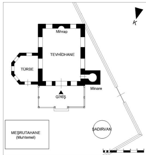
Şekil 3.133. Zağferanlık Tekkesi tevhidhane ve türbe planı, Reyhan Mh./Bursa, 17. yy. (Rölöve, Osmanoglu İ., Taşkın C., 2015), [15].
