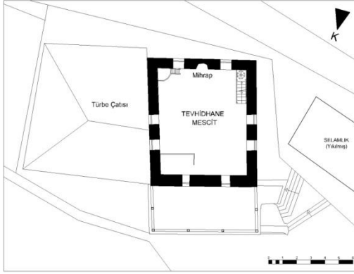
Şekil 3.115. Hüsameddin Tekke tevhidhane planı (BVBMA.'den düzeltilerek çizilmiştir, Osmanoğlu İ., Taşkın C., 2015).
