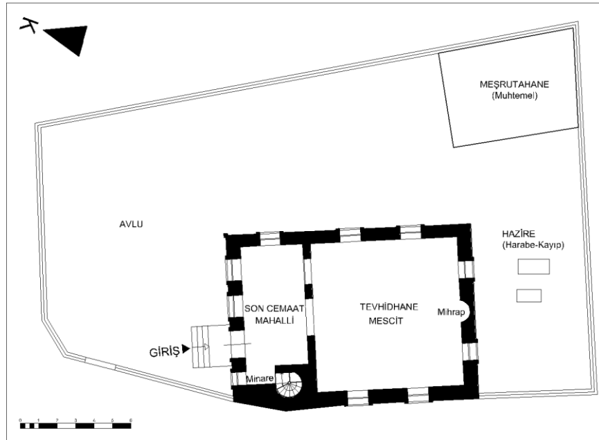
Şekil 3.4. Ahmed Paşa-yı Fenari Tekkesi planı, Ahmet Paşa Mh./Bursa, 15.yy., Halvetiyye, (Rölöve, Osmanoğlu İ., Taşkın C., 2015), [15].
