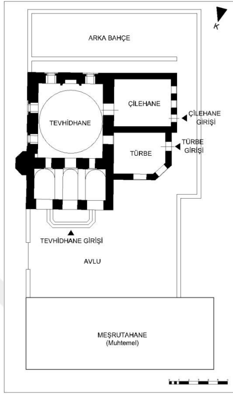
Şekil 3.142. Emîniyye Tekkesi tevhidhane, çilehane ve türbe planı, Ali Paşa Mh./Bursa, 17.yy., Nakşibendiyye (Rölöve, Osmanoğlu İ., Taşkın C., 2015).
