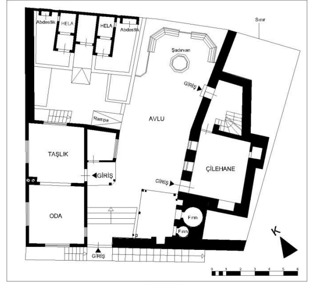
Şekil 3.57. Somuncu Baba Tekkesi zemin kat planı, Molla Fenari Mh./Bursa, 15. yy. (BVBMA.'den düzeltilerek çizilmiştir, Osmanoğlu İ., Taşkın C., 2015).
