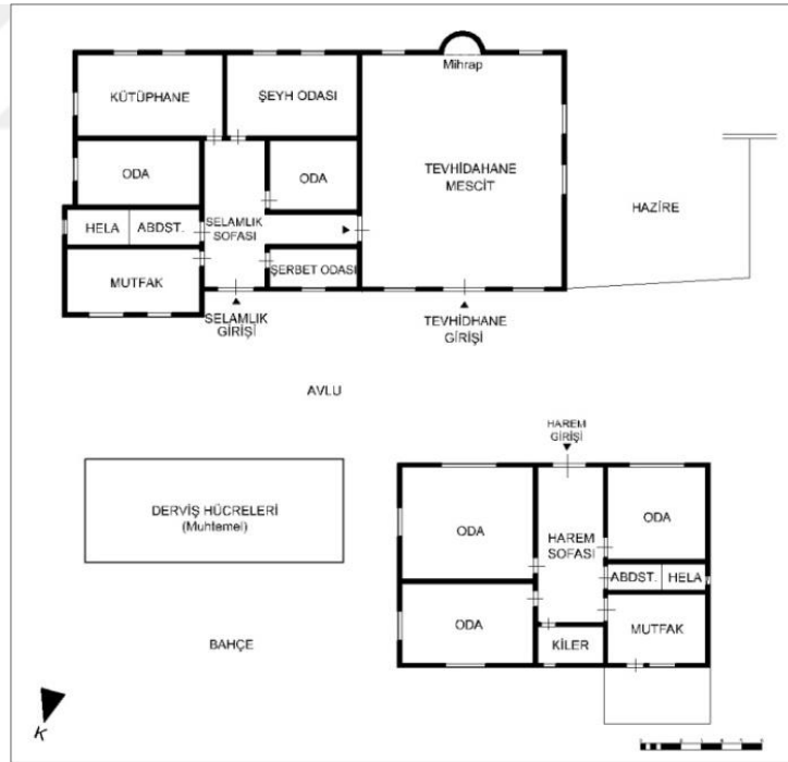
Şekil 3.172. Eşrefzâde Tekkesi tevhidhane, selamlık ve harem zemin kat planı, İncirli Mh. /Bursa, 17. yy., Kadiriyye/Eşrefiyye (BVBMA.'den düzeltilerek çizilmiştir, Osmanoğlu İ., Taşkın C., 2015).
