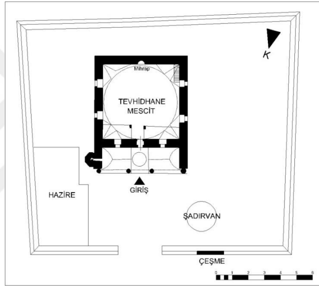
Şekil 3.97. Nasuhi Tekkesi, Tevhidhane olarak kullanılan Alâaddin Paşa Cami'nin planı (BVBMA'den ve yerinde rölöve ile düzeltilerek çizilmiştir, Osmanoğlu İ., Taşkın C., 2015), [15].
