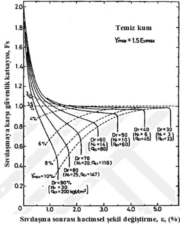
Şekil 4.10: Çeşitli Sıvılaşma için faktörlerine karşılık gelen hacimsel yoğunlaştırılmış şekil değiştirme (Ishihara ve Yoshimine 1992)
