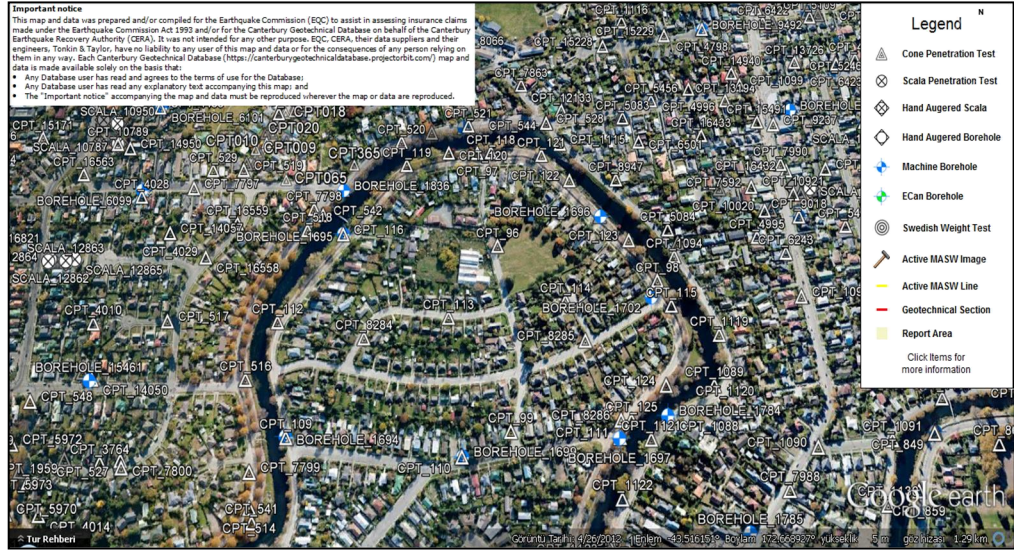
Şekil 2.9: CPT yapılan noktalara örnek bir alan
