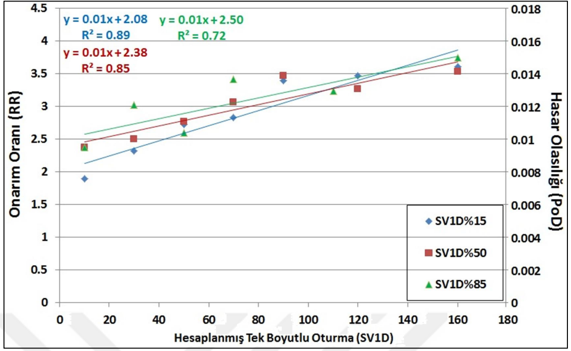
Şekil 5.16: AC tipi borular için S_{V1D} %15, %50 ve %85 kullanılarak hesaplanan hasar ilişkileri
