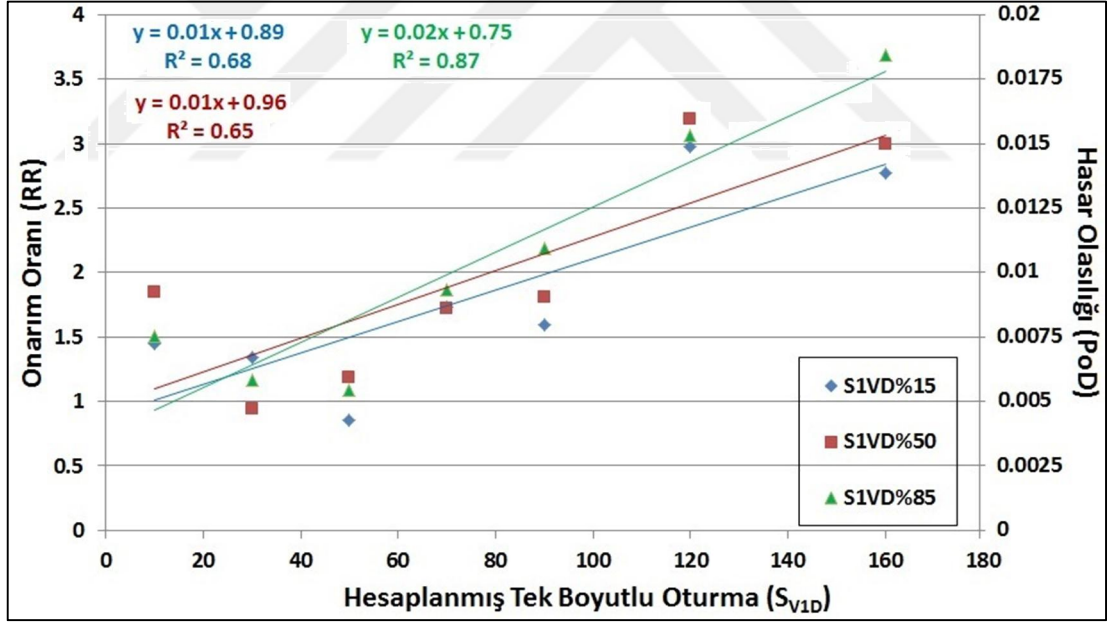
Şekil 5.17: CI tipi borular için S_{V1D} %15, %50 ve %85 kullanılarak hesaplanan hasar ilişkileri
