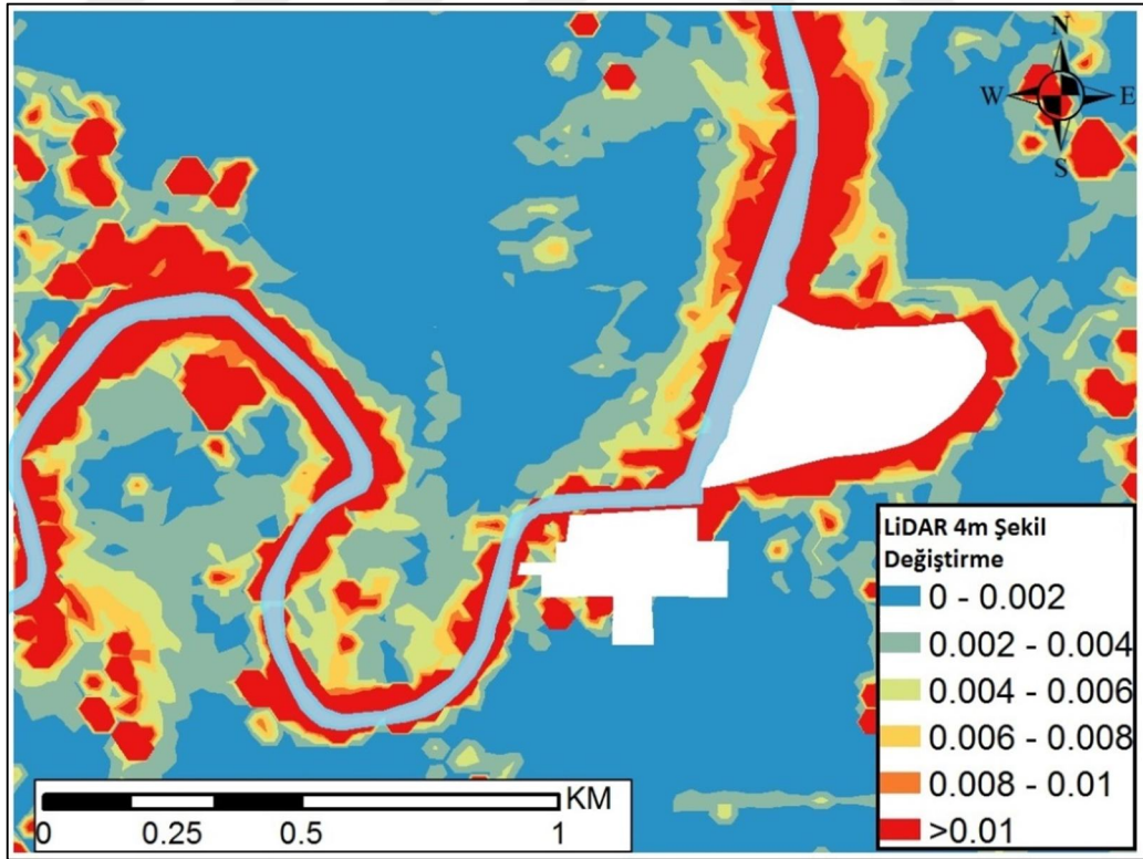
Şekil 3.34: LiDAR 4 m yatay şekil değiştirme haritası
