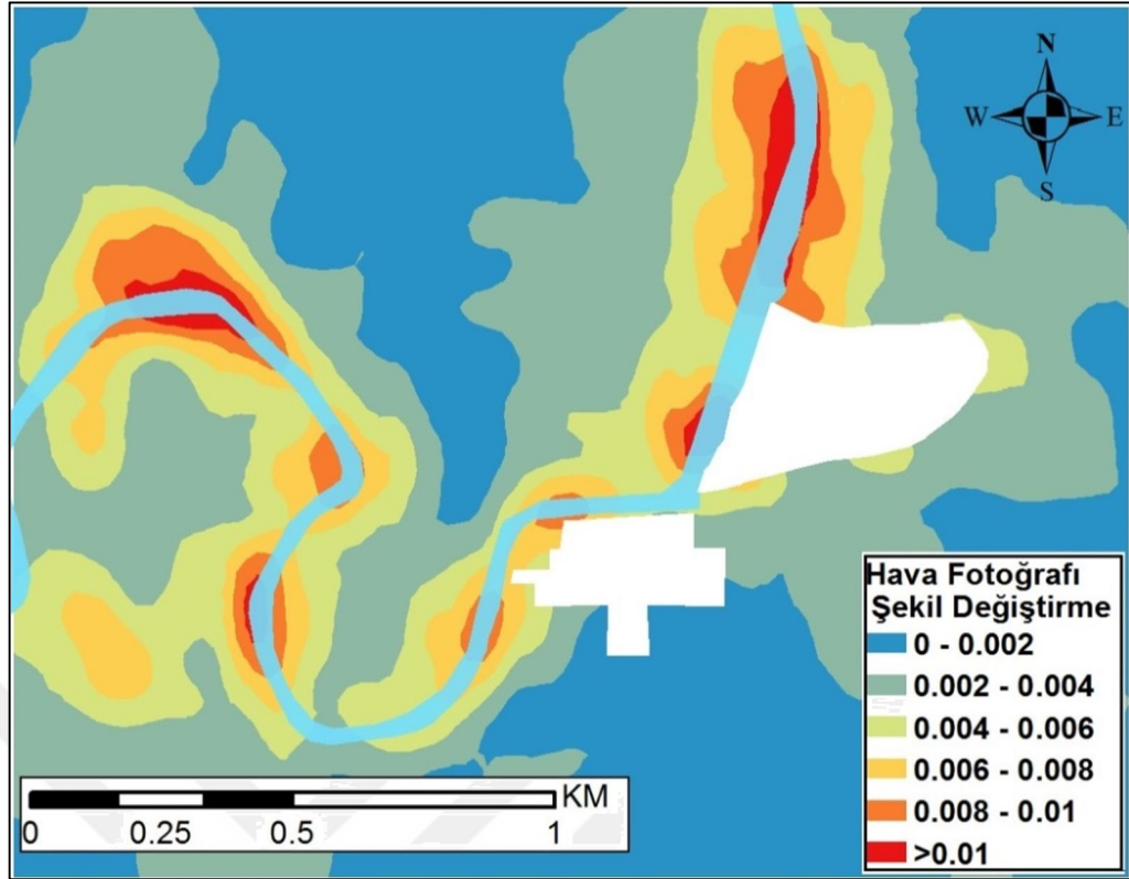
Şekil 3.35: Hava fotoğrafı yatay şekil değıştirme haritası
