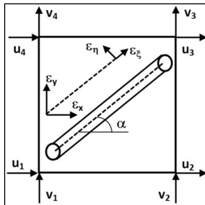
Şekil 3.32: Boru doğrultusunda ve bu doğrultuya dik şekil değiştirmelerin gösterimi.
