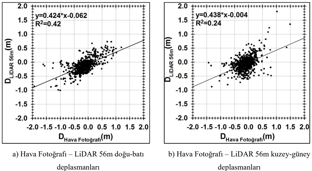
Şekil 3.10: Hava Fotoğrafı LiDAR 56 m deplasmanları.
