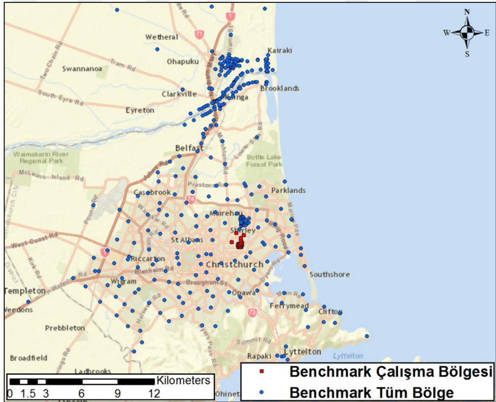
Şekil 3.9: Benchmark ölçümleri.
