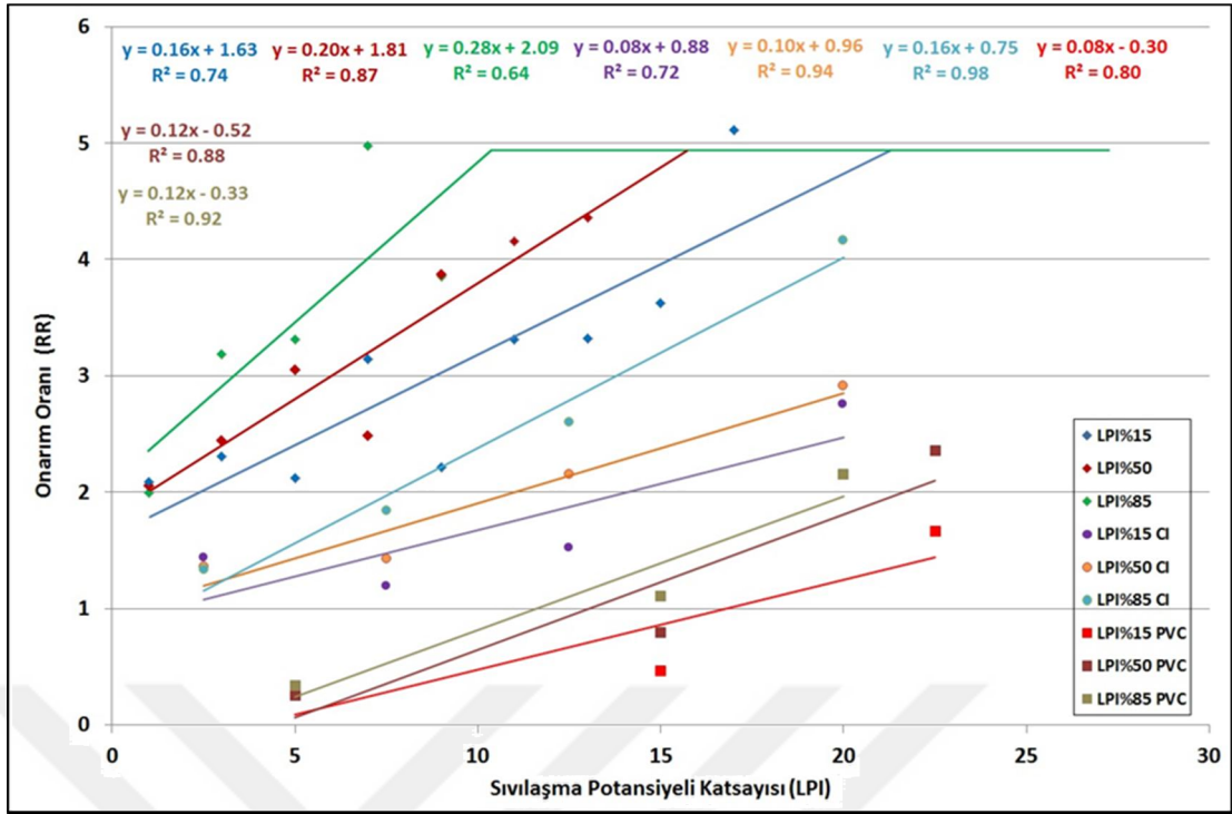
Şekil 5.22: LPI parametresi kullanılarak hesaplanan hasar ilişkileri
