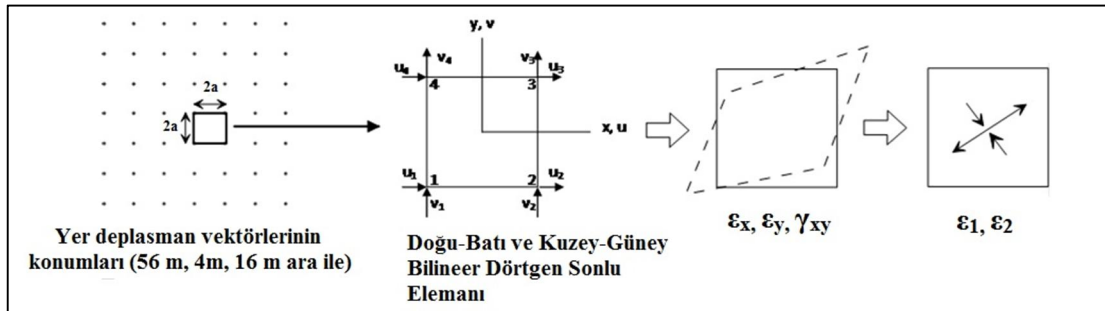
Şekil 3.31: Yatay yer değiştirmeler yardımıyla yatay şekil değiştirmelerin ve asal şekil değiştirmelerin hesaplanma süreci
