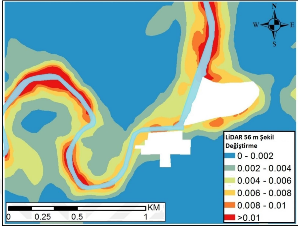
Şekil 3.33: LiDAR 56 m yatay şekil değiştirme haritası
