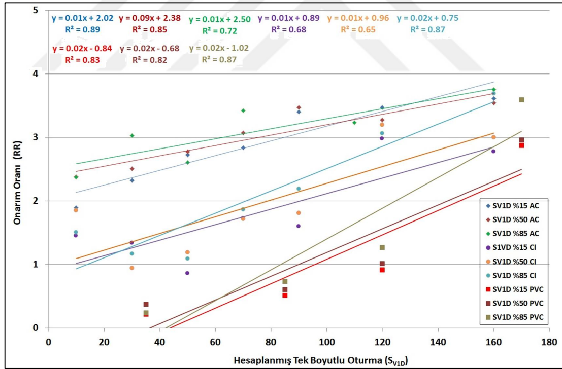
Şekil 5.23: S_{VID} parametresi kullanılarak hesaplanan hasar ilişkileri
