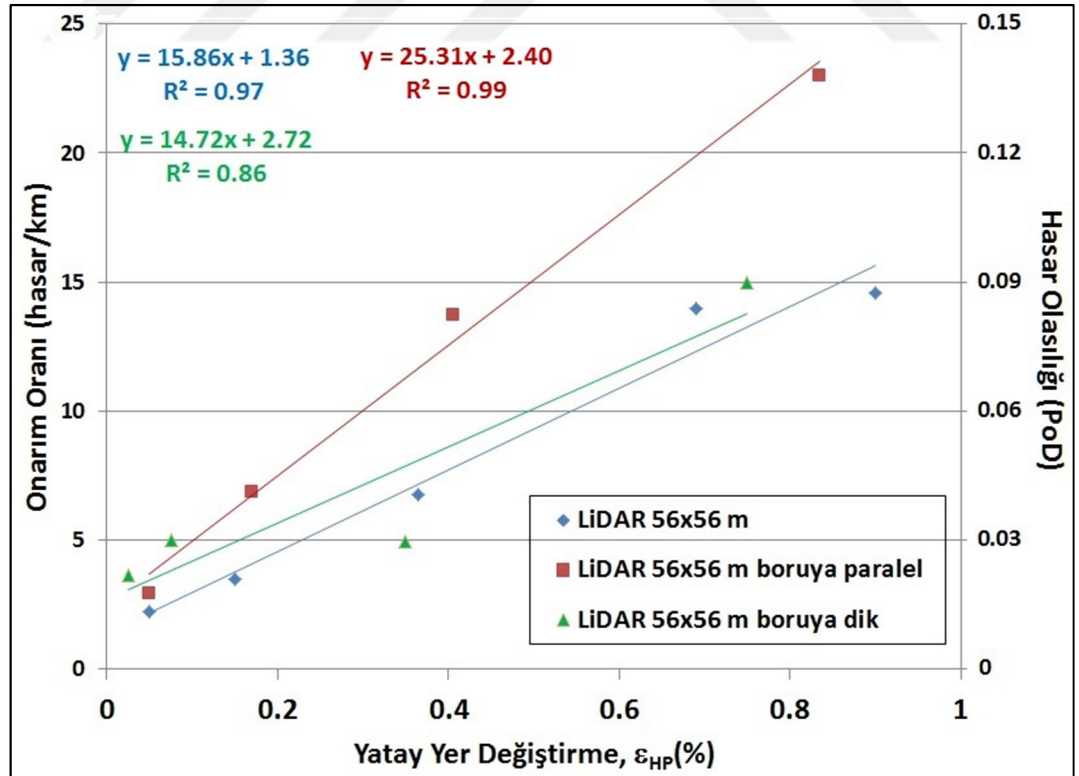
Şekil 5.9: CI tipi borular için hava fotoğrafı, LiDAR 56m ölçümleri ile hesaplanan hasar ilişkileri (en büyük asal yatay yer değiştirme, boruya paralel ve boruya dik)
