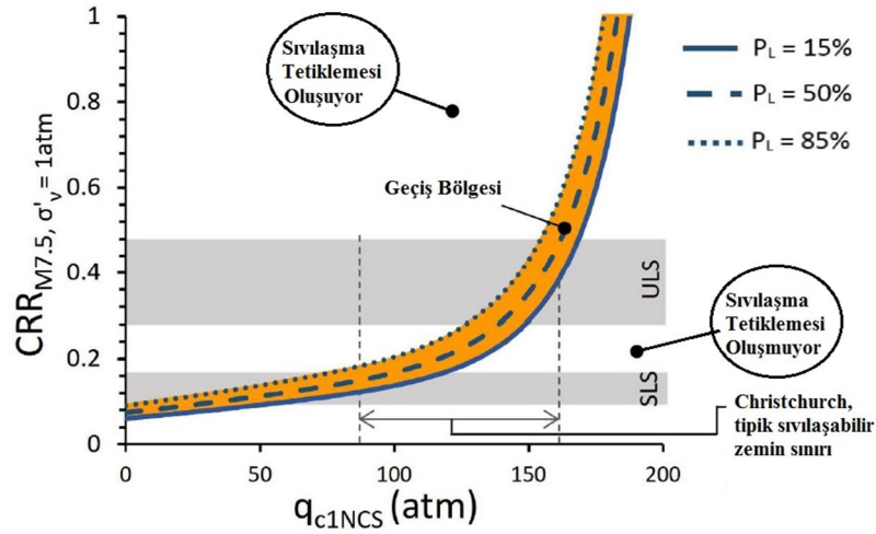
Şekil 4.6: CRR ve q_{1NCS} 'ye bağlı P_L = 15\% , 50\% ve 85\% eğrileri (Boulanger ve Idriss 2014).
