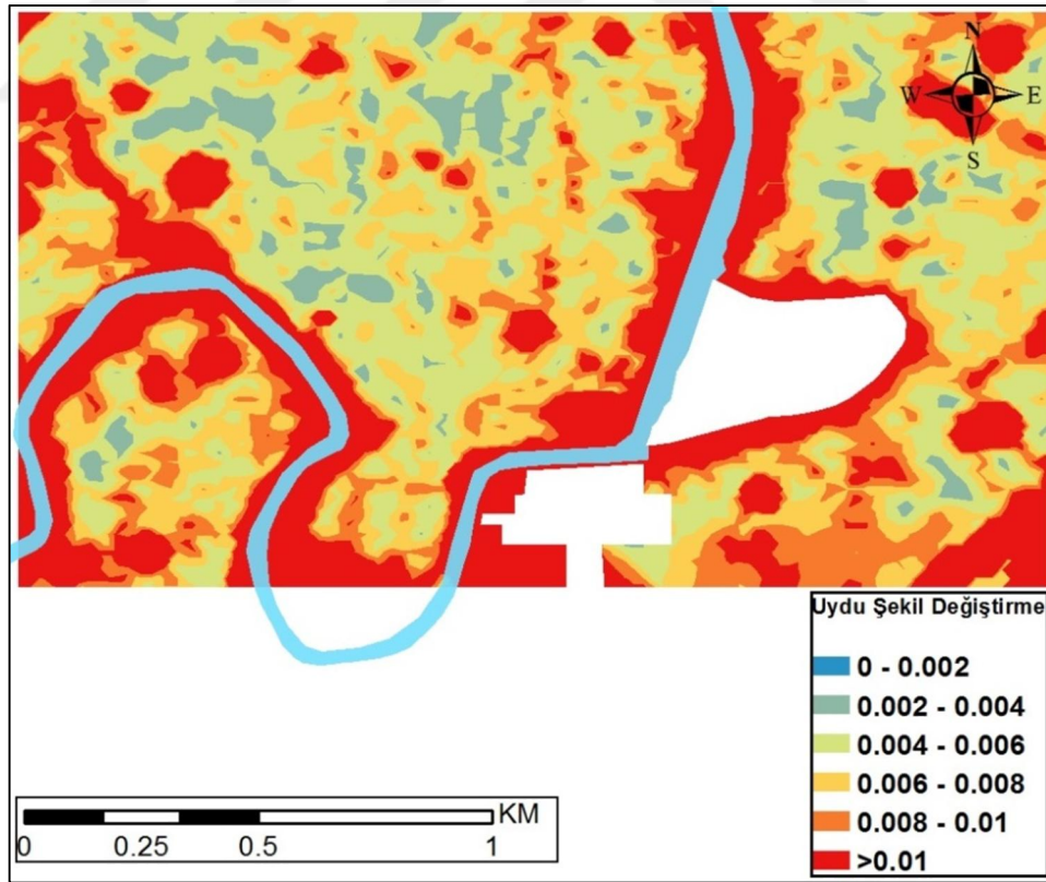
Şekil 3.36: Uydu ölçümleri yatay şekil değıştirme haritası
