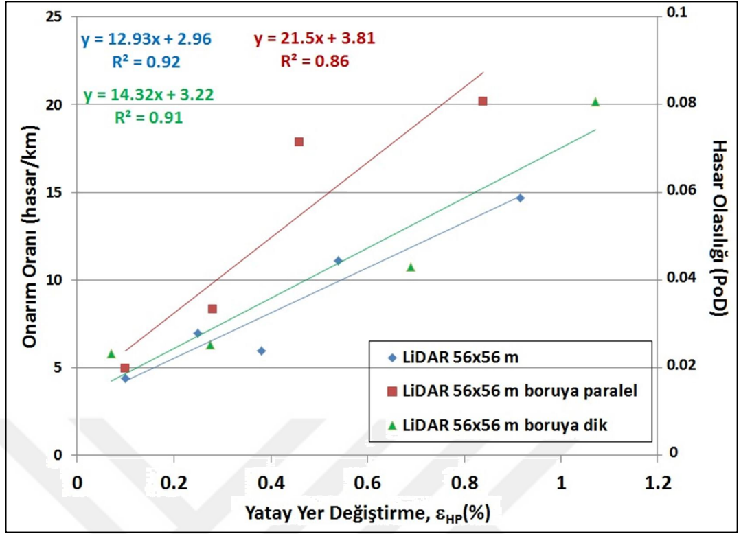
Şekil 5.8: AC tipi borular için hava fotoğrafı, LiDAR 56m ölçümleri ile hesaplanan hasar ilişkileri (en büyük asal yatay yer değiştirme, boruya paralel ve boruya dik)
