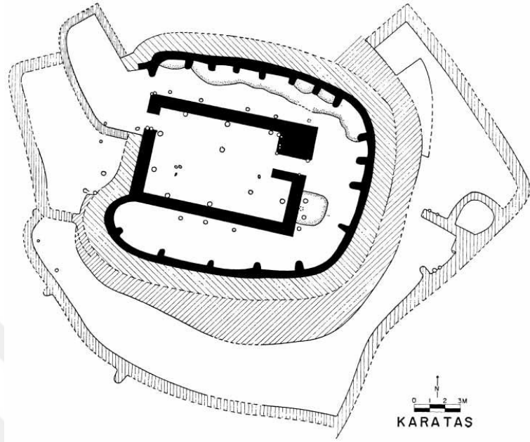
Çizim 3: Karataş-Semayük – I. tabakadaki binanın planı (Mellink ve Angel 1966, 247 çiz. 2)
