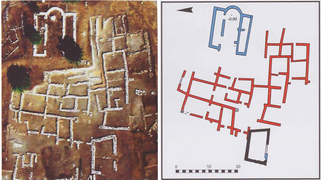
Resim 44: Bademağacı Höyüğü – Çok Odalı Yapı fotoğrafı ve planı (Duru 2016, 88 res. 247-248)
