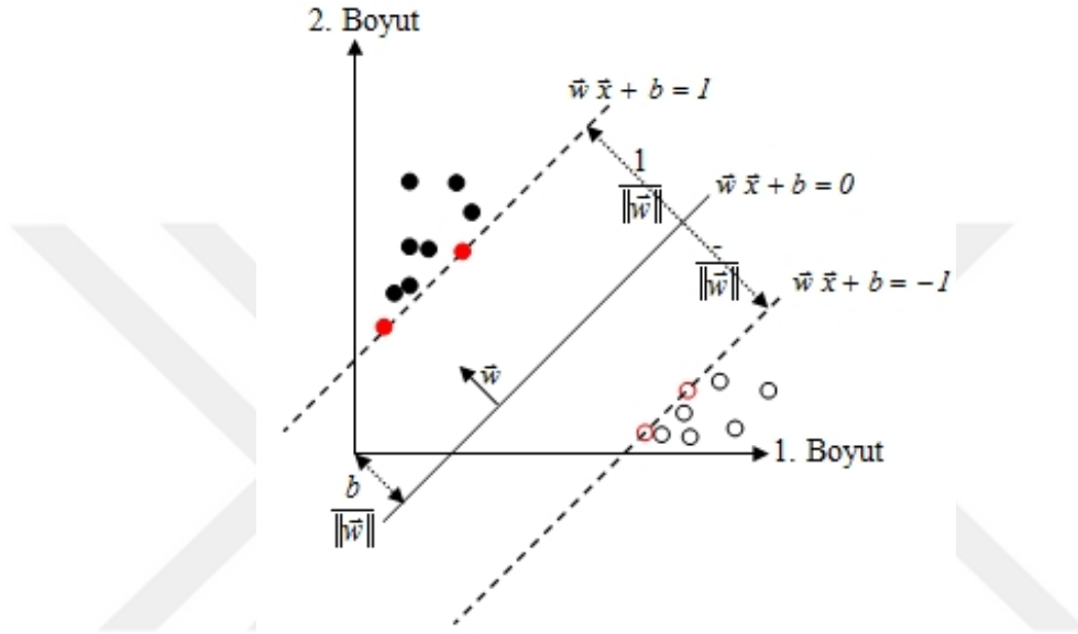
Şekil 7. 5. SVM sınıflandırıcısı çalışma prensibi
