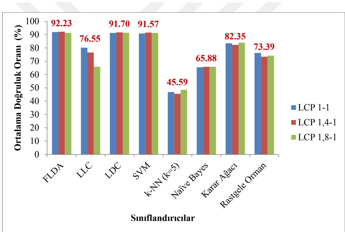
Şekil 9. 1. 108-boyutlu LCP-tabanlı öznitelik vektörlerinin 3-sınıflı sınıflandırılma çalışmasından elde edilen sonuçlar
