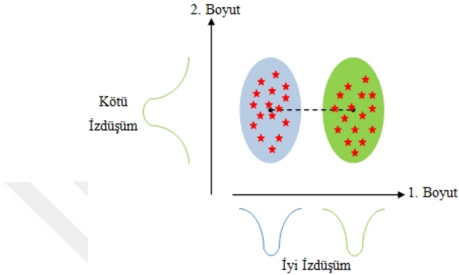
Şekil 7. 4. FLDA sınıflandırıcısı çalışma prensibi
