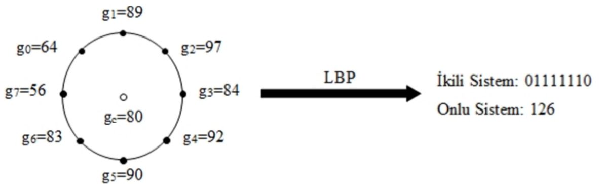
Şekil 6. 2. Gri seviye bir imgenin LBP gösterimi
