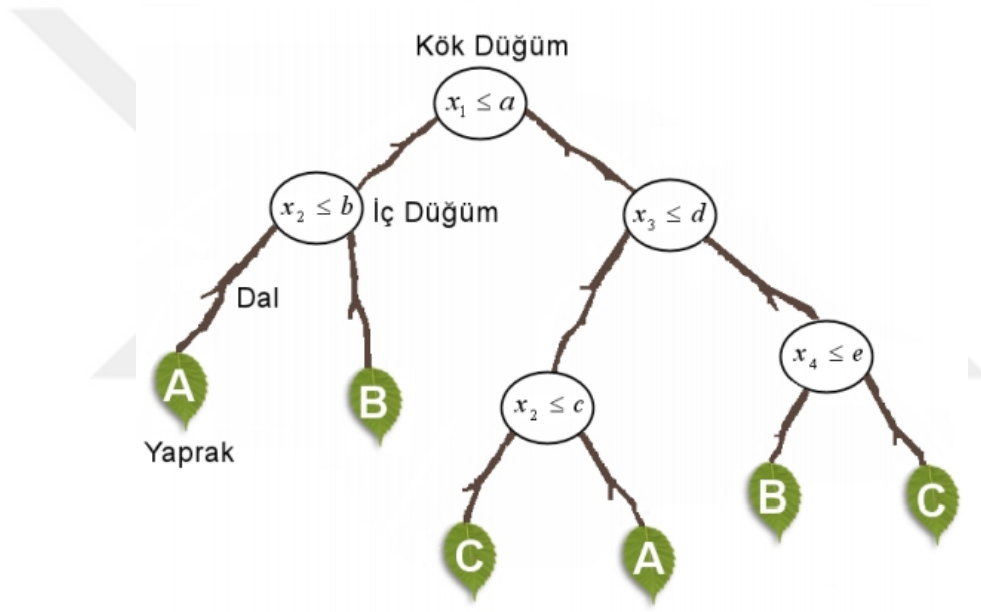
Şekil 7. 2. Karar ağacı sınıflandırıcısı çalışma prensibi (Kavzoğlu ve Çölkesen'den, 2010)
