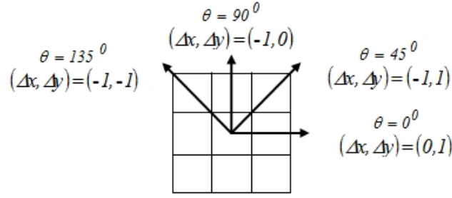
Şekil 6. 3. GLCM gösterimi
