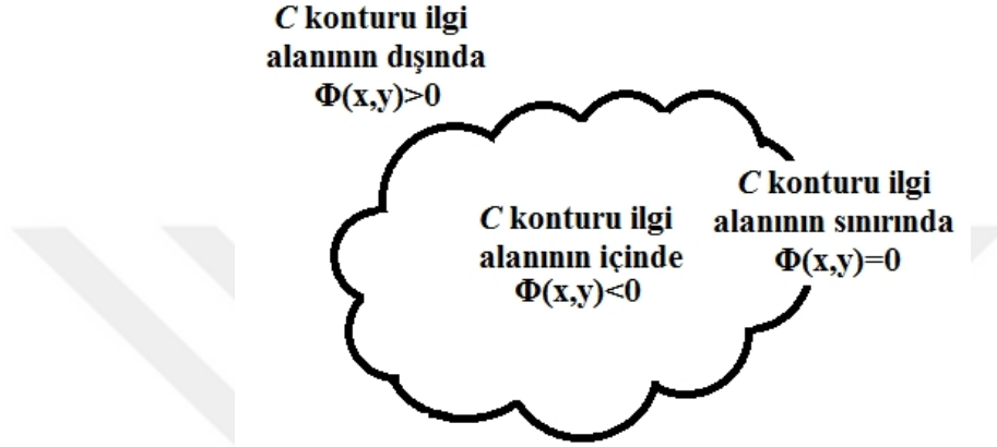
Şekil 5. 1. Kontur gelişimi
