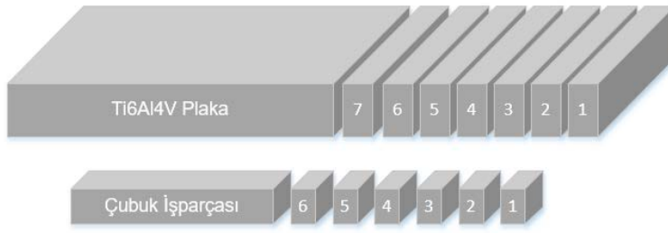
Şekil 7.1. Hazırlanan çubuk işparçası ve kesilmiş işparçalarının şematik görünümü
