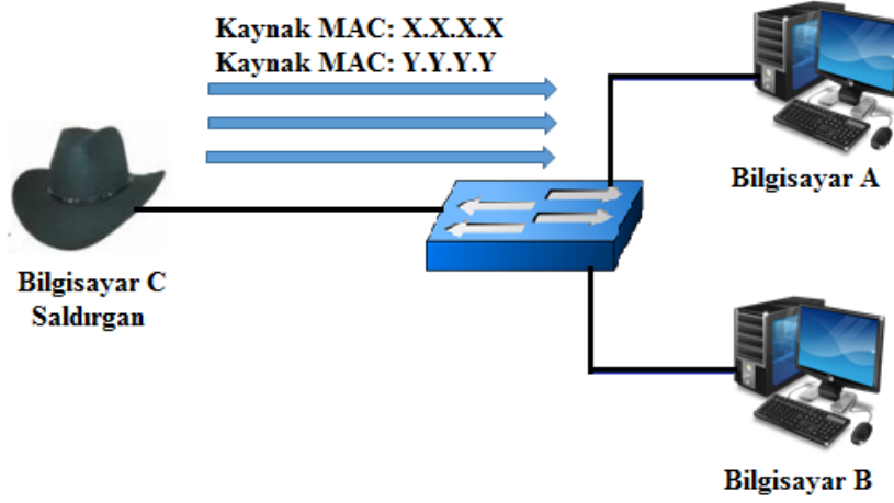
Şekil 2.17 MAC flooding saldırısı
