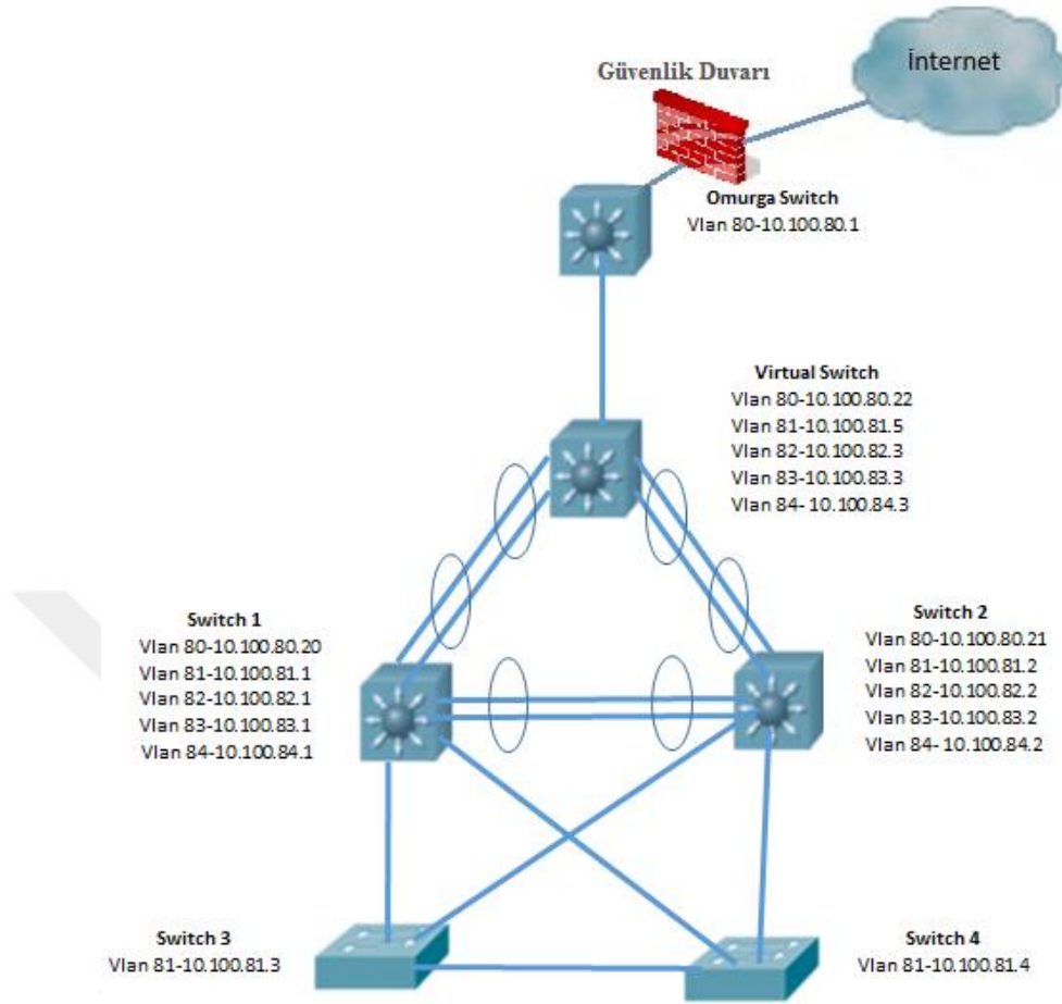
Şekil 3.5 Anahtar (switch) VLAN ve IP yapıları
