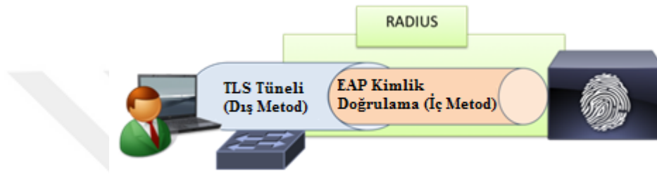
Şekil 2.16 EAP - TTLS bağlantısı (İnt.Kyn.28).
