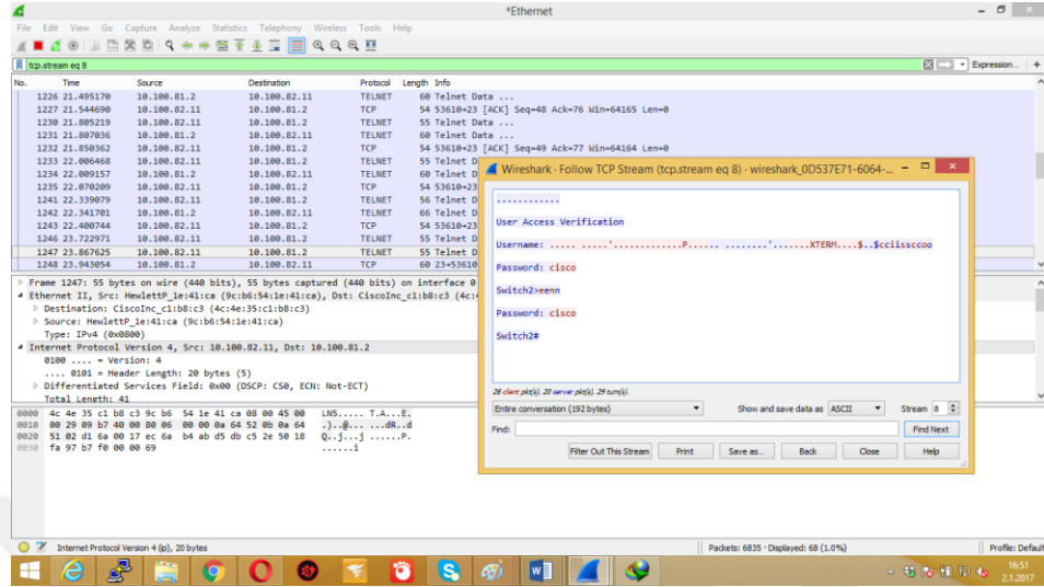
Resim 4.5 Paket analizi
