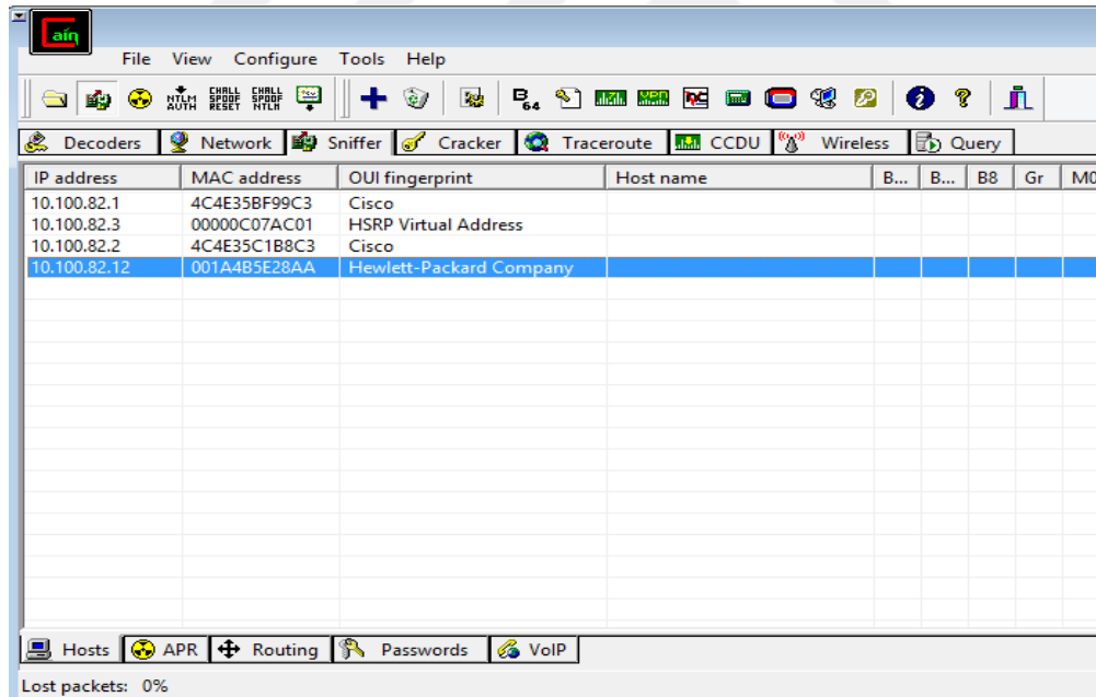
Resim 2.6 Cain&Abel programı
