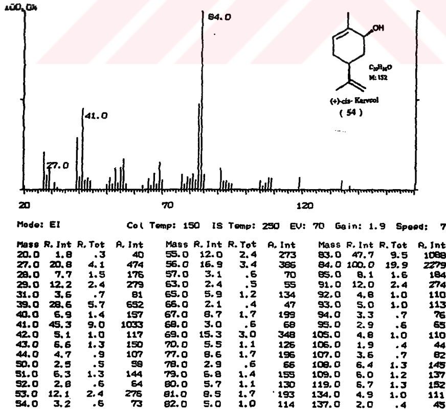
Şekil 4.9 cis-Karveol 'ün Kütle Spektrumu
