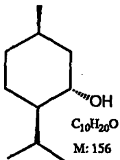
(+)- İzomentol ( 26 )
