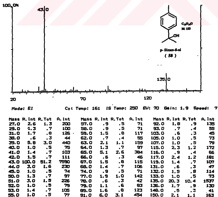
Şekil 4.13 p-Simen-8-ol 'ün Kütle Spektrumu
