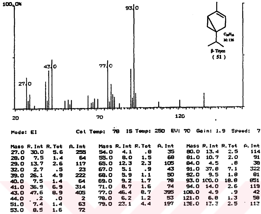
Şekil 4.6 \beta -Tuyen 'in Kütle Spektrumu
