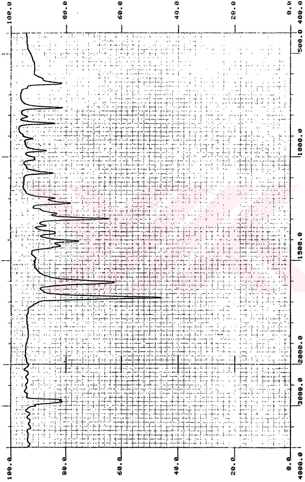
Şekil 4.21 Piperitenonoksit'in IR Spektrumu
