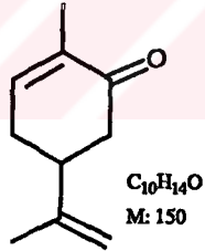
Karvon ( 23 )
