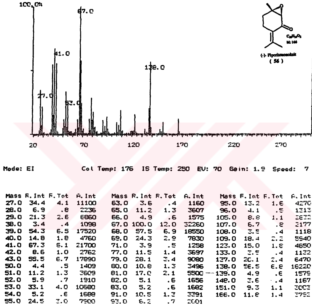
Şekil 4.27 Piperitenonoksit'in Kütle Spektrumu
