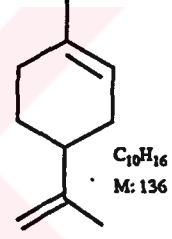
Limonen ( 6 )
