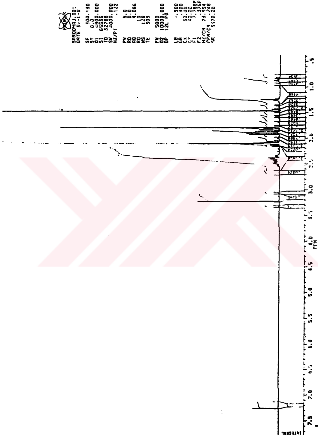
Şekil 4.22 Piperitenonoksit'in ^1\text{H} -NMR Spektrumu
