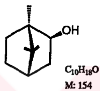
(+)- İzoborneol ( 19 )
