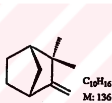
Kamfen ( 5 )
