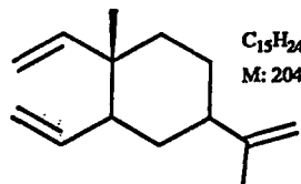
d-β- Elemen ( 41 )
