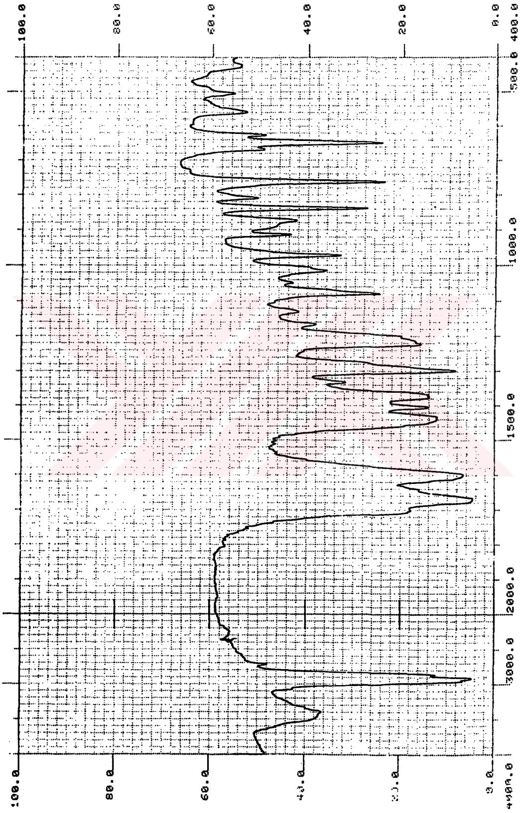
Şekil 4.2 Buhar Distilasyonu ile Elde Edilen Uçucu Yağın IR Spektrumu
