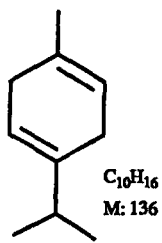
\gamma Terpinen ( 16 )
