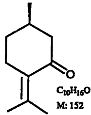
(+)- Pulegon ( 31 )
