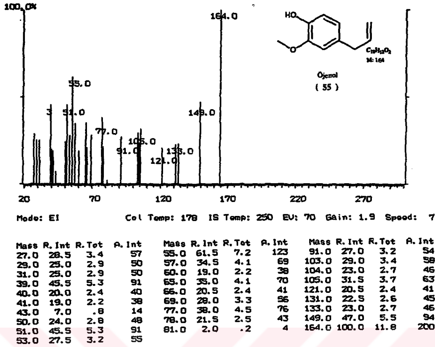
Şekil 4.10 Öjenol 'ün KütLe Spektrumu
