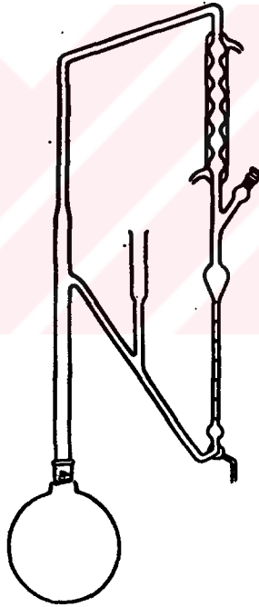
Şekil 3.2 Clevenger Apareyi
