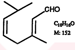
Citral ( 35 )
