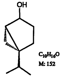
Sabinenhidrat ( 33 )
