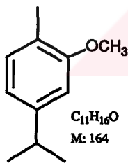
Metilkarvakrol ( 22 )
