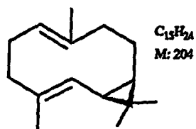
Bisiklogermakren ( 44 )
