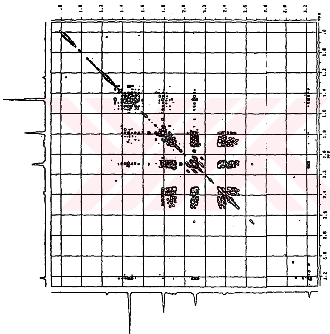
Şekil 4.23 Piperitenonoksit'in COSY Spektrogramu
