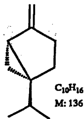
(+)- Sabinen ( 13 )
