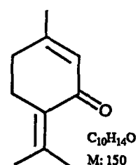
Piperitenon ( 29 )
