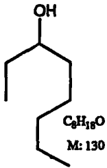
3- Oktanol ( 1 )
