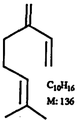
Mirsen ( 7 )
