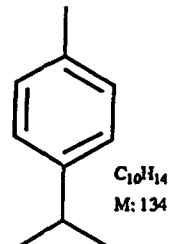
p- Simen ( 14 )
