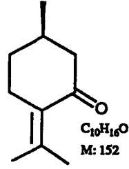
d- Pulegon ( 32 )
