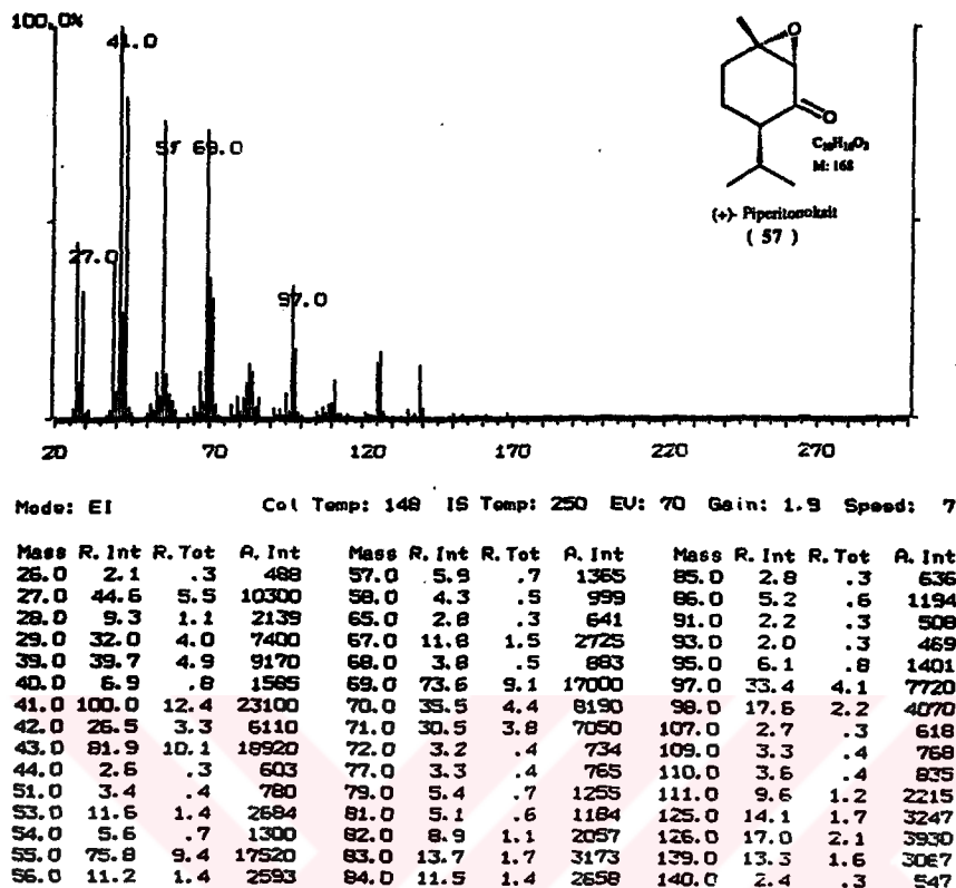
Şekil 4.12 Piperitonoksit - II 'nin Kütle Spektrumu
