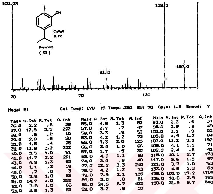
Şekil 4.8 Karvakrol 'ün Kütle Spektrumu
