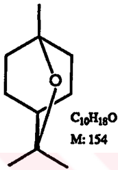
1,8- Sineol ( 34 )
