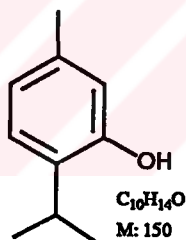
Timol ( 39 )
