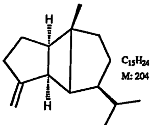
β- Burbonen ( 40 )
