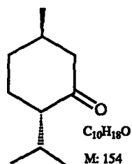
d- Menton ( 27 )
