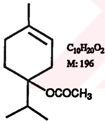
Terpinilasetat ( 38 )
