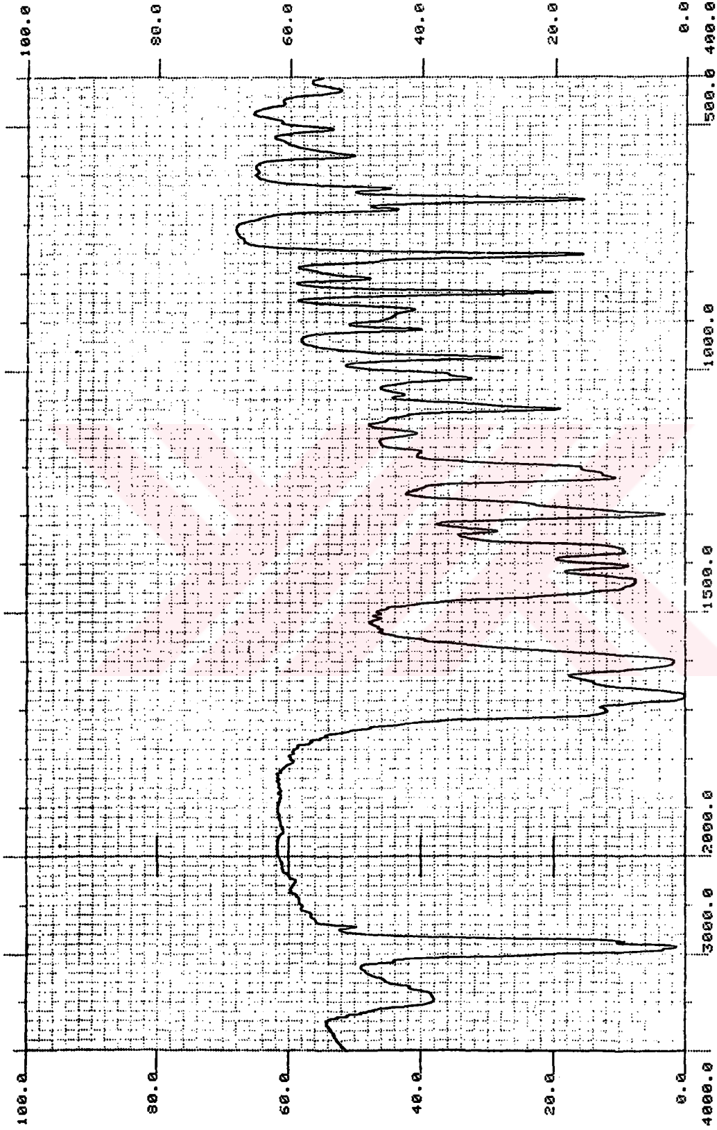
Şekil 4.1 Su Distilasyonu ile Elde Edilen Uçucu Yağın IR Spektrumu
