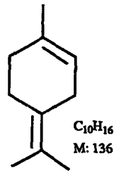
Terpinolen ( 17 )
