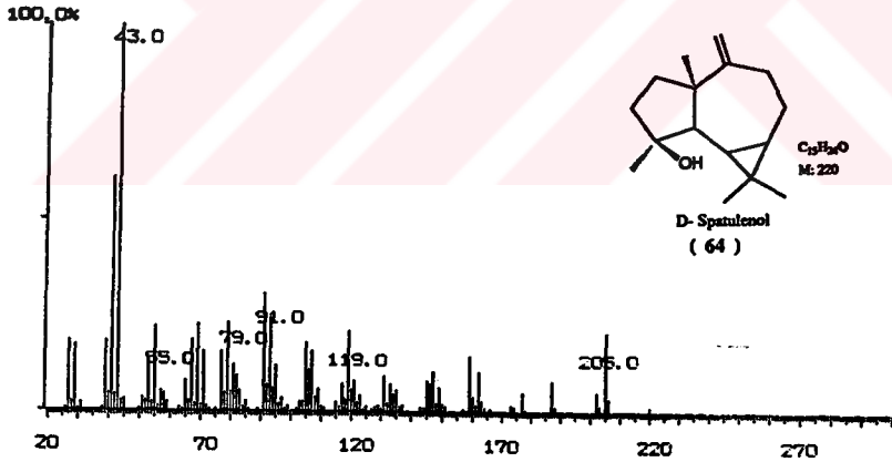
Şekil 4.18 α-Kubeben 'in Kütle Spektrumu
