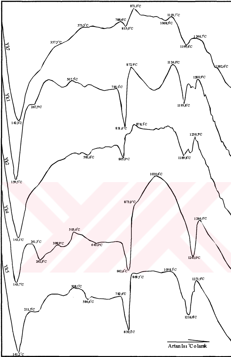
Şekil 3.5.b: Sazak Formasyonuna ait Kırmızı renkli magnezyumlu Kiltaşlarının DTA Grafikleri
