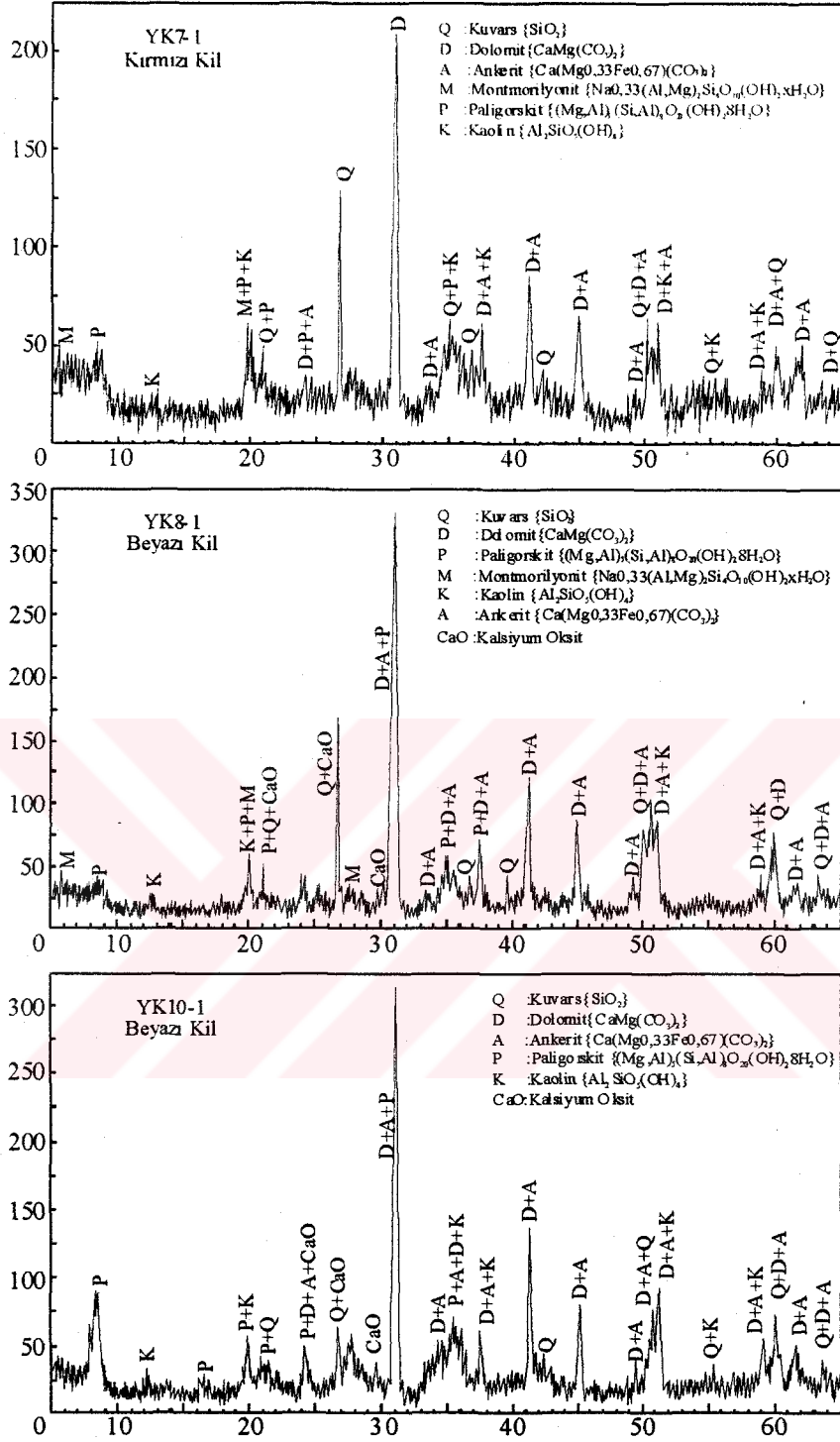
Şekil 3.4.b: Magnezyumlu Kiltaşlarının çekilen difraktogram.
