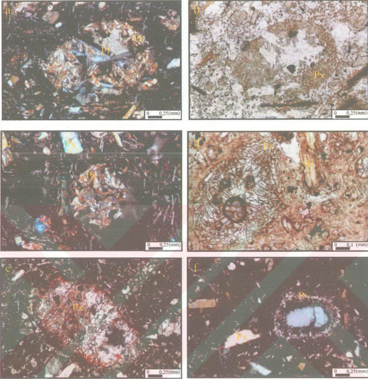
Şekil 3.17: Bazı lav örneklerinde tespit edilen mikro anklavlar ve ksenokristaller.
