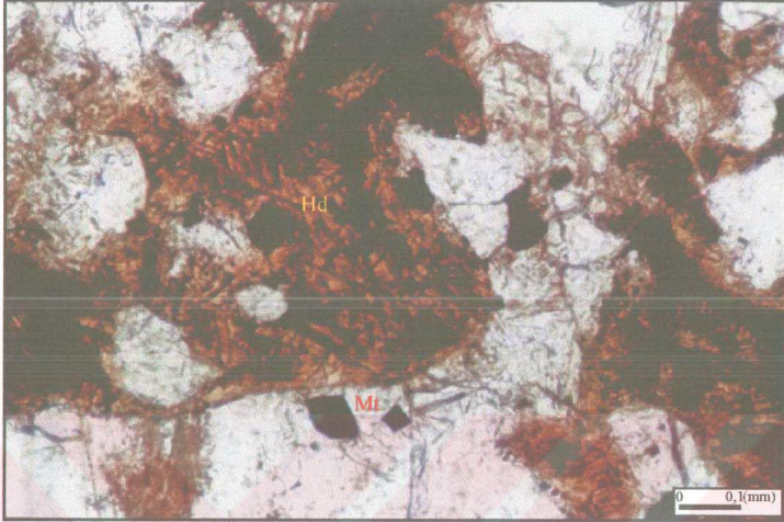
Şekil 3.13: Hornblend ve manyetit minerallerinin görünümü (Tek Nikol).
