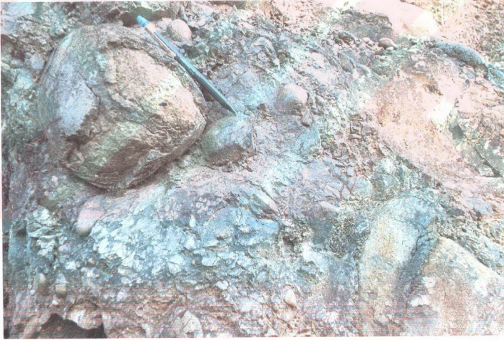
Şekil 2.11: Ofiyolitik elemanlardan oluşan blok ve iri çakıl içerikli Karadere Formasyonunun arazide görünümü.
