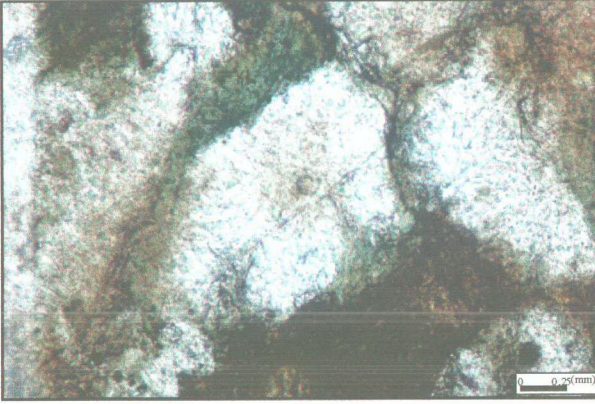
Şekil 3.2: Metadolerit dayklarında gözlenen kloritleşme (Çift Nikol).
