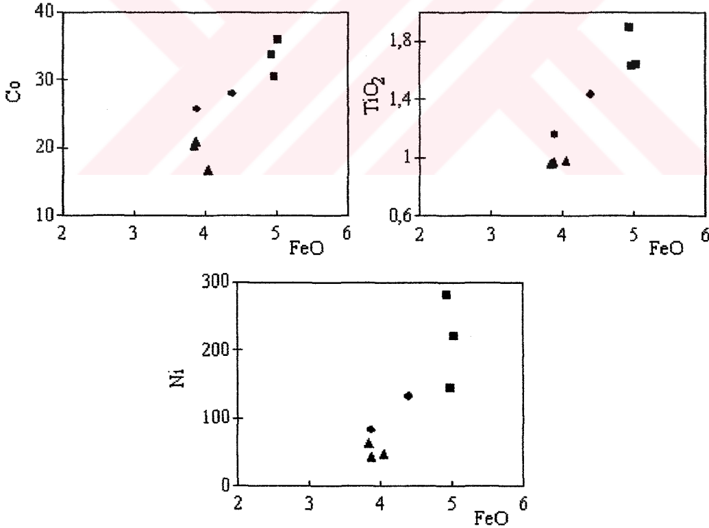
Şekil 4.13: Lavların FeO-Ni, FeO-Co ve FeO- \text{TiO}_2 diyagramları.
