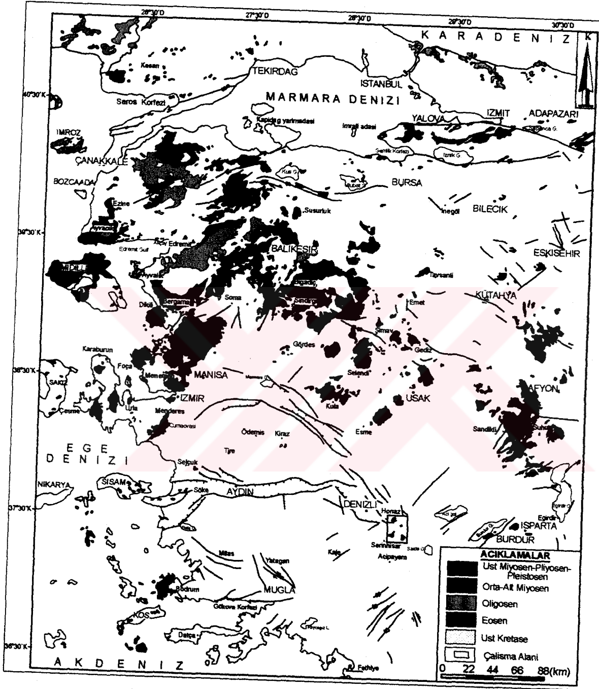
Şekil 1.3: Batı Anadolu volkanitleri yaş haritası
