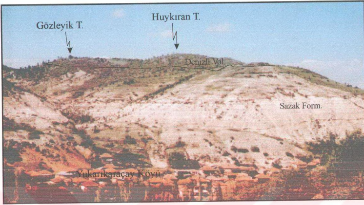
Şekil 2.15: Yukarıkaraçay kuzeyindeki Gözleyik tepedeki lavların görünümü.
