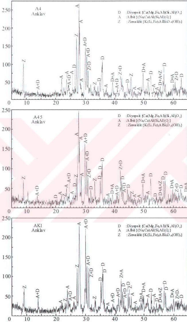
Şekil 3.16.b: Anklavların XRD incelemeleri
