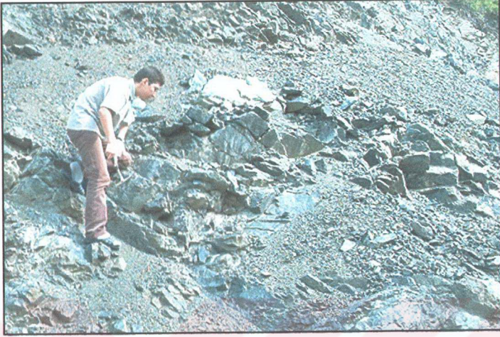
Şekil 2.9: Çarşafdüzü mevkiî doğusunda bulunan Honaz Ofiyolitindeki serpantinleşmiş Harzburgitlerin genel görünümü.
