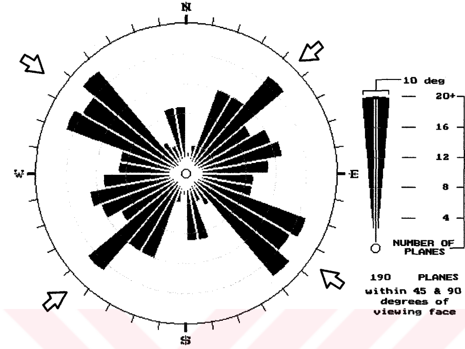
Şekil 5.7: Mesozoyik yaşlı kireçtaşlarından alınan 232 adet çatlak ölçümü sonucu oluşturulan doğrultu gül diyagramı.
