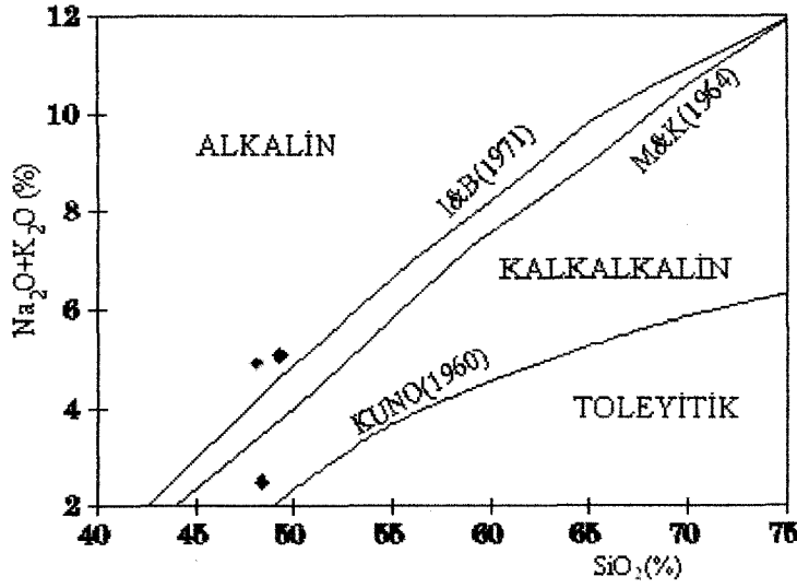
Şekil 4.21: Anklav örneklerinin toplam alkali silika diyagramı.
