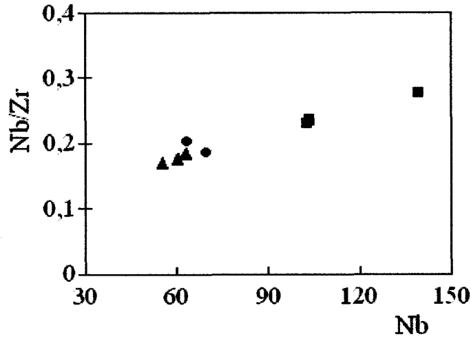
Şekil 4.19: Nb-Nb/Zr diyagramı.
