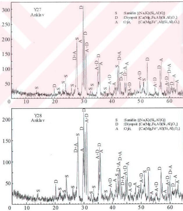
Şekil 3.16.a: Anklavların XRD incelemeleri
