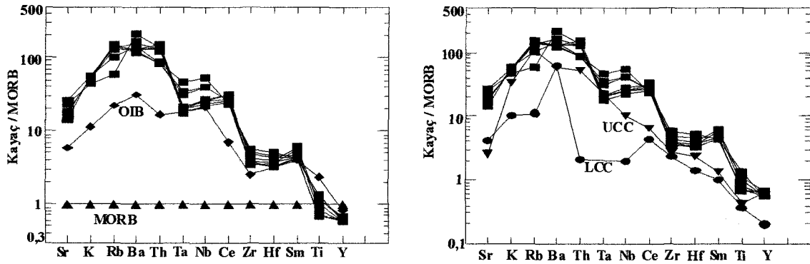
Şekil 4.12: Denizli Volkanitleri lavlarının kayaç/MORB spider diyagramı (■:Denizli volkanitleri, ◆:Okyanus adası bazaltı (OIB), ▲:Okyanus ortası sırt bazaltları (N tipi MORB) ▼:Üst Kıta kabuğu (UCC), ●:Alt kıta Kabuğu (LCC)).
