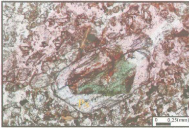
Şekil 3.10: (a) Piroksen kristalleri ortası kloritleşmiş (Tek Nikol) ve (b) Piroksen içinde piroksen kapanımı (Çift Nikol) (Px:piroksen)
