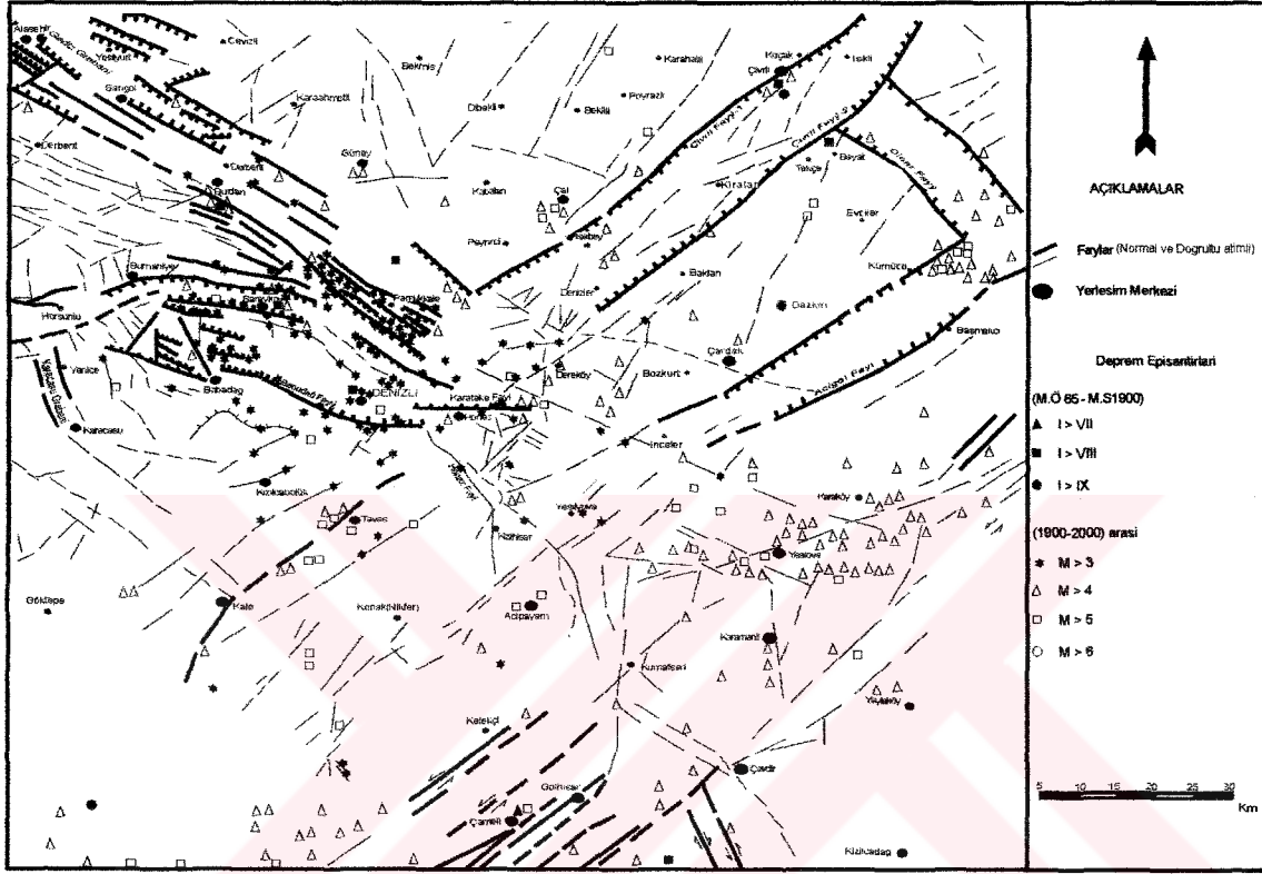
Şekil 5.2: Denizli ve yakın çevresinin sismotektonik haritası (Özpınar ve Gökgöz, 1999)
