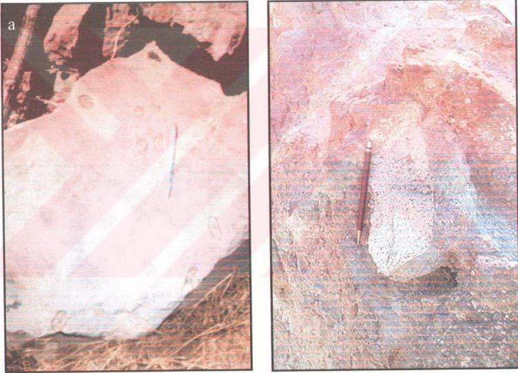
Şekil 2.22: Lavlar içerisindeki elipsoidal şekilli anklavlar (a) ve kuvarsit anklavı (b).
