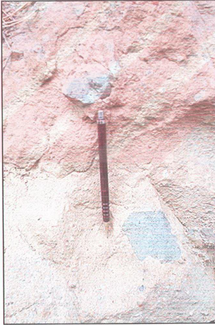
Şekil 2.24: Yeşilyuva kuzeyindeki Bilmecegürü mevkiindeki Kızılburun Formasyonu içindeki farklı boyutta bazaltik lav parçalarının görünümü.
