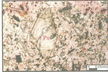
Şekil 3.7: Trakiandezitlerde piroksen minerallerinde gözlenen zonlu doku. (a: Çift Nikol - b: Tek Nikol)
