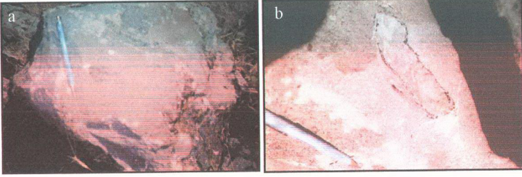
Şekil 2.21: Lavlar içerisindeki diyopsitit anklavı (a) ve açık yeşil renkli anklav (b)
