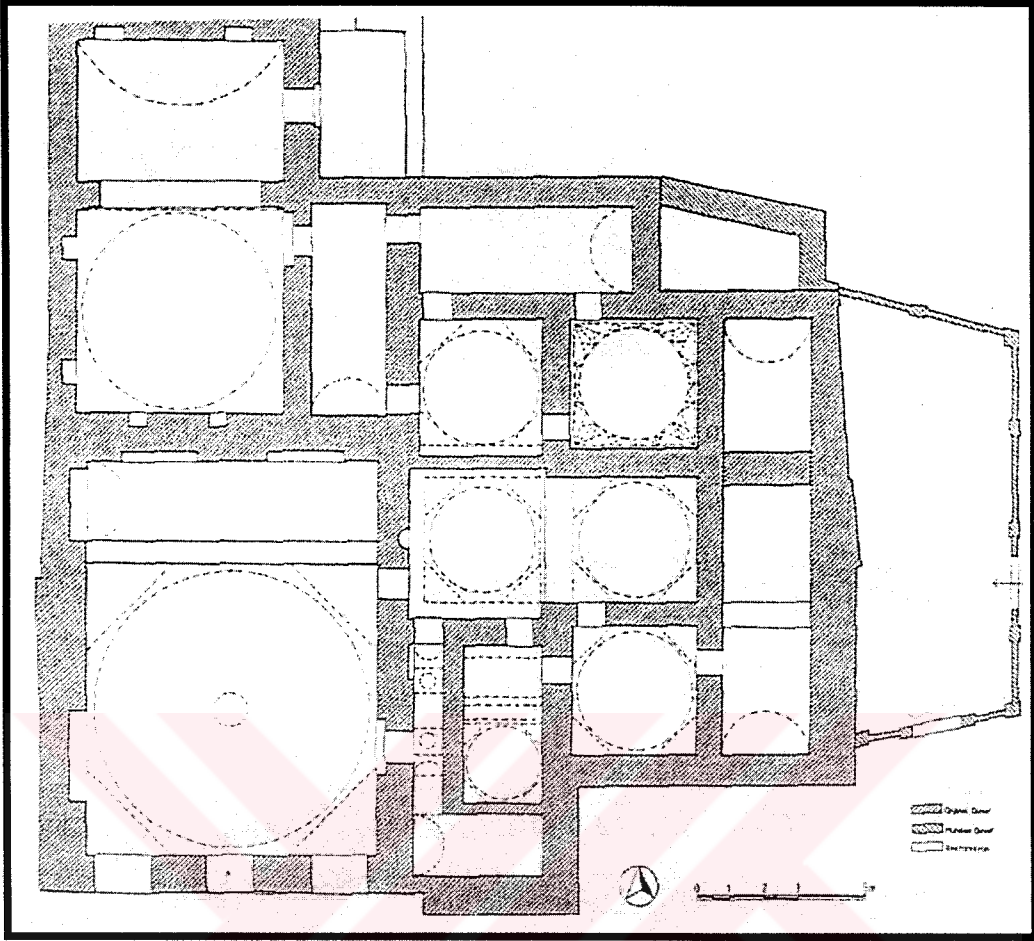
Harita 6. 3 Sarı Ahmet Paşa Hamamı Plan Şeması (Ünal, 1998, s.85)
