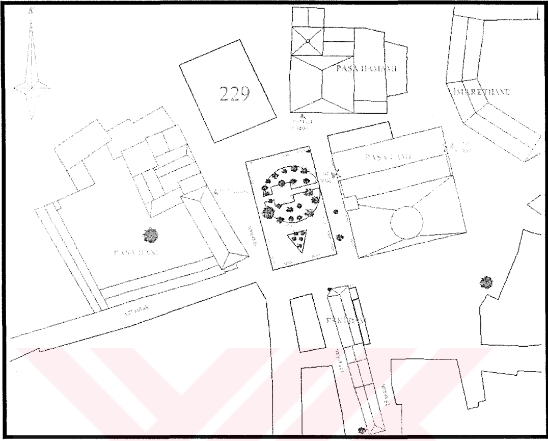
Çizim 6.1 Sarı Ahmet Paşa Külliyesi Vaziyet Planı
