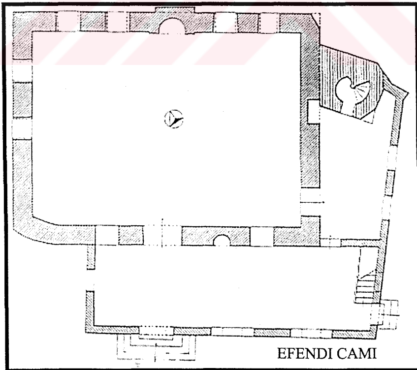
Harita 4. 10 Efendi Cami Plan Şeması (Ünalın, 1998, s.50)
