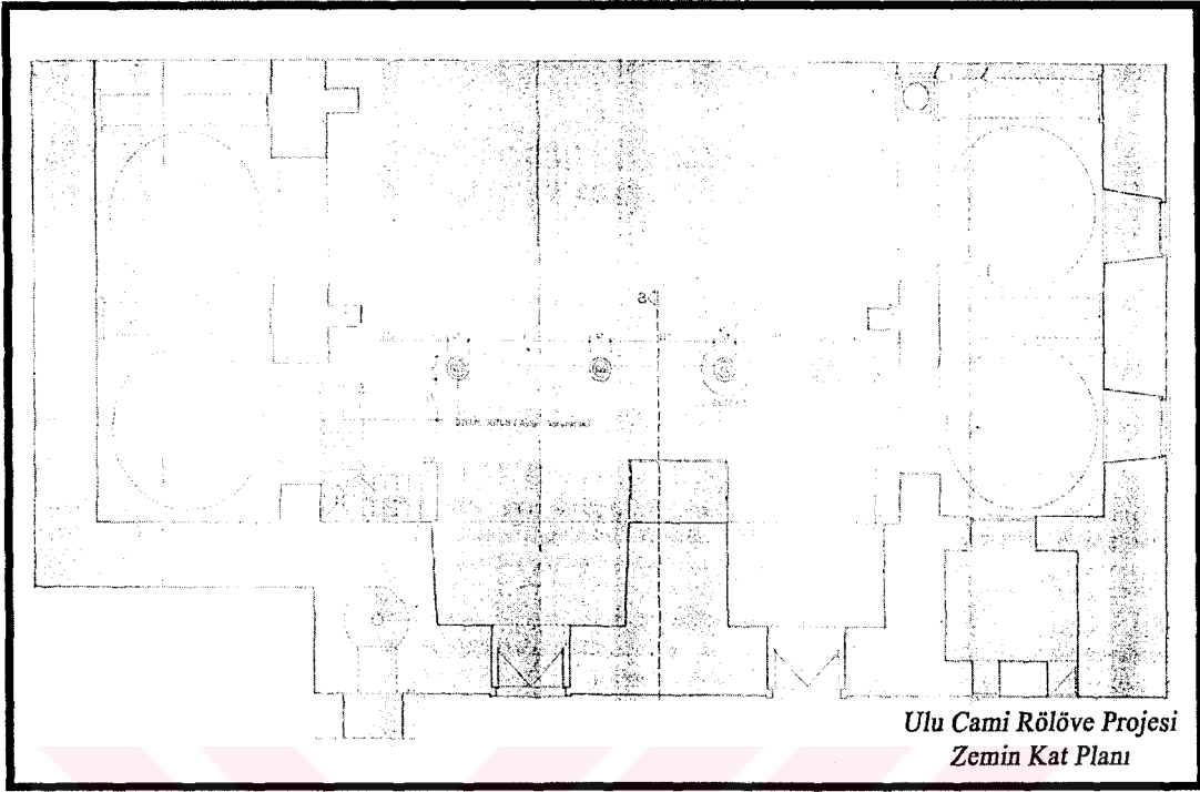
Harita 4. 4 Ulu Cami Zemin Kat Planı (İzmir Vakıflar Bölge Müdürlüğü)
