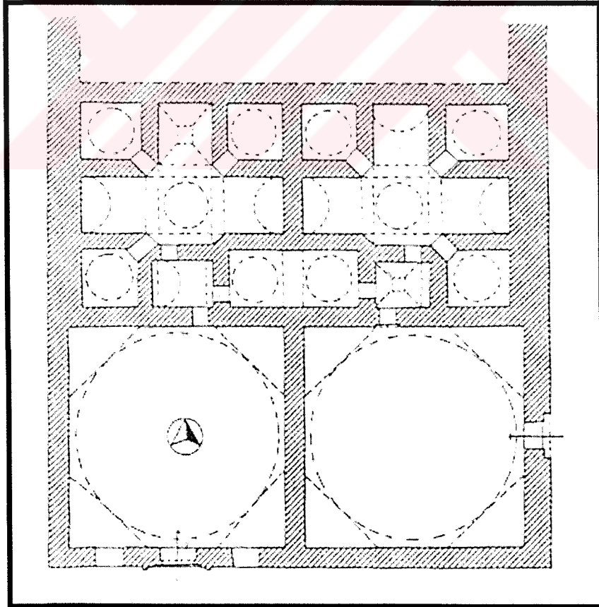
Harita 4. 14 Gülruh Sultan (Yeni) Hamamı Plan Şeması (Ünalan, 1998, s.90)
