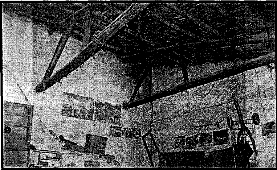
Resim 6. 42 Han Avlusunun Batı Cephesinde Bulunan Nalbandın Tavanı
