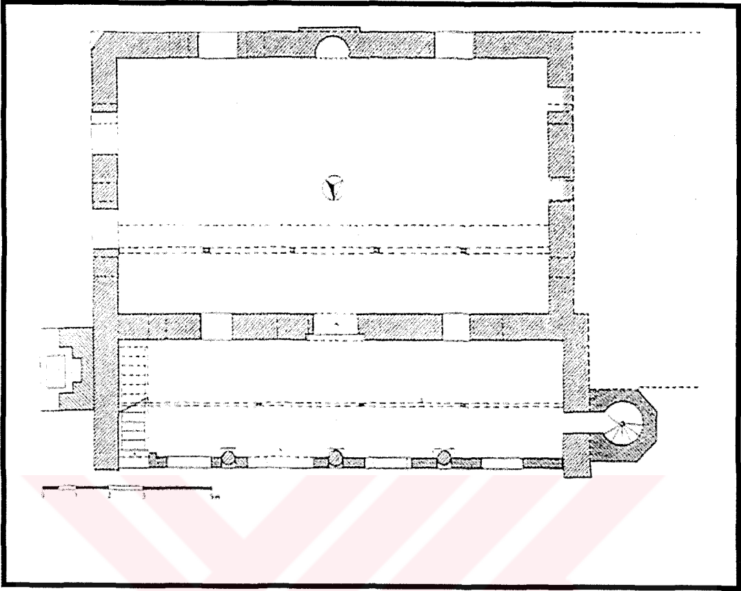
Harita 4. 8 Köfünlü Kara Mehmet Cami Plan Şeması
