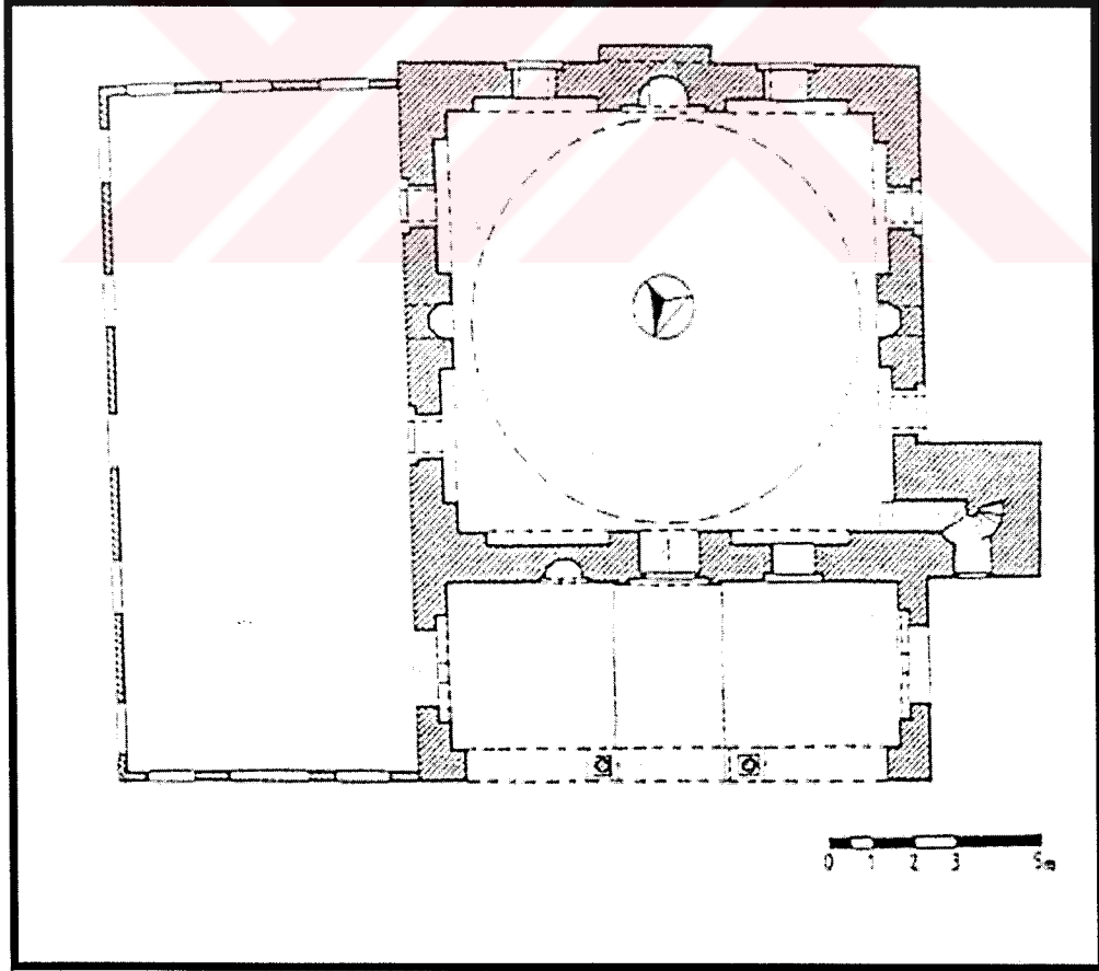
Harita 4. 9 Gülruh Sultan (Yeni) Cami Plan Şeması (Ünalan, 1998, s.21)
