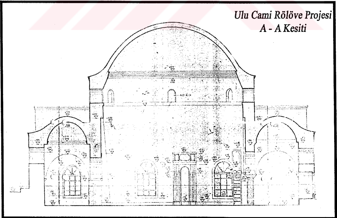
Harita 4. 6 Ulu Cami Kesiti (İzmir Vakıflar Bölge Müdürlüğü)
