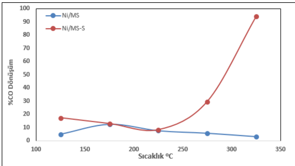
Şekil 6.24. Ni/MS ve Ni/MS-S katalizörlerinin CO metanlaşma reaksiyonu için sıcaklığa bağlı aktivite sonuçları
