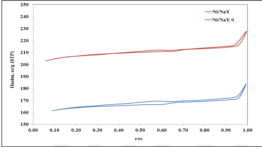
Şekil 6.11. Farklı hazırlama yöntemi ile sentezlenmiş NaY zeolit destekli nikel içeren katalizörlere ait N 2 adsorpsiyon/desorpsiyon izotermi
