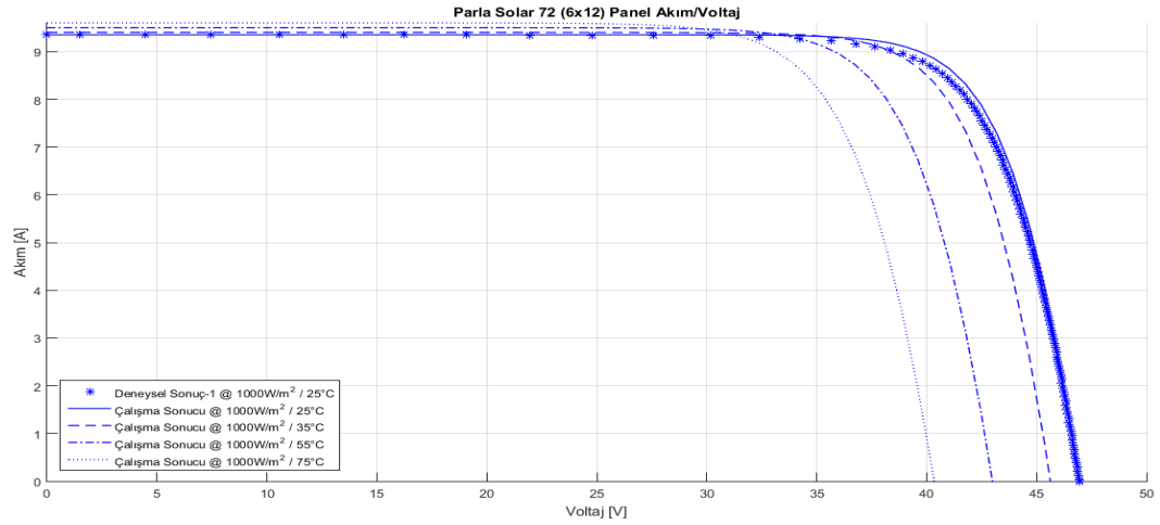
Şekil 5.64: Parla Solar 2 Full Cell Panel (I-V) Grafiği (G=1000 W/m²)
