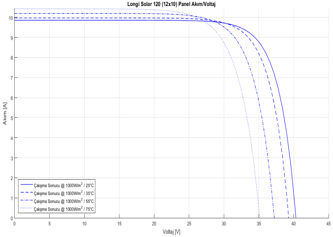
Şekil 5.43: Longi Solar Longi Mono Perc Half Cut 310W Panel (I-V) Grafiği (G=1000 W/m²)
