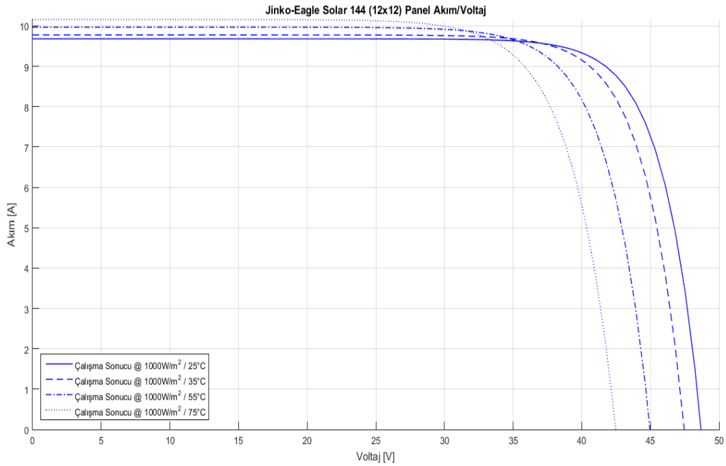
Şekil 5.23: Jinko- EaglePercMono Half Cell JKM370-390M-72H-A1-En Panel (I-V) Grafiği (G=1000 W/m²)
