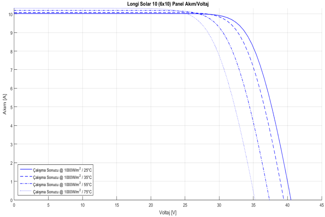
Şekil 5.38: Longi Solar Longi Mono Perc 310W Panel (I-V) Grafiği (G=1000 W/m²)
