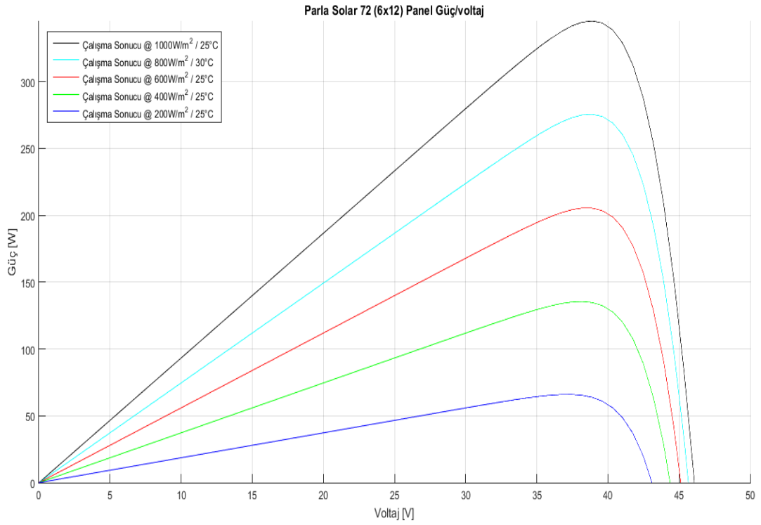
Şekil 5.46: Parla Solar (5-Mono-72) Panel (P-V) Grafiği (T=25 °C)
