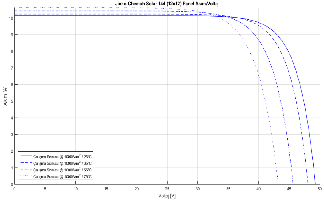
Şekil 5.9: Jinko-Cheetah Solar Cheetahperc Half Cell JKM380-400M-72H-A1-EN Panel (I-V) Grafiği (G=1000 W/m 2 )
