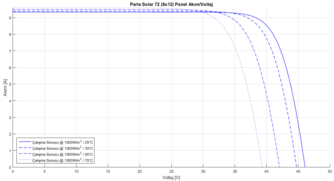
Şekil 5.48: Parla Solar (5-Mono-72) Panel (I-V) Grafiği (G=1000 W/m²)
