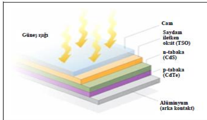
Şekil 3.5: Kadmiyum Tellur PV Hücresi Yapısı (Alkan, 2016)
