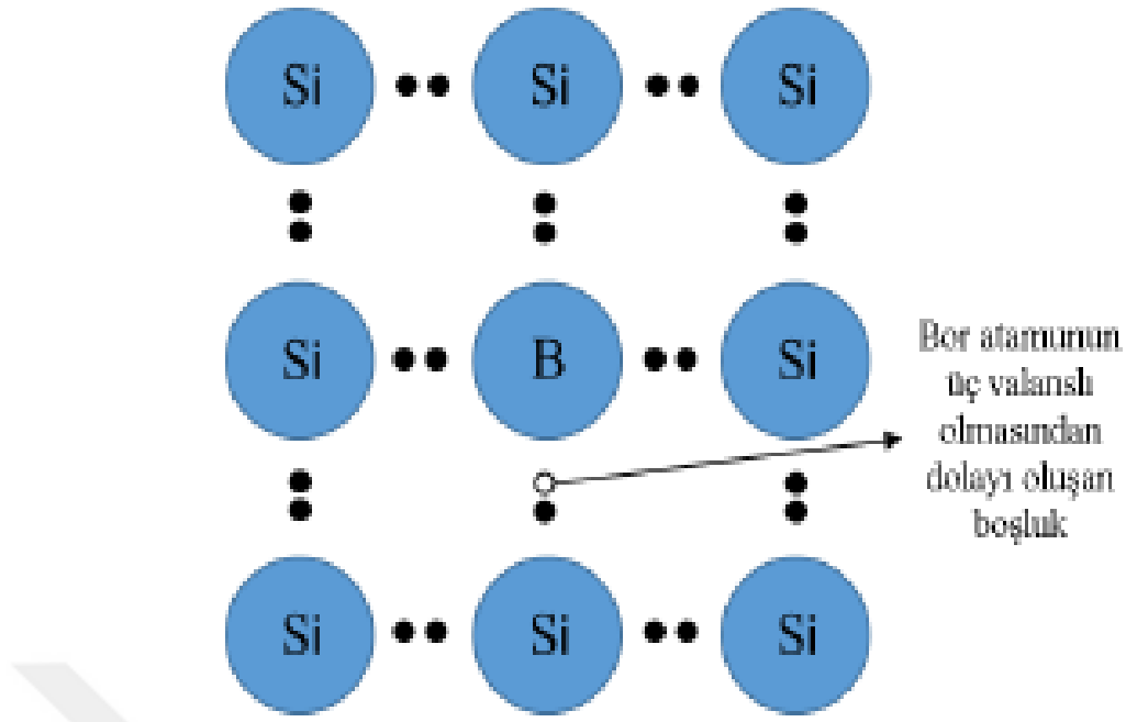
Şekil 2.12: p-Tipi Katkılama (Dalkılıç, 2019)
