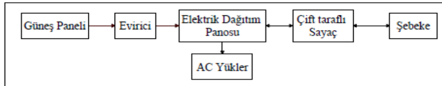
Şekil 3.12: Şebekeye Bağlı (On-Grid) PV Sistem Şematik Gösterimi (Alkan, 2016).
