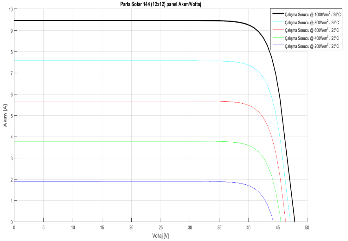
Şekil 5.59: Parla Solar 1 Half Cut Cell Panel (I-V) Grafiği ( T=25^\circ\text{C} )
