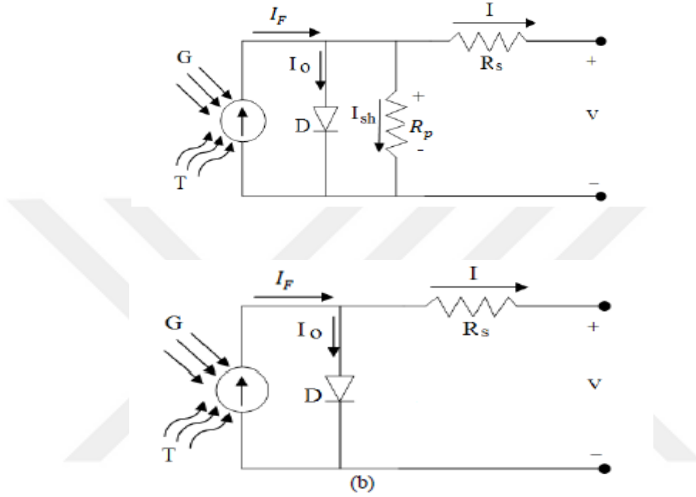
Şekil 4.5: (a) Güneş Hücresi Eşdeğer Devre Modeli (b) Basitleştirilmiş Eşdeğer Devre Modeli (Şahin ve Okumuş, 2013).
