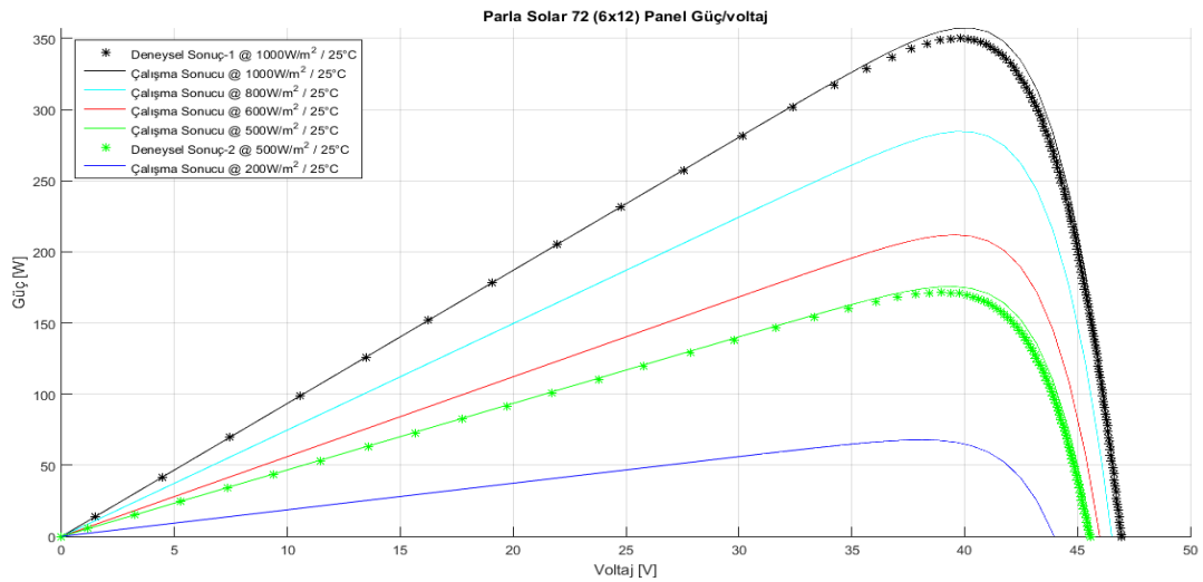
Şekil 5.62: Parla Solar 2 Full Panel (P-V) Grafiği (T=25 °C)
