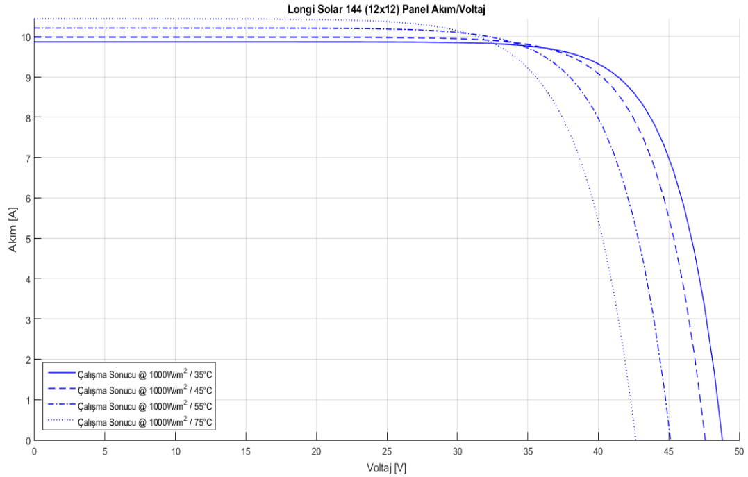
Şekil 5.33: Longi Solar LR6-72HPH Perc Half Mono365-385M Panel (I-V) Grafiği (G=1000 W/m²)
