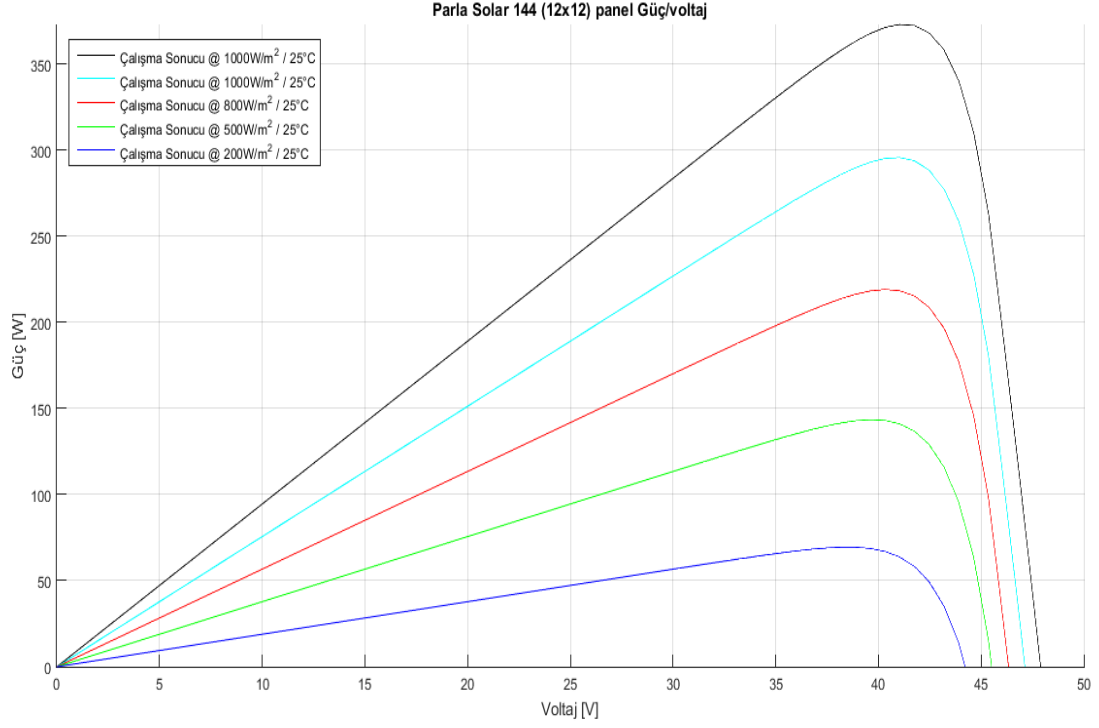
Şekil 5.58: Parla Solar 1 Half Cut Cell Panel (P-V) Grafiği ( T=25^\circ\text{C} )
