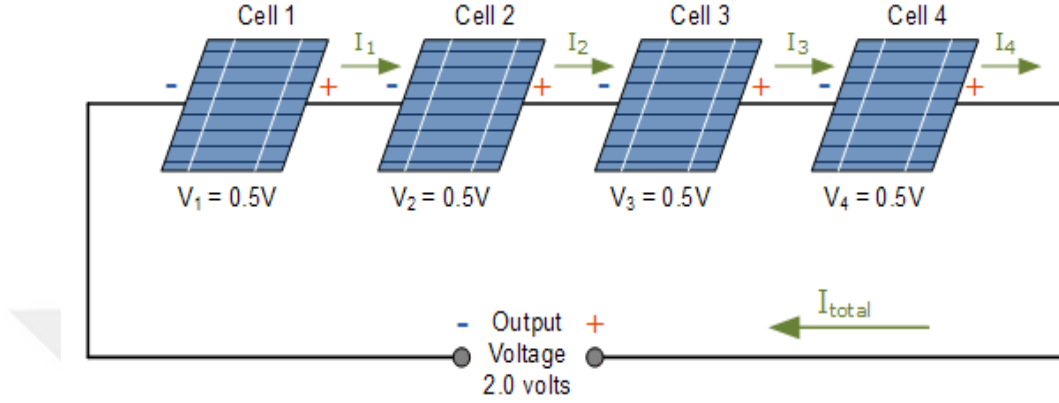
Şekil 3.10: Seri Bağlı Güneş Hücreleri (Url-14, 2014)
