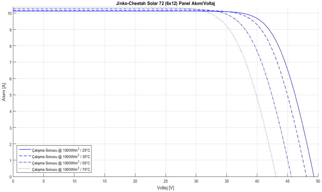
Şekil 5.4: Jinko-Cheetah Solar Panel (I-V) Grafiği (G=1000 W/m²)
