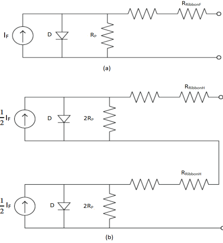
Şekil 4.2: (a) Tam Bir Hücreden Oluşan Hücre Modeli (b) Seri Bağlı İki Yarı Kesik Hücreden Oluşan Hücre Modeli (Guo ve diğ., 2013).
