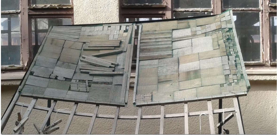
Resim 4.8. Dış ortam şartlarında 1 yıl süreyle bekletilen deney örneklerinin 45° eğik konumda standartlara yerleştirilmesi
