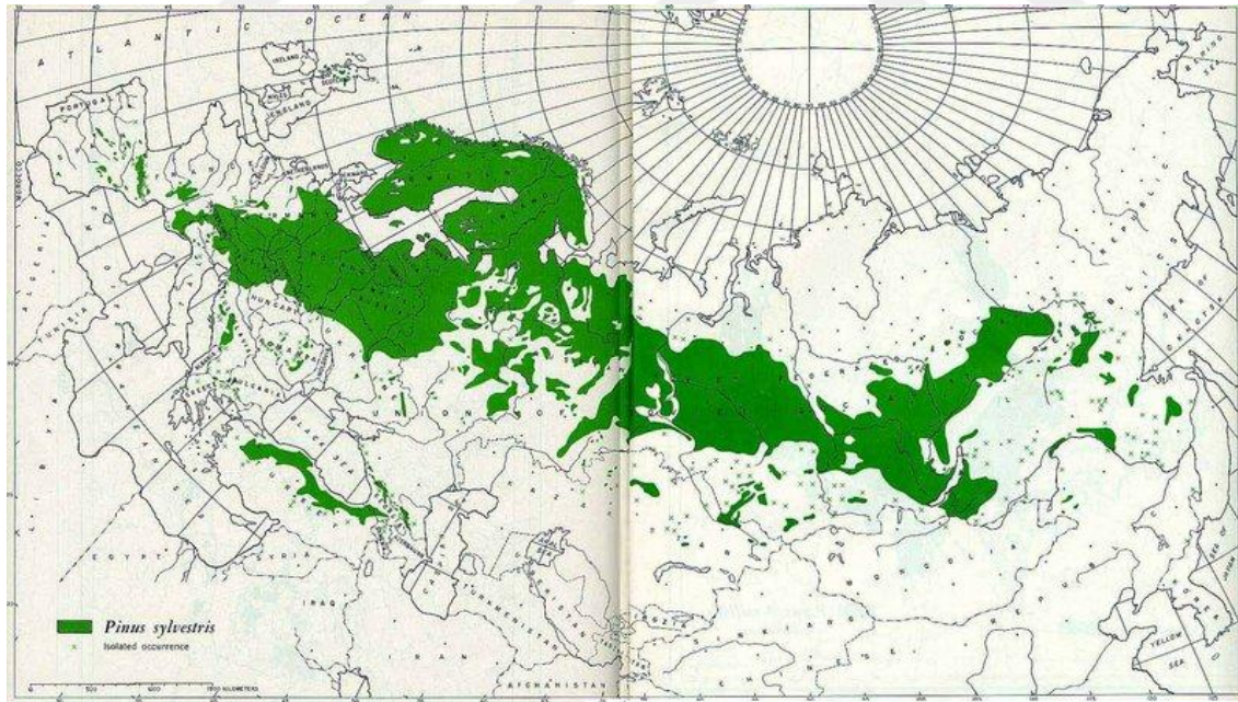
Harita 3.1. Dünyadaki Sarıçam yayılışı
