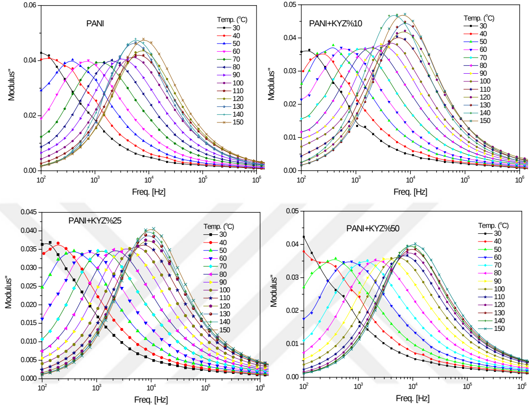
Şekil 3.12 Frekansa bağlı sanal elektriksel modulus grafiği; a) PANI, b) PANI+%10 KYZ13, c) PANI+%25 KYZ13, d) PANI+%50 KYZ13.
