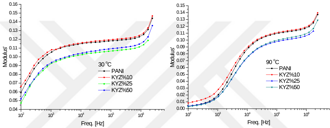
Şekil 3.11 Frekansa bağı reel elektriksel modulusun farklı sıcaklıklardaki grafiğı; a) 30°, b) 90°.
