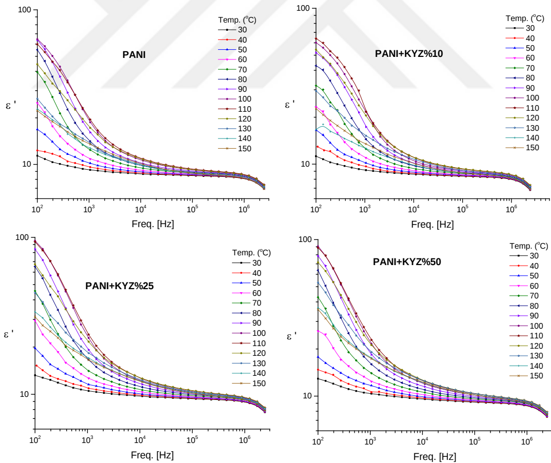
Şekil 3.6 Frekansa bağlı reel dielektrik sabitinin değişim grafiği; a) PANI, b) PANI+%10 KYZ13, c) PANI+%25 KYZ13, d) PANI+%50 KYZ13.
