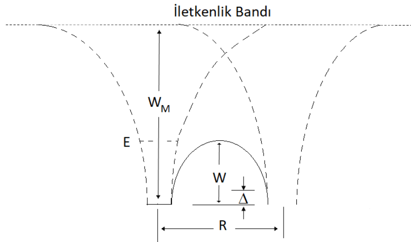
Şekil 2.6 R mesafesindeki bir taşıyıcının deneyle bağdaşmış potansiyeli
