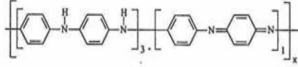
Protoemeraldin bazı
