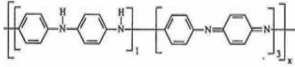
Nigranilin bazı
