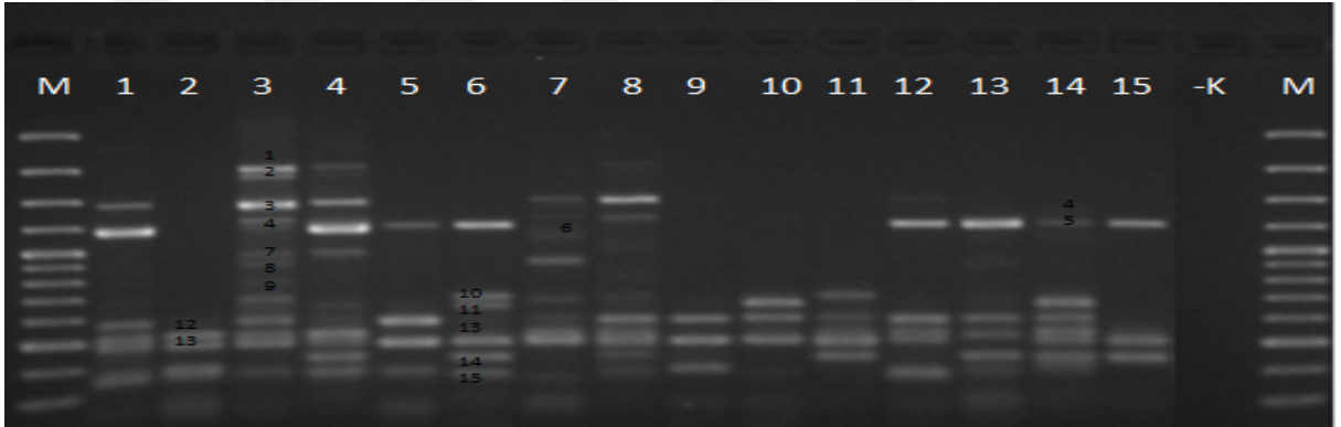
Şekil 4. 14. UBC 840 primeri ile tescil edilmiş tritikale çeşitlerinin ISSR-PCR bant profilleri
