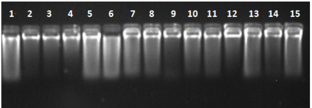
Şekil 3. 1. Tescilli Tritikale Çeşitlerine Ait DNA Jel Elektroforez Görüntüleri
