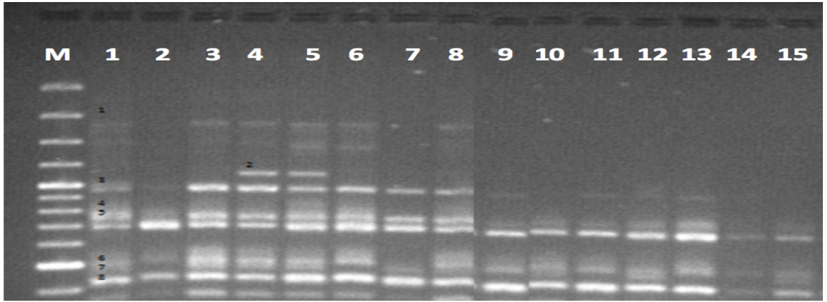
Şekil 4. 2. UBC 810 primeri ile tescil edilmiş tritikale çeşitlerinin ISSR-PCR bant profilleri
