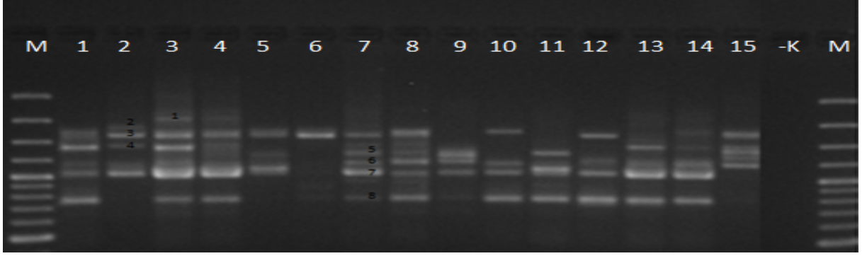
Şekil 4. 6. UBC 820 primeri ile tescil edilmiş tritikale çeşitlerinin ISSR-PCR bant profilleri
