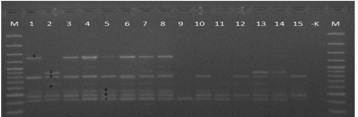
Şekil 4. 8. UBC 824 primeri ile tescil edilmiş tritikale çeşitlerinin ISSR-PCR bant profilleri
