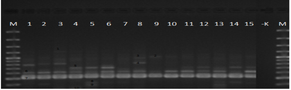
Şekil 4. 13. UBC 835 primeri ile tescil edilmiş tritikale çeşitlerinin ISSR-PCR bant profilleri
