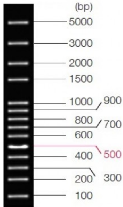
Şekil 3. 2. 100 bp plus DNA marker
