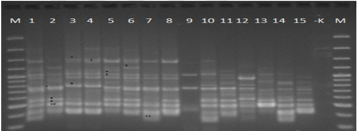
Şekil 4. 16. UBC 847 primeri ile tescil edilmiş tritikale çeşitlerinin ISSR-PCR bant profilleri
