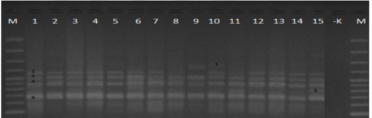
Şekil 4. 5. UBC 818 primeri ile tescil edilmiş tritikale çeşitlerinin ISSR-PCR bant profilleri
