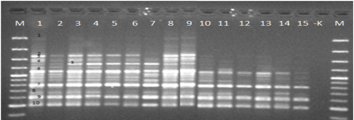
Şekil 4. 10. UBC 827 primeri ile tescil edilmiş tritikale çeşitlerinin ISSR-PCR bant profilleri
