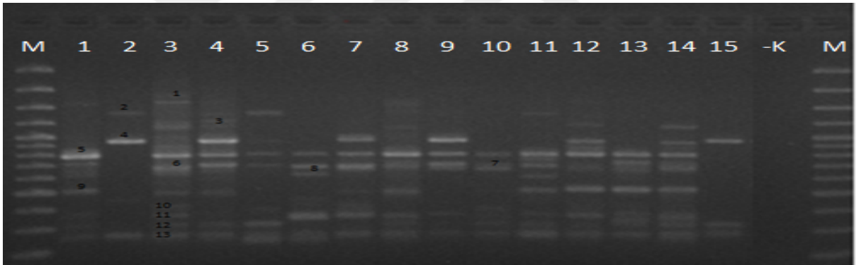
Şekil 4. 12. UBC 834 primeri ile tescil edilmiş tritikale çeşitlerinin ISSR-PCR bant profilleri
