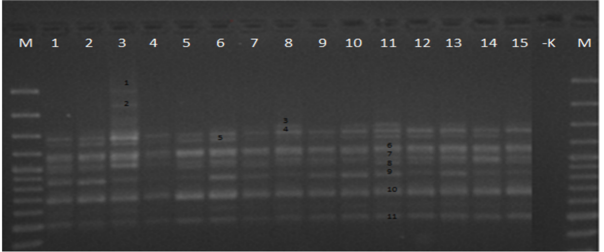
Şekil 4. 4. UBC 813 primeri ile tescil edilmiş tritikale çeşitlerinin ISSR-PCR bant profilleri
