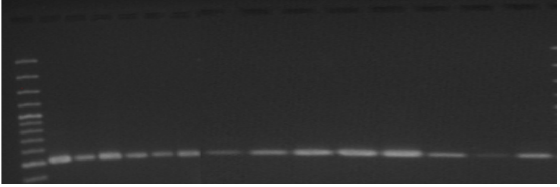
Şekil 4. 17. UBC 809 primeri ile tescilli tritikale çeşitlerinin ISSR-PCR bant profilleri
