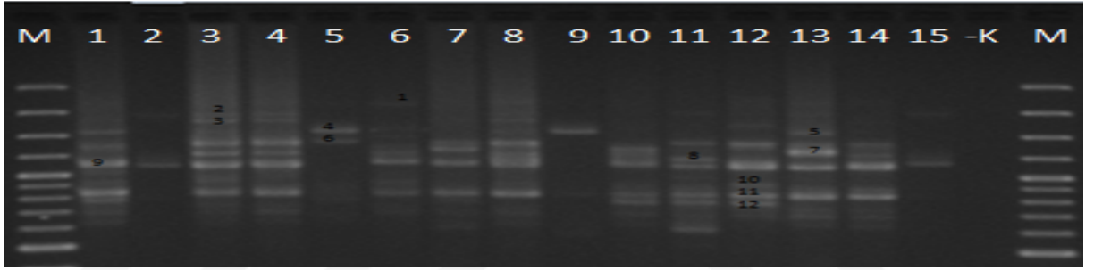
Şekil 4. 7. UBC821 primeri ile tescil edilmiş tritikale çeşitlerinin ISSR-PCR bant profilleri
