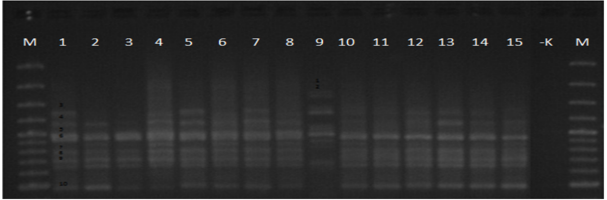
Şekil 4. 9. UBC 826 primeri ile tescil edilmiş tritikale çeşitlerinin ISSR-PCR bant profilleri
