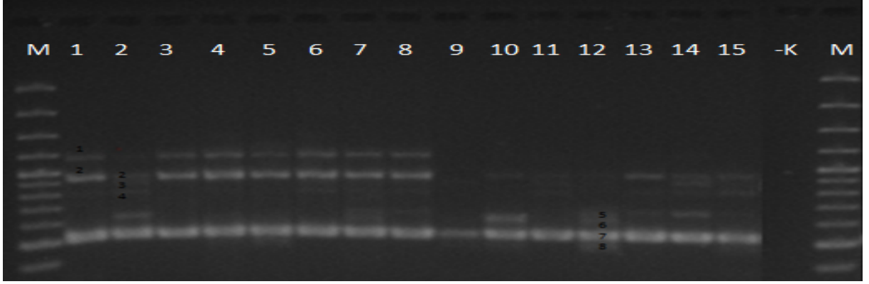
Şekil 4. 15. UBC 844 primeri ile tescil edilmiş tritikale çeşitlerinin ISSR-PCR bant profilleri
