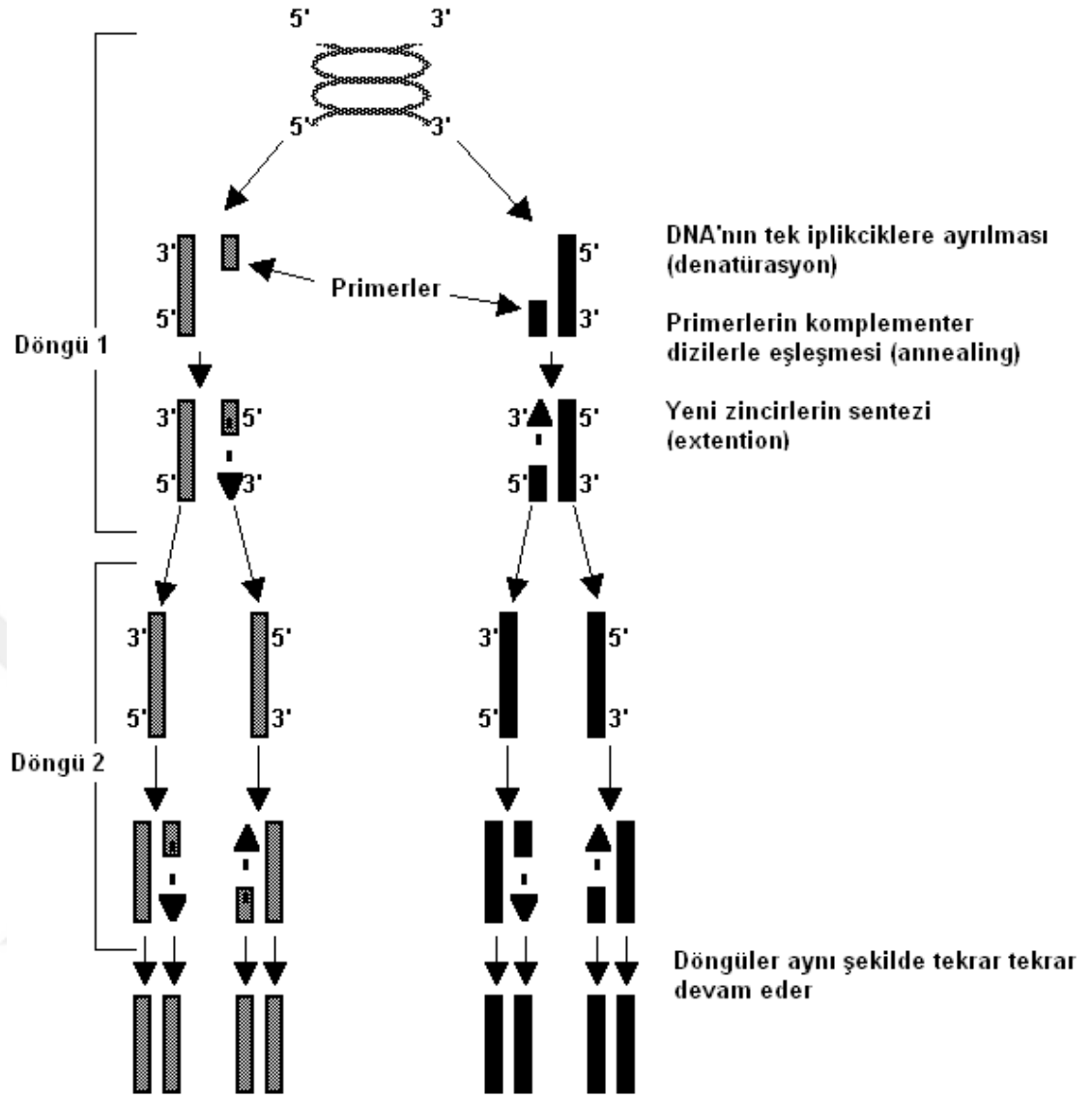
Şekil 1. 1. PCR çalışma prensibi
