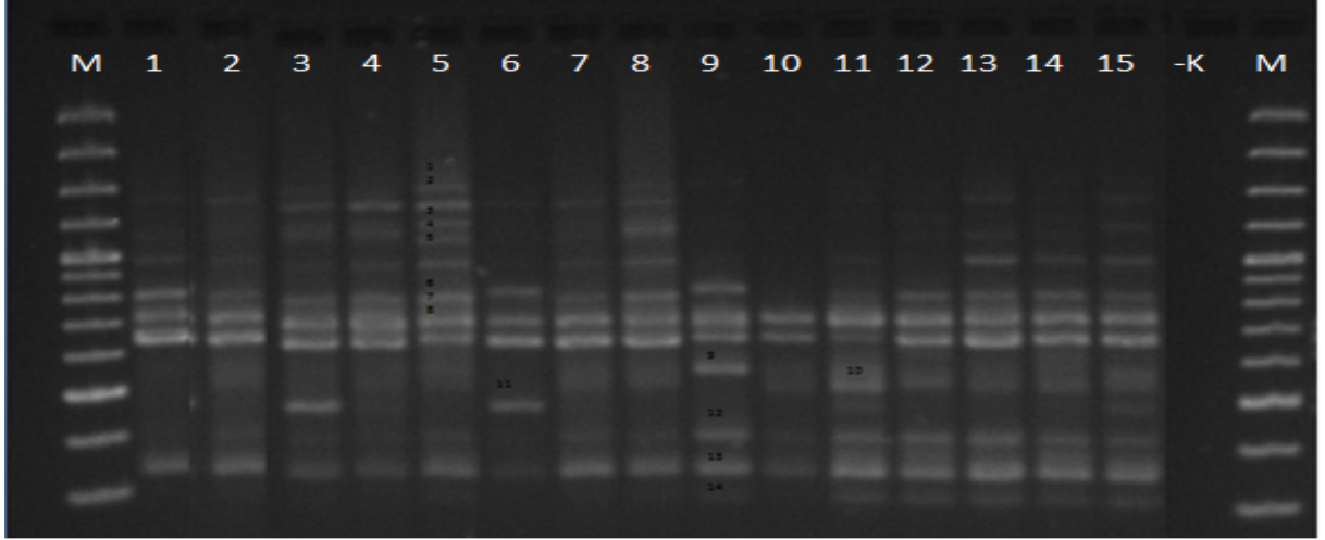
Şekil 4. 11. UBC 830 primeri ile tescil edilmiş tritikale çeşitlerinin ISSR-PCR bant profilleri
