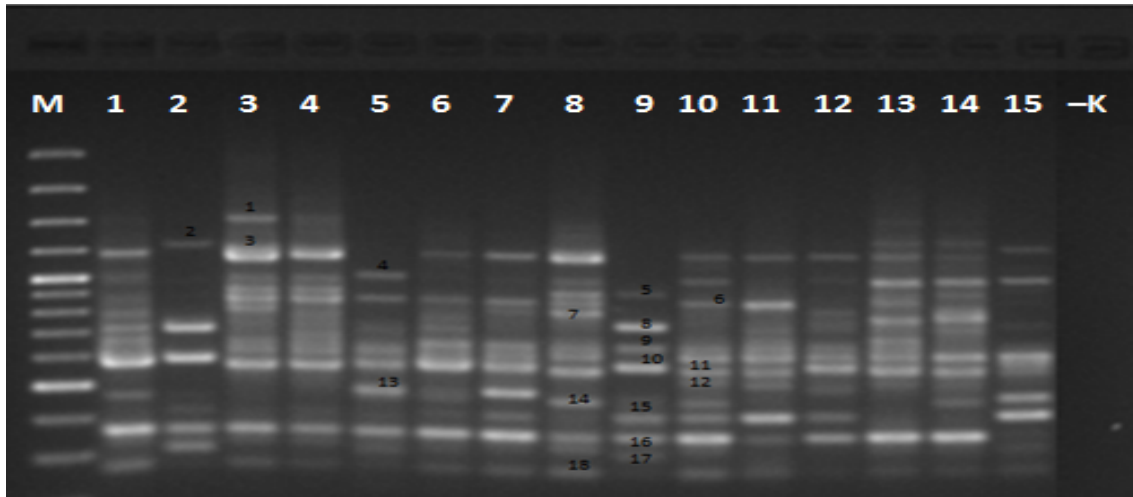
Şekil 4. 1. UBC 808 primeri ile tescil edilmiş tritikale çeşitlerinin ISSR-PCR bant profilleri
