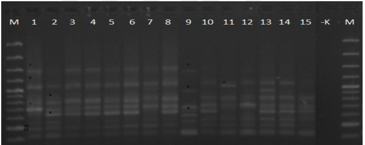
Şekil 4. 3. UBC 812 primeri ile tescil edilmiş tritikale çeşitlerinin ISSR-PCR bant profilleri
