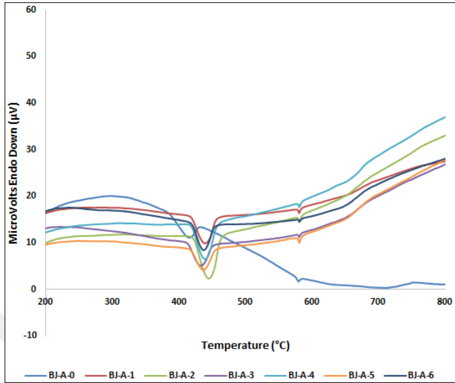
Şekil C-3.1 Borjips ve nano-Al 2 O 3 ieren harlara ait DTA sonuları
