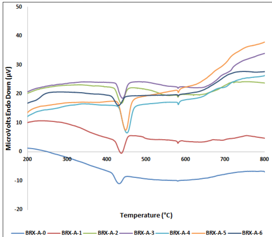
Şekil C-3.2 Boraks atıėı ve nano-Al 2 O 3 ieren harlara ait DTA sonuları
