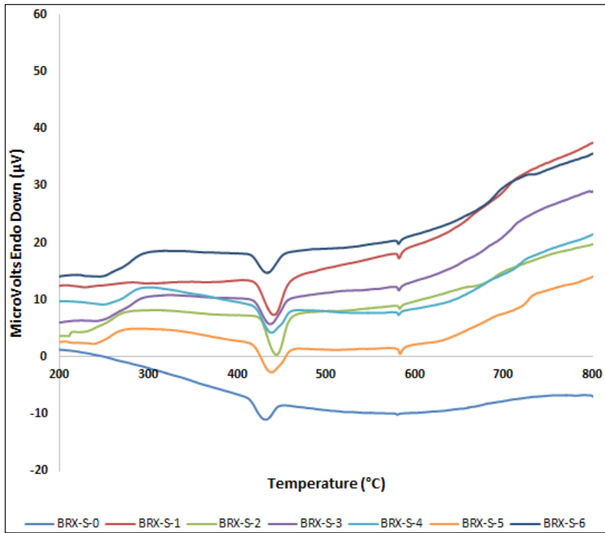
Şekil C-2.2 Boraks atığı ve nano-SiO 2 ieren harlara ait DTA sonuları
