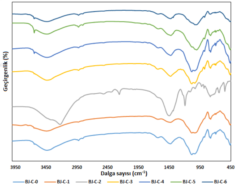
Şekil B-1.1 Borjips ve nano-CuO içeren harların FT-IR spektrumları
