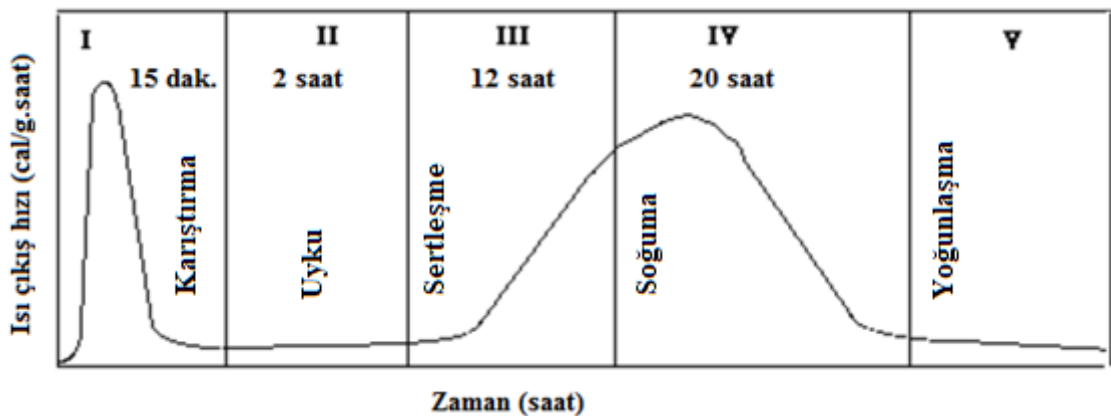
Şekil 2.2 Portland çimentosunun hidratasyonu sırasında ısı çıkış hızı [10]
