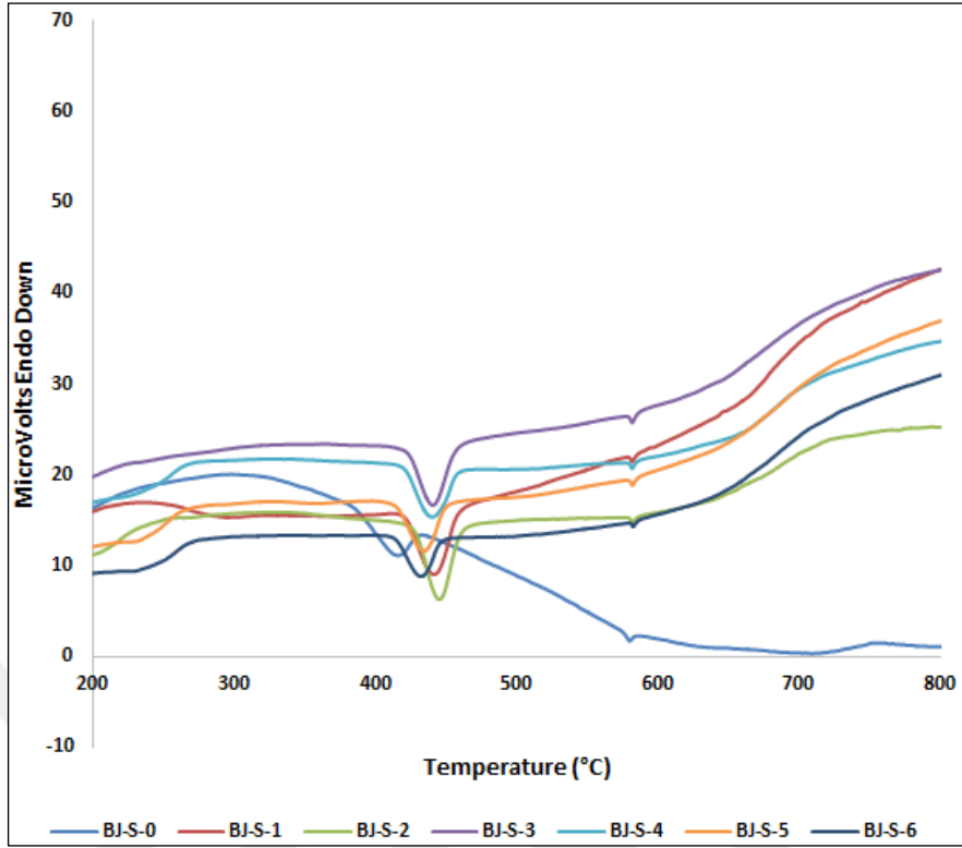
Şekil C-2.1 Borjips ve nano-SiO 2 ieren harlara ait DTA sonuları
