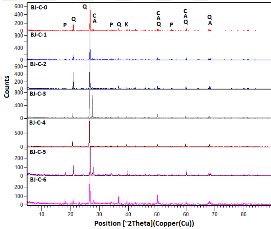
Şekil A-1.1 Borjips ve nano-CuO içeren harçların XRD paternleri
